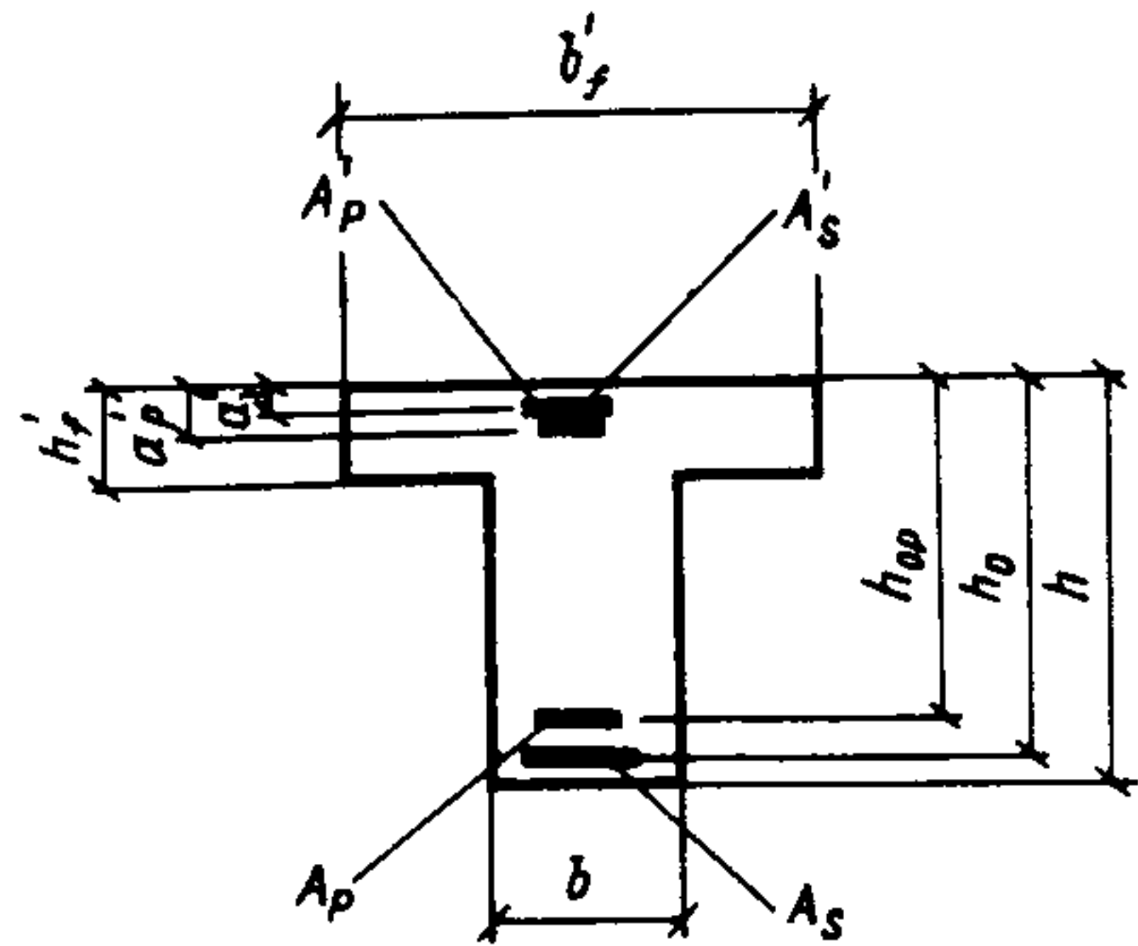
Рис. 5. Расчетная схема поперечного сечения балки
