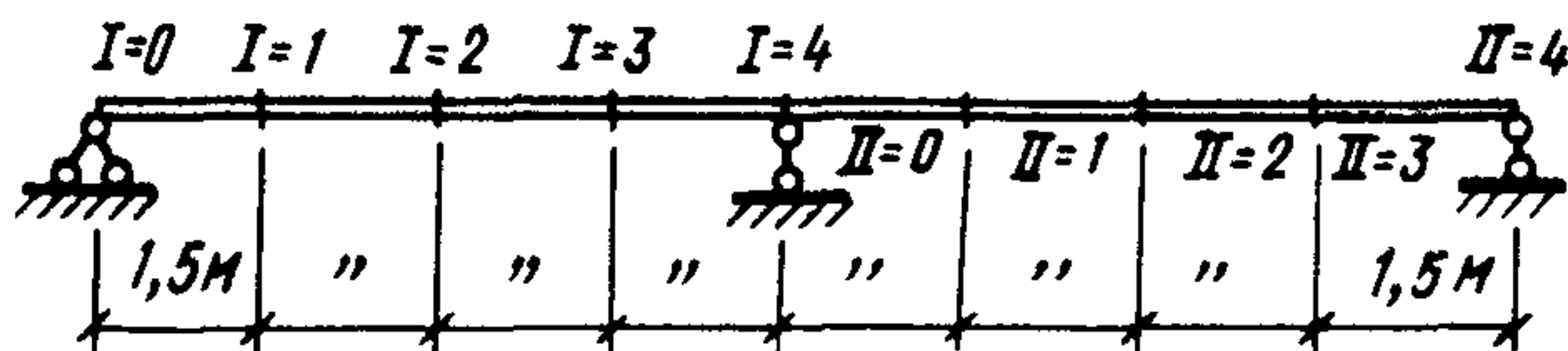
Рис. 8. Схема разбиения балки на участки
