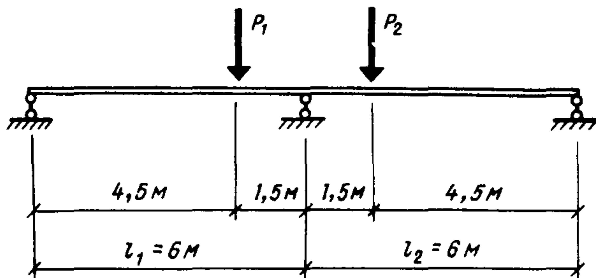
Рис. 7. Схема нагружения балки
