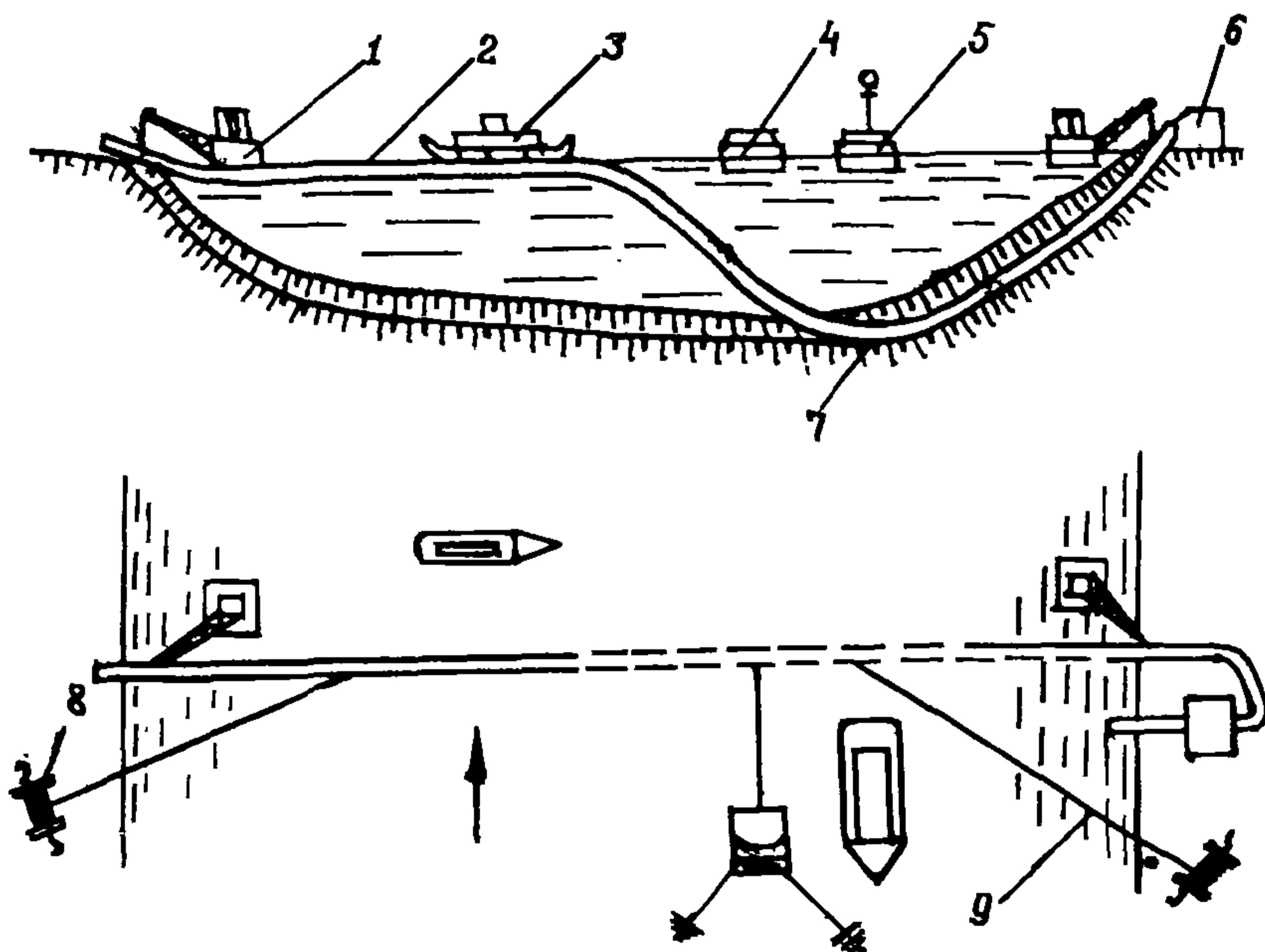
Рис.9. Схема укладки трубопровода способом свободного погружения:
