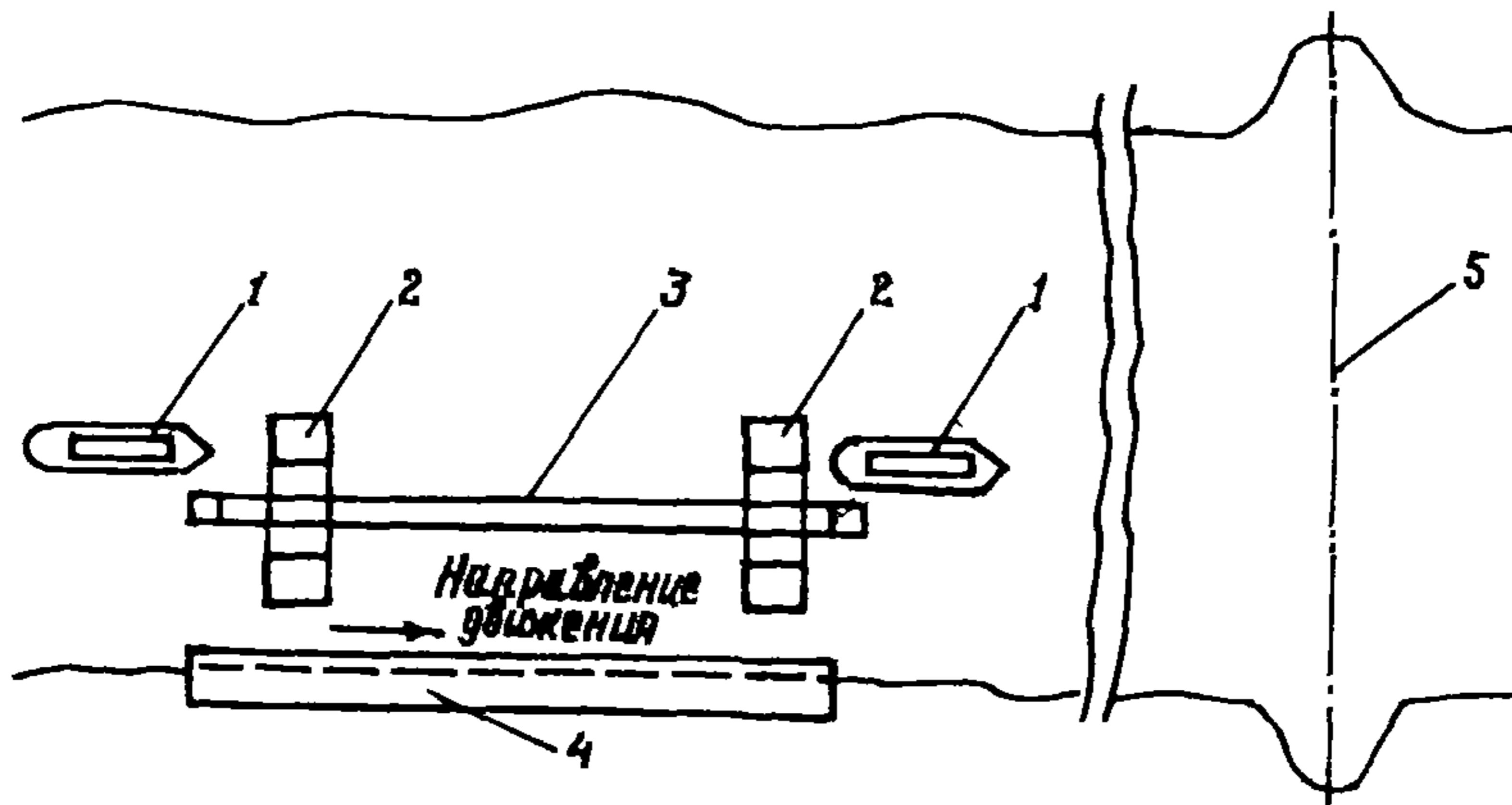
Рис.7. Схема транспортировки трубопровода катерами: 1-буксирные катера; 2-портальные опоры; 3-трубопровод; 4-стапельная площадка; 5-створ перехода
