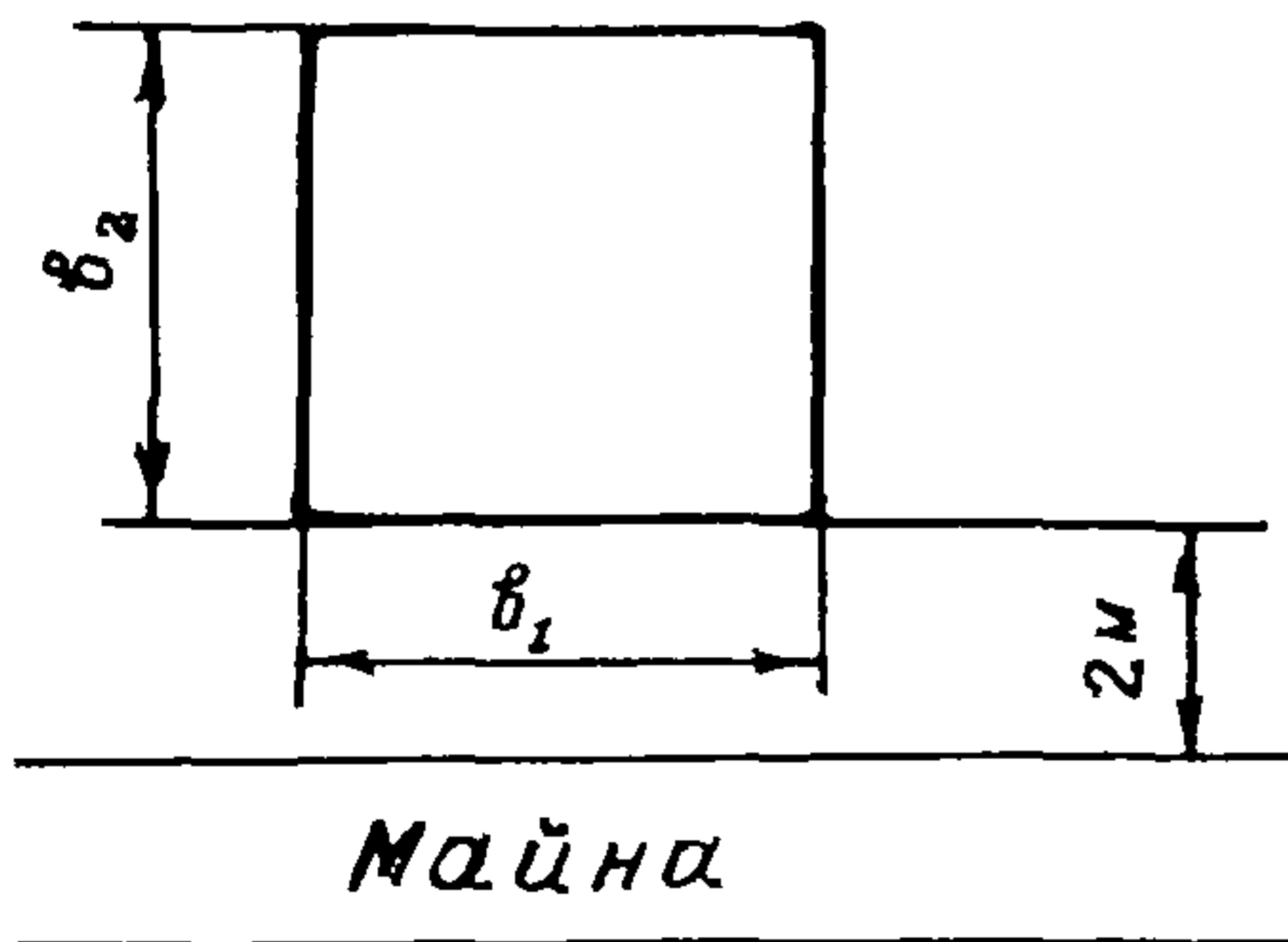
Рис.10. Расчетная схема определения толщины льда:
