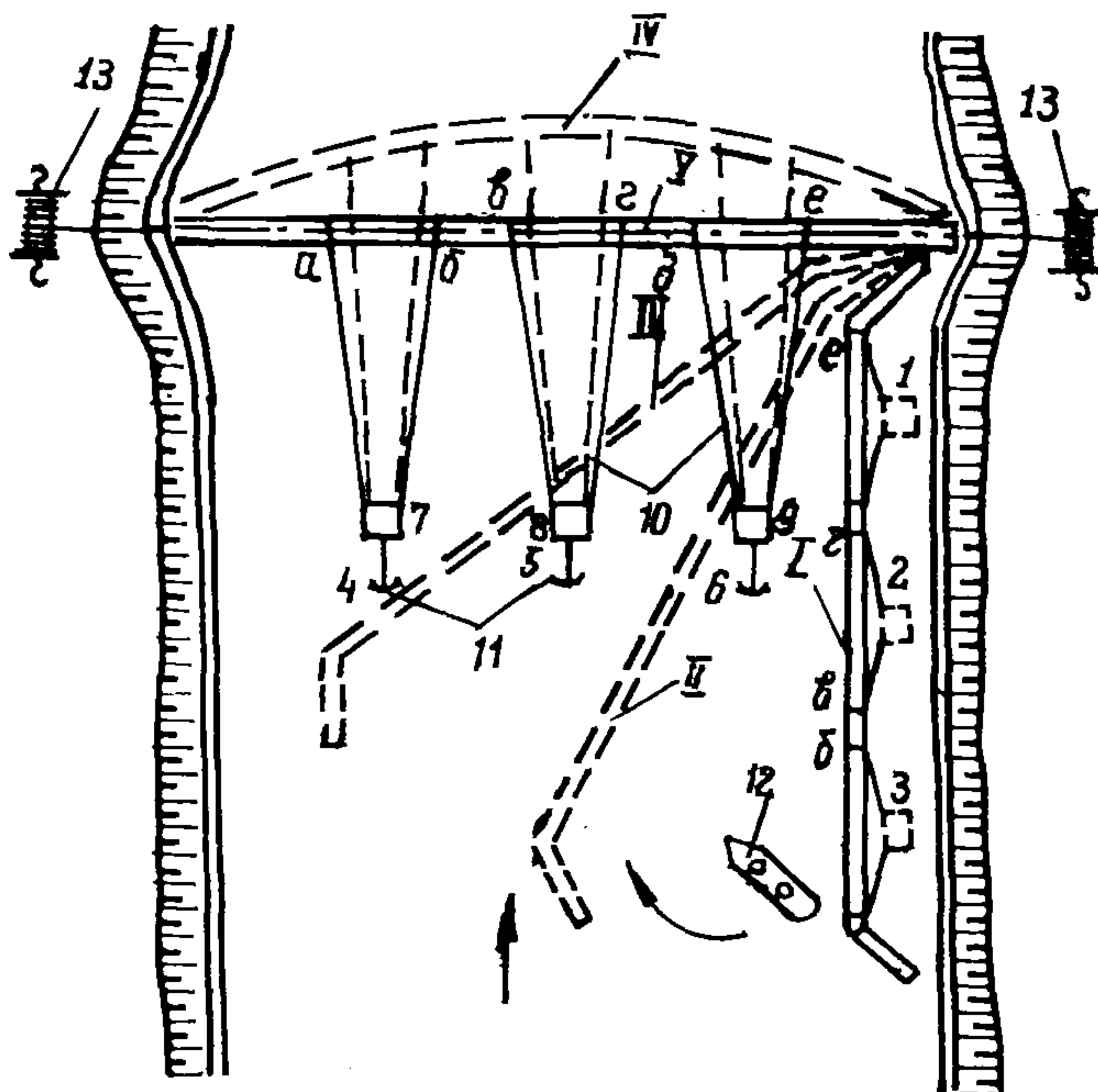
Рис.8. Схема установки трубопровода в створ перехода разворотом на плаву:
