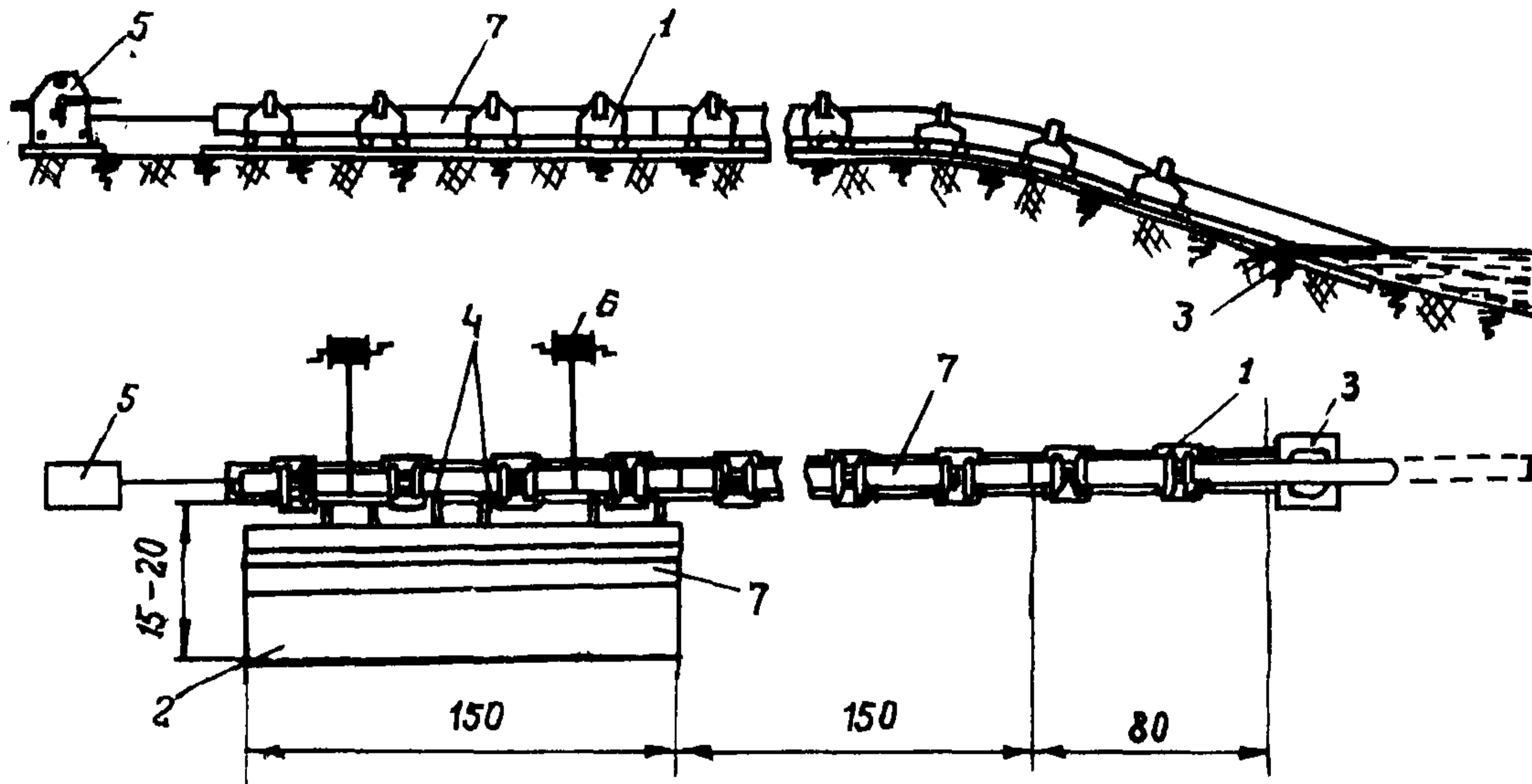
Рис.3. Схема роликовой спусковой дорожки для укладки трубопровода диаметрами I220, I420 мм: 1-роликовые опоры; 2-сталь; 3-приручное спусковое устройство; 4-балки перегружателей; 5-тор- 6-мовная лебедка; 6-устройство для перекаtywания плетей; 7-плеть трубопровода
