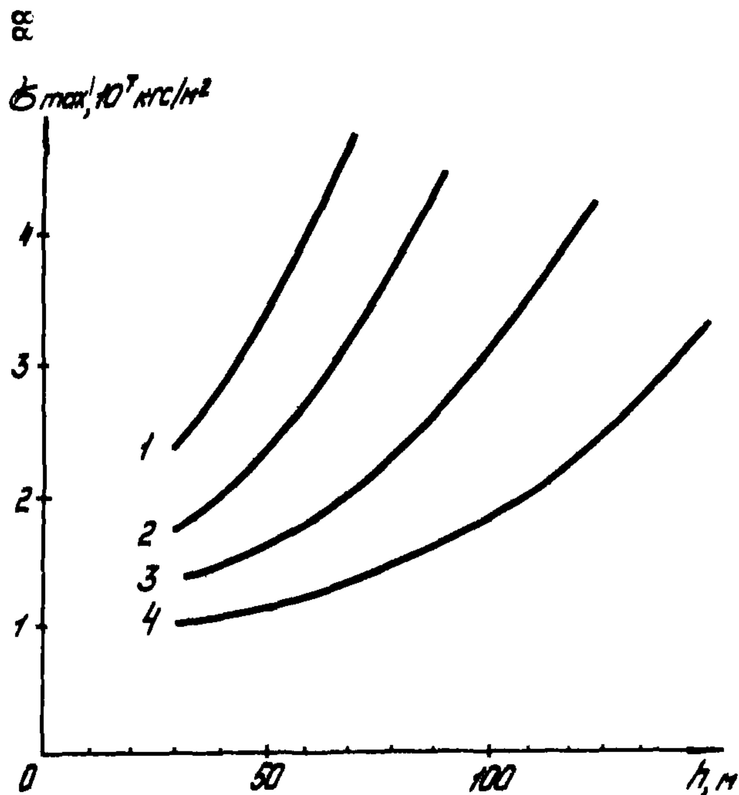
Рис.12. График зависимости максимальных напряжений в нижней части упругого изгиба трубопровода от глубины укладки при различных усилиях натяжения N , тс: 1 - 50; 2 - 100; 3 - 150; 4 - 200
