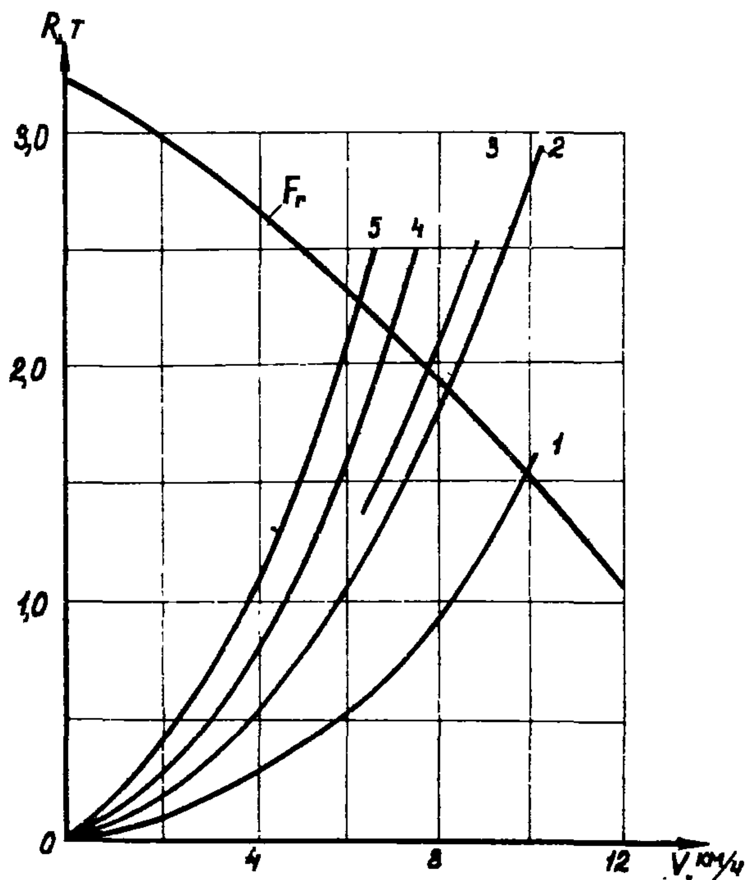
Рис. 10. Графики зависимости буксировочного сопротивления плота от скорости буксировки при различном количестве плетей в плоту n и длине буксирного троса l_{TR} (м):
