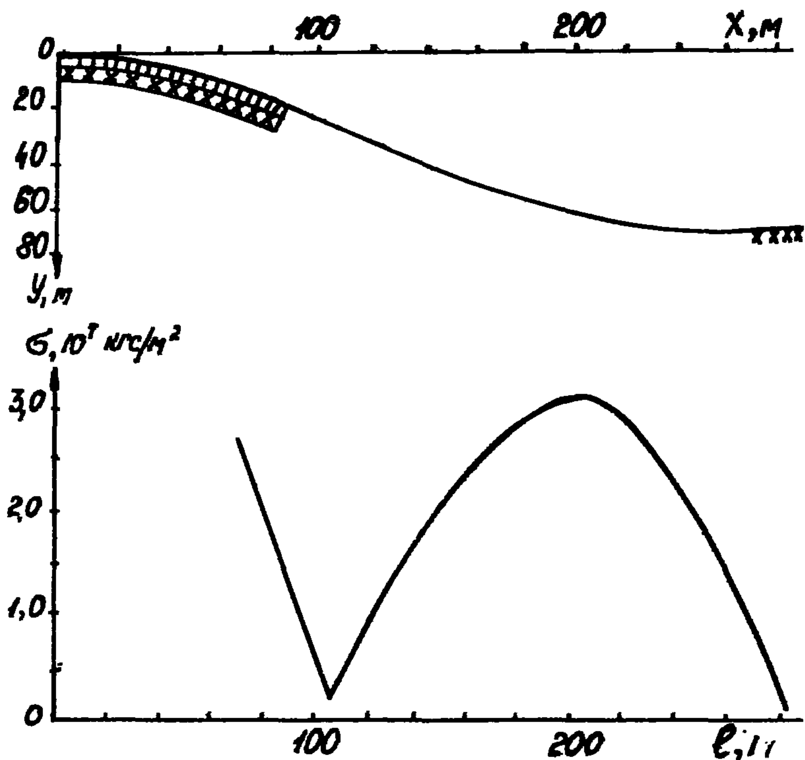
Рис. II. Конфигурация трубопровода и эпюра напряжений ( \sigma ) при укладке на глубину 67 м
