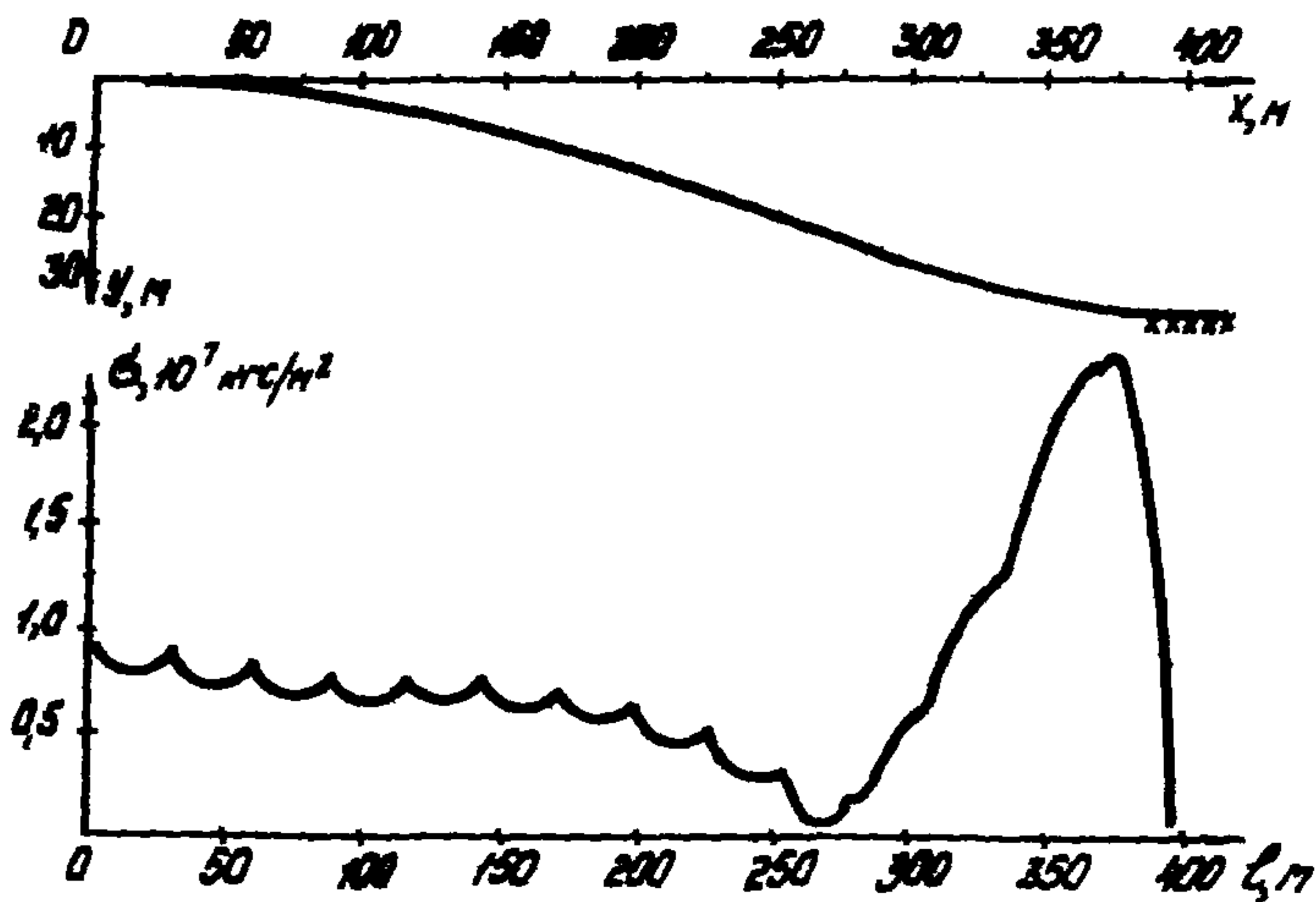
Рис.7. Конфигурация трубопровода и эпюра напряжений ( \sigma ) при укладке свободным погружением
