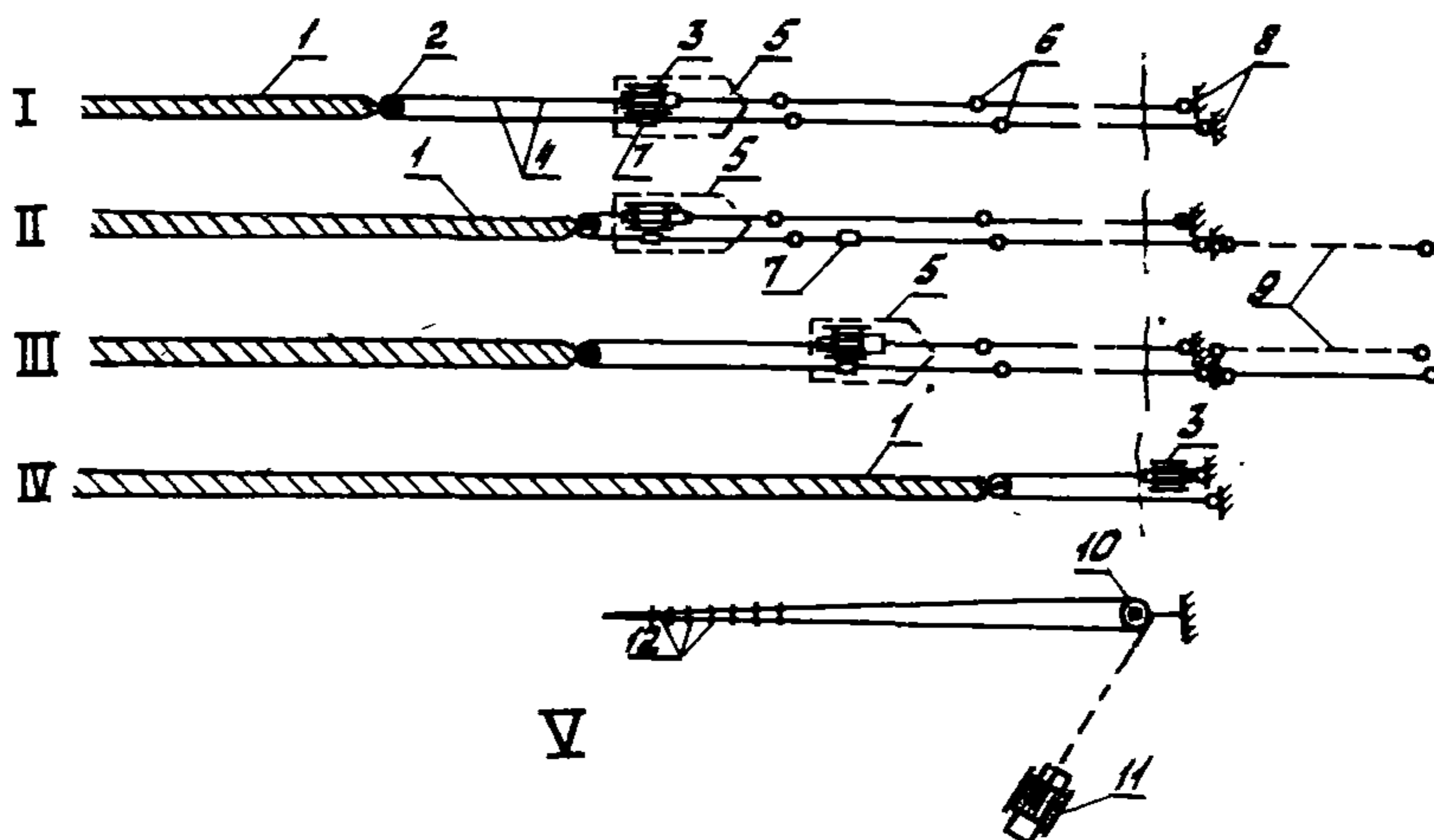
Рис.2. Схема протаскивания трубопровода лебедкой Ш-151, установленной на барже:
