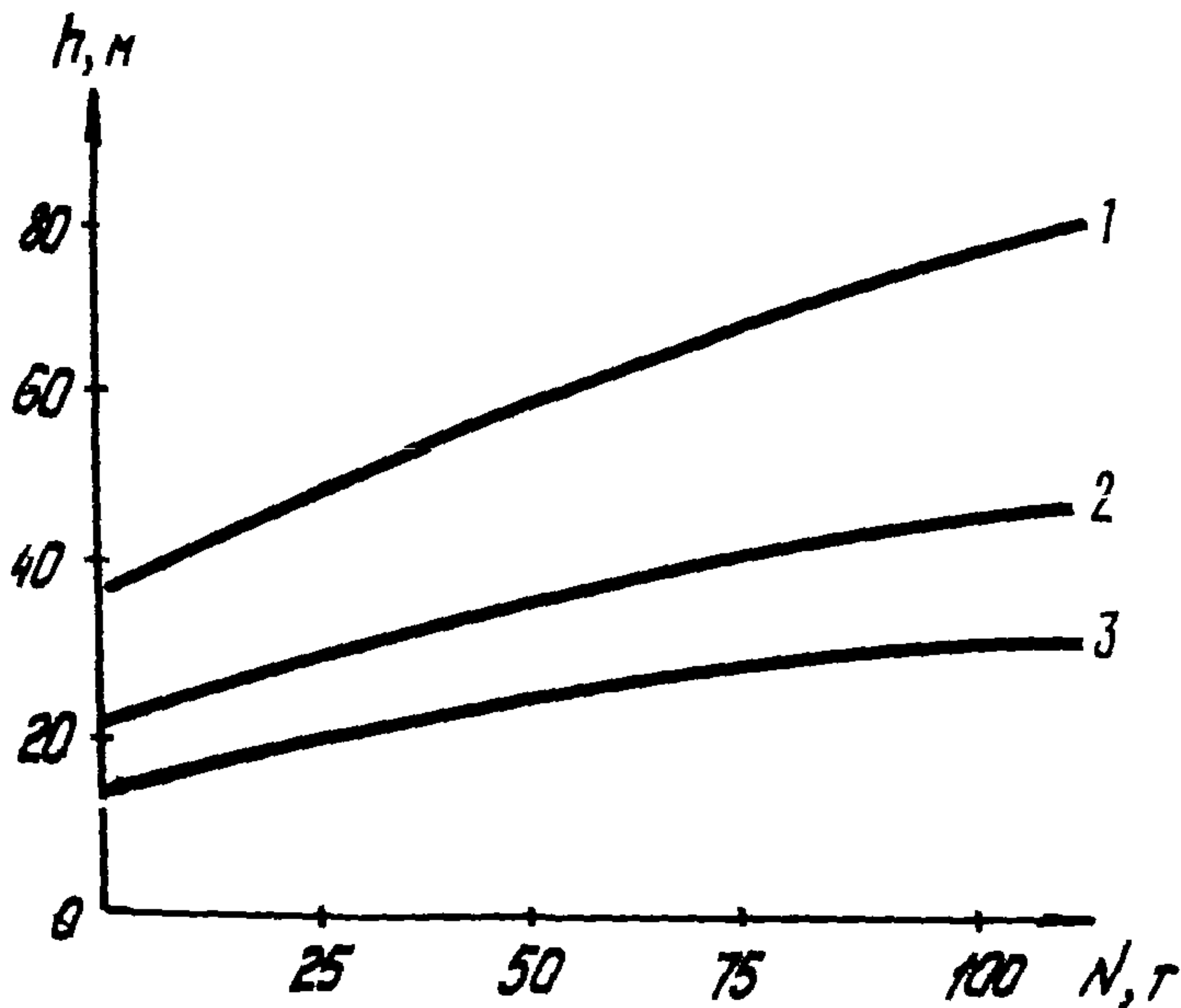
Рис. 9. Графики зависимости h = f(N) при различном запасе плавучести плети P_{пл} (кгс/м): 1 - 29; 2 - 58; 3 - 100
