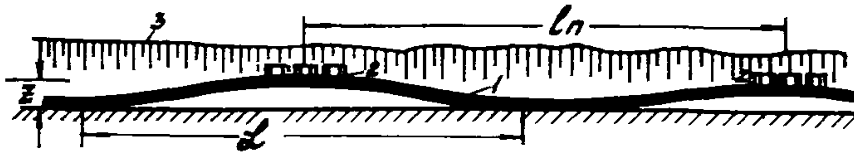
Рис.3. Схема групповой установки понтонов:
