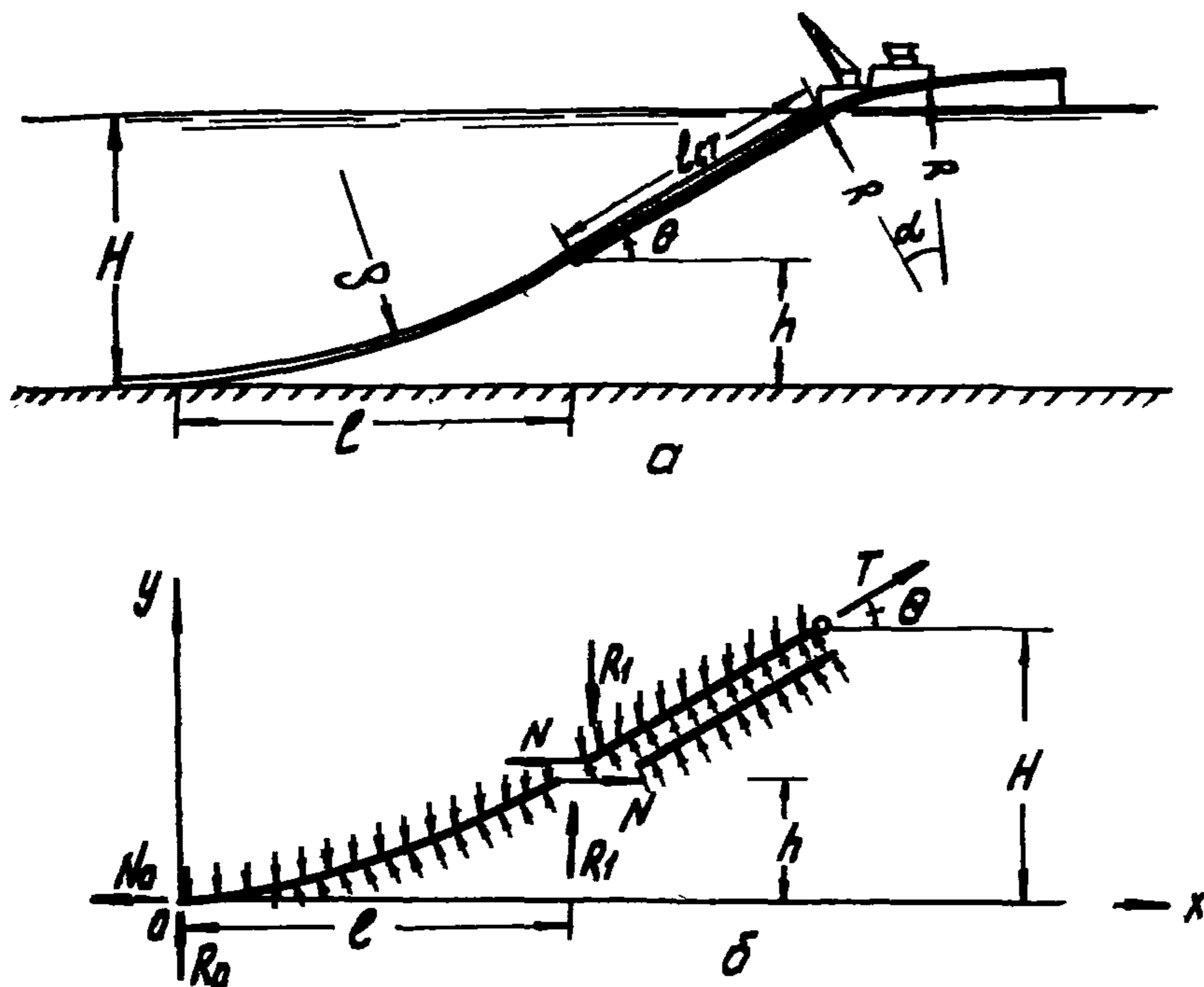
Рис. 7. Схемы укладки трубопровода с трубоукладочной баржи (прямолинейный стингер):
