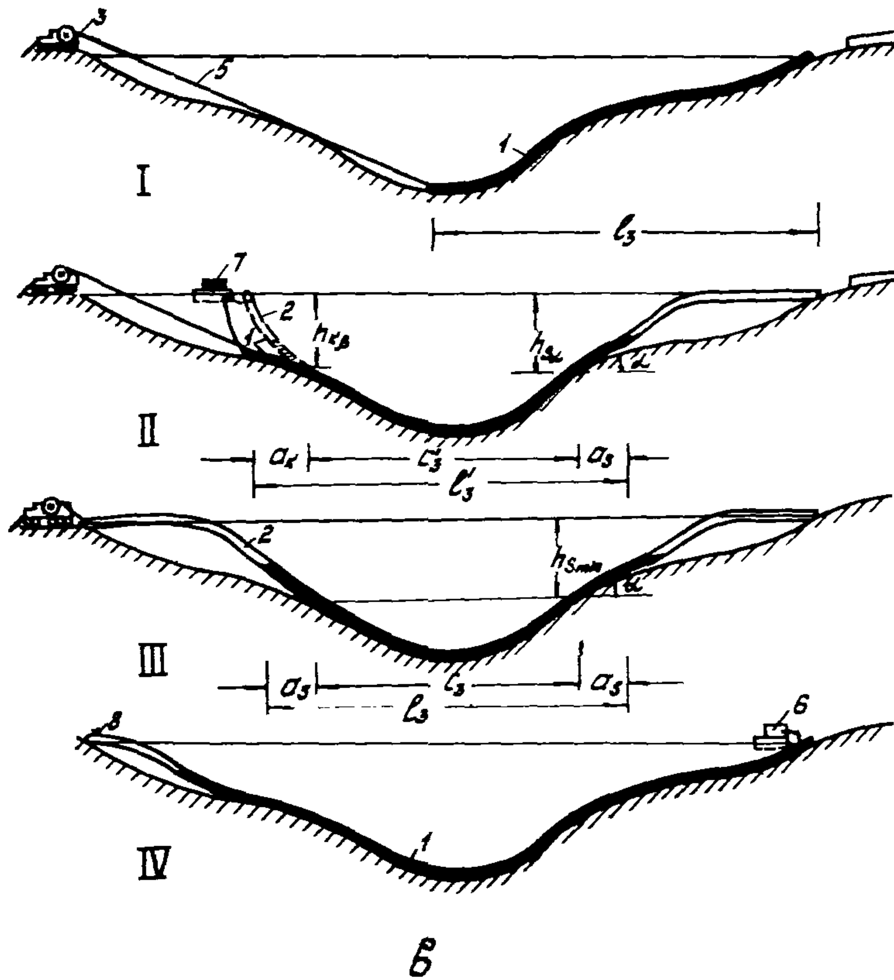
Рис.4. Технологические схемы укладки трубопроводов с регулируемым плавучестью:
