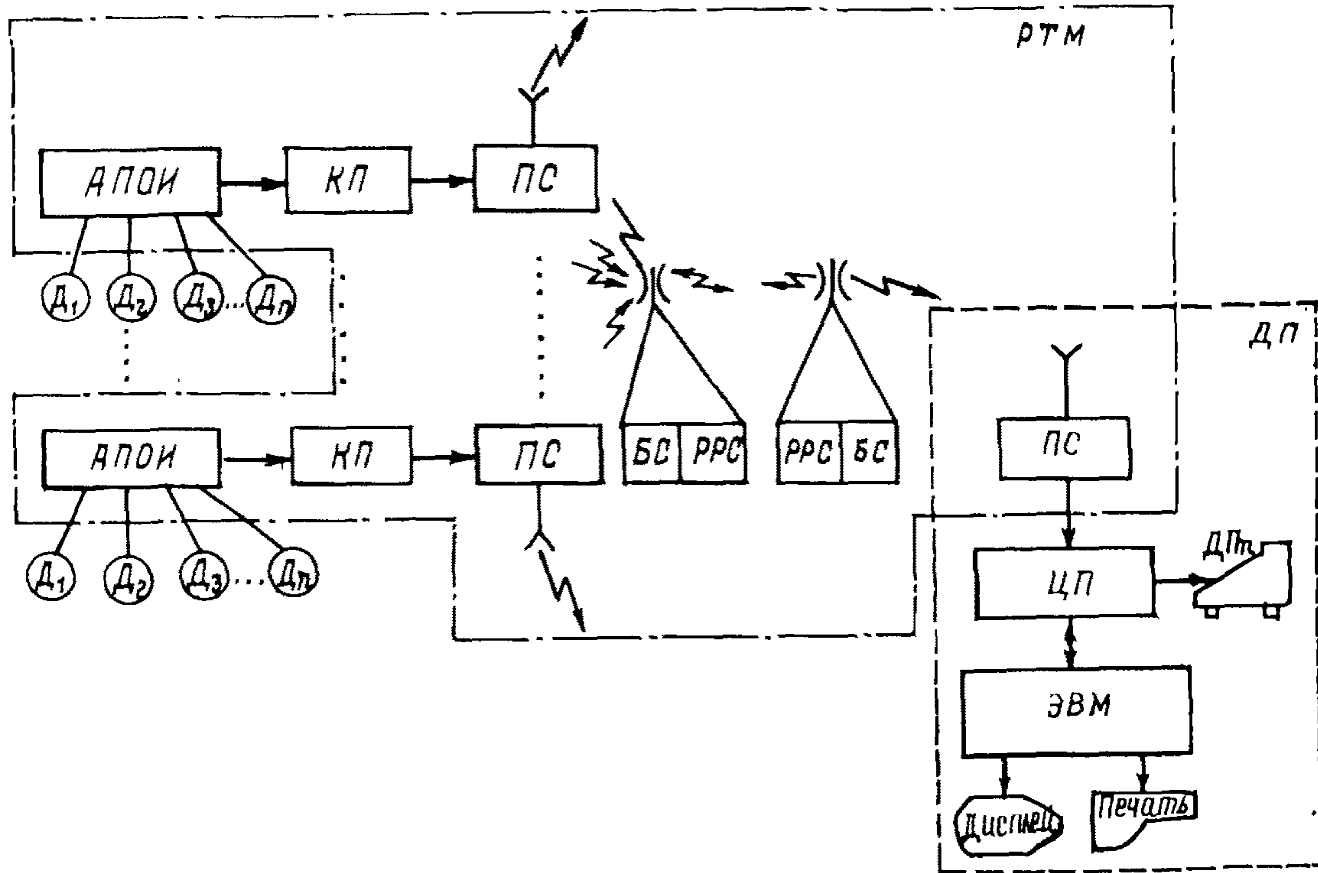
Рис.3. Функциональная схема КТС АСУ ТП:
