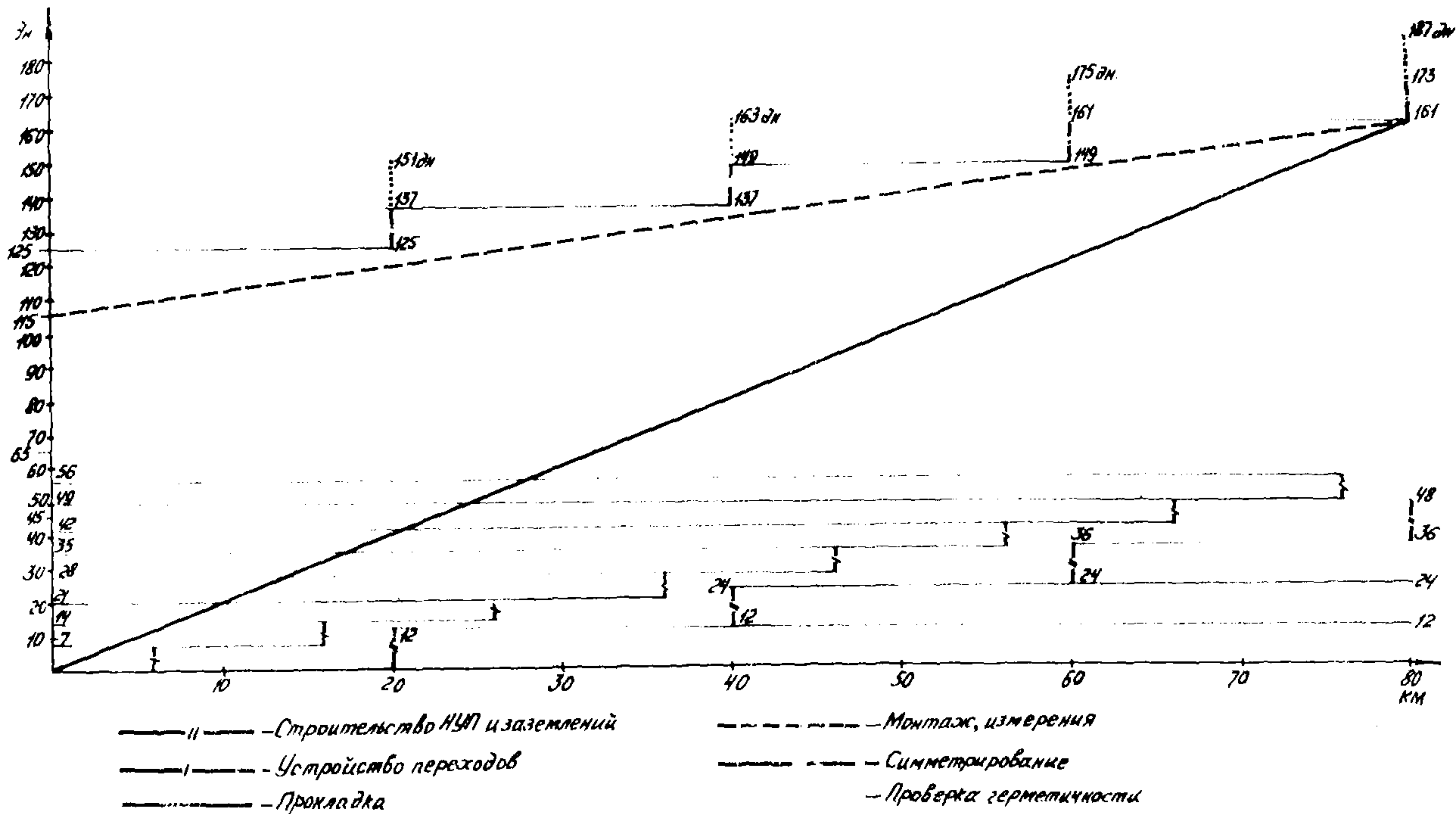
Рис.5. График строительства кабельной линии колонной "малого" типа:
