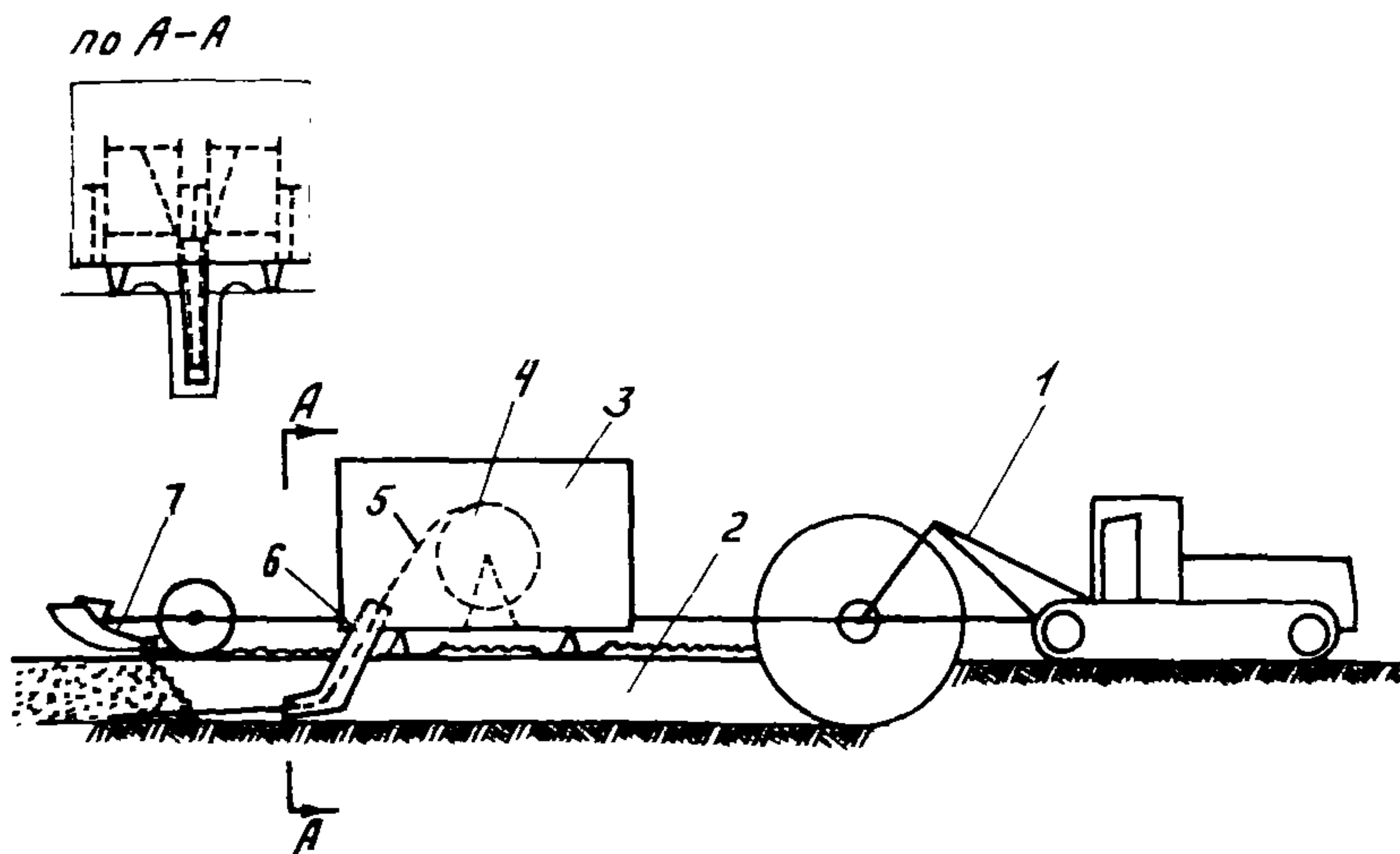
Рис.3. Механизированная колонна "малого" типа:
