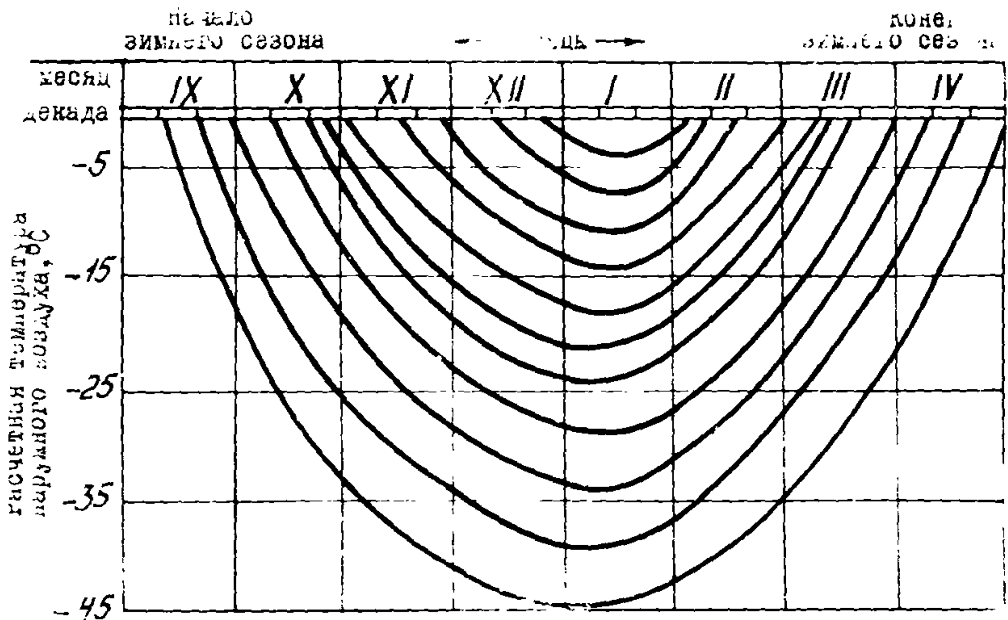
Рис. I. Графики зависимости температуры наружного воздуха от продолжительности зимнего периода
