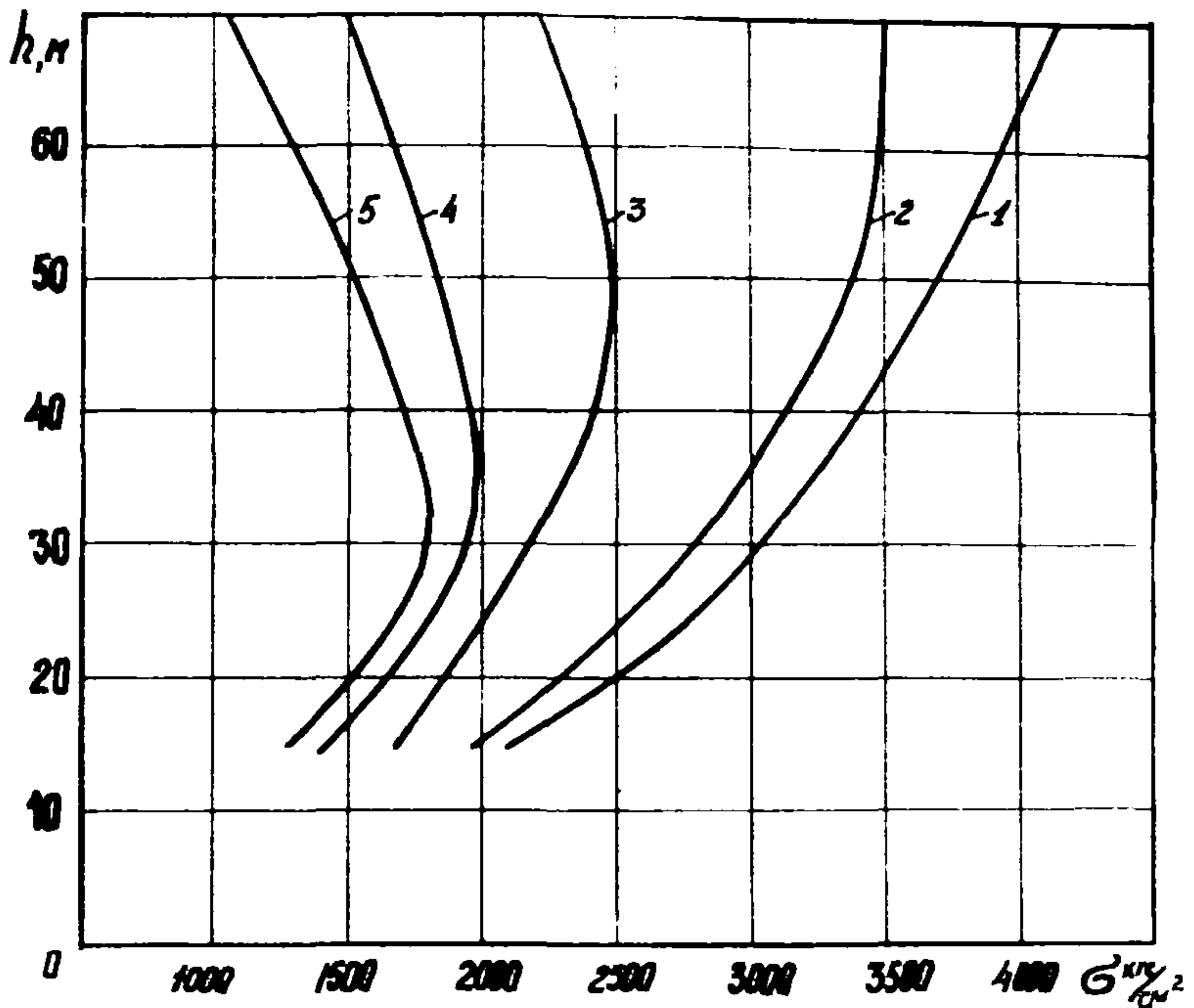
Рис. 22. Зависимость максимальных продольных напряжений на нижнем участке изгиба в трубопроводе диаметром 529 мм с толщиной стенки 10 мм от глубины укладки при различных усилиях натяжения T :
