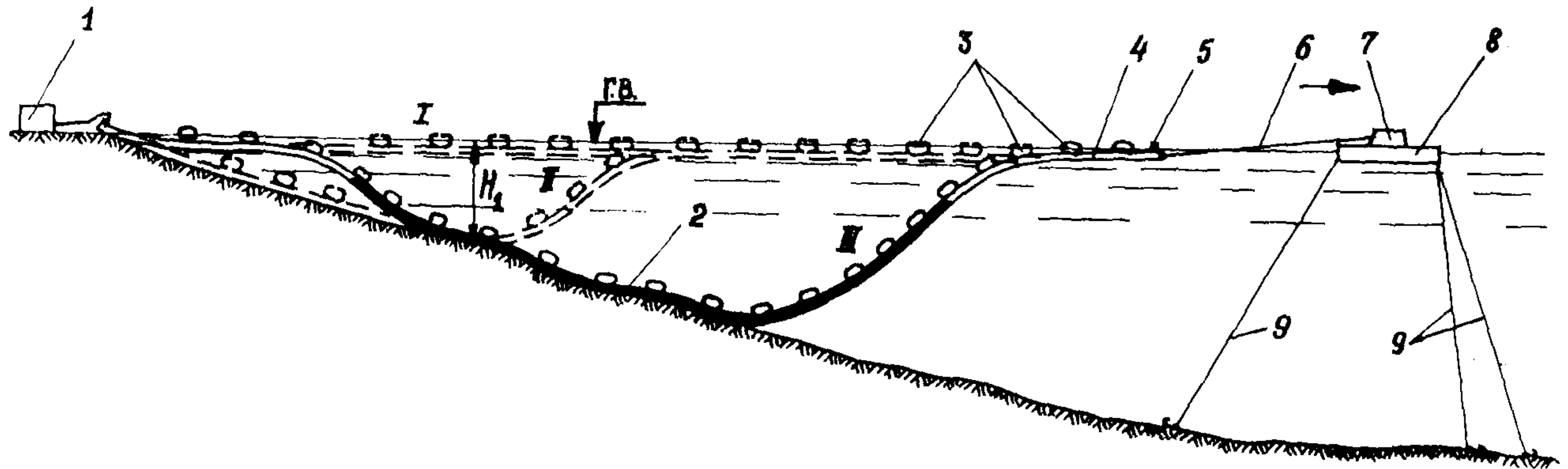
Рис. 10. Схема укладки трубопровода с погружением конечного участка на большие глубины и натяжением трубопровода:
