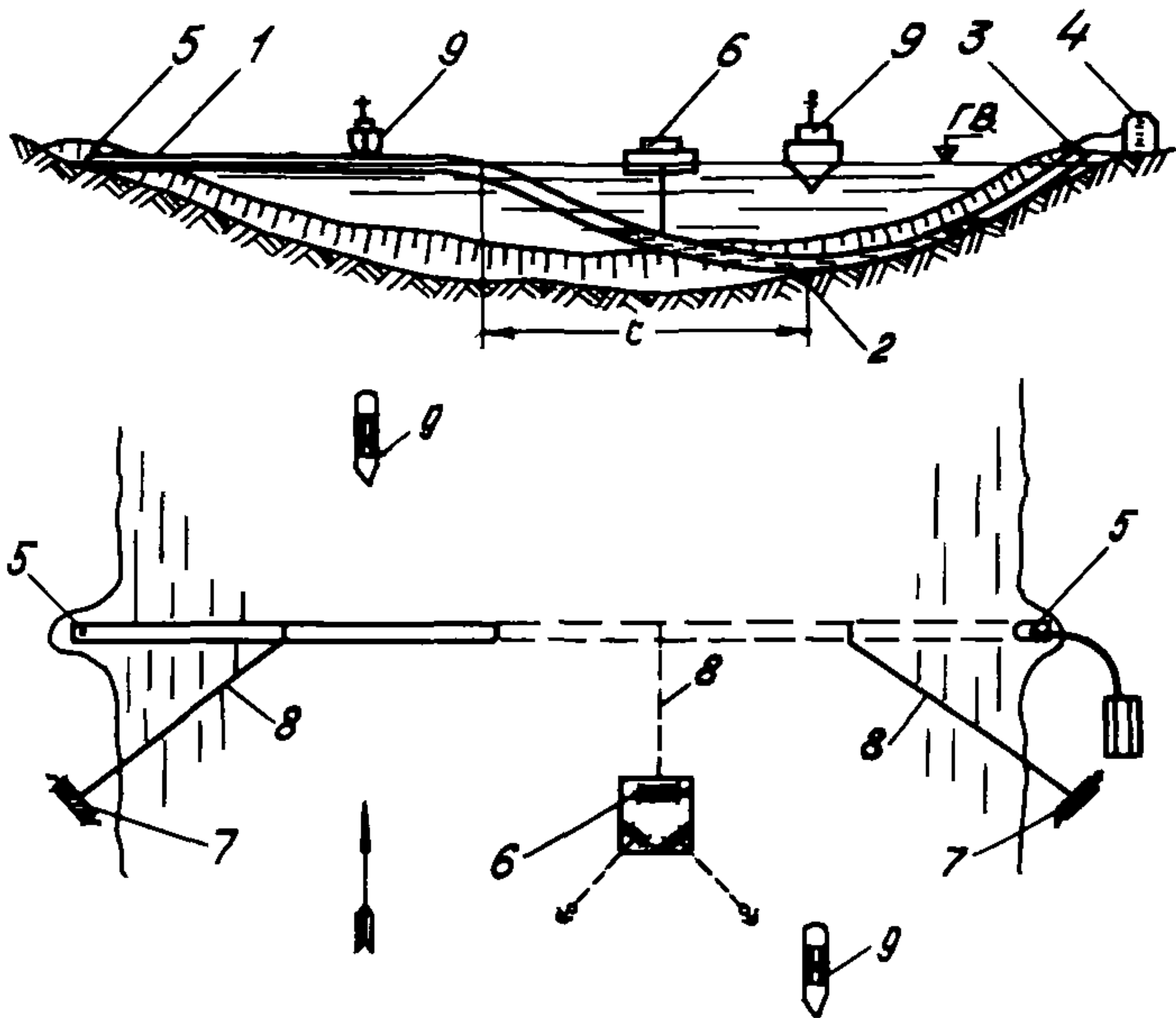
Рис.3. Схема I - погружение плавающего небалластированного трубопровода путем залива в него воды:
