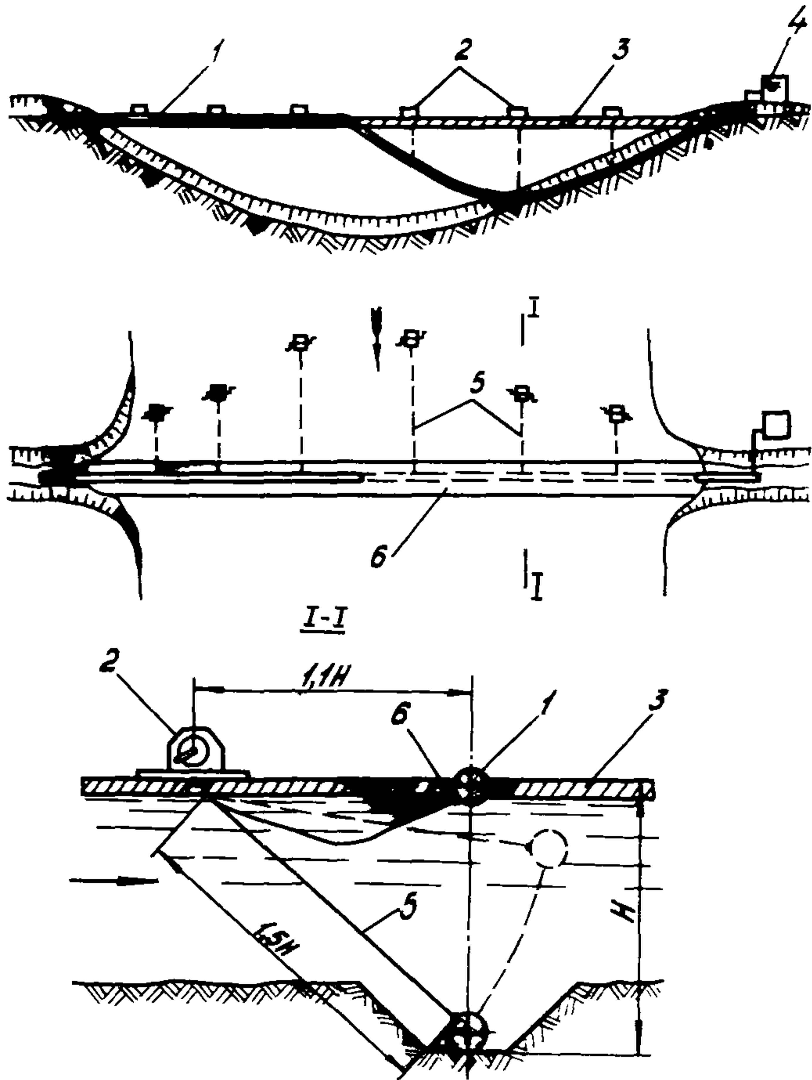
Рис. I. Схема укладки троса схода способом свобод. отг погружения в зимних условиях с предварительной раз- боткой гд. ны:
