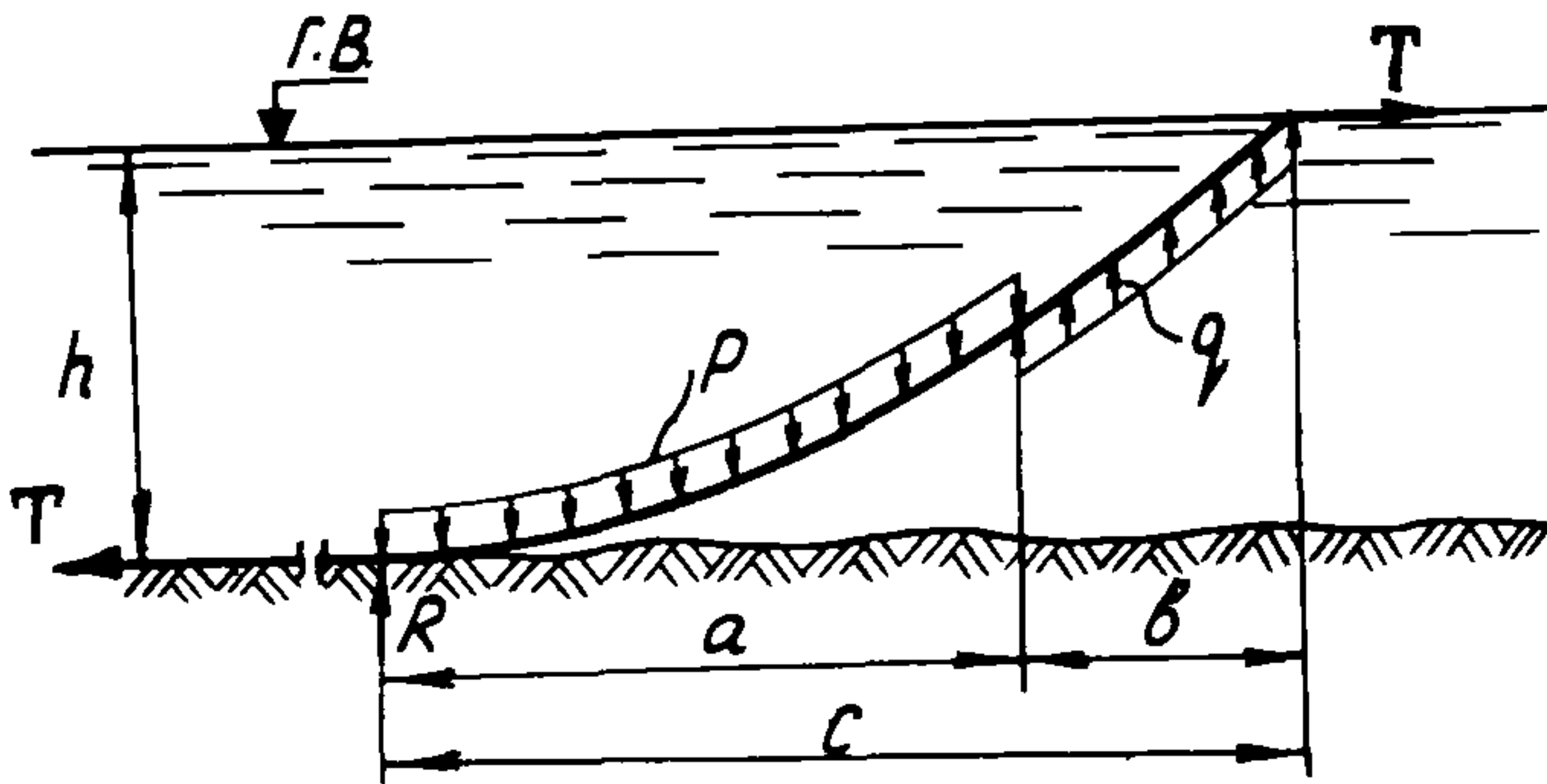
Рис. 18. Расчетная схема трубопровода при концевом изгибе
