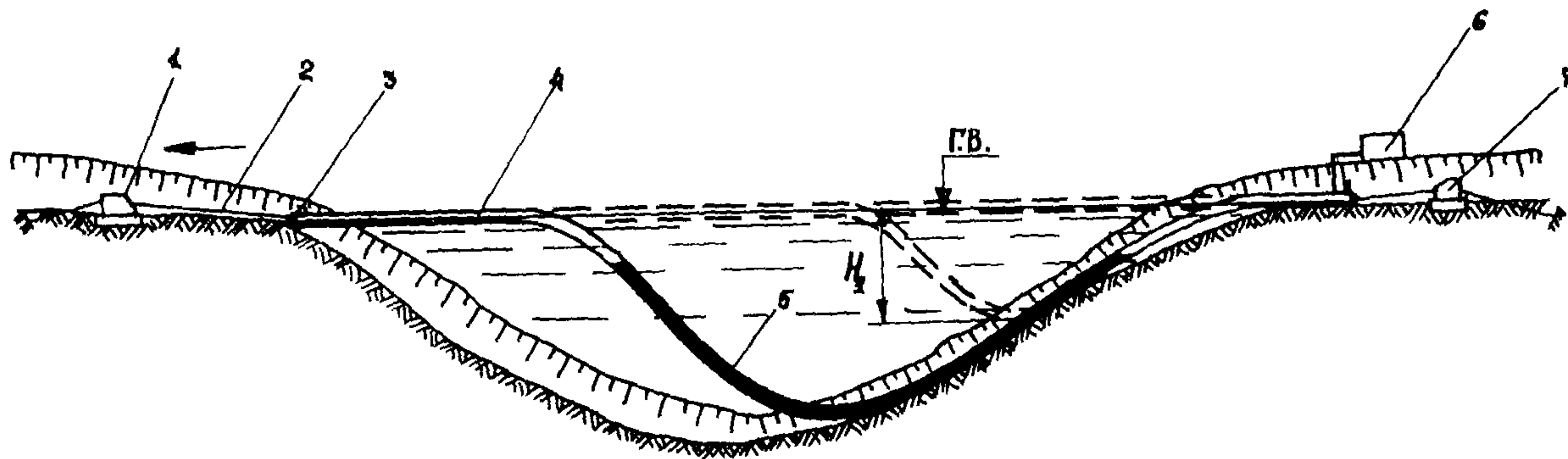
Рис.9. Схема укладки трубопровода способом погружения с применением растягивающего усилия:
