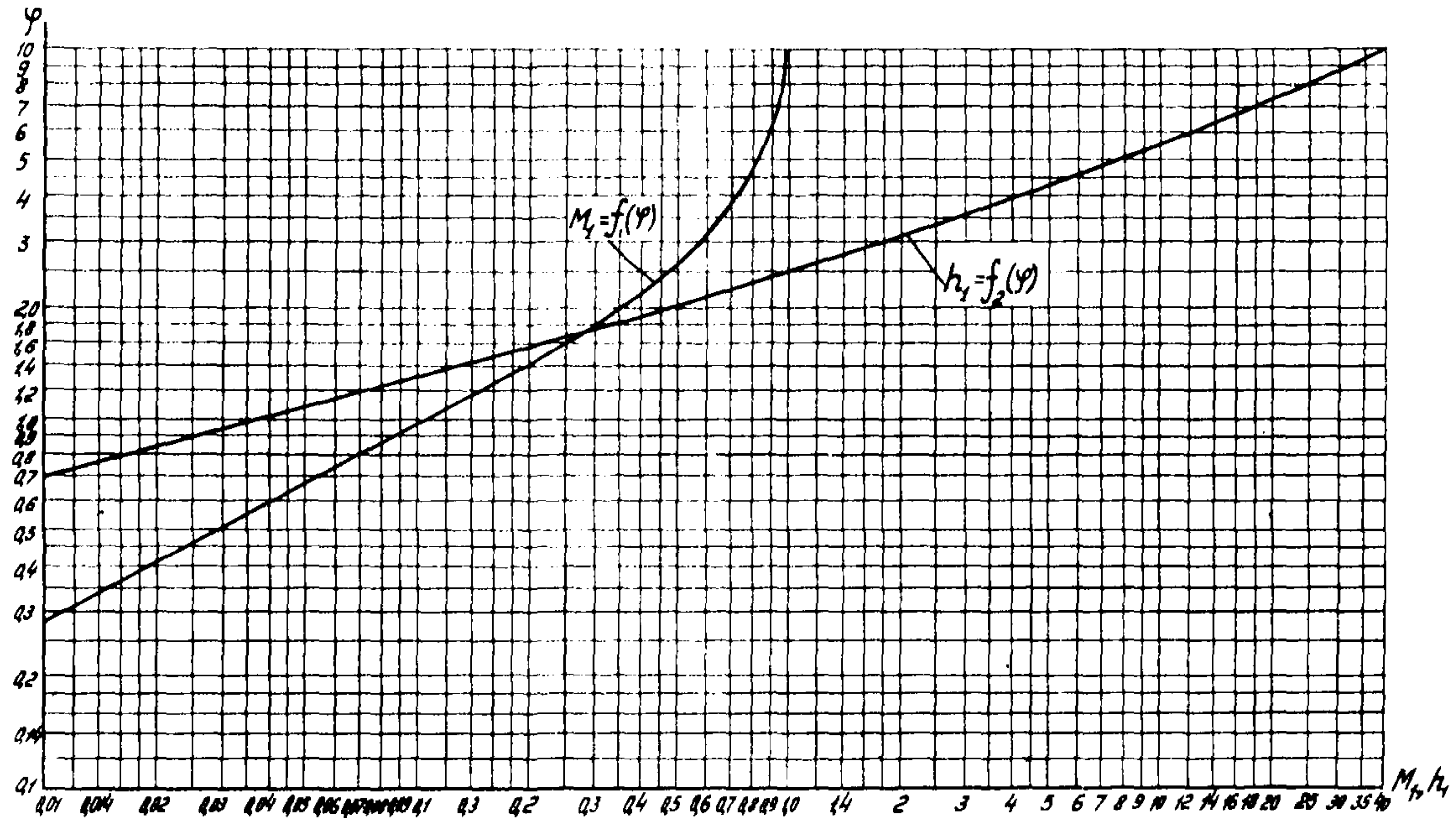
Рис. 20. Графік залежності безрозмірних параметрів M_1 і h_1 від параметра \varphi
