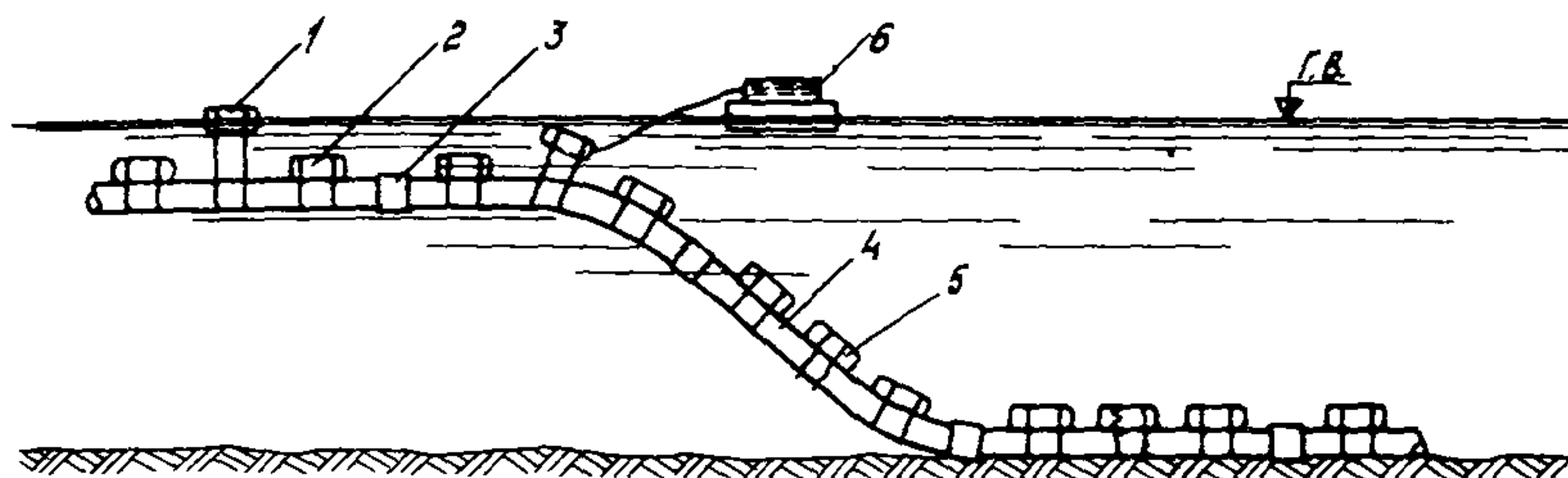
Рис.5. Схема VI - погружение балластированного трубопровода с прикрепленными понтонами путем заливки воды в удерживающие понтоны:
