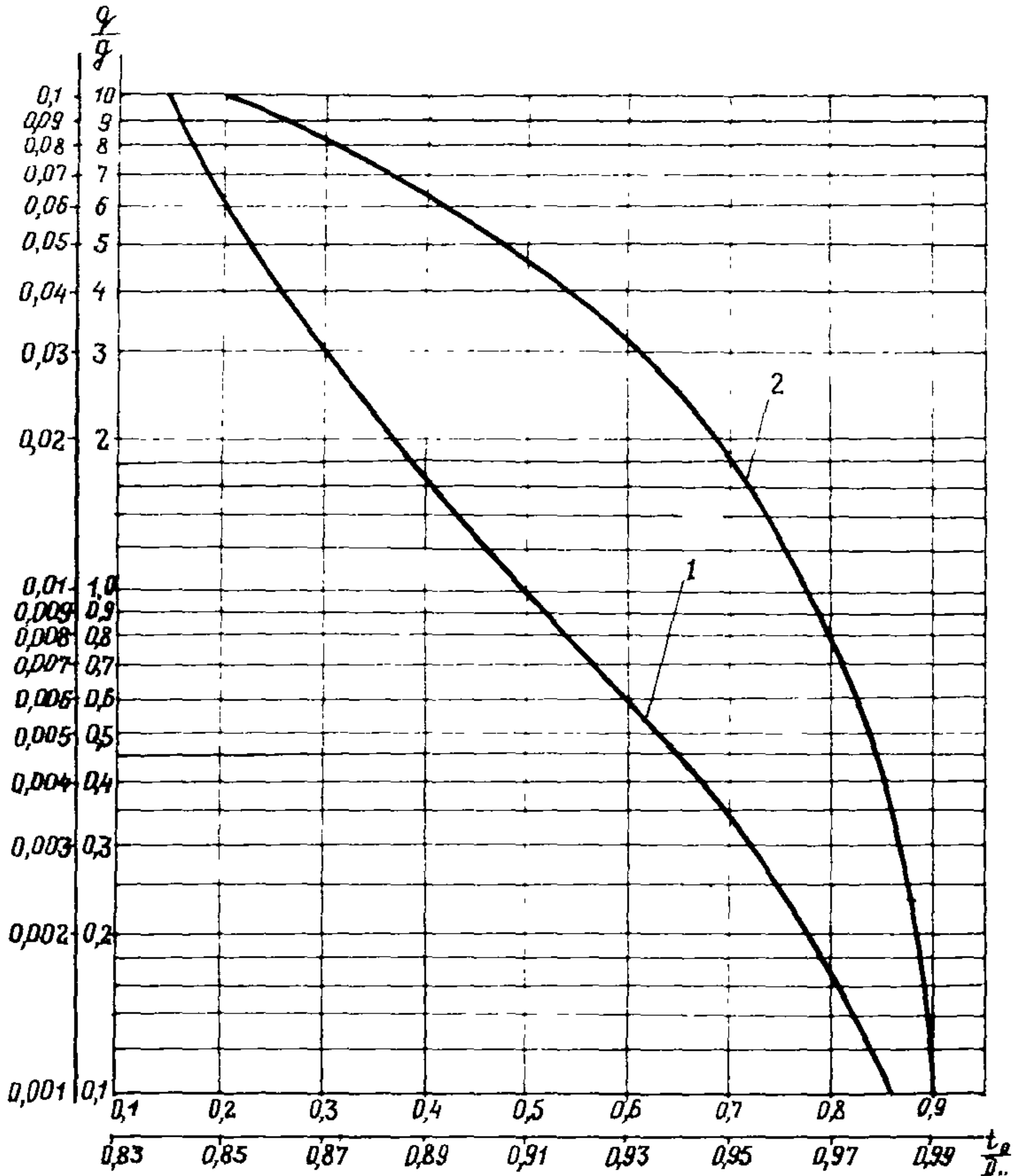
Рис. 14. График зависимости \frac{t_o}{D_n} = f\left(\frac{q}{g}\right) для определения осадки плавящего трубопровода:
