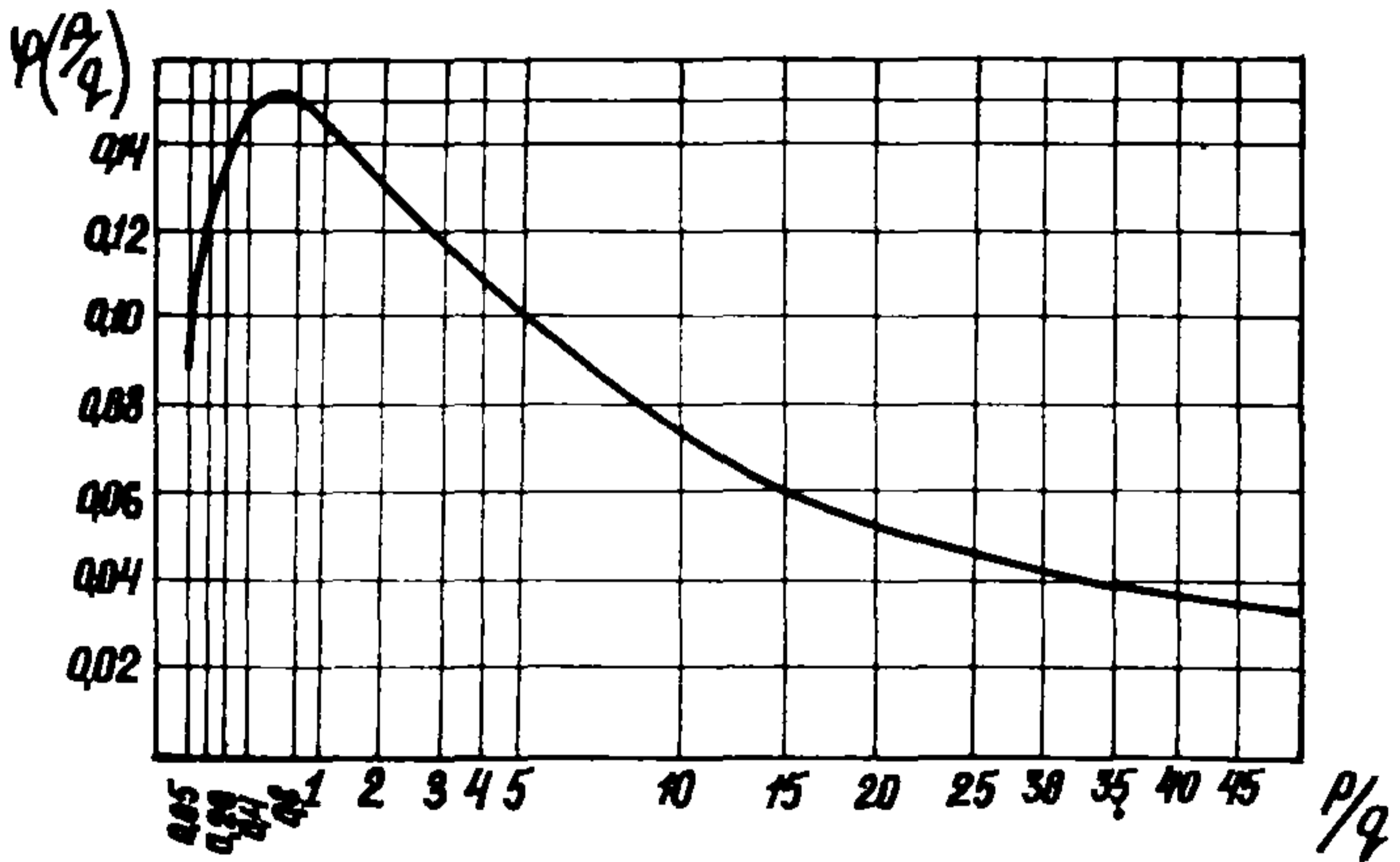
Рис.16. График зависимости функции \varphi от отношения \frac{P}{q}
