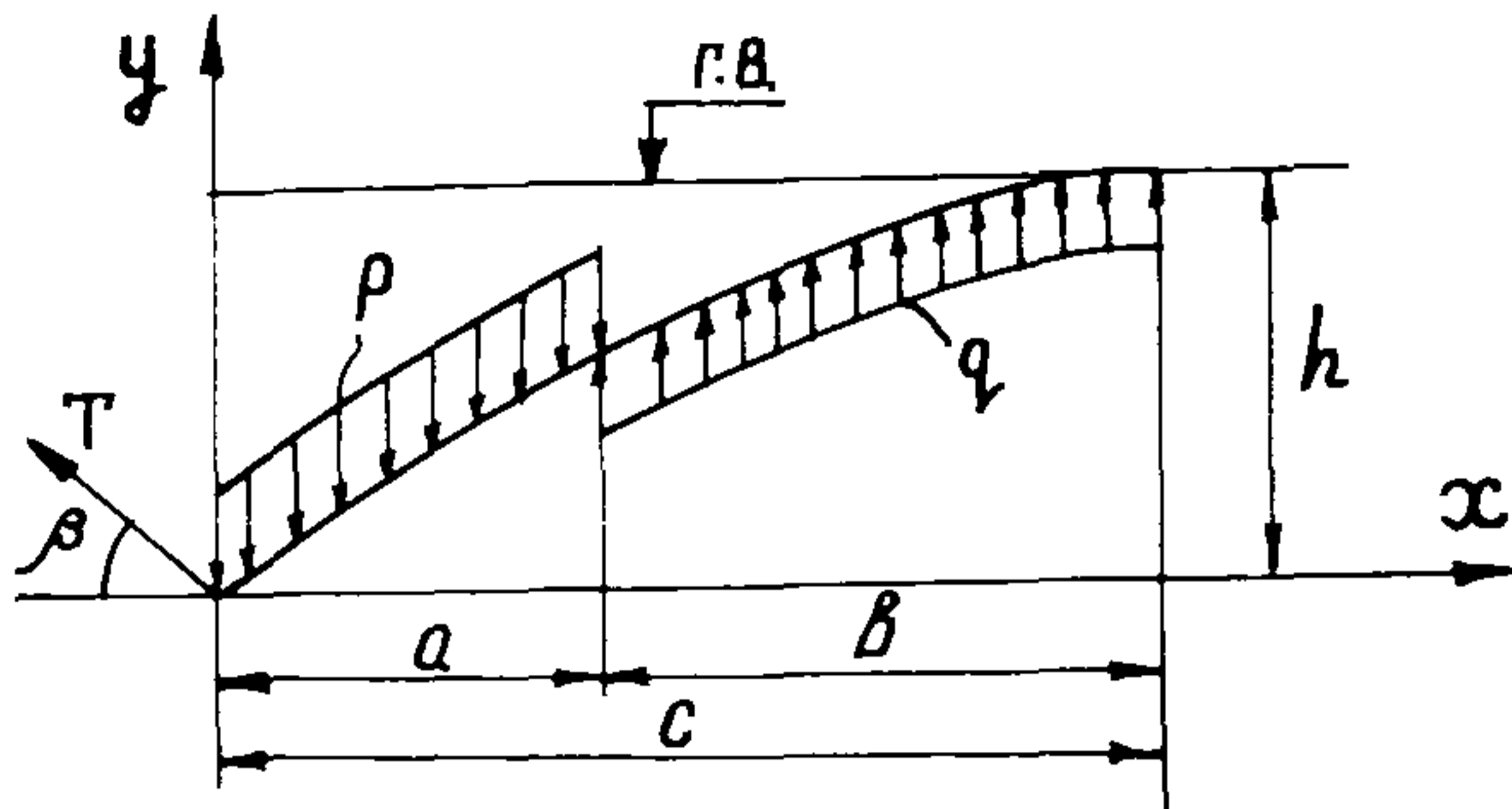
Рис.15. Расчетная схема трубопровода при консольном изгибе
