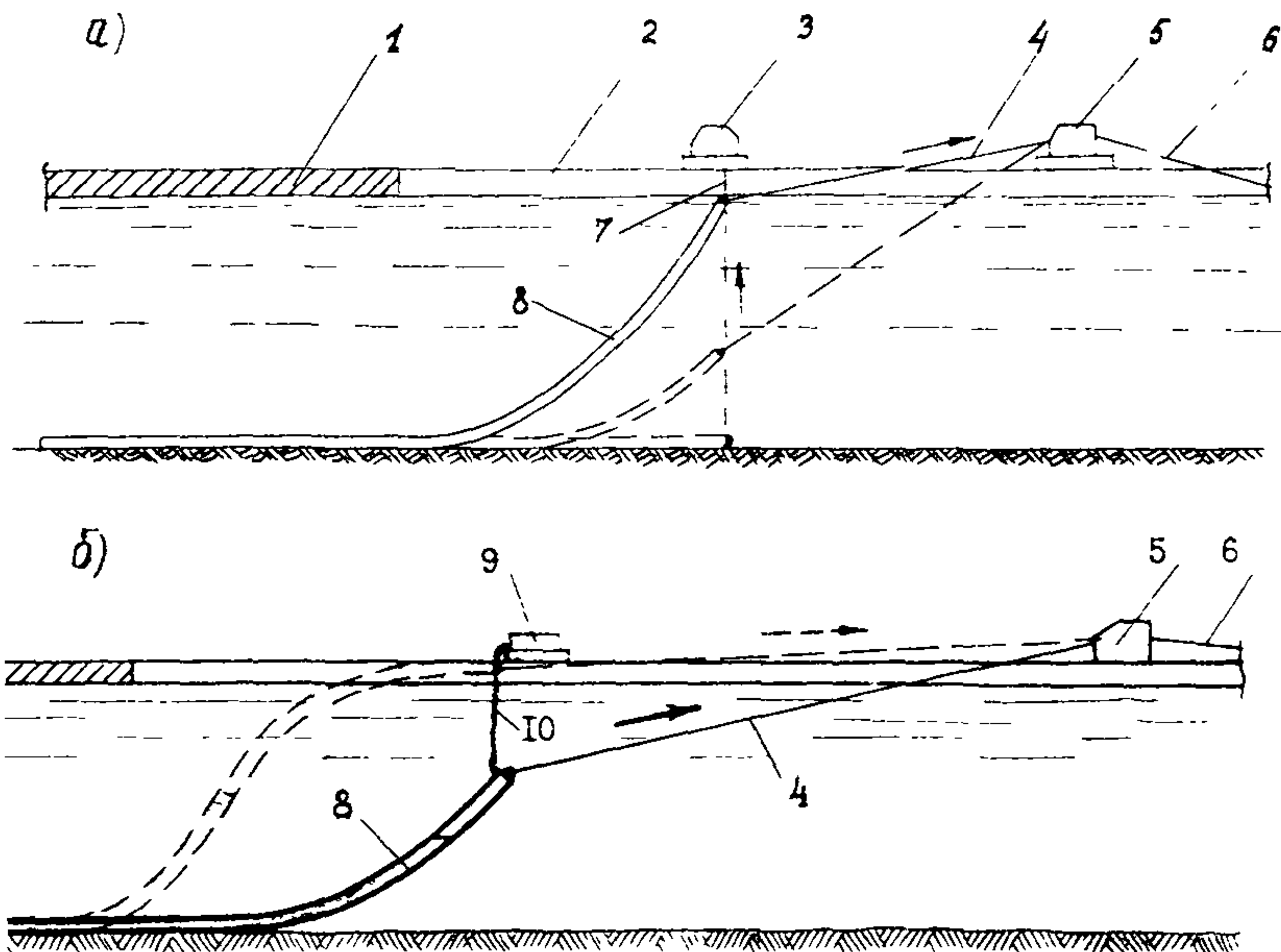
Рис. 13. Схема подъема конечного участка трубопровода с натяжением со льда с помощью грузоподъемных средств (а) и закачки воздуха в трубопровод (б):
