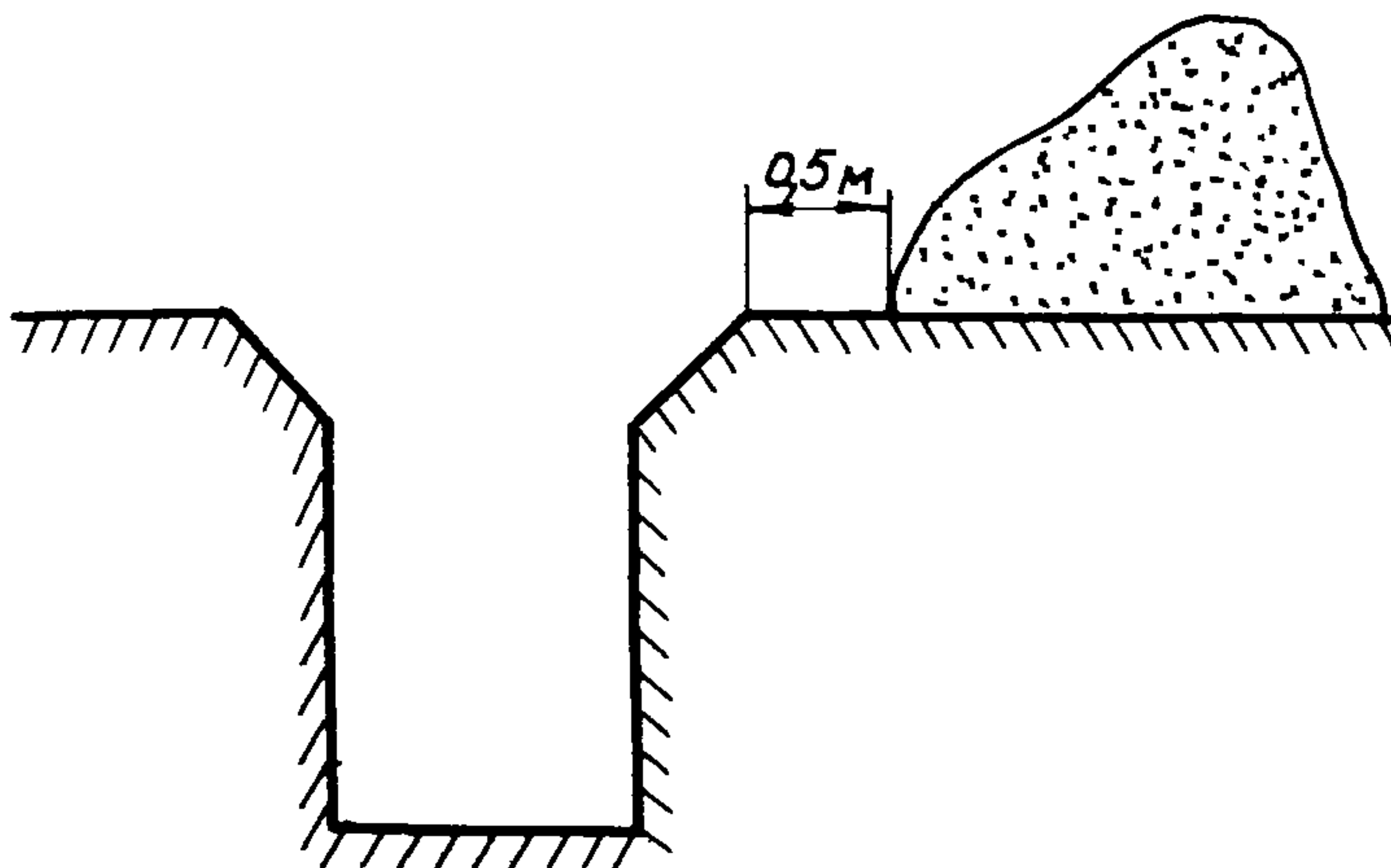
Рис.7. Расположение отвала грунта при рытье траншей
