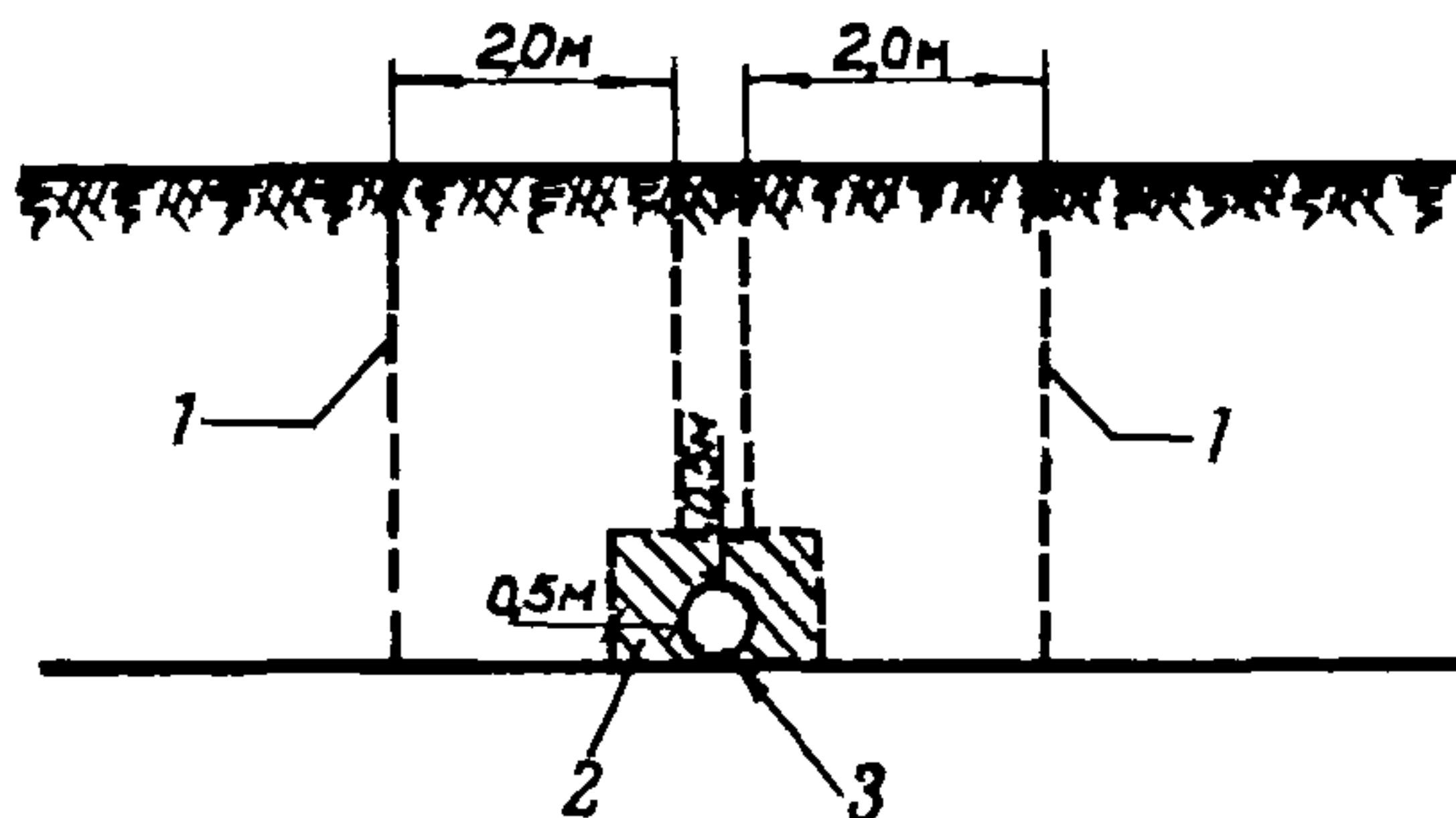
Рис.2. Разработка траншей вблизи действующих подземных коммуникаций:
