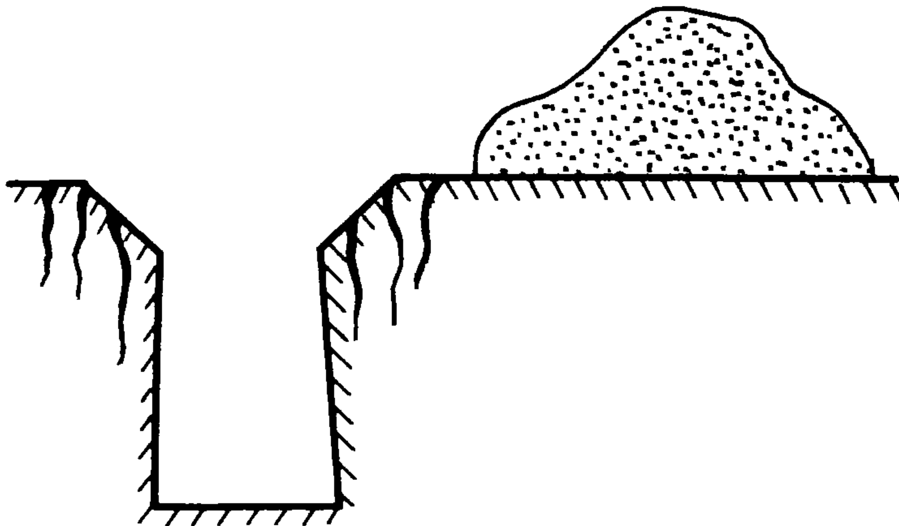
Рис.8. Опасное состояние стенок траншей
