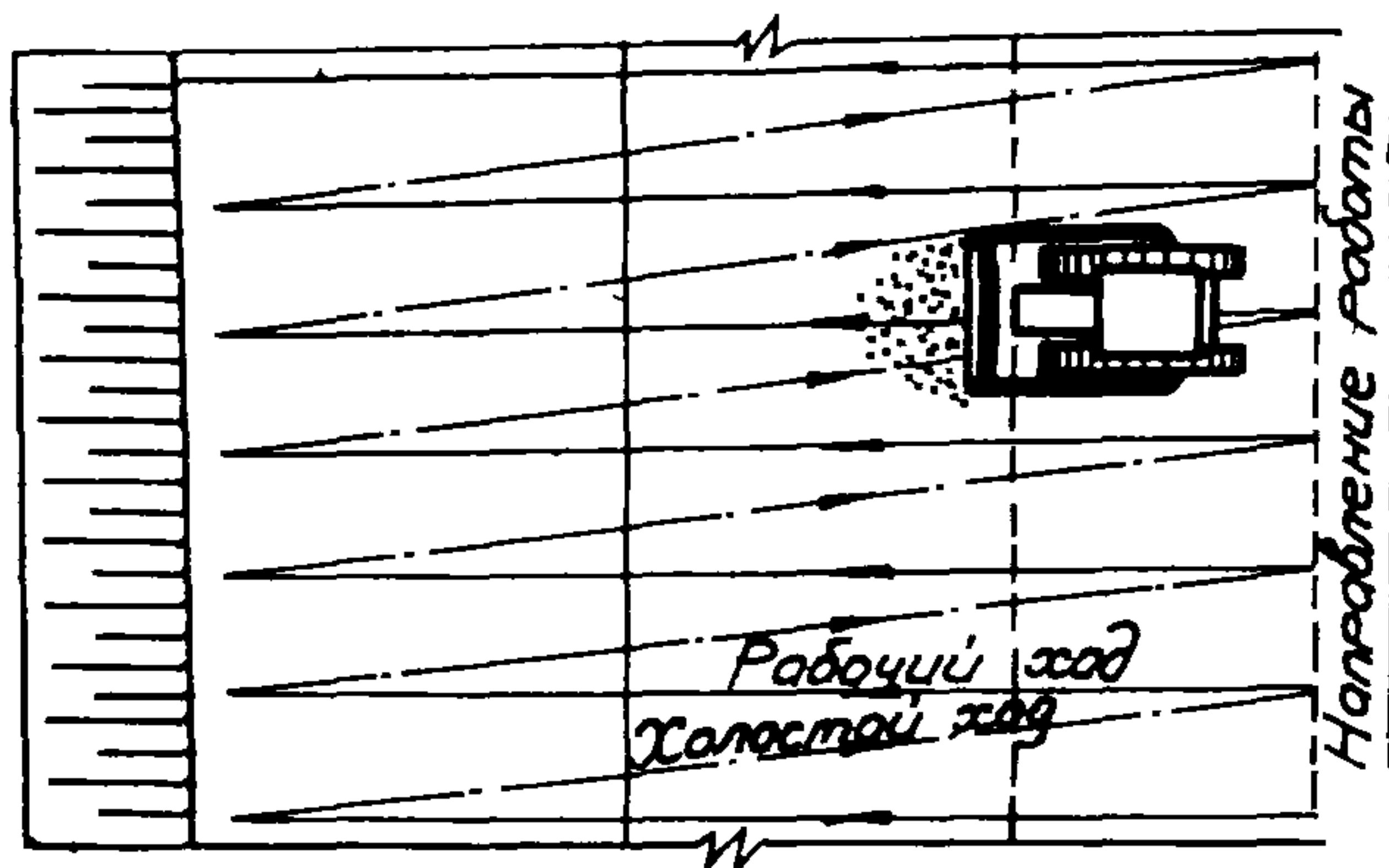
Рис.14. Разработка полки бульдозером
