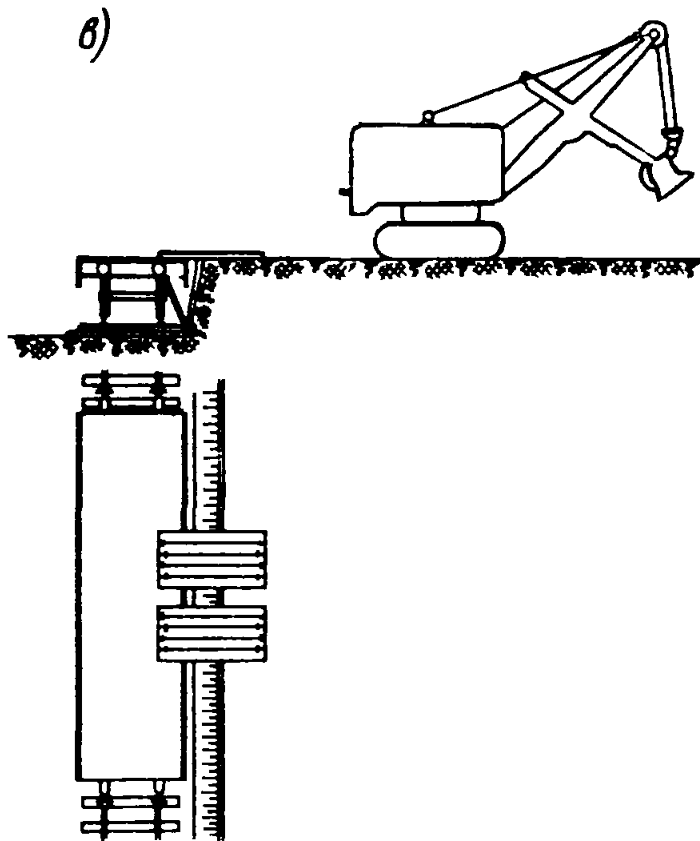
Рис.16. Погрузка одноковшового экскаватора на железнодорожную платформу:
