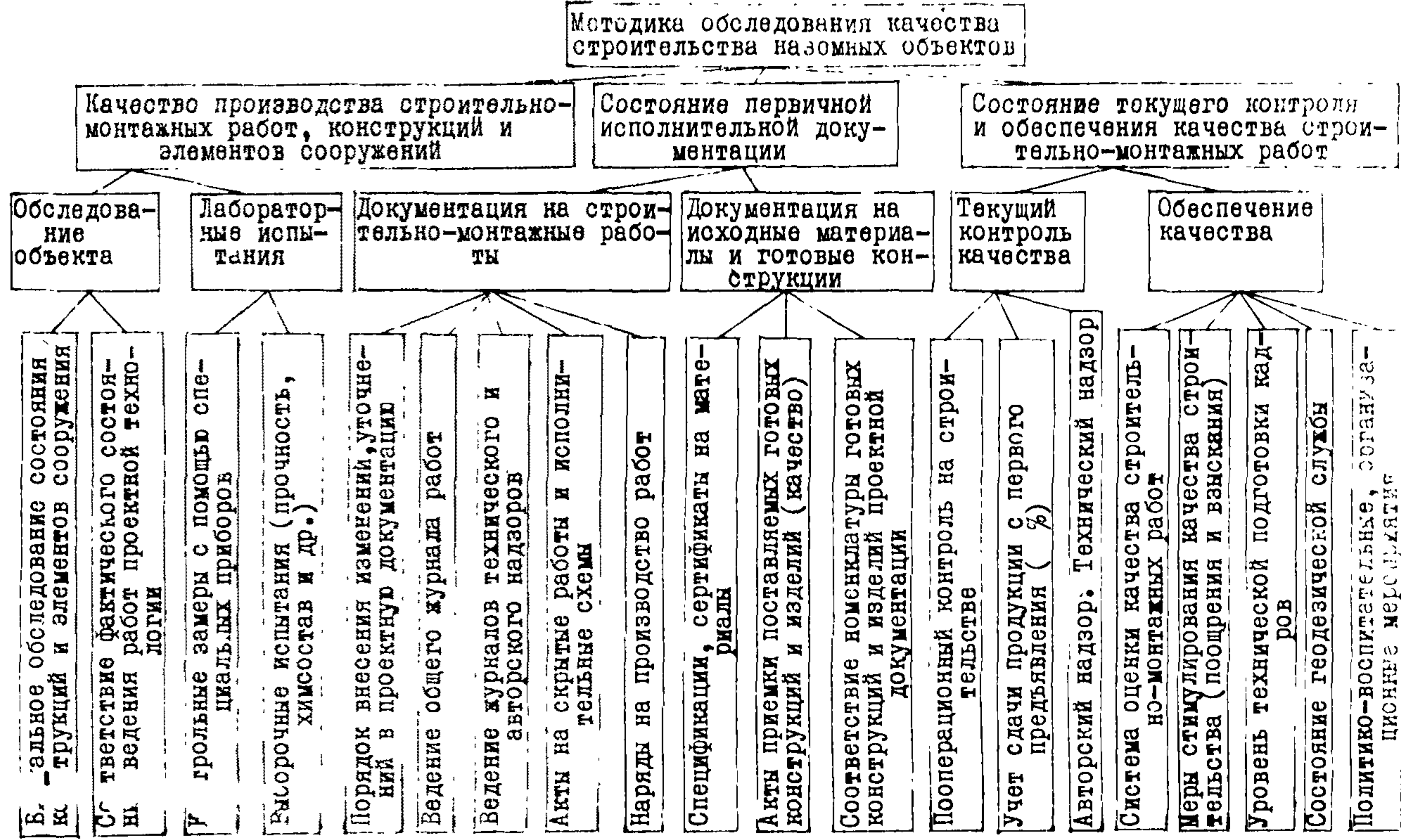
Рис. 3. Порядок обследования качества строительства наземных объектов
