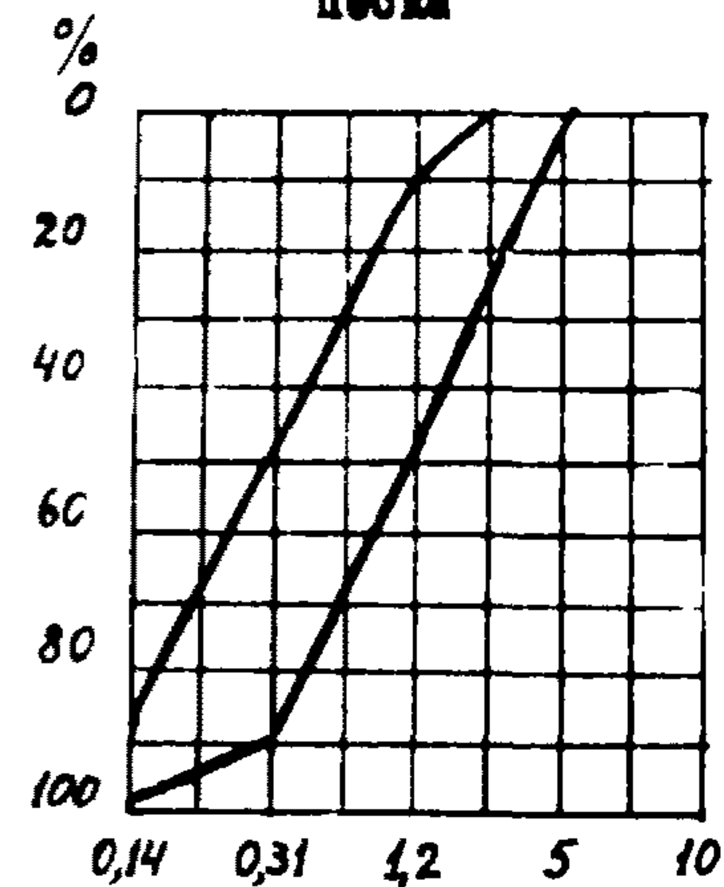
Пределные кривые просеивания песка
