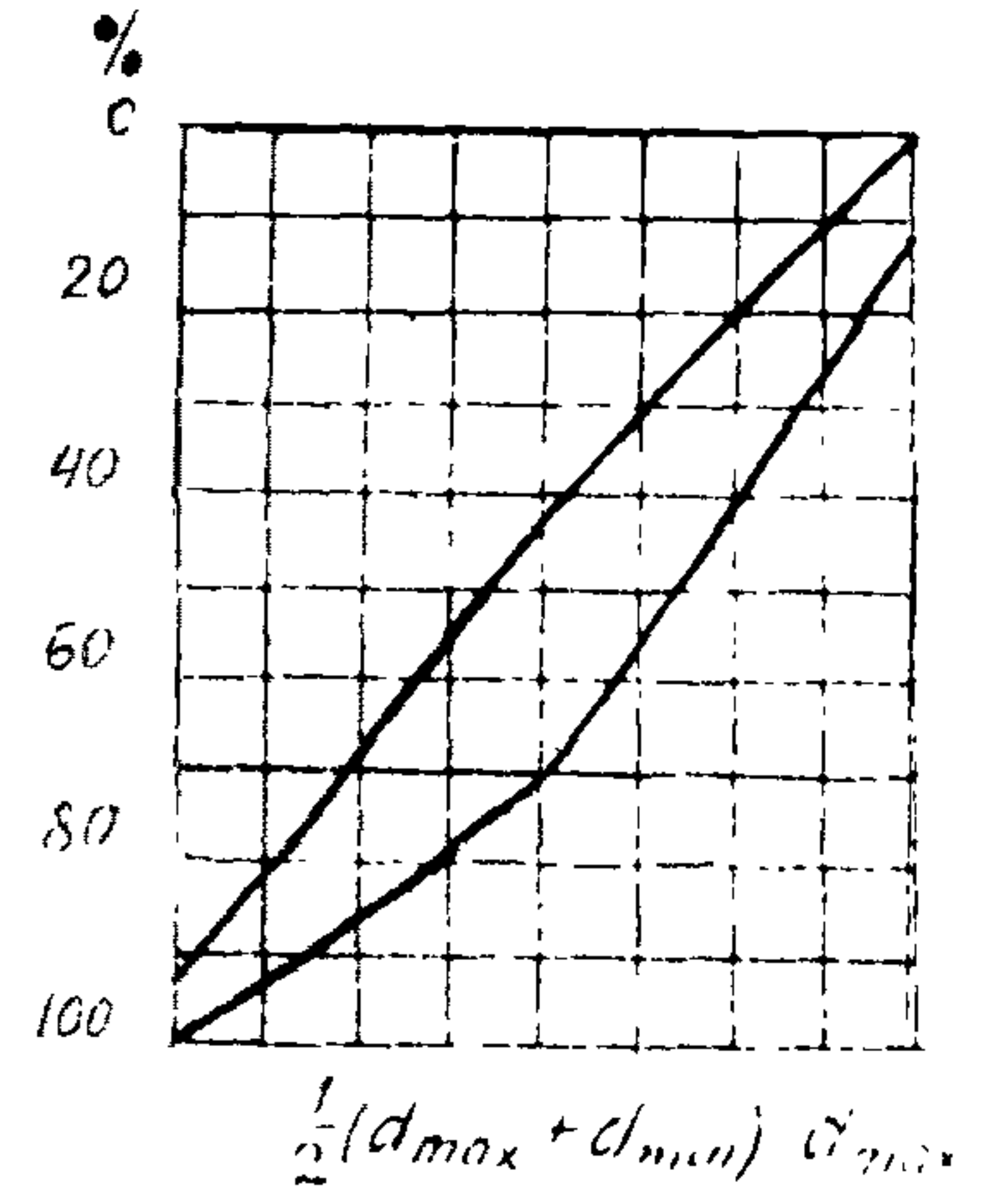
Предельные кривые просеивания гравия
