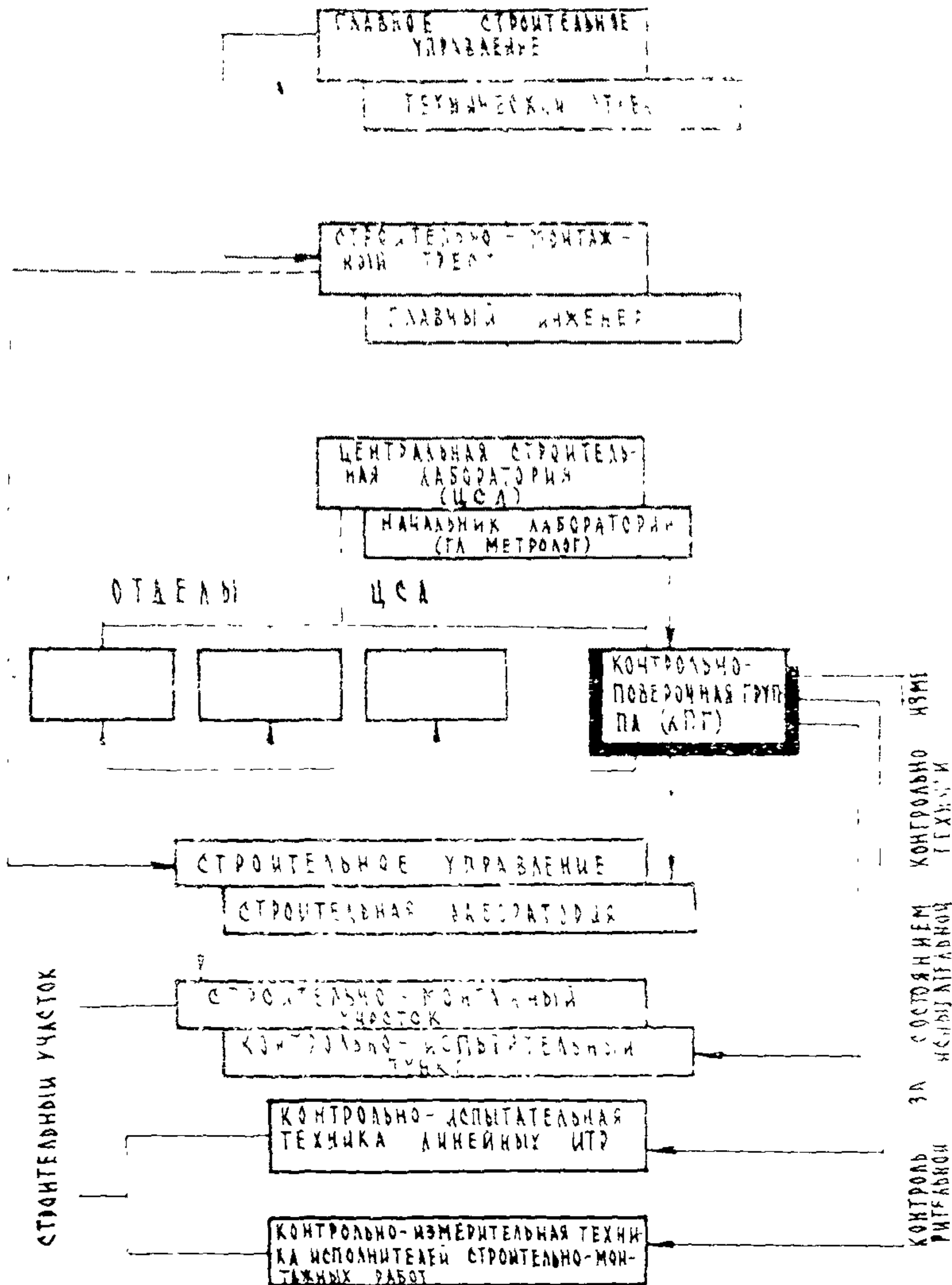
Рис. 8. Схема метрологического обслуживания строительства наземных сооружений
