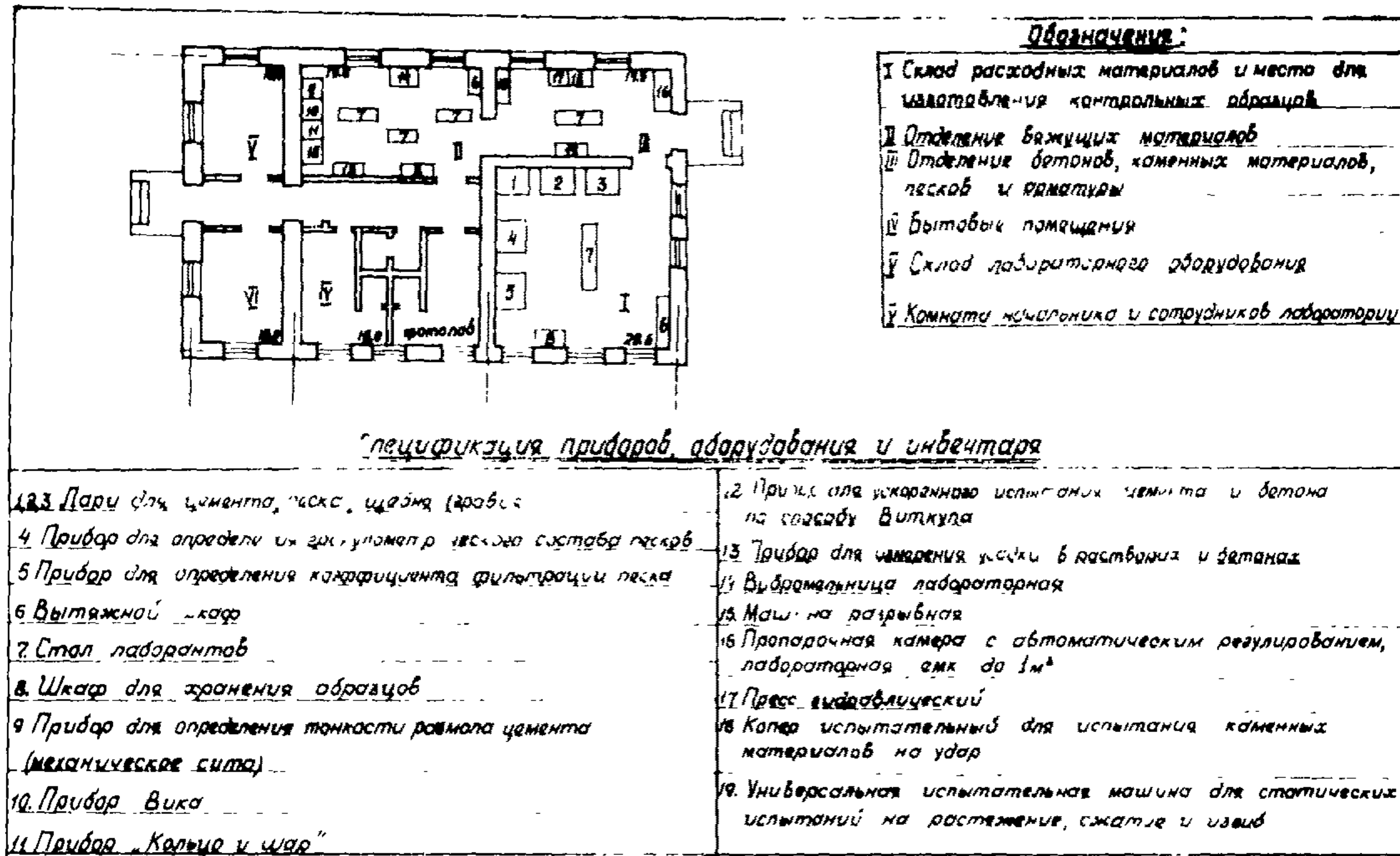
Рис.7. Схема размещения основного оборудования заводской лаборатории
