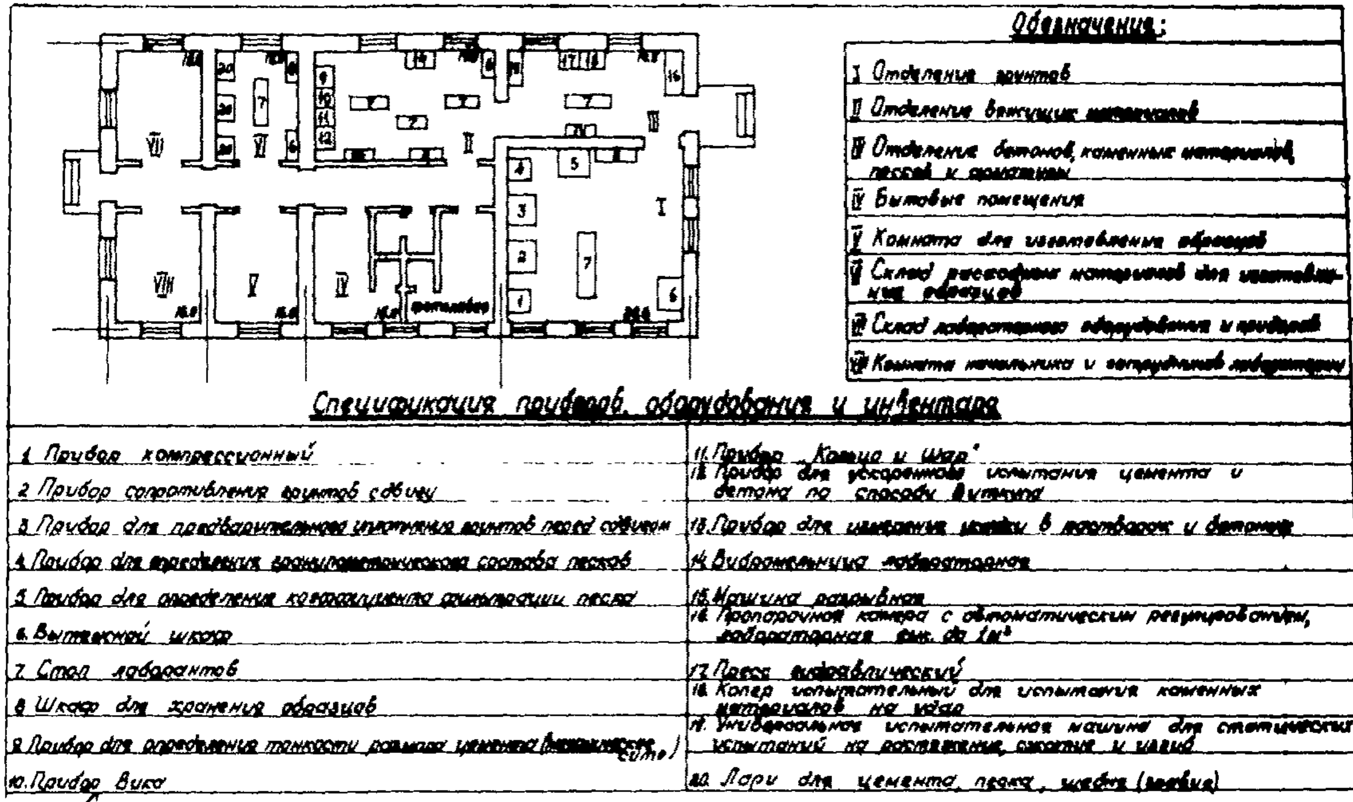
Рис. 6. Схема размещения основного оборудования заводской лаборатории
