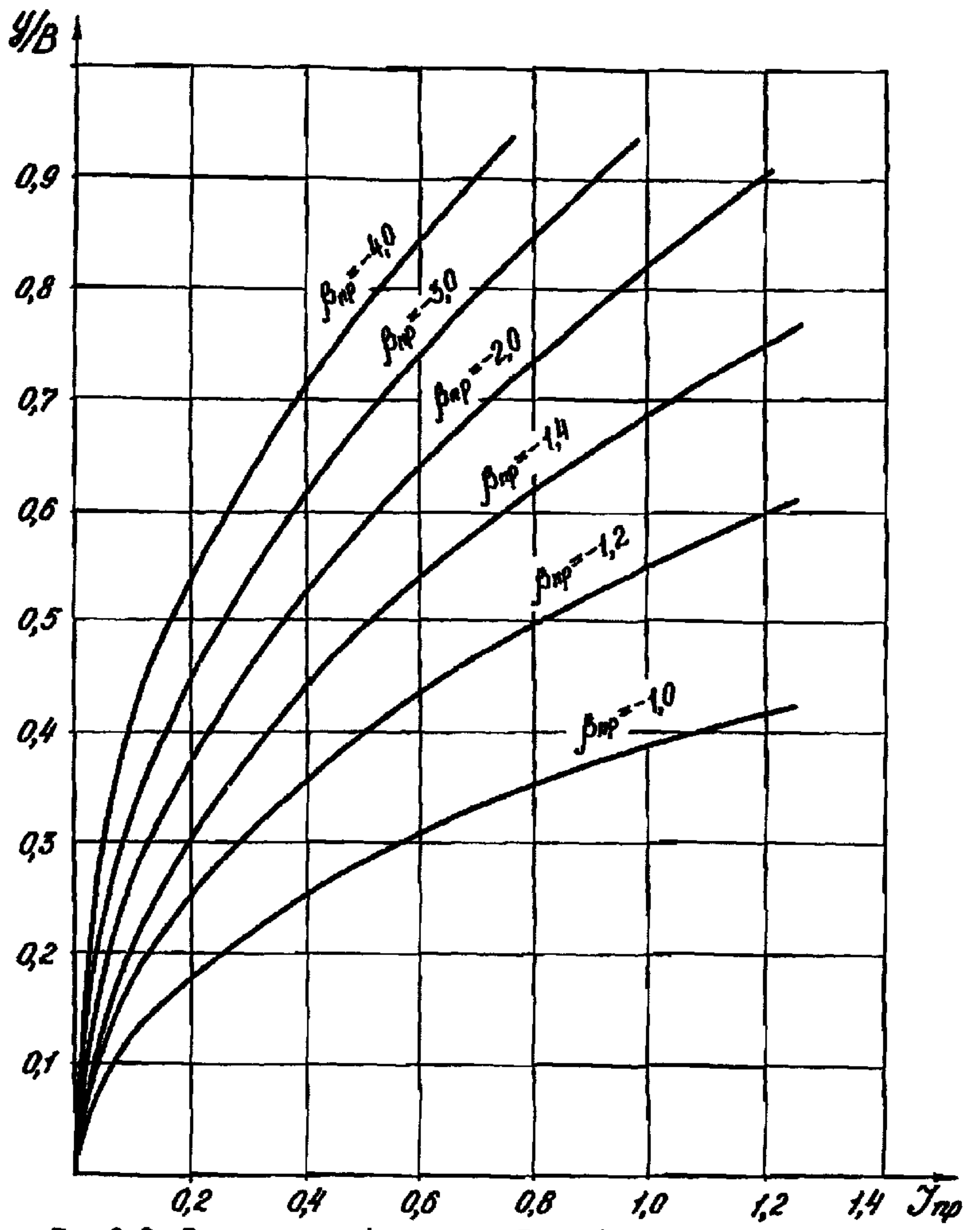
Рис.3.2. Зависимость безразмерной глубины многолетнего промерзания под краем здания от безразмерного времени при t_{зр}^{min} \leq 0
