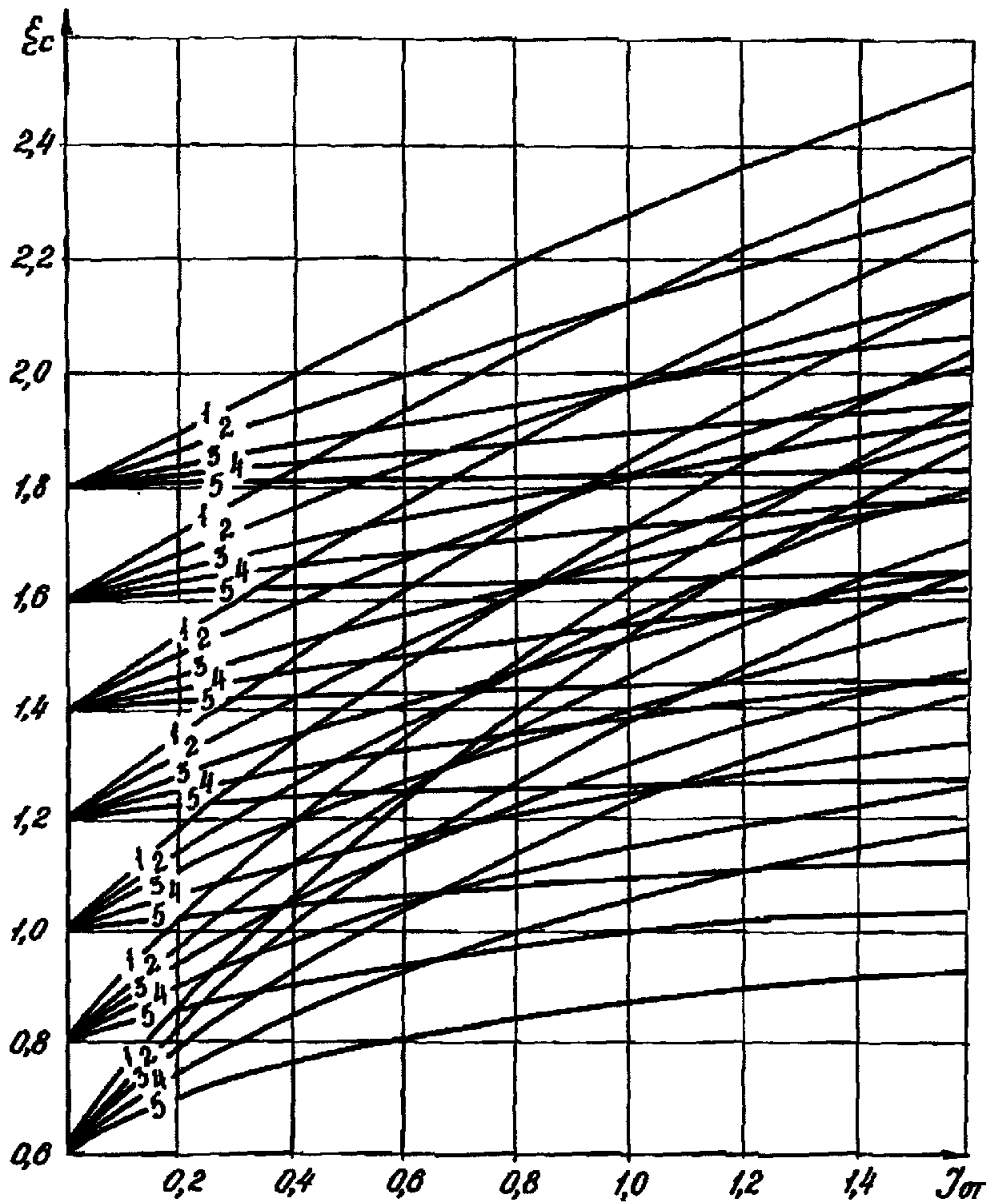
Рис.3.3. Зависимость безразмерной глубины многолетнего оттаивания под серединой здания от безразмерного времени для различных значений H_0
