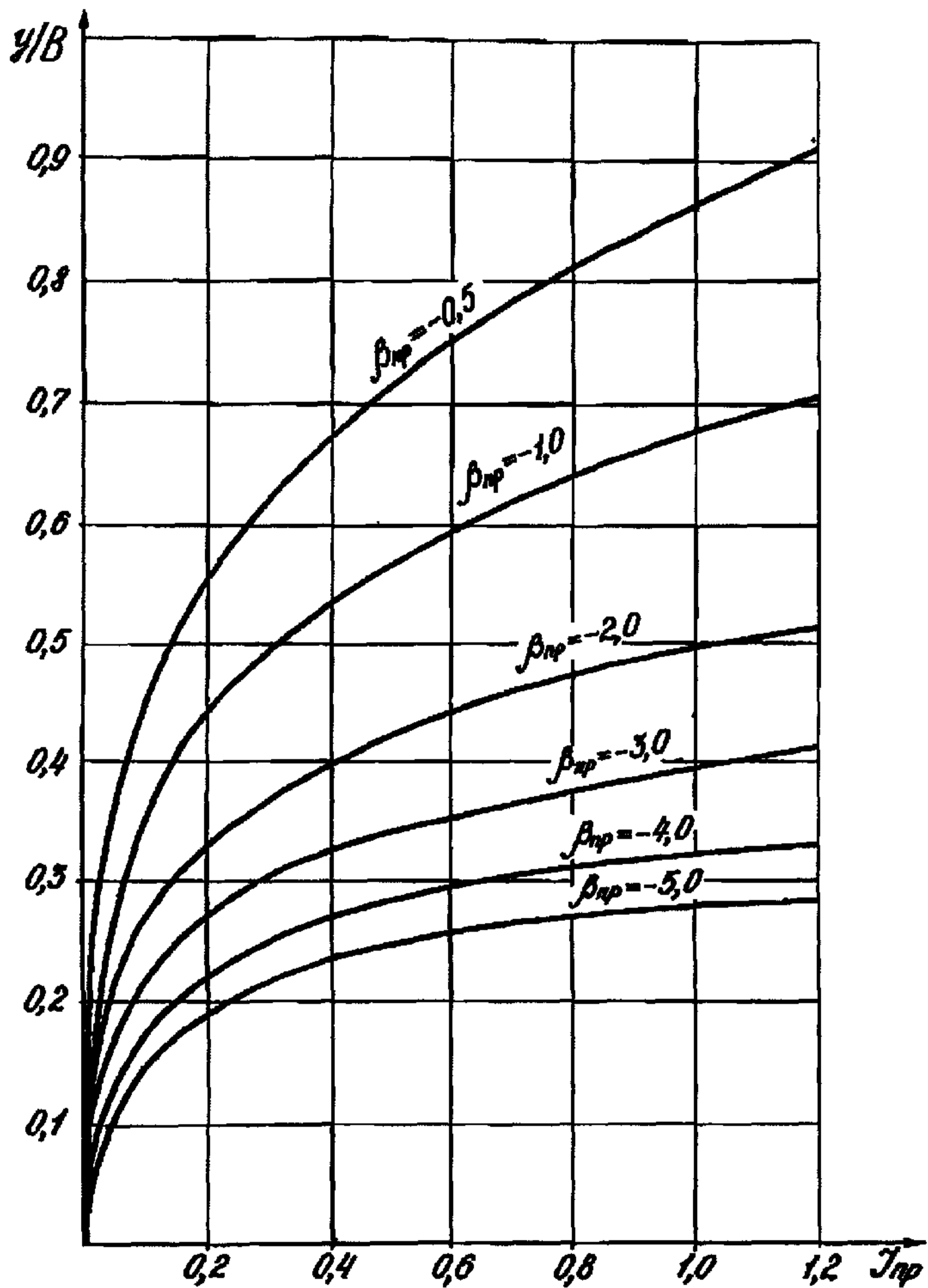
Рис.3.1. Зависимость безразмерной глубины многолетнего промерзания под серединой здания от безразмерного времени при t_{пр}^{мин} > 0
