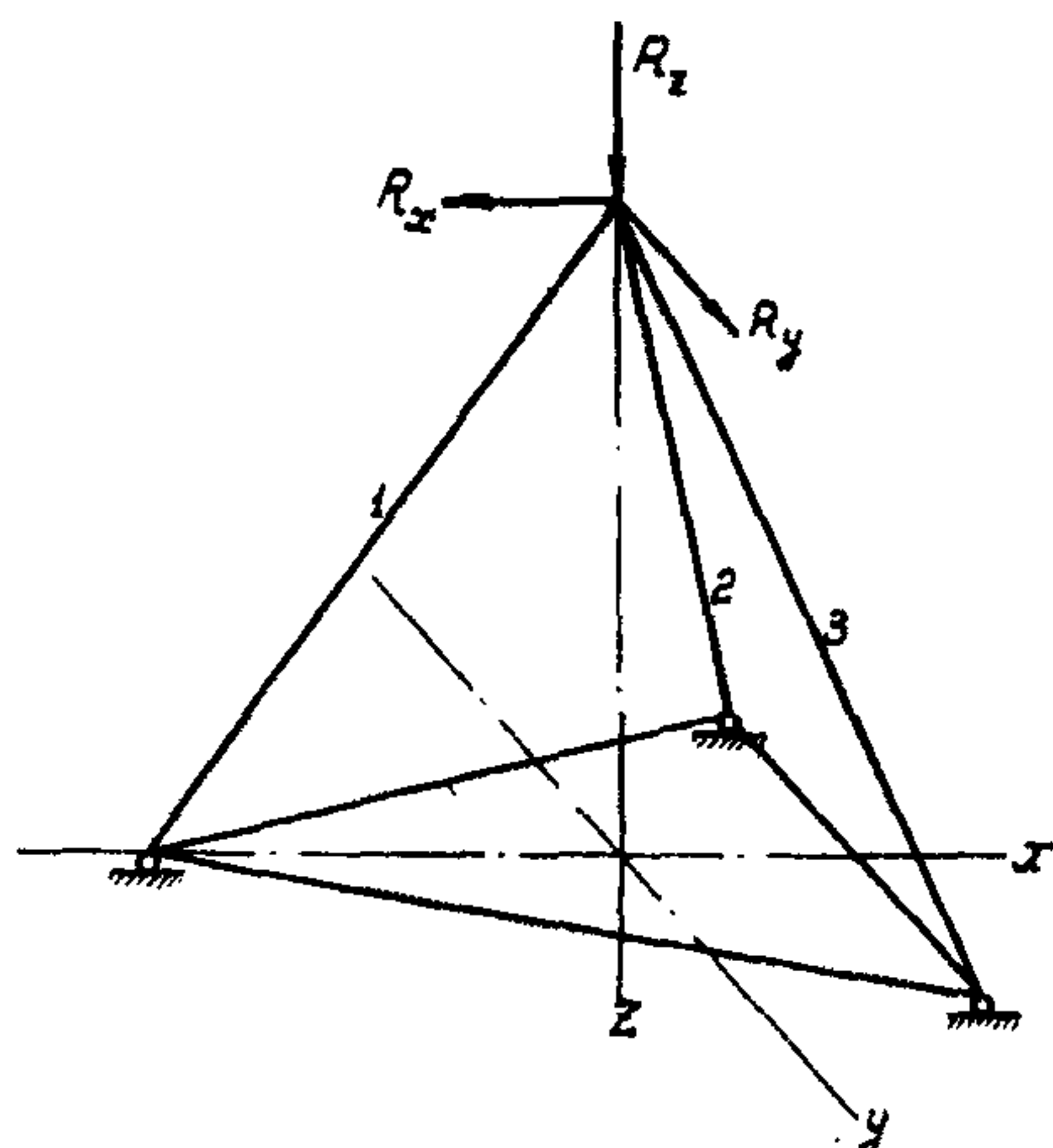
Рис.7. Схема силоизмери- теля, 1,2,3 – стержни
