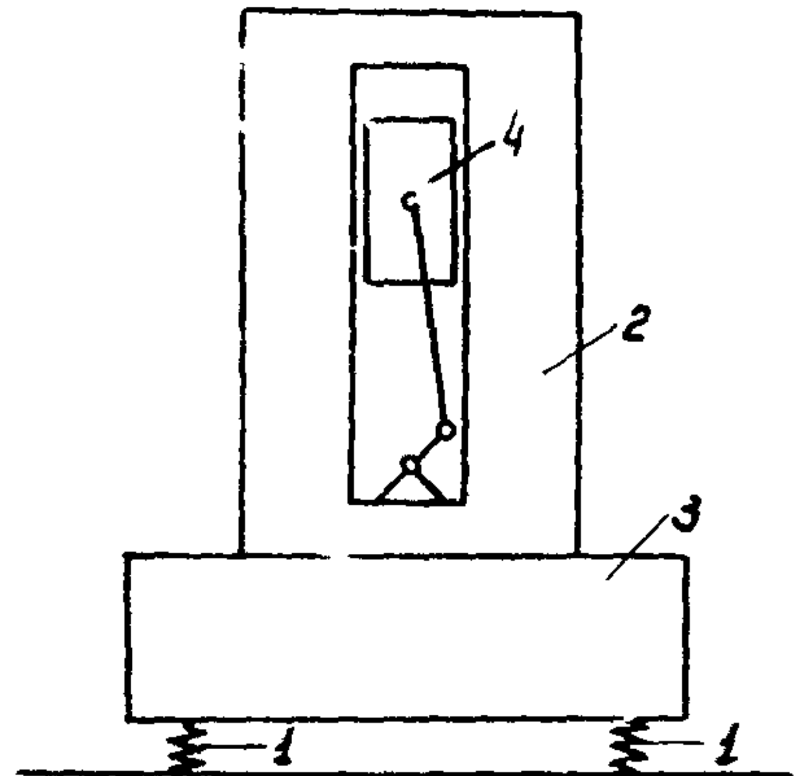
Рис. 3. Схема стенда с шестью степенями свободы для определения динамических нагрузок от машин; 1 - упругие опоры; 2 - машина, 3 - опорная плита, 4 - движущая часть машины
