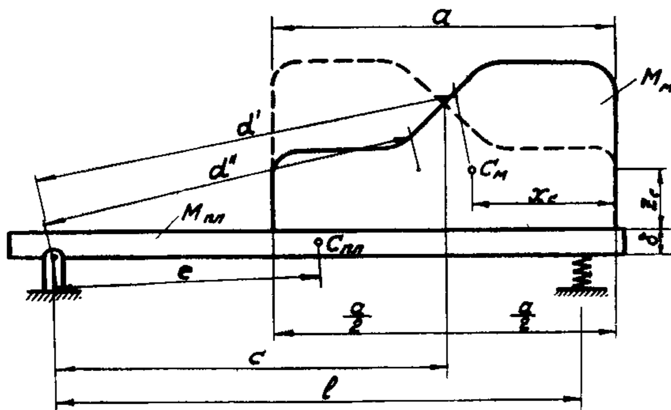
Рис.15. Схема определения положения центра тяжести машин методом упругих опор; S_{пл} – центр тяжести плиты, S_M – центр тяжести машины
