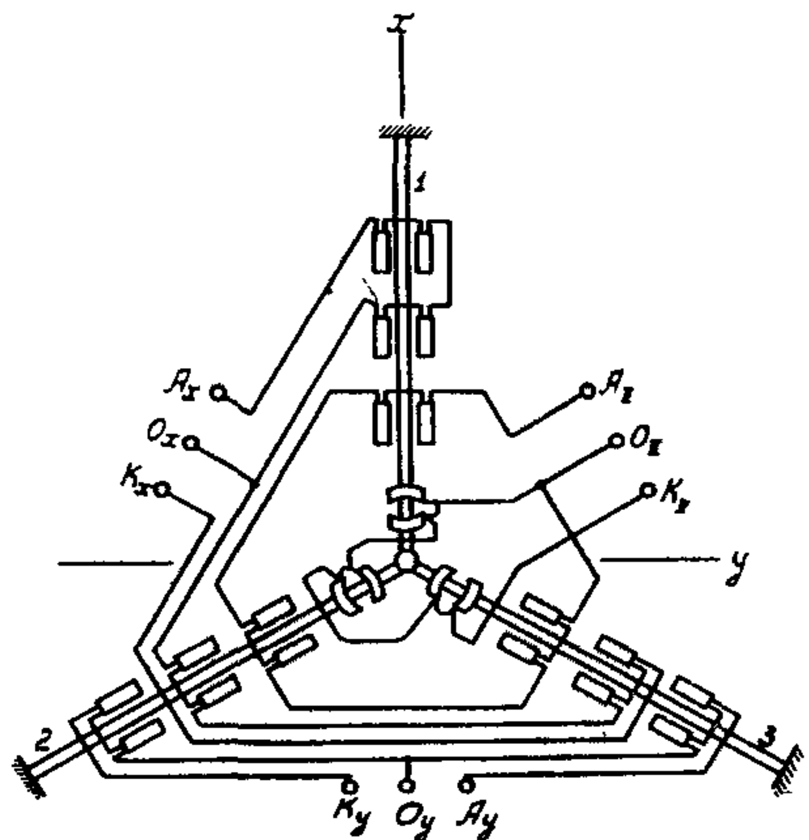
Рис. 8. Схема размещения и коммутации датчиков на шейках стержней измерительного штатива силоизмерителя; 1, 2, 3 — стержни, A_x, O_x, K_x, A_y, O_y, K_y, A_z, O_z, K_z — клеммы полумостов, измеряющих составляющие R_x, R_y, R_z динамической силы, A_x, A_y, A_z — активные датчики, K_x, K_y, K_z — компенсационные датчики
