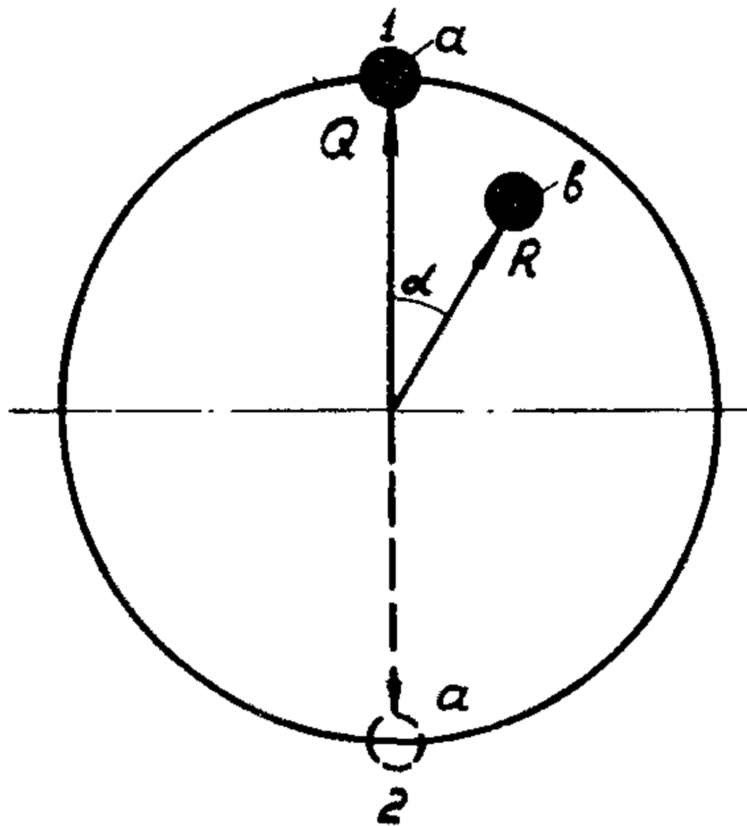
Рис.9. Схема расположения пробного груза a и неуравновешенности b в роторе
