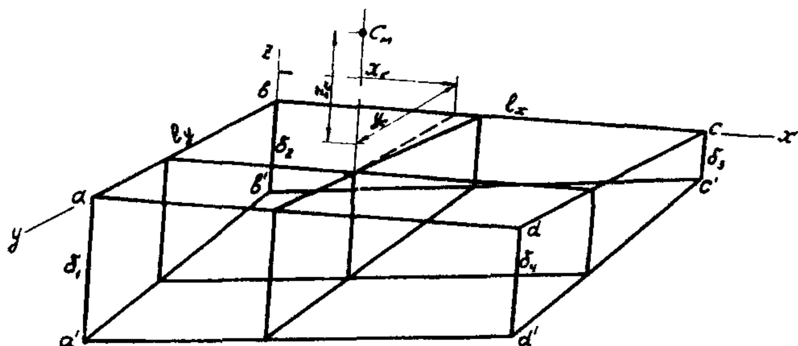
Рис.13. Схема определения положения центра тяжести машины методом замера статических осадок; \alpha bcd и \alpha'b'c'd' - места опирания плиты стенда на упругие опоры до и после установки машины на стенд (машина и упругие опоры на схеме не показаны); C_M - центр тяжести машины
