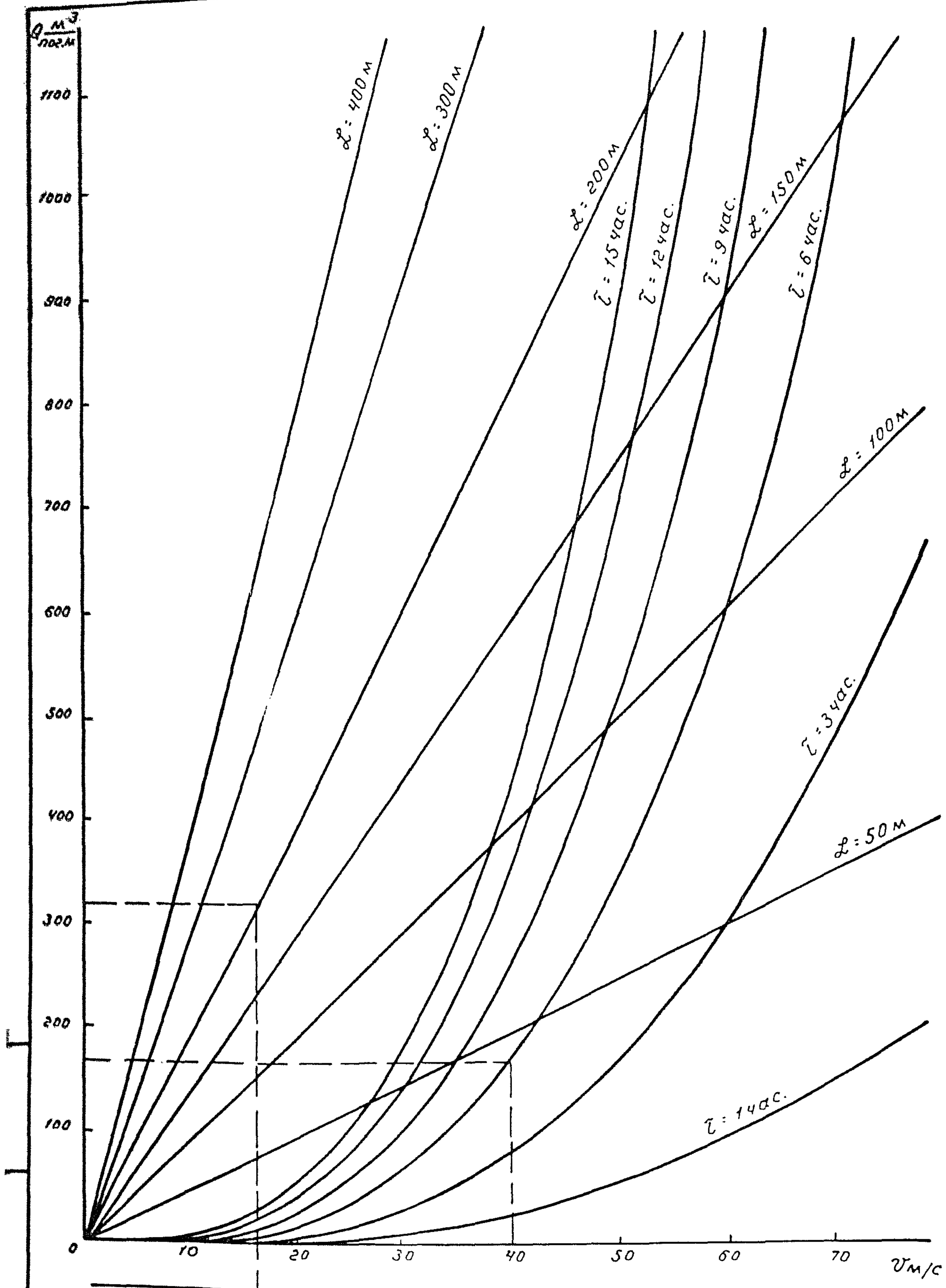
График для определения расчетного объема снегопереноса
