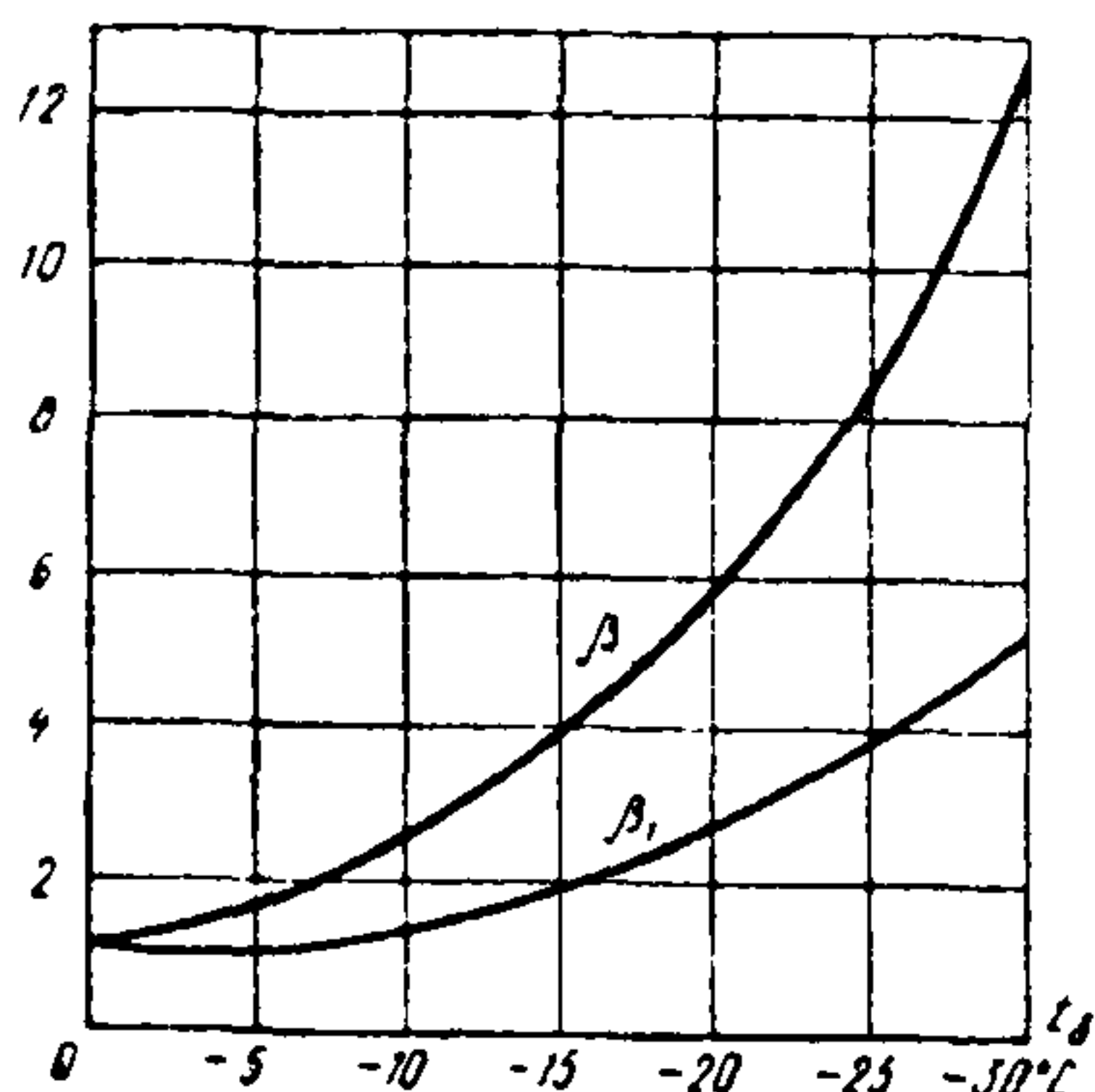
Рис. 7. Зависимость коэффициентов \beta и R_1 от температуры внутреннего воздуха охлаждаемых помещений t_v
