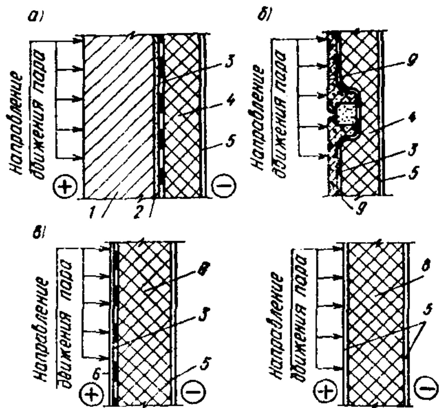
Рис. 3. Схемы тепло-пароизоляции стен и перегородок
