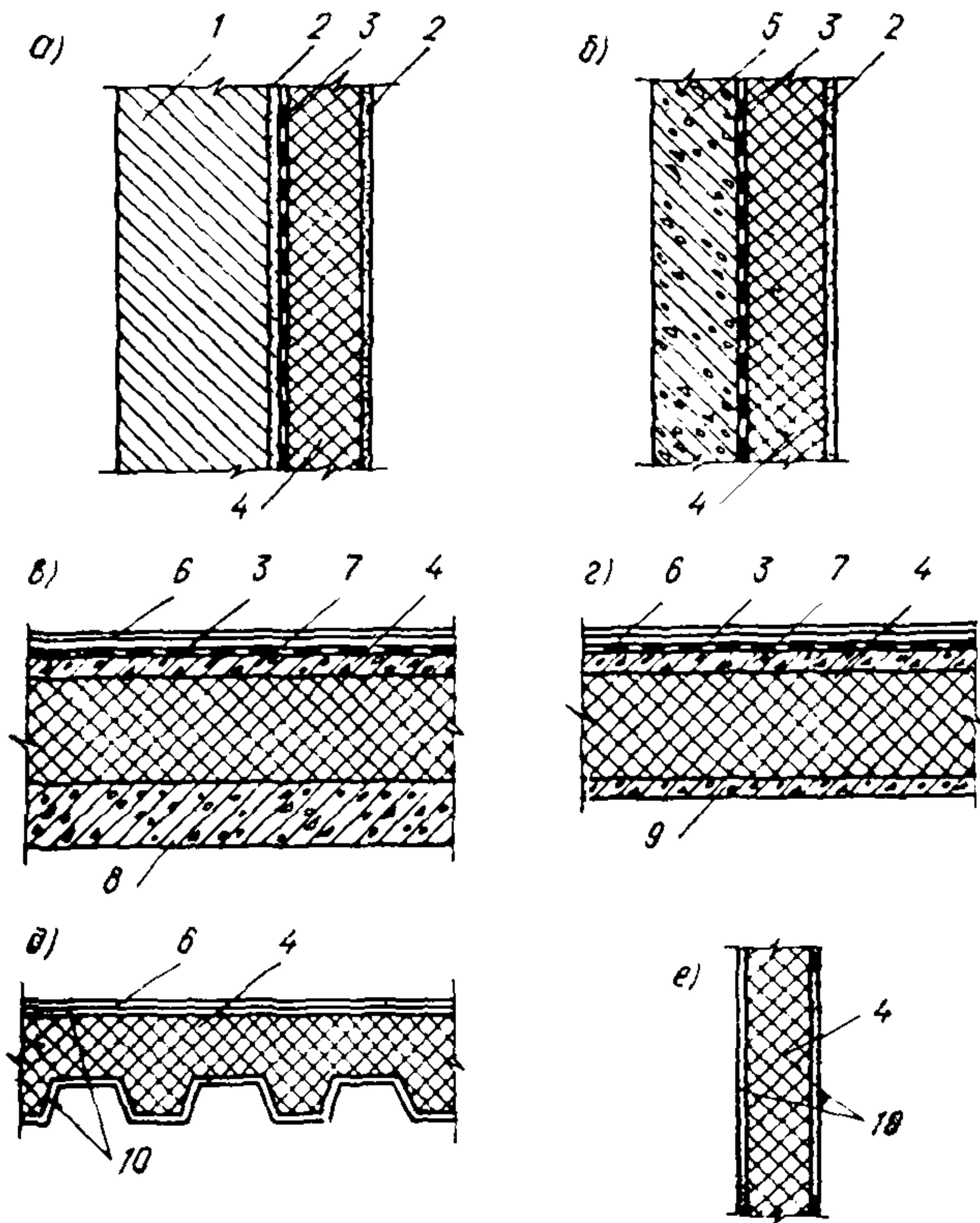
Рис. 6. Схемы ограждающих конструкций зданий холодильников
