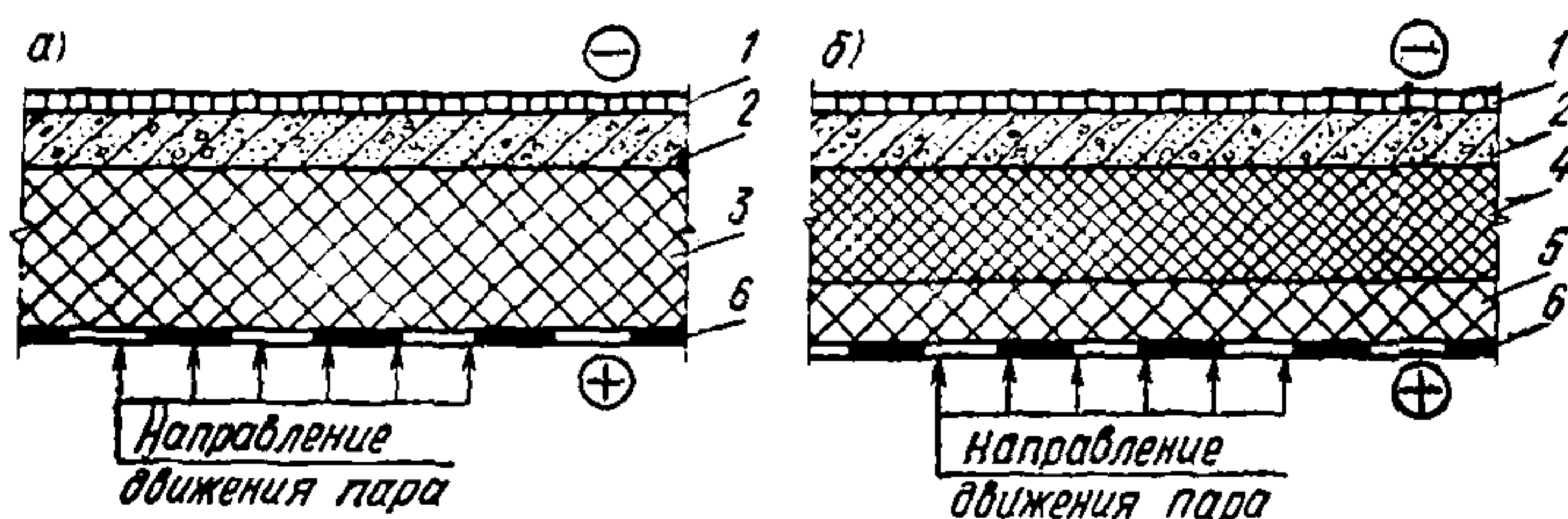
Рис. 8. Расчетная схема для определения сопротивления паропроницанию R_{\text{пи}}^{\text{тр}} конструкций обогреваемых полов
