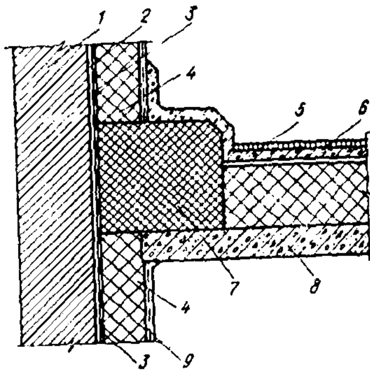
Рис. 1. Примыкание междуэтажных перекрытий к наружным стенам
