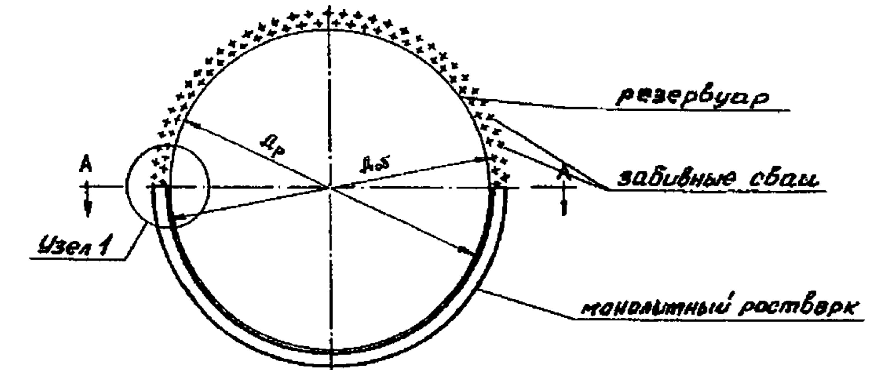
а). План фундамента
