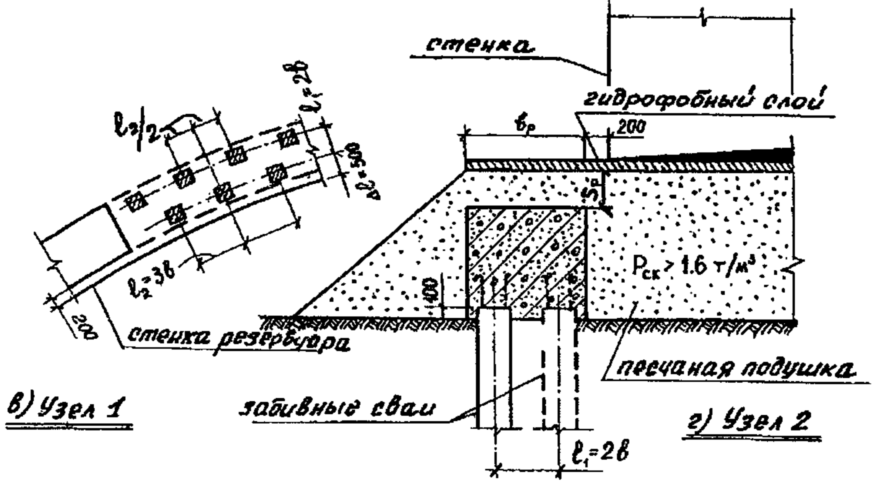
Рис. I Конструкция кольцевого фундамента
