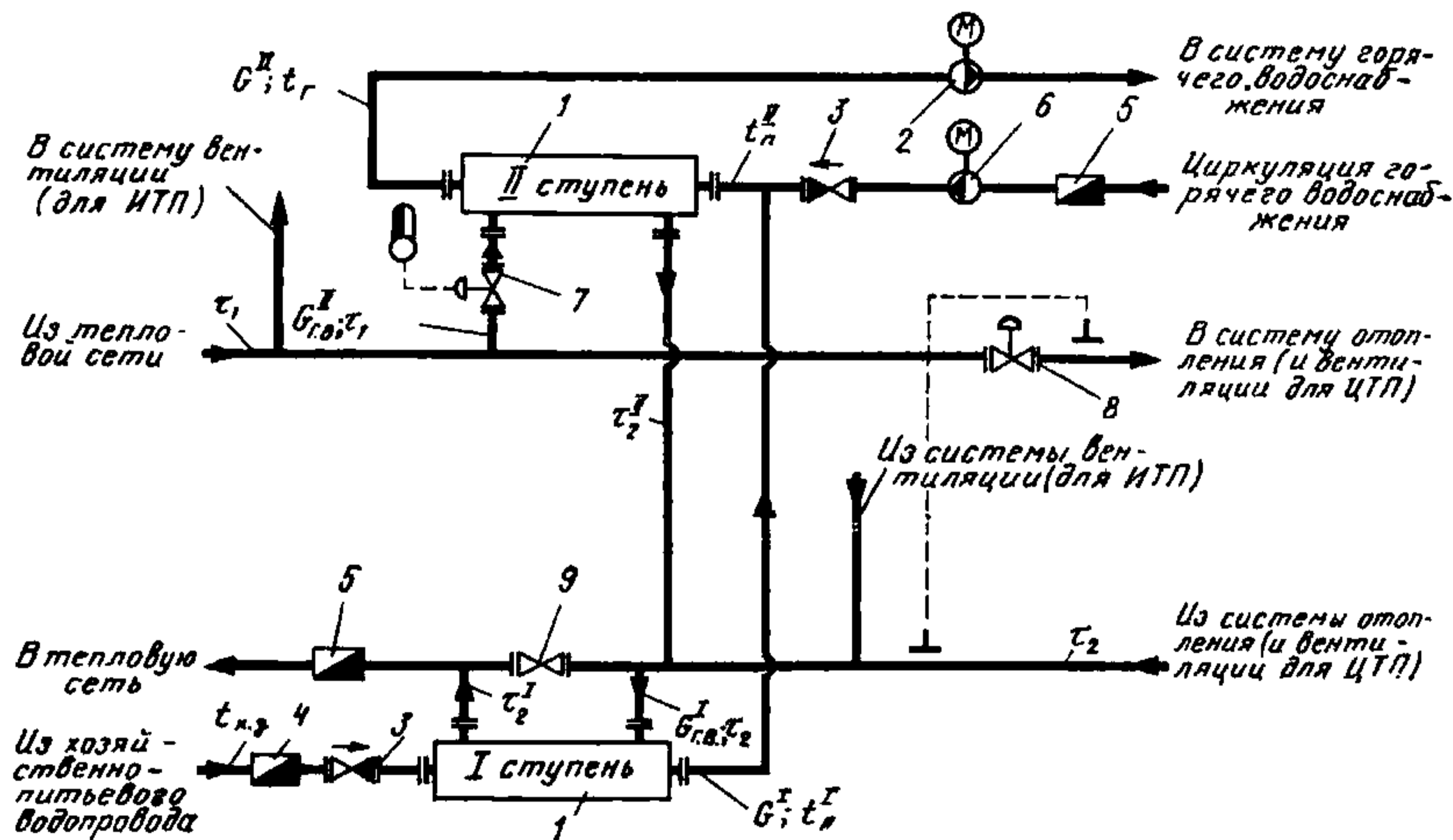
Рис. 2. Двухступенчатая смешанная схема присоединения водонагревателей горячего водоснабжения
