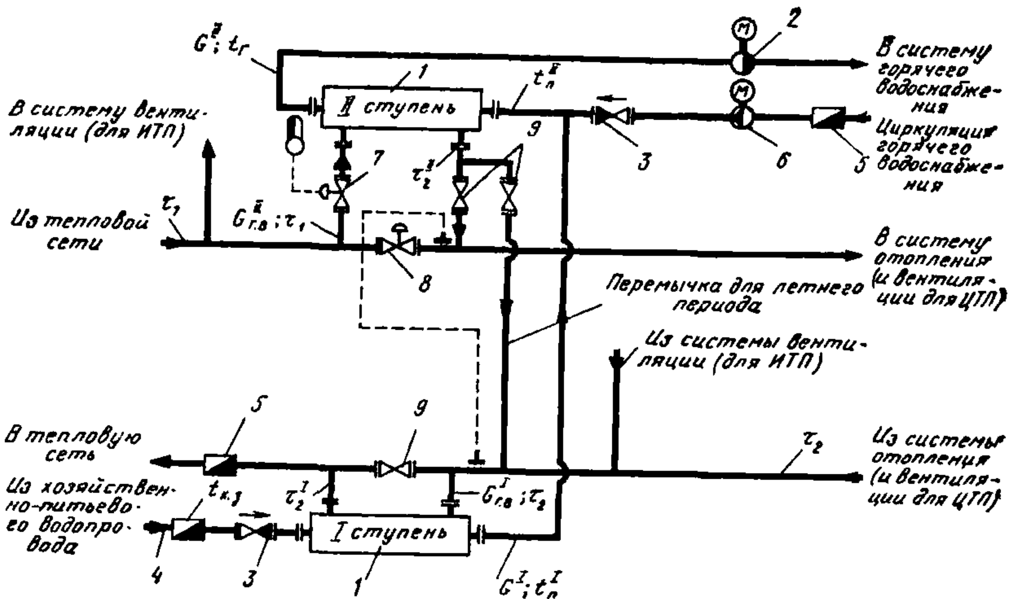
Рис. 3. Двухступенчатая последовательная схема присоединения водонагревателей горячего водоснабжения
