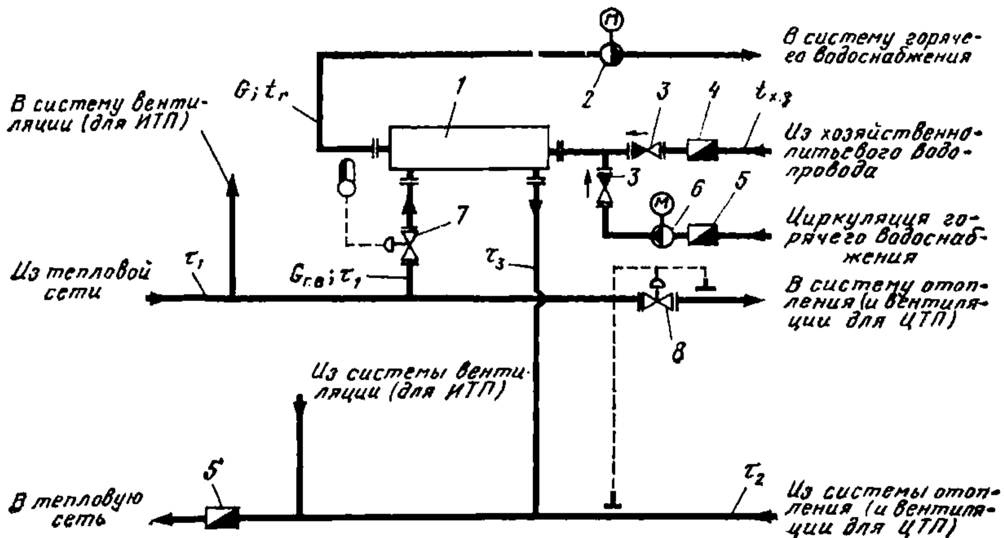
Рис. 1. Параллельная схема присоединения водонагревателей горячего водоснабжения
