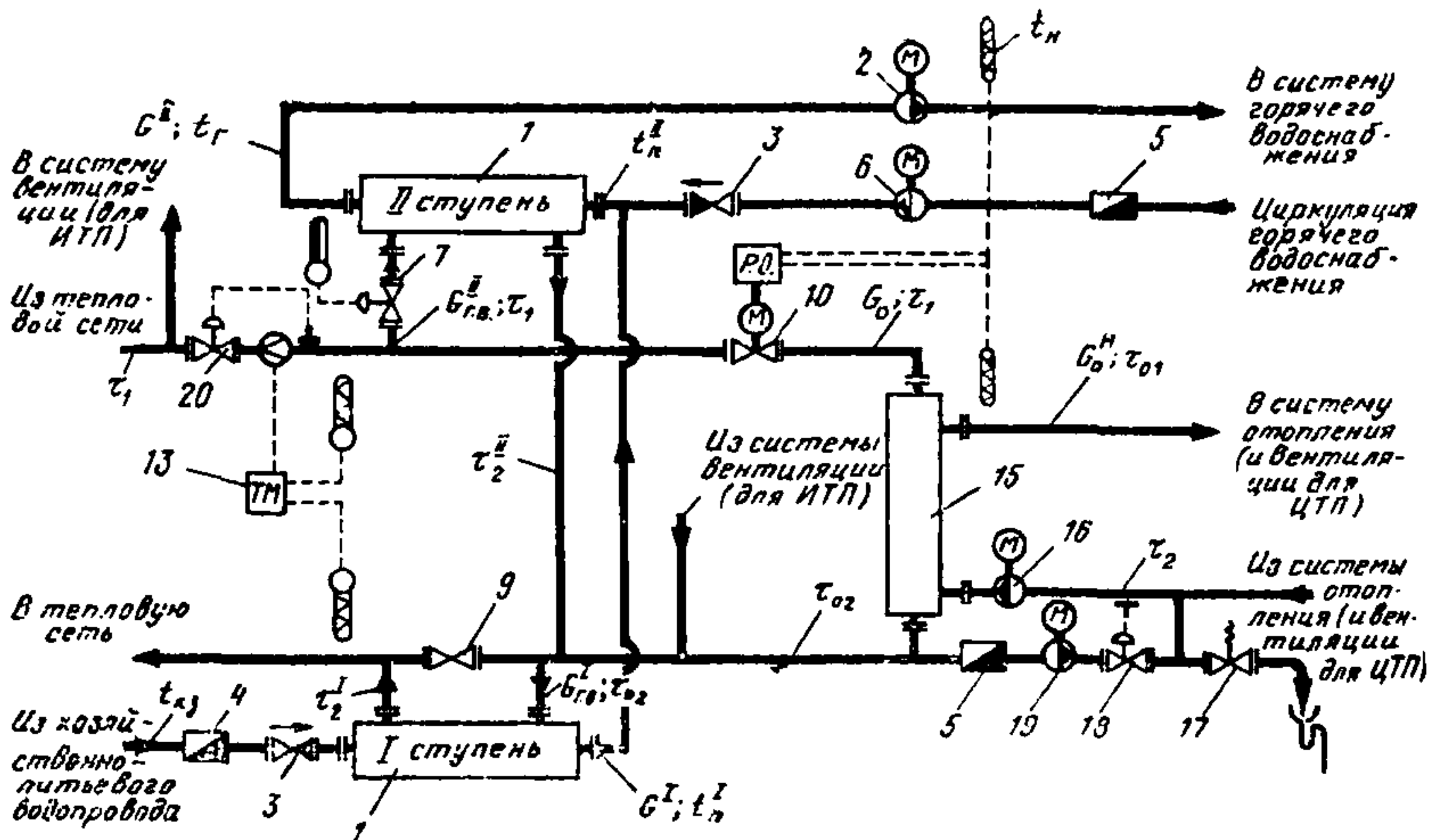
Рис. 9. Двухступенчатая смешанная схема присоединения водонагревателей горячего водоснабжения с ограничением максимального расхода воды из тепловой сети на ввод при применении регулятора расхода тепла на отопление с независимым присоединением системы отопления
