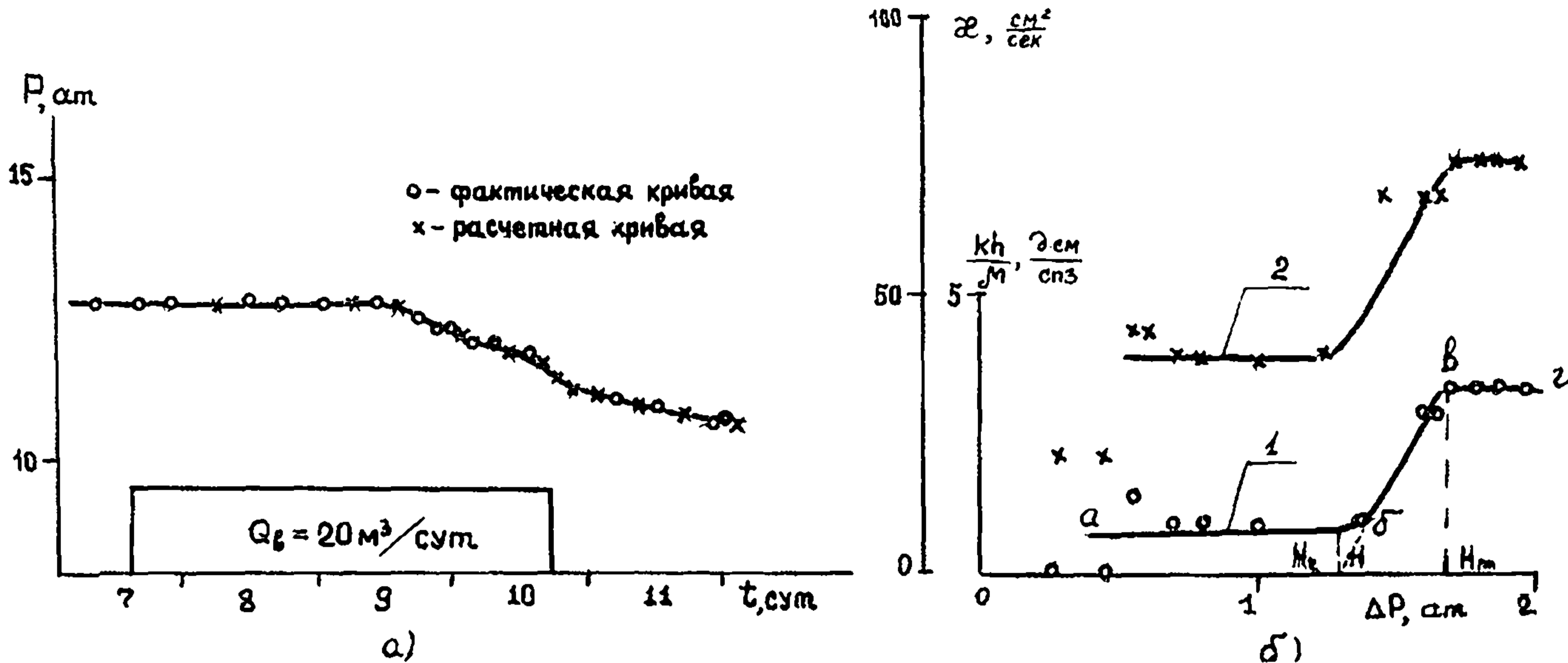
Рис. 28а) Кривая реагирования, полученная при исследовании скв. 1006 1010 Усинского месторождения методом гидропрослушивания б) реологические кривые фильтрации, построенные по результатам исследования скв. 1006-1010 1 - зависимость \frac{kh}{\mu} от \Delta P ; 2 - зависимость \zeta от \Delta P , - соответственно градиенты динамического давления сдвига начала и полного разрушения структуры нефти
