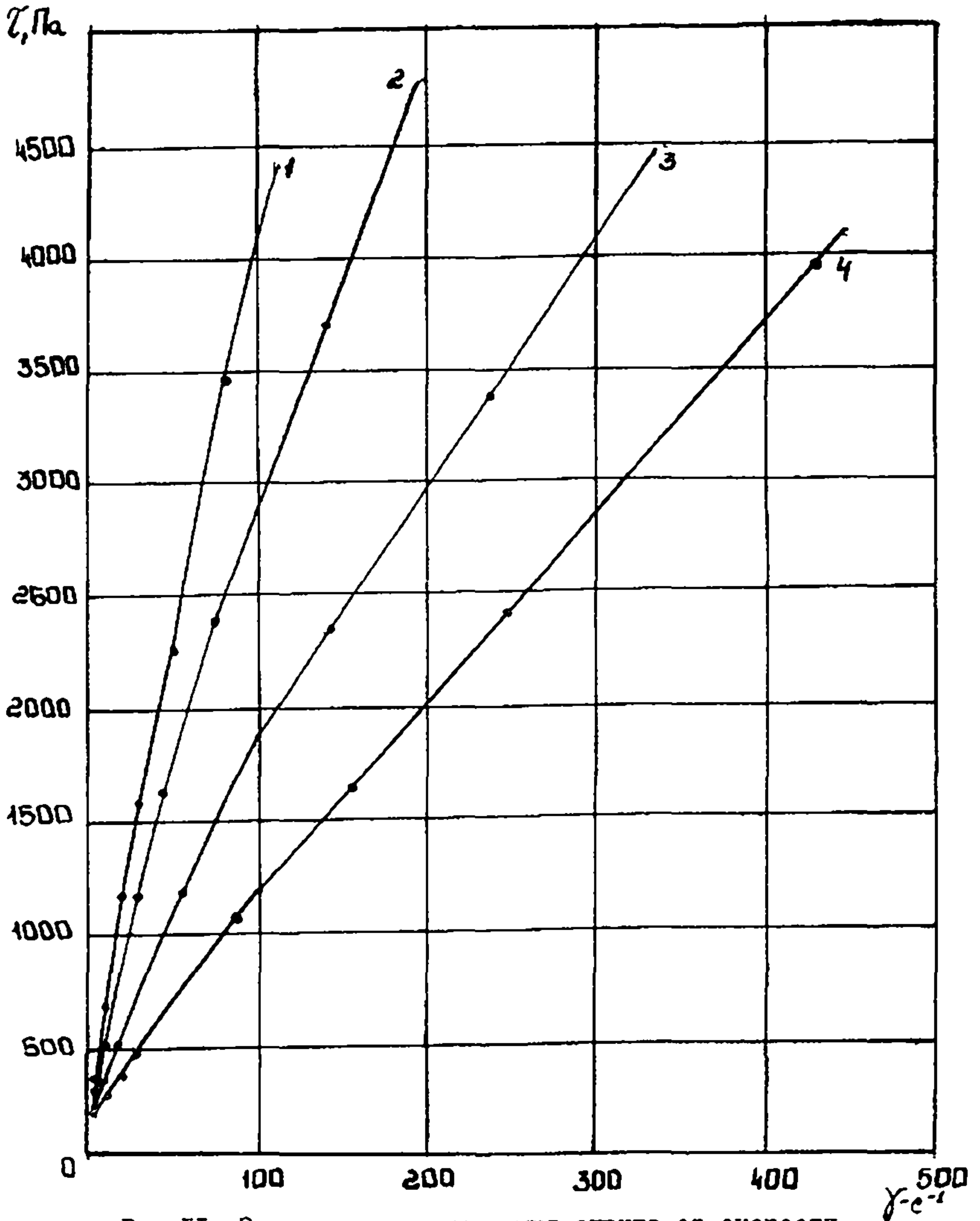
Рис. II. Зависимость напряжения сдвига от скорости сдвига Юнлорской нефти для температур: I-2°C; 2-4°C; 3-15°C; 4-20°C
