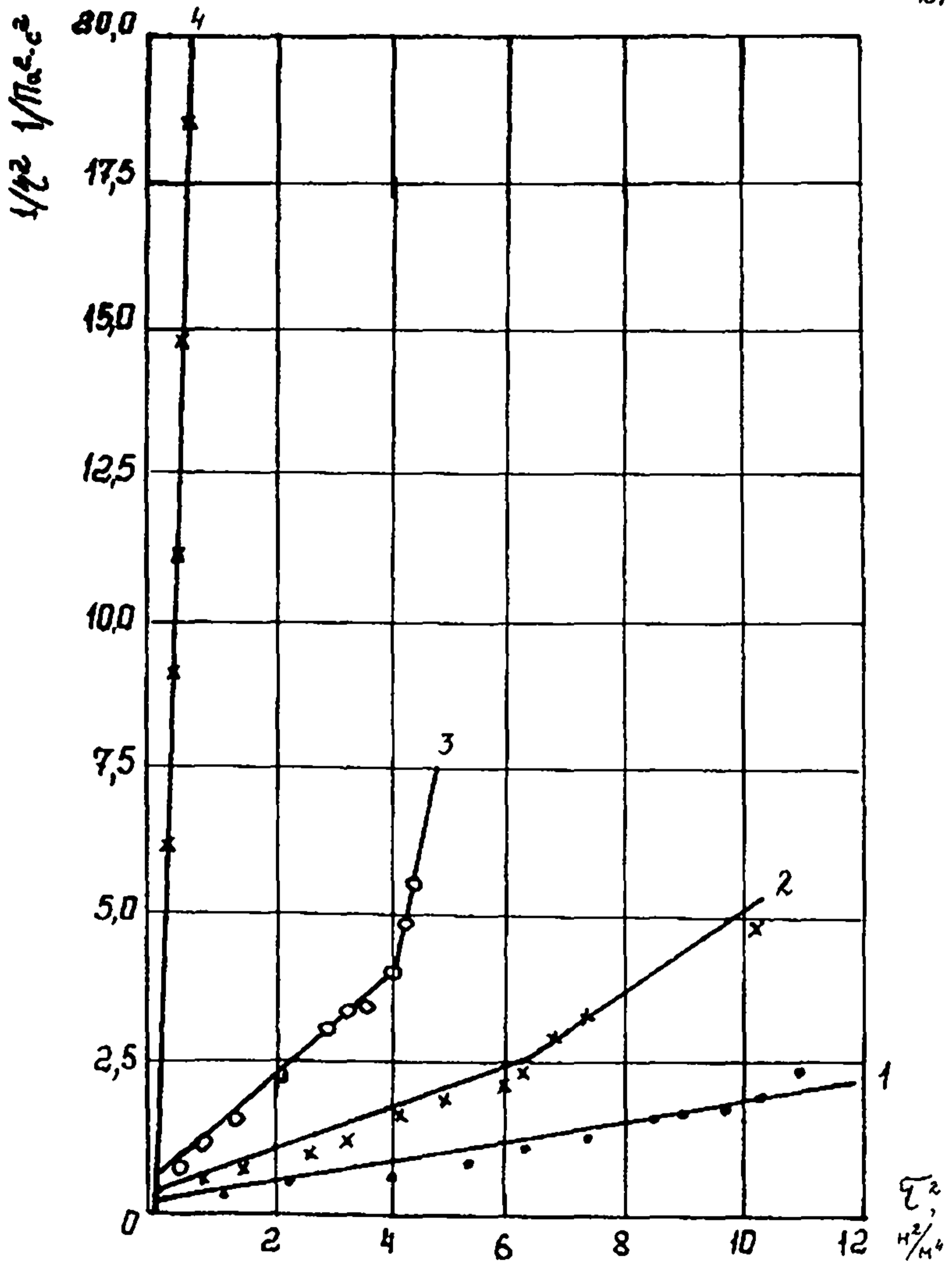
Рис. 9. Реограмма нефти Возейского месторождения (дегазированная)
