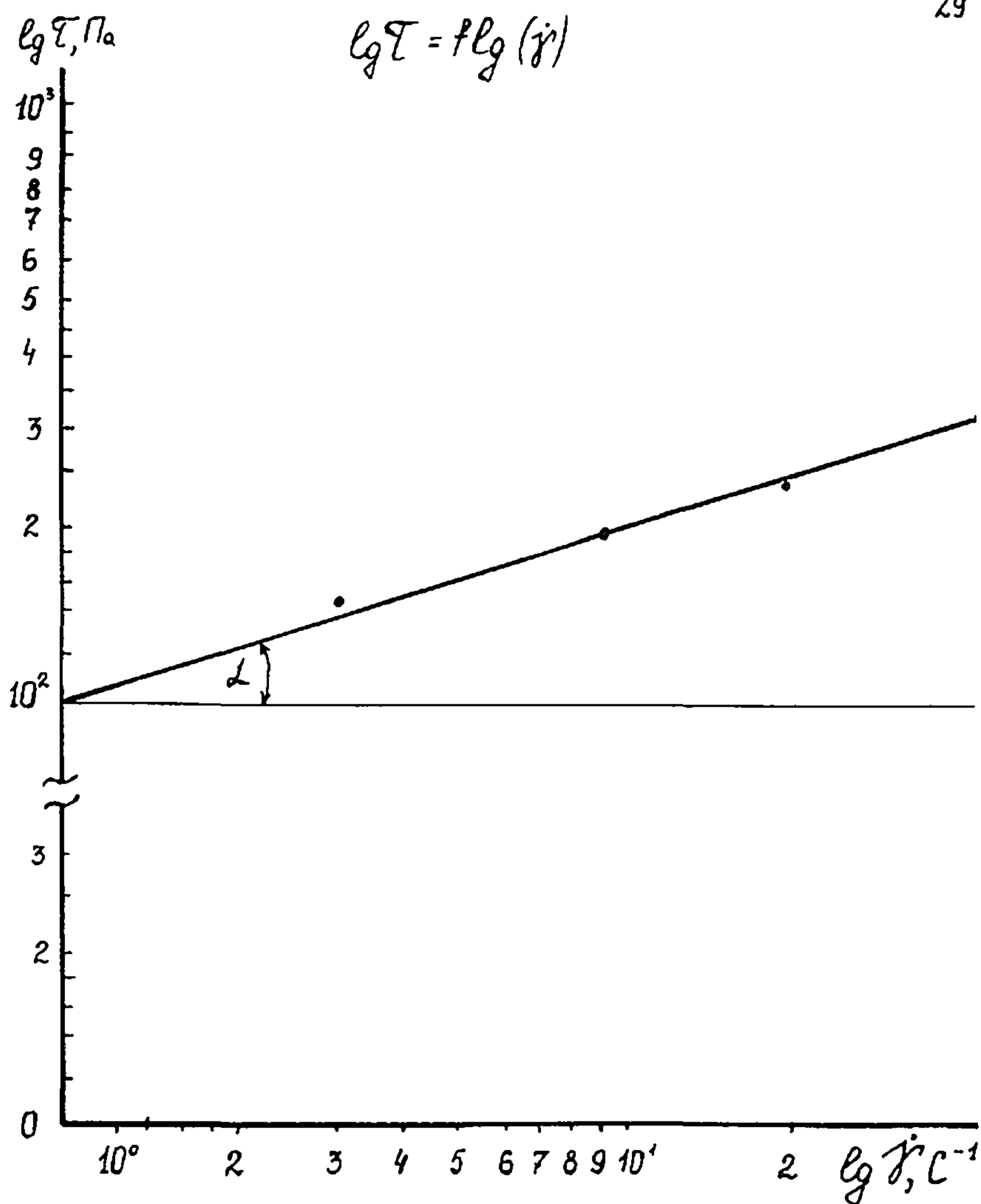
Рис. 12. Реограмма Яулорской нефти
