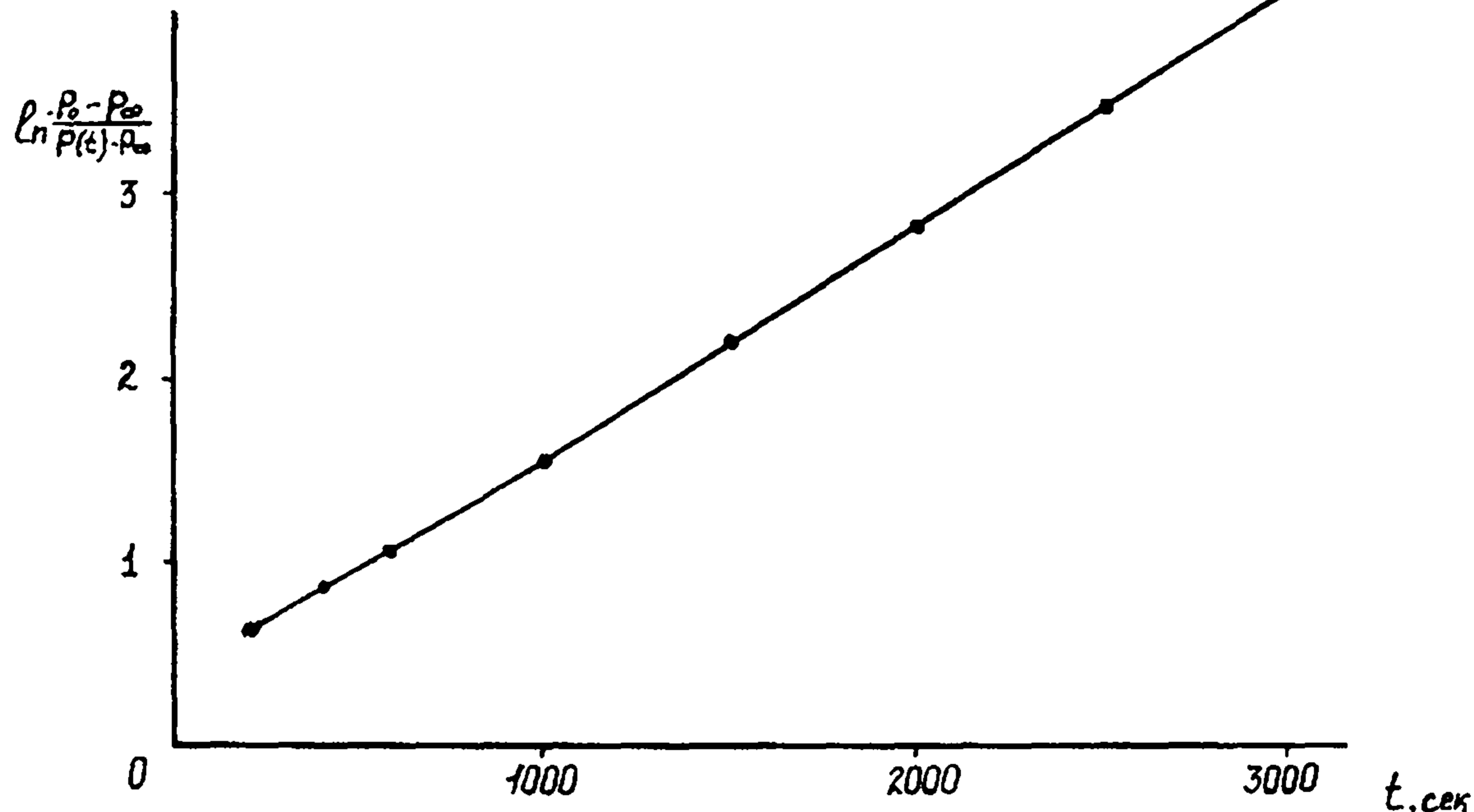
Рис.21. Вспомогательная зависимость для определения времени релаксации по данным Усинской нефти
