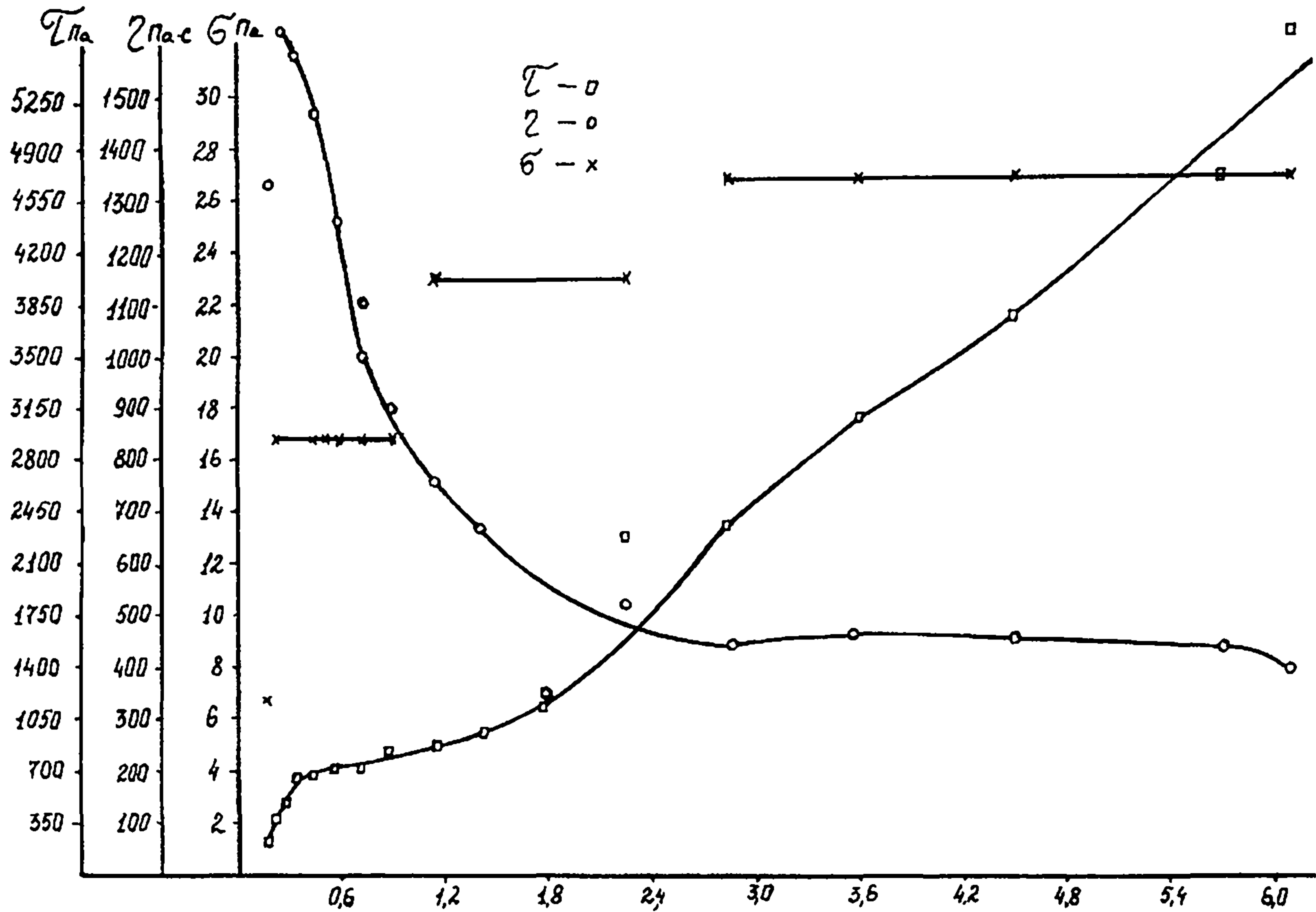
Рис. 13. Реологические зависимости \tau , \dot{\gamma} , G для нефти Усинского месторождения, t = 20^\circ\text{C}
