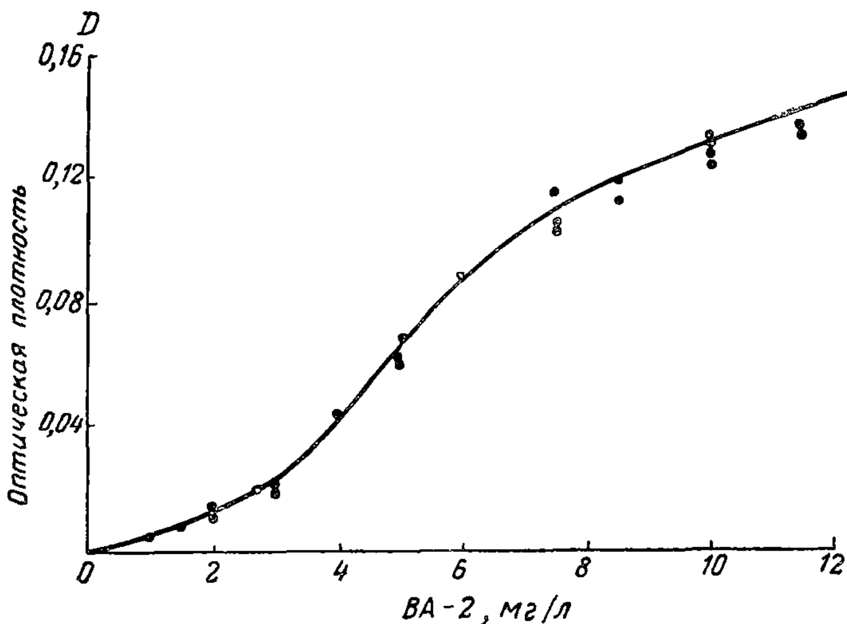
Рис 22 Калибровочная кривая для определения ВА-2
