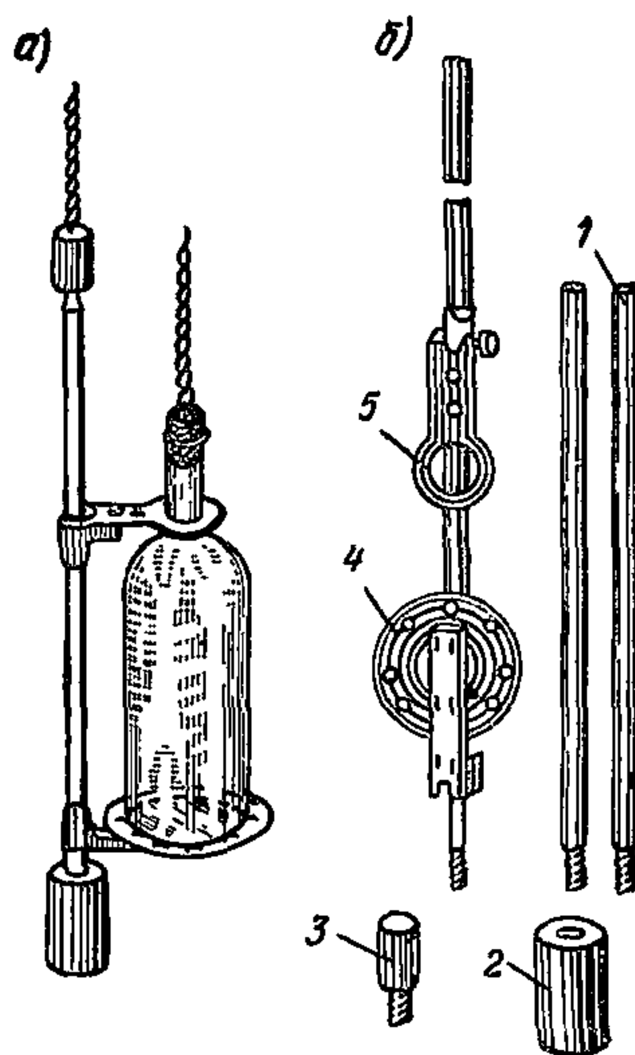
Рис. 3. Штанга с ручкой для взятия проб воды:
