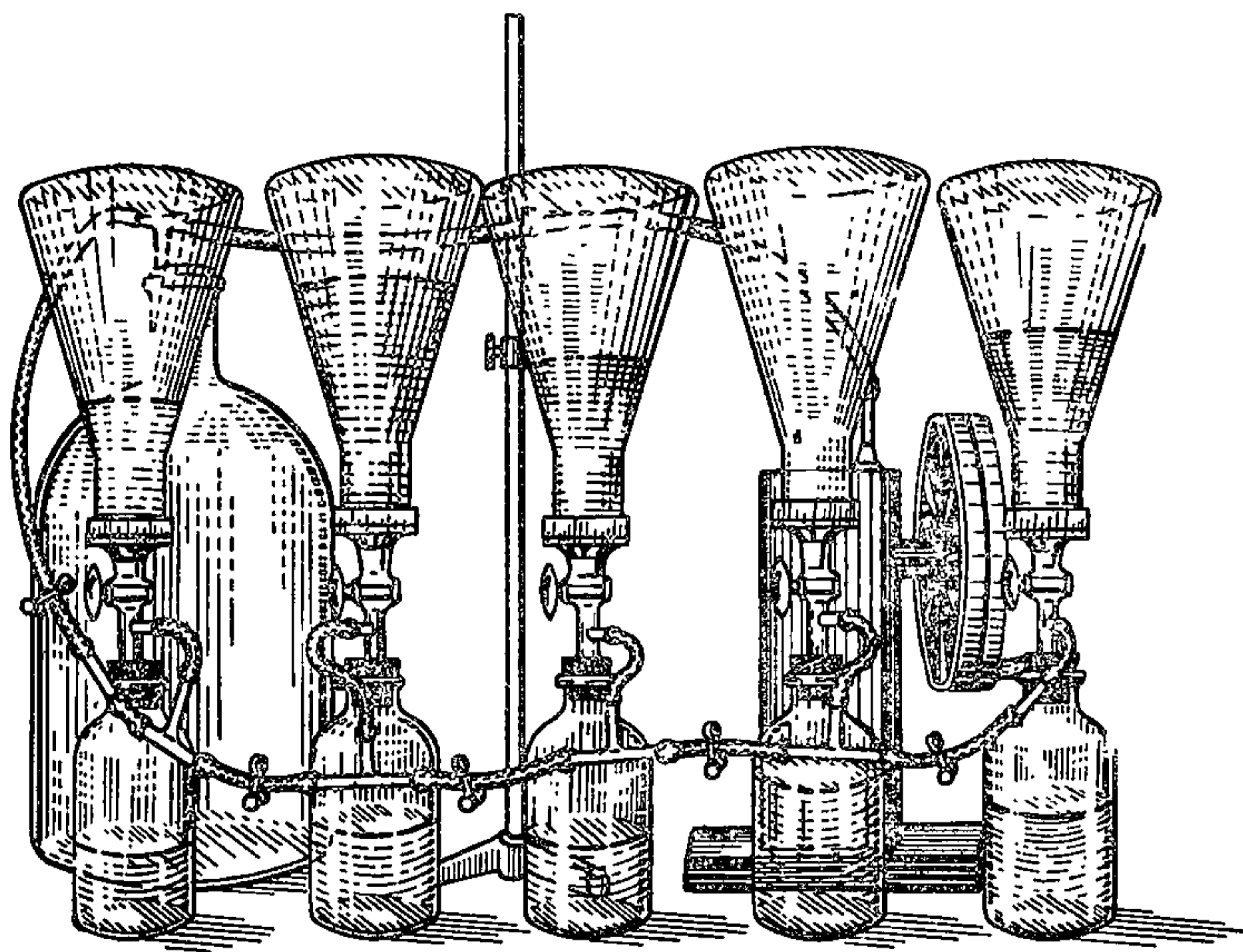
Рис. 11. Установка для определения взвешенных веществ
