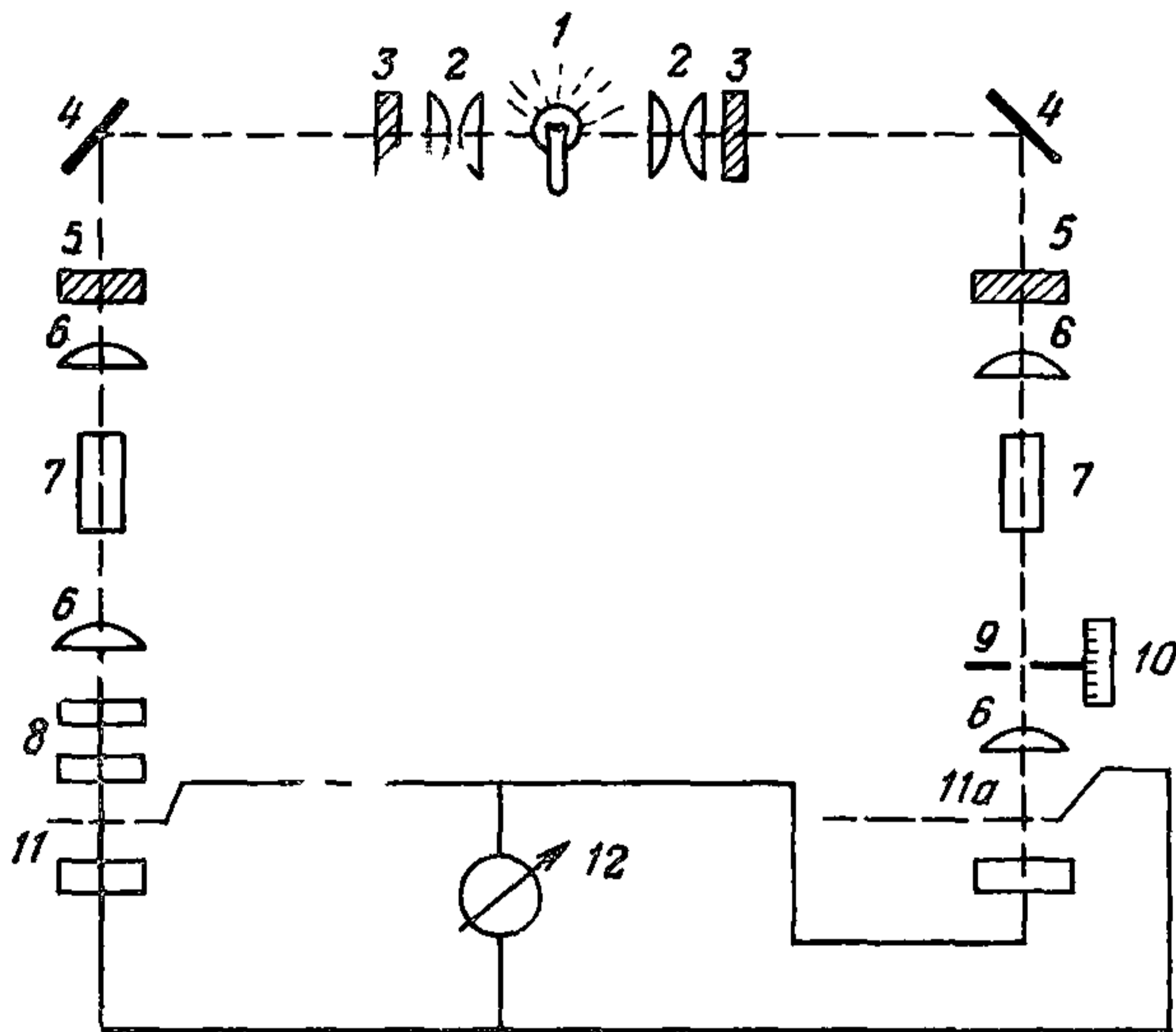
Рис. 19. Схема фотоколориметра ФЭК-М
