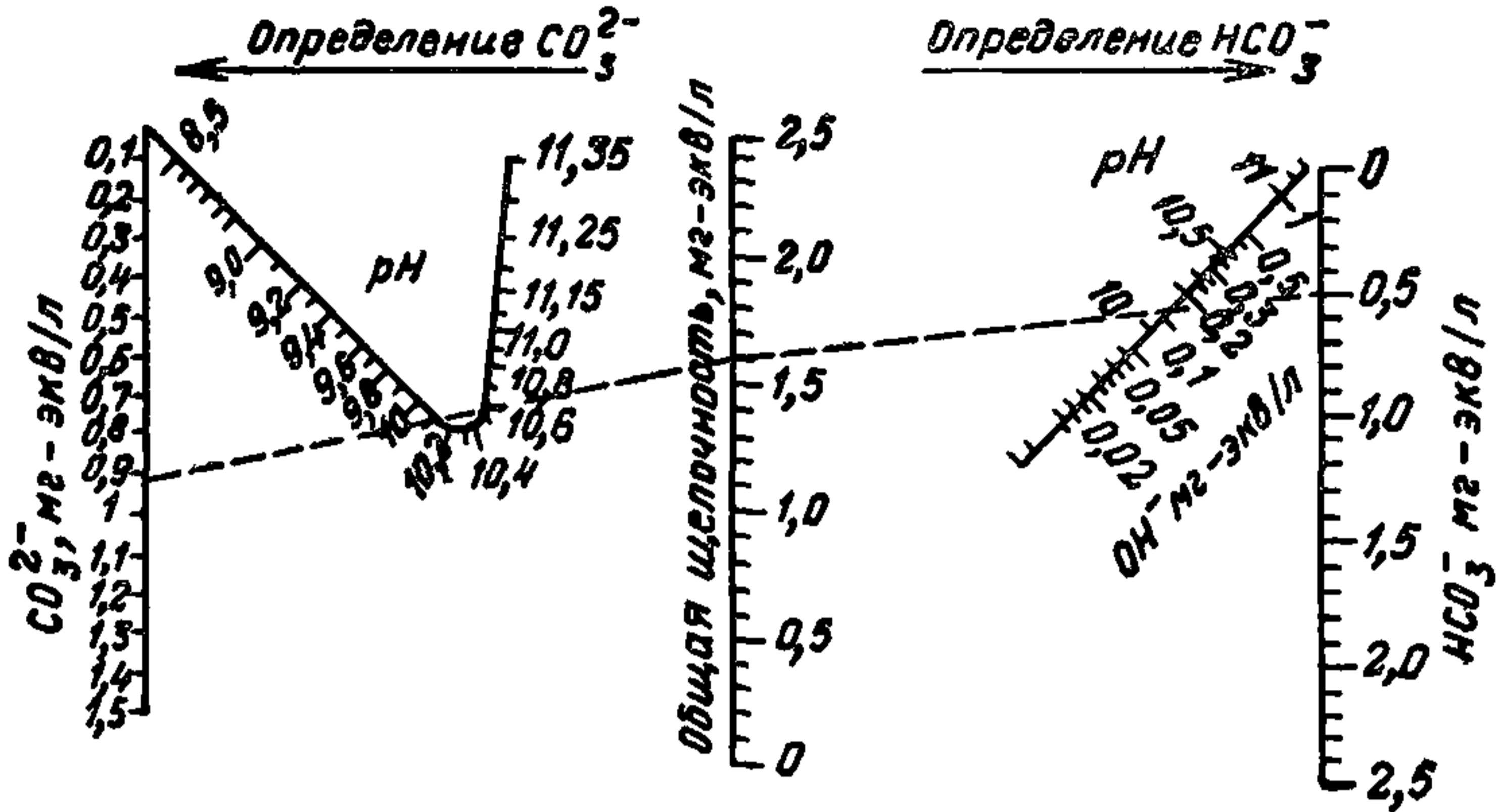
Рис. 12. Номограмма для определения трех форм щелочи ( \text{НСО}_3^- , \text{СО}_3^{2-} , \text{ОН}^- )
