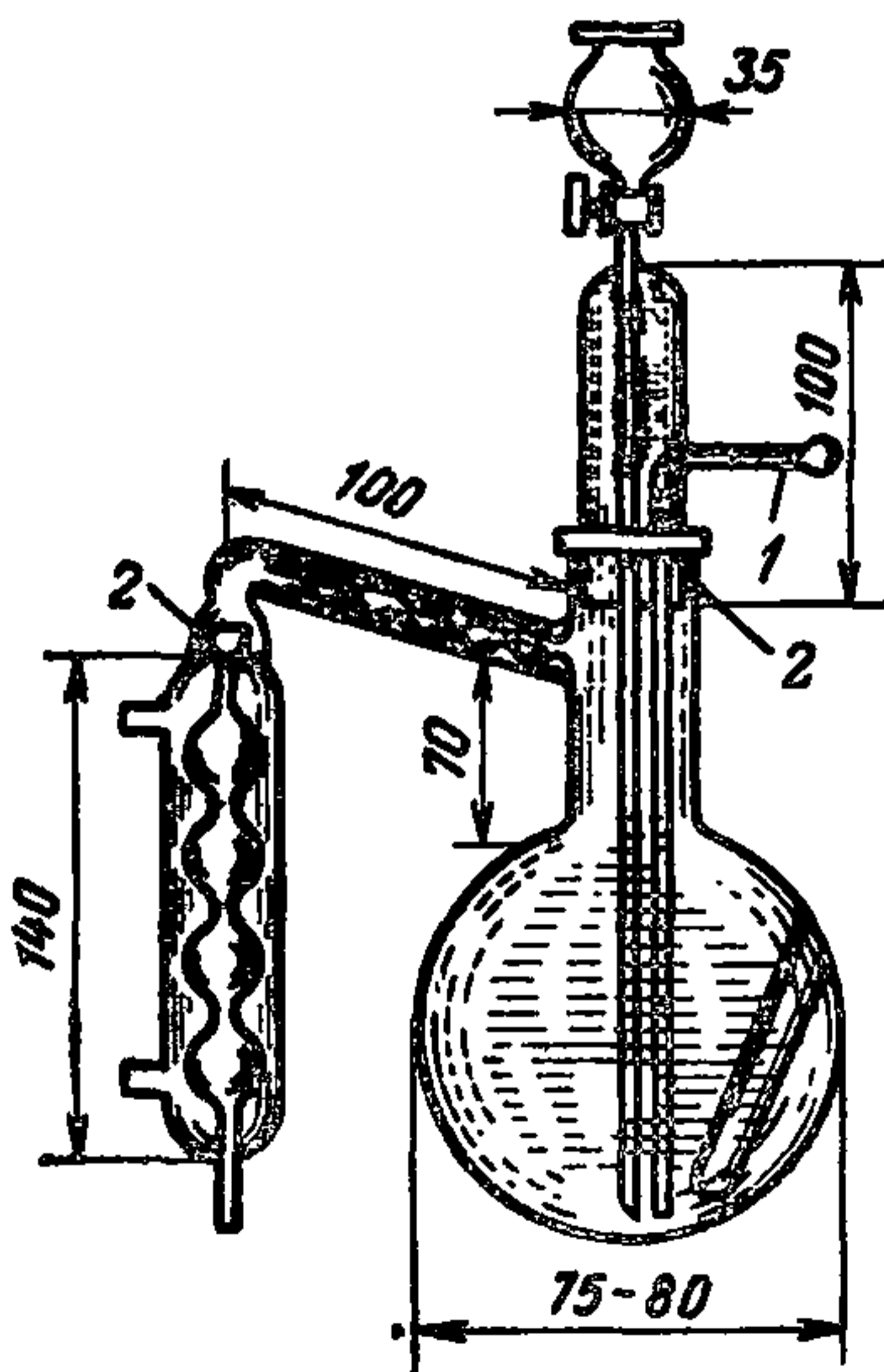
Рис. 16. Аппарат для отгонки фтора
