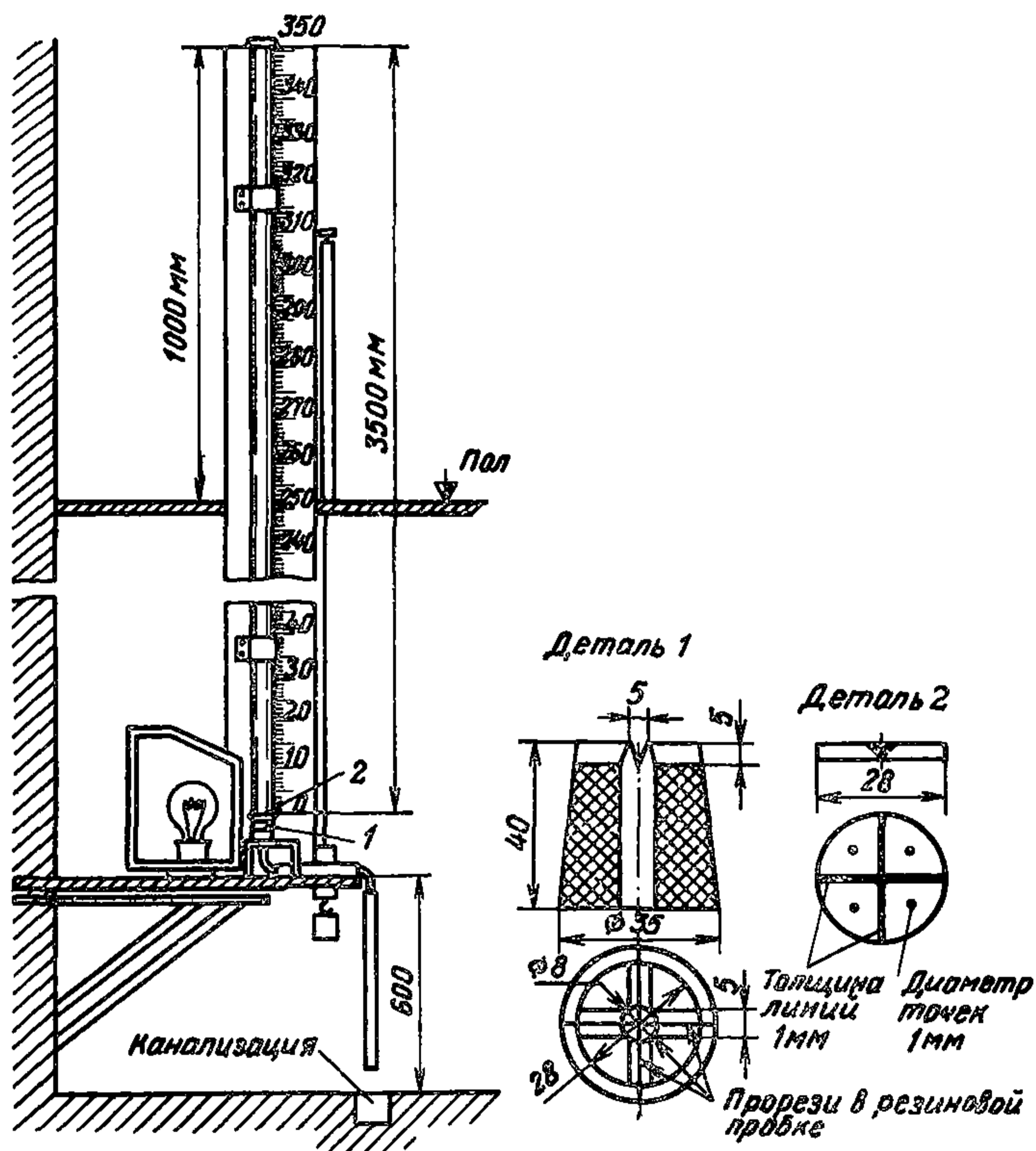
Рис. 9. Прибор для определения прозрачности воды по кресту
