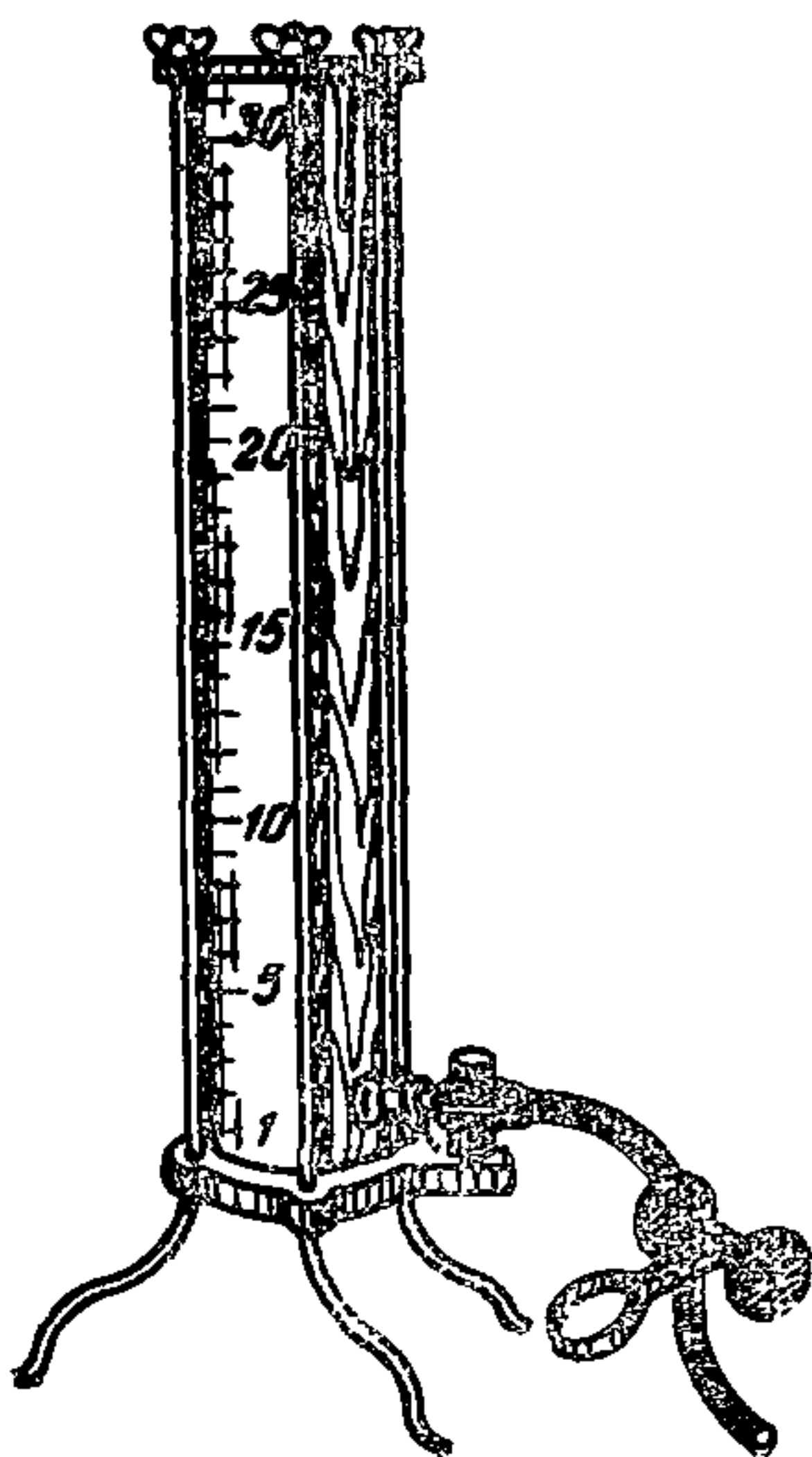
Рис. 7. Цилиндр для определения прозрачности воды
