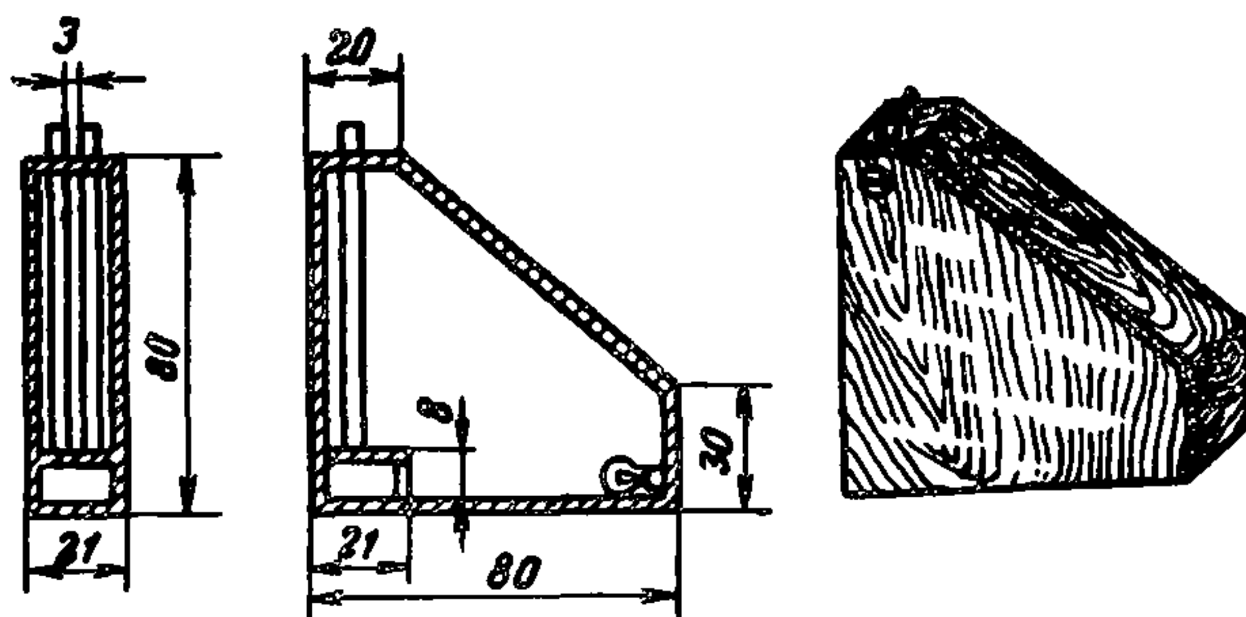
Рис. 10. Мутномер Бейлиса
