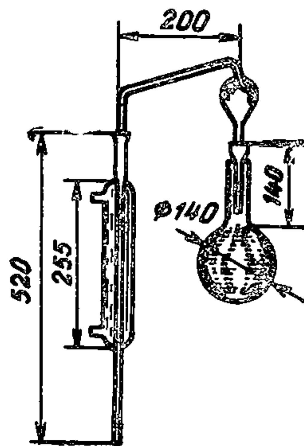
Рис. 15. Прибор для отгонки аммиака
