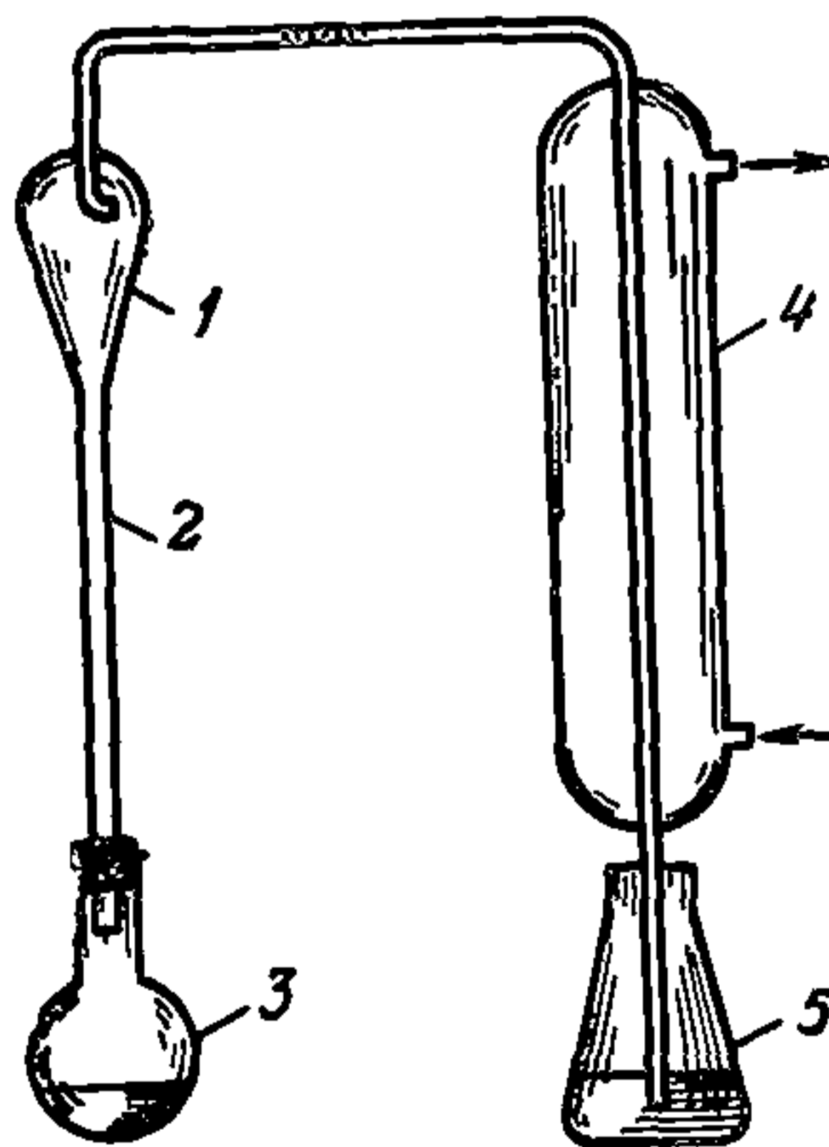
Рис. 18. Прибор для гидролиза полиакриламида и отгонка аммиака
