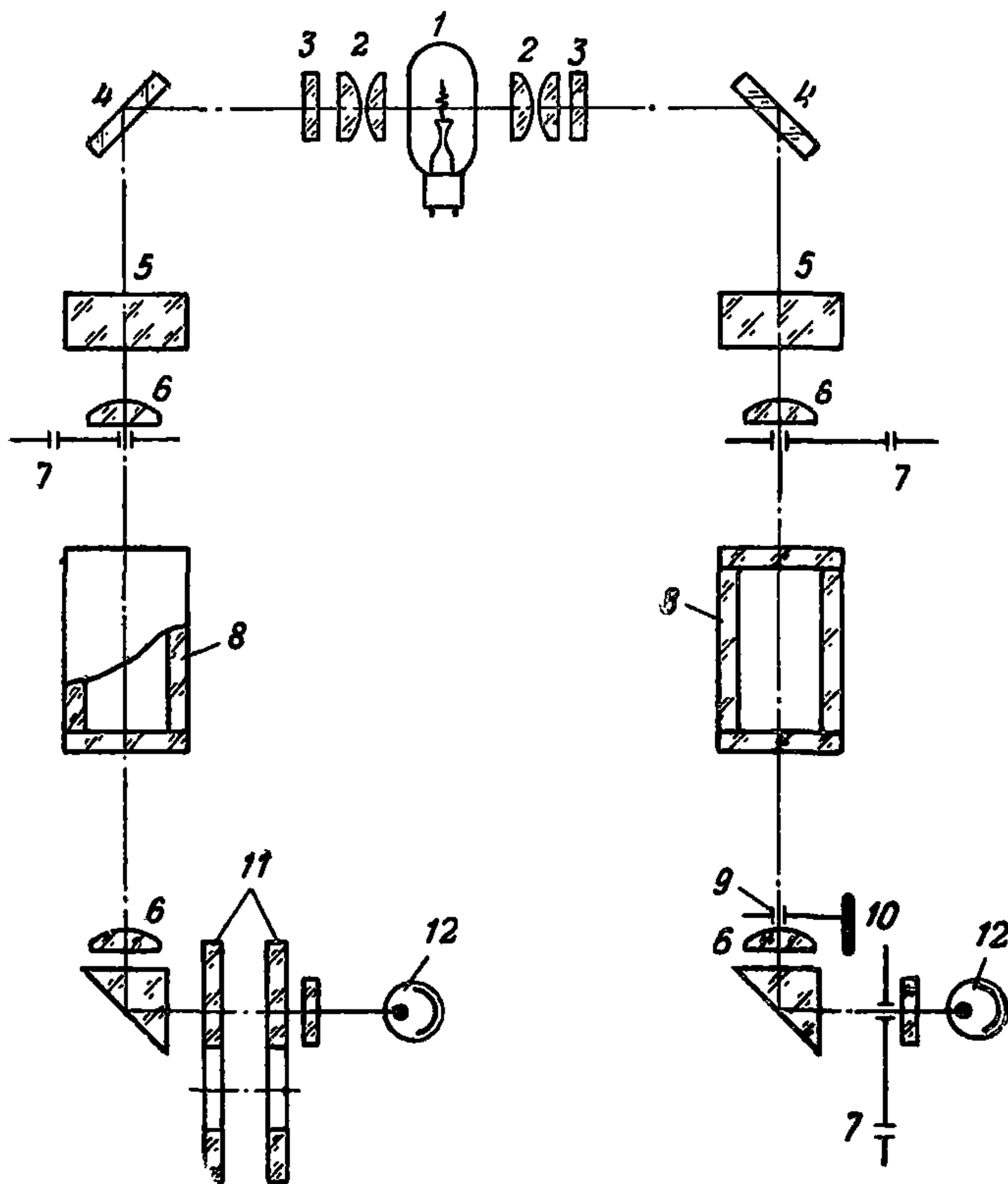
Рис. 20. Схема фотоколориметра ФЭК-Н
