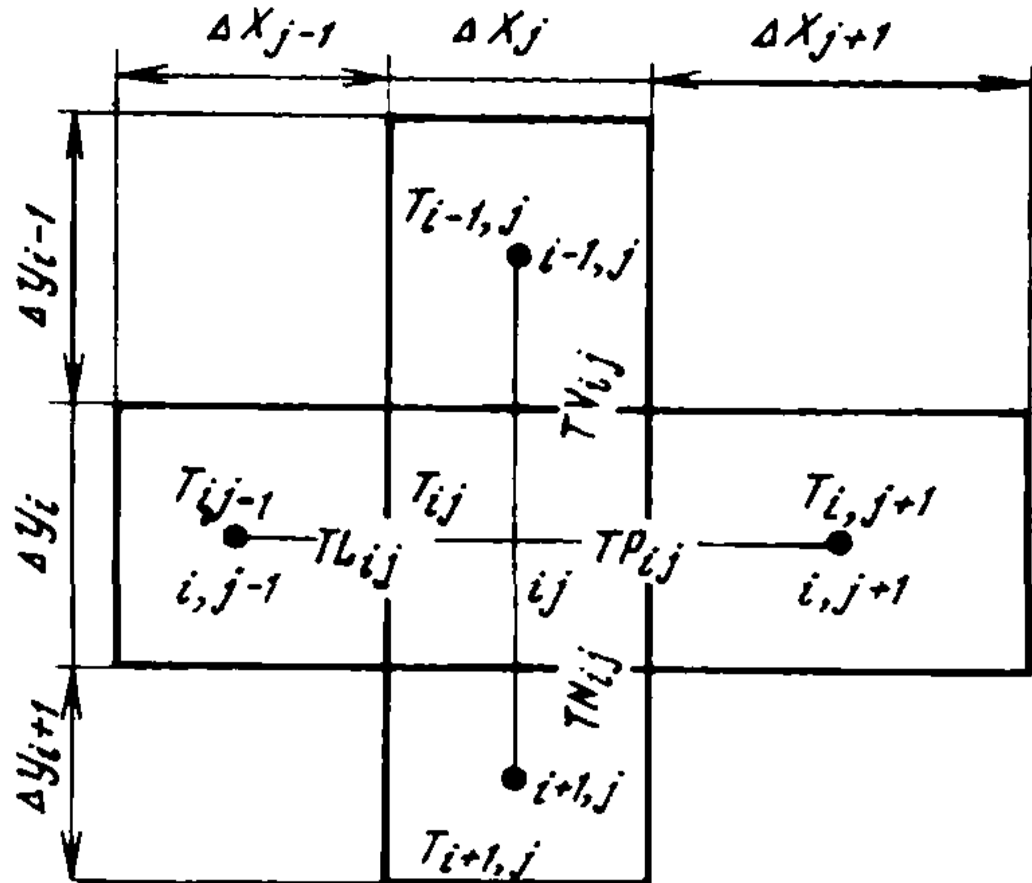
Рис. 2. Элемент неравномерной сетки
