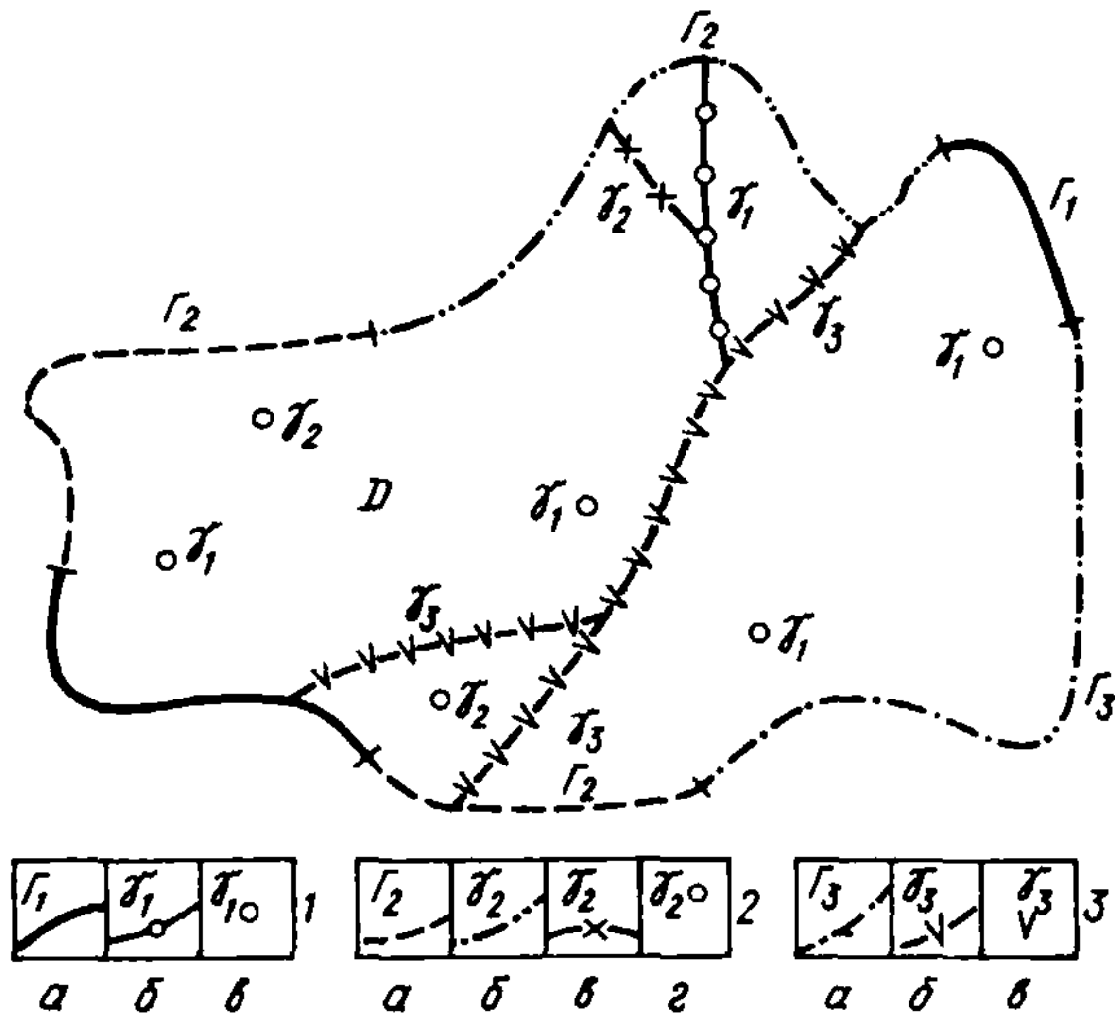
Рис. 1. Фильтрационная схема
