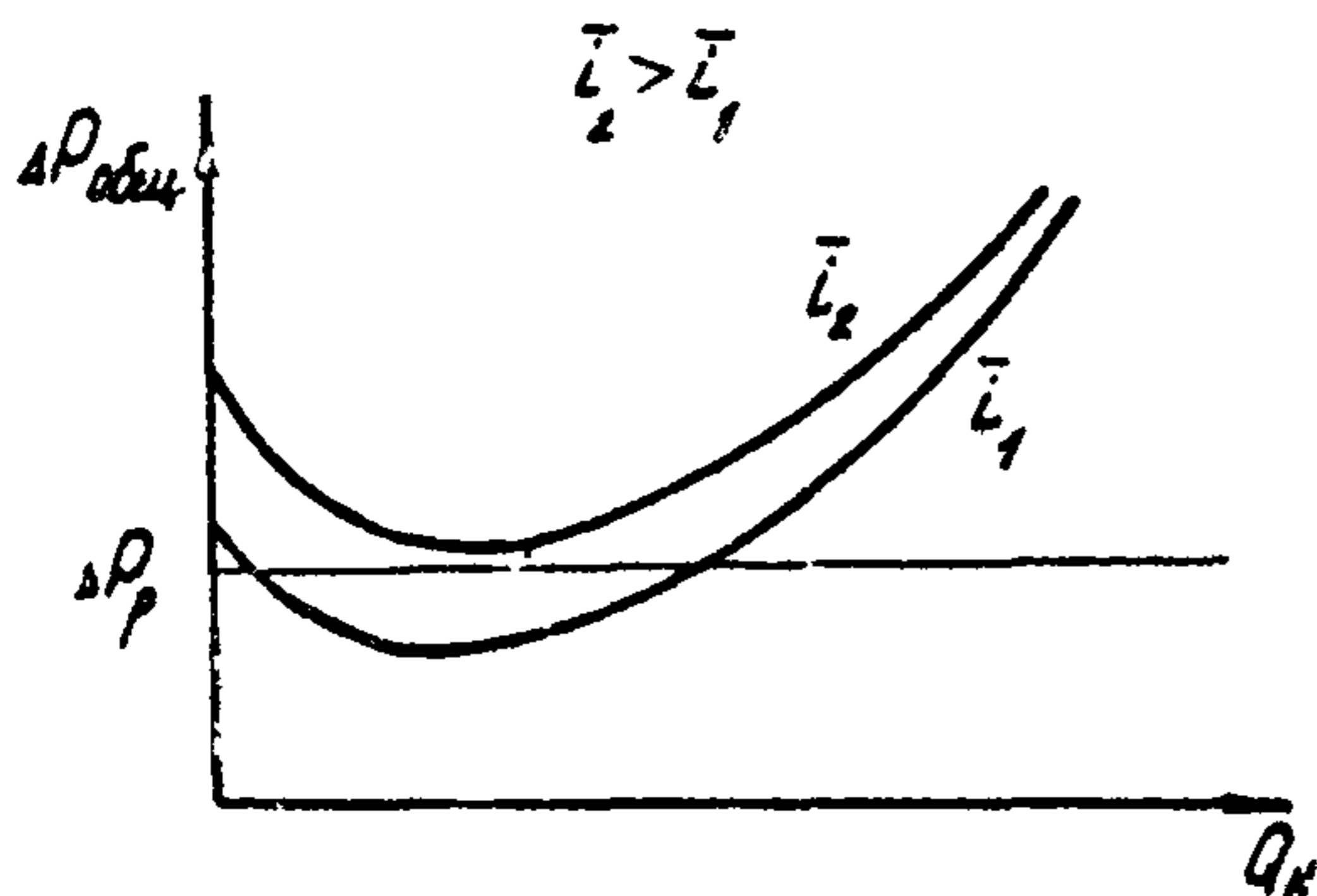
Рис. I1. Изменение гидравлической характеристики трубопровода путем сглаживания профиля трассы ( d = const, \Gamma_{\varphi} = const )
