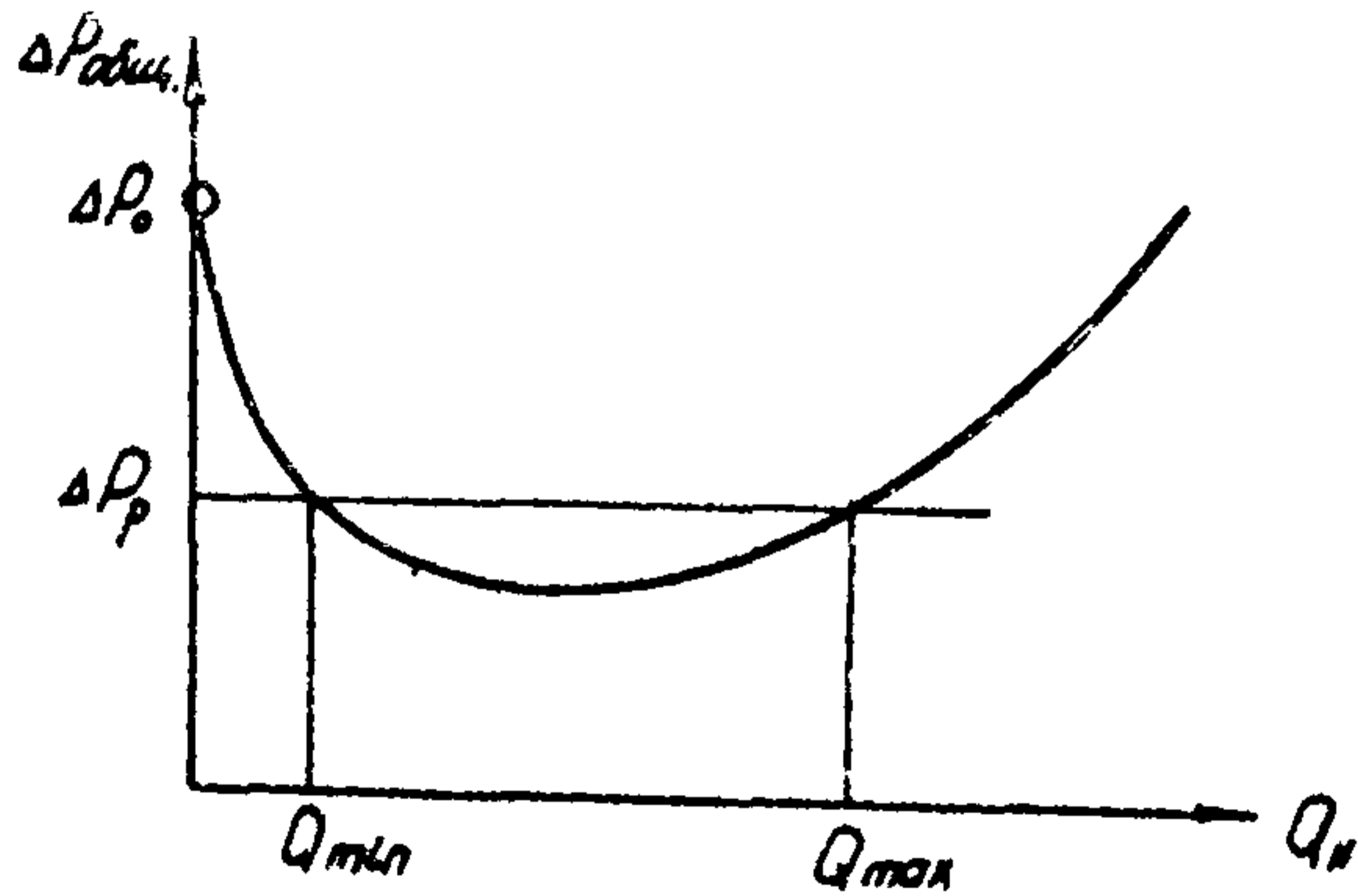
Рис. 10. Определение диапазона изменения пропускной способности трубопровода ( d = const , \tau_p = const )
