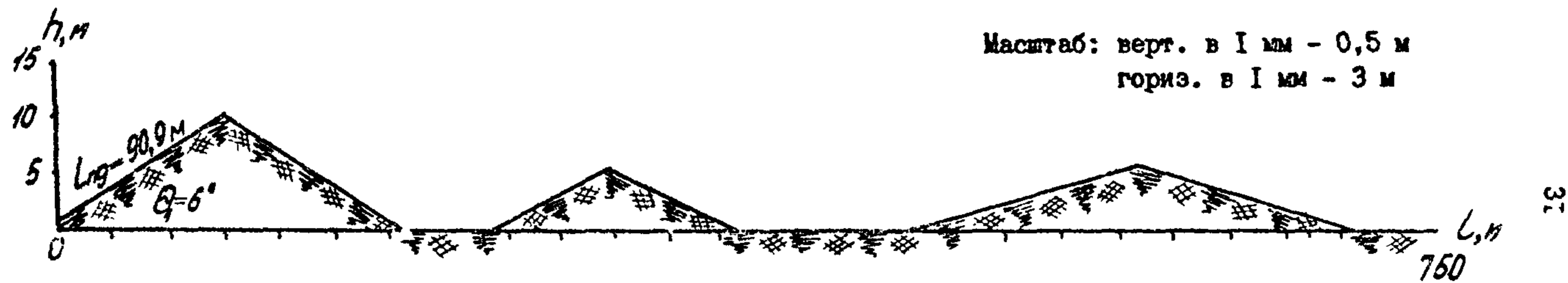
Рис. 8. Продольный профиль трассы пролегания трубопровода
