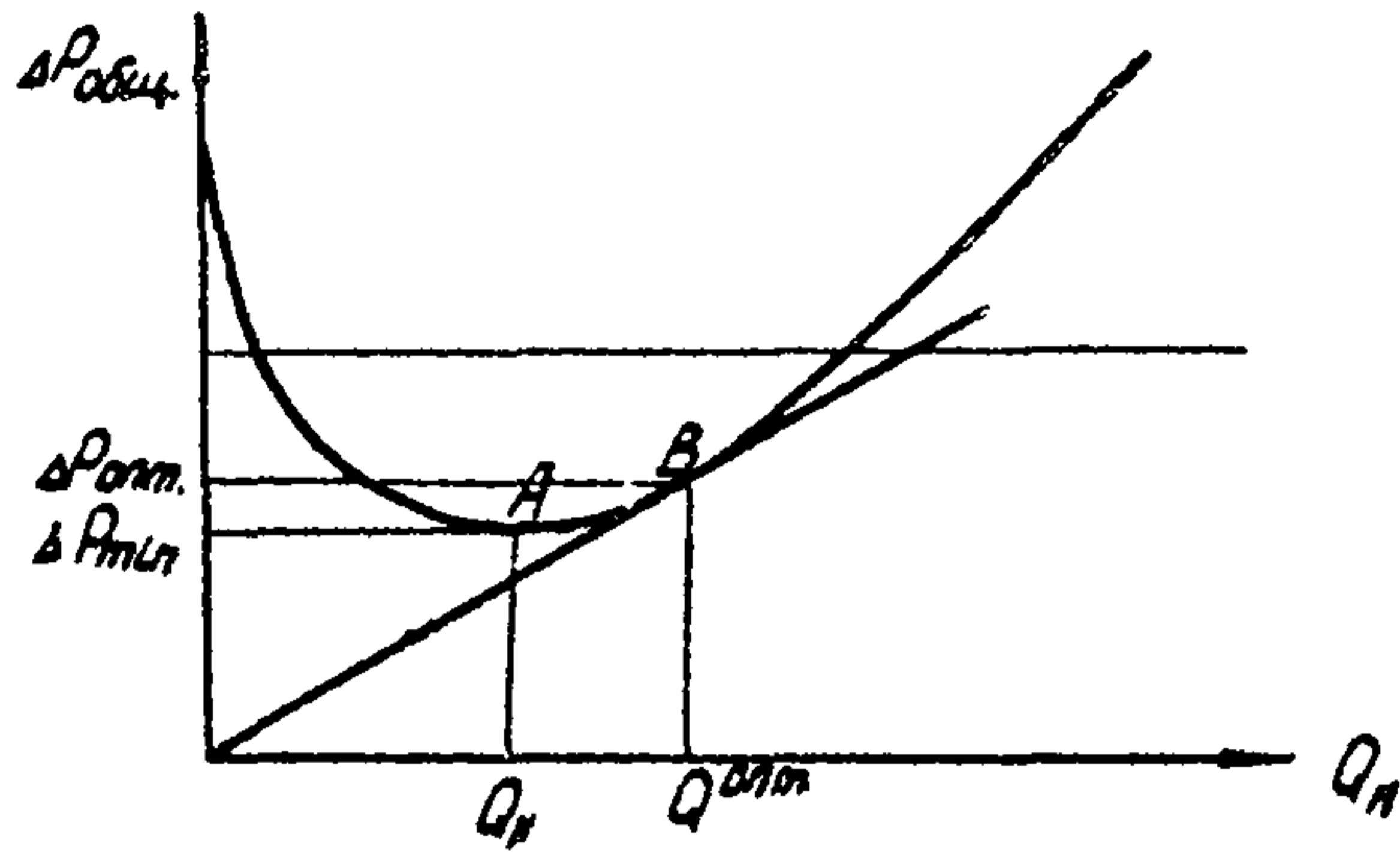
Рис. 9. Определение оптимальных условий эксплуатации "рельефного" трубопровода ( d = const , \tau_p = const )
