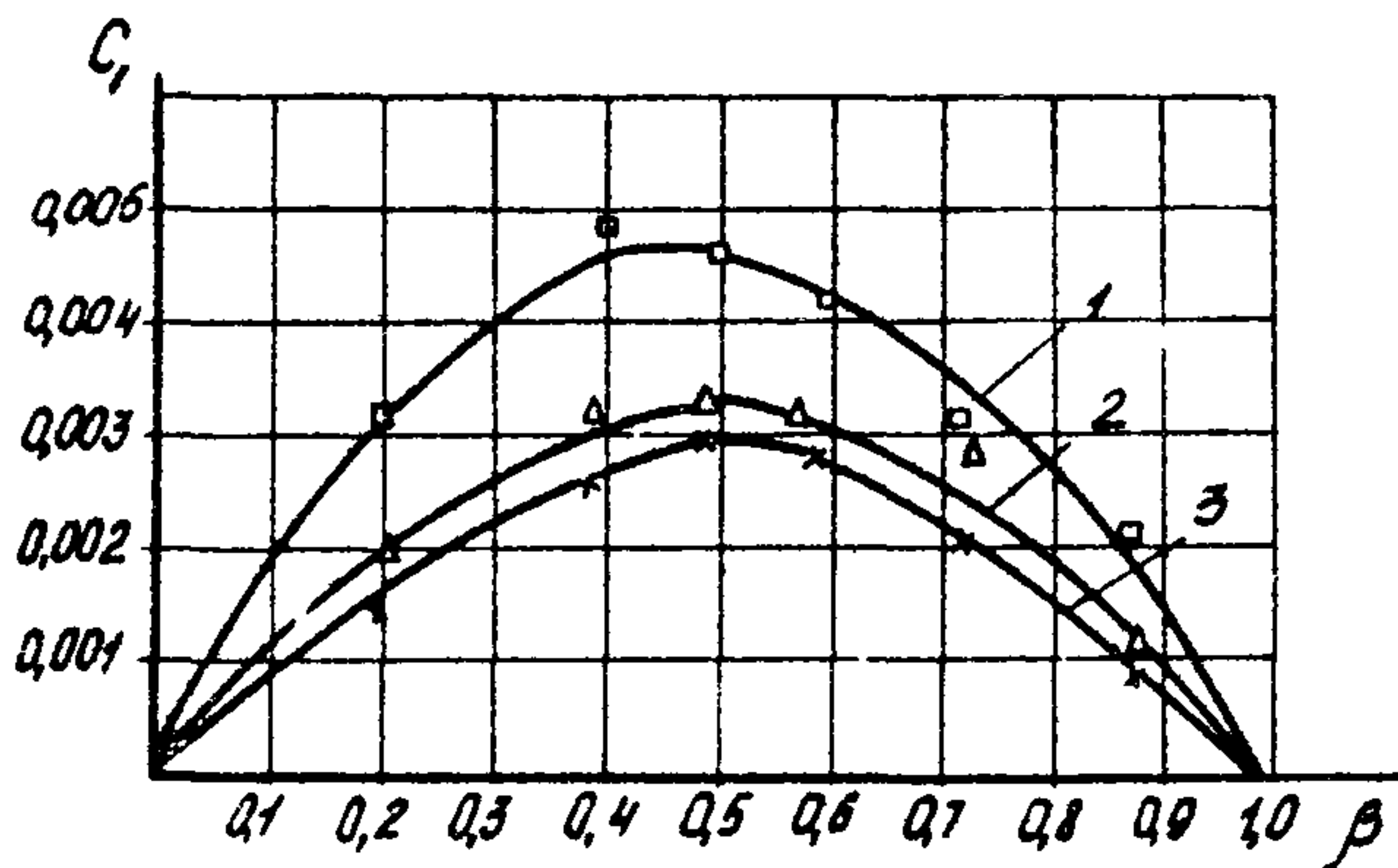
Рис. 5. Изменение коэффициента C_1 в зависимости от изменения \beta :
