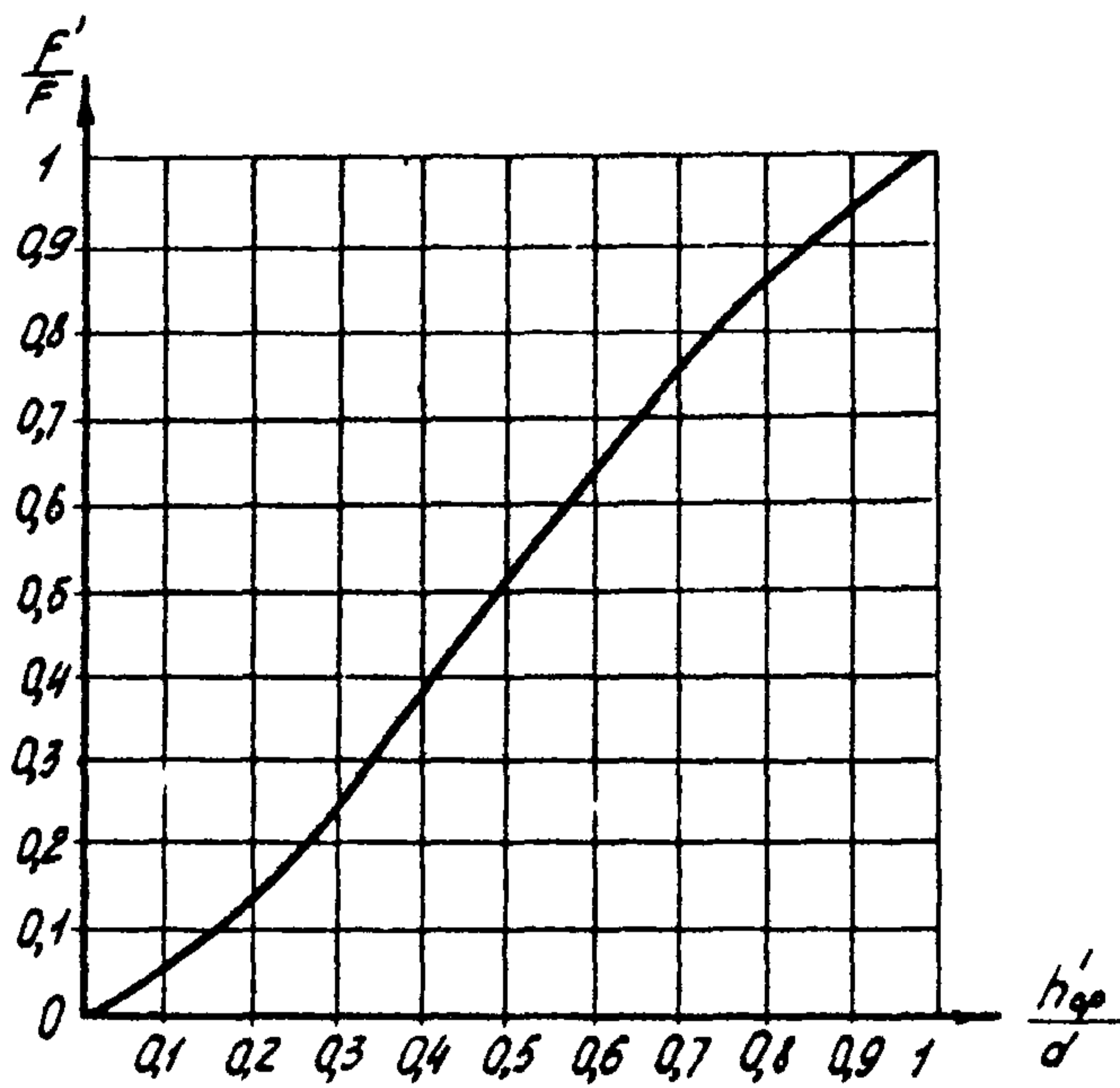
Рис. 6. Изменение \frac{F'}{F} = f\left(\frac{h'_{gp}}{d}\right)
