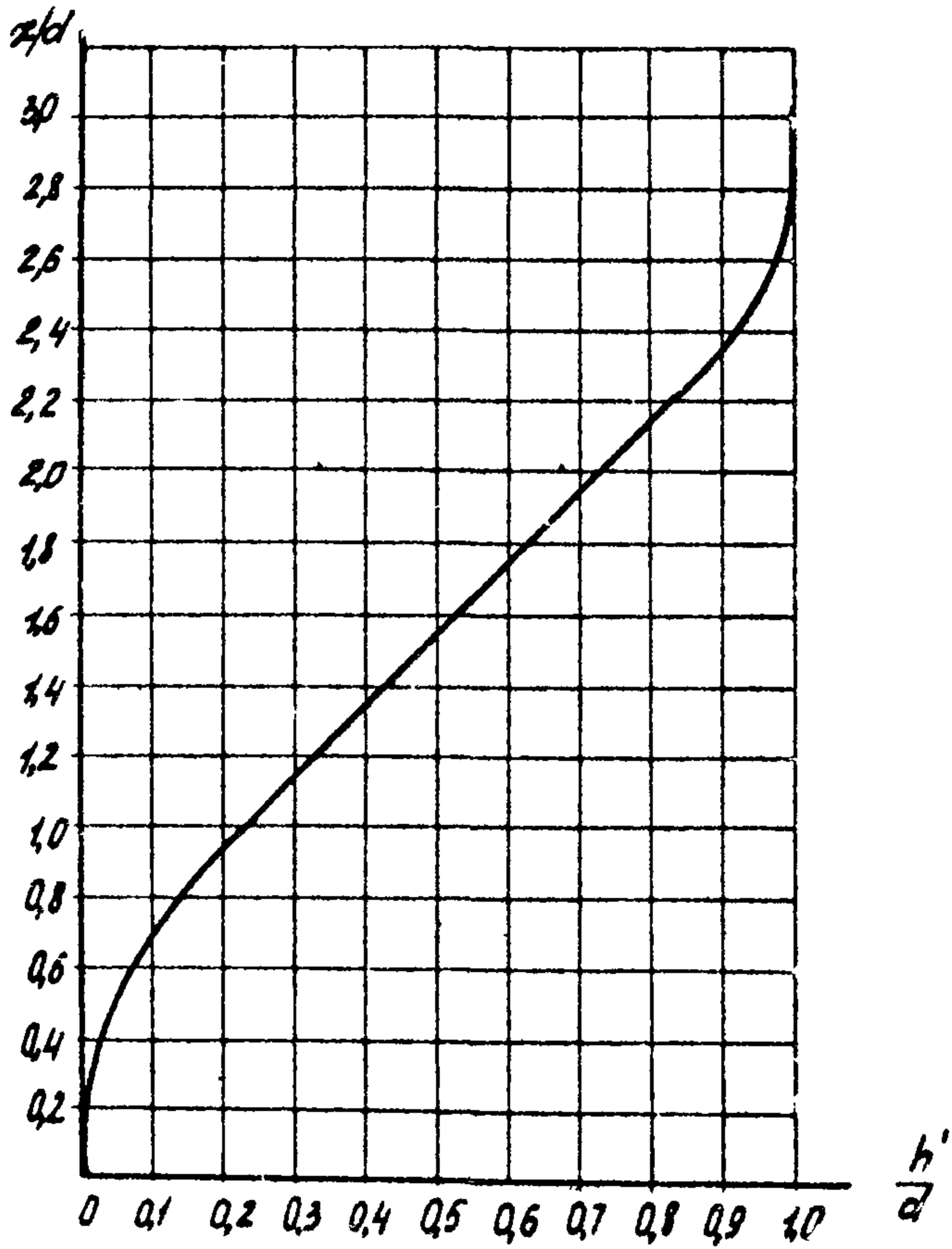
Рис. 7. Зависимость отношения \frac{z}{d} от изменения \frac{h'}{d}
