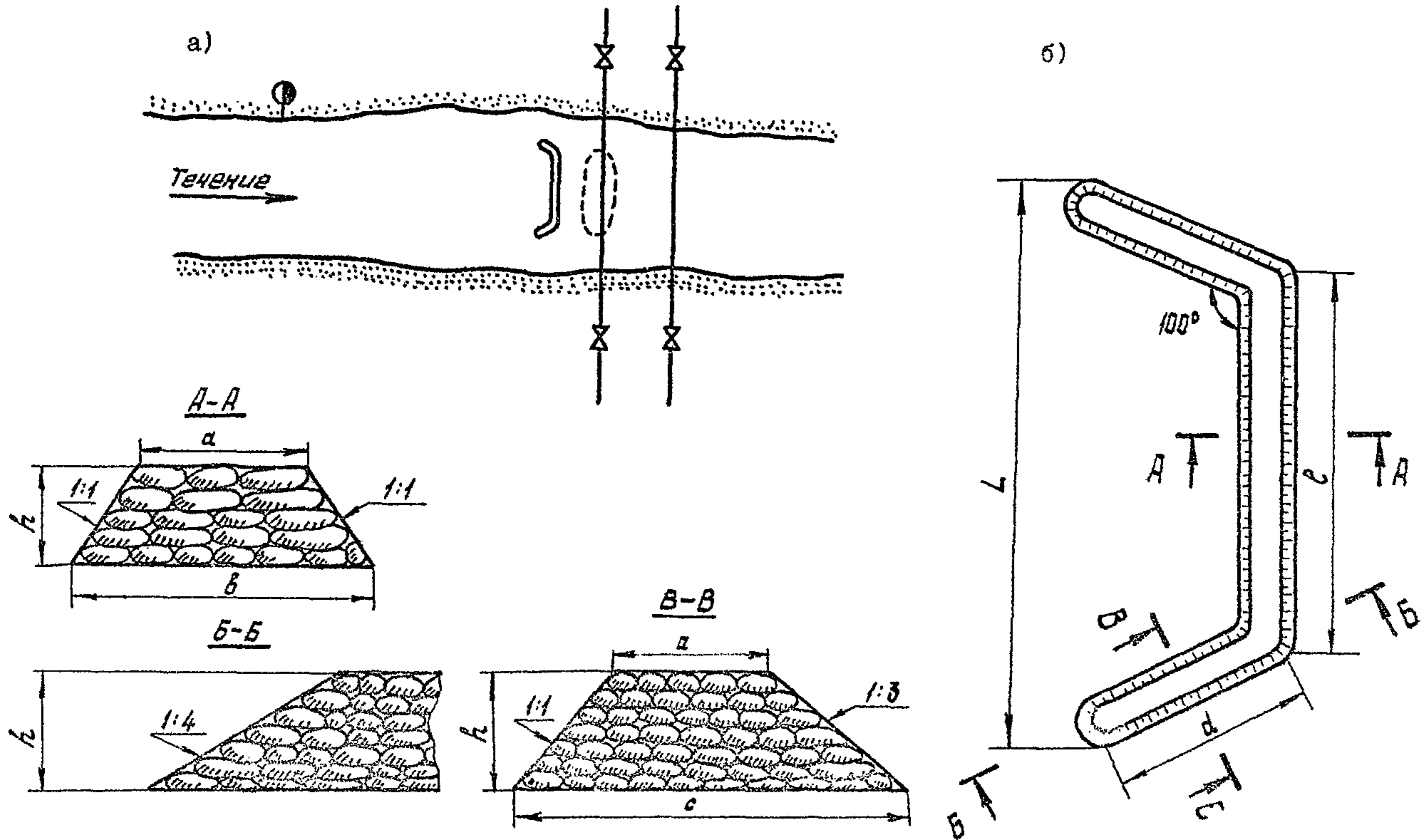
а) - положение в плане; б) - конструкция донного порога
