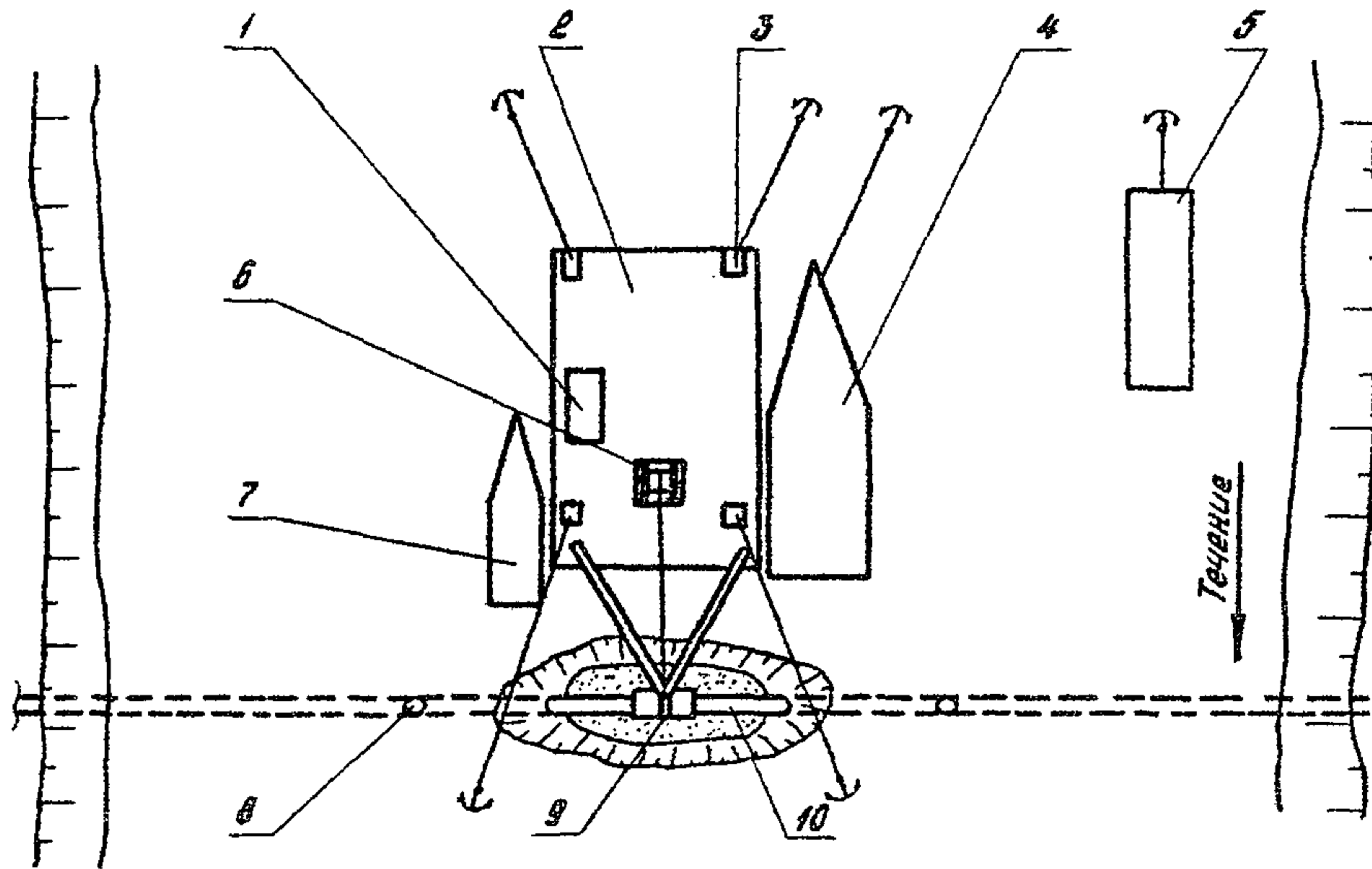
Схема расстановки машин и механизмов при ремонте ППМН с применением разъемных муфт
