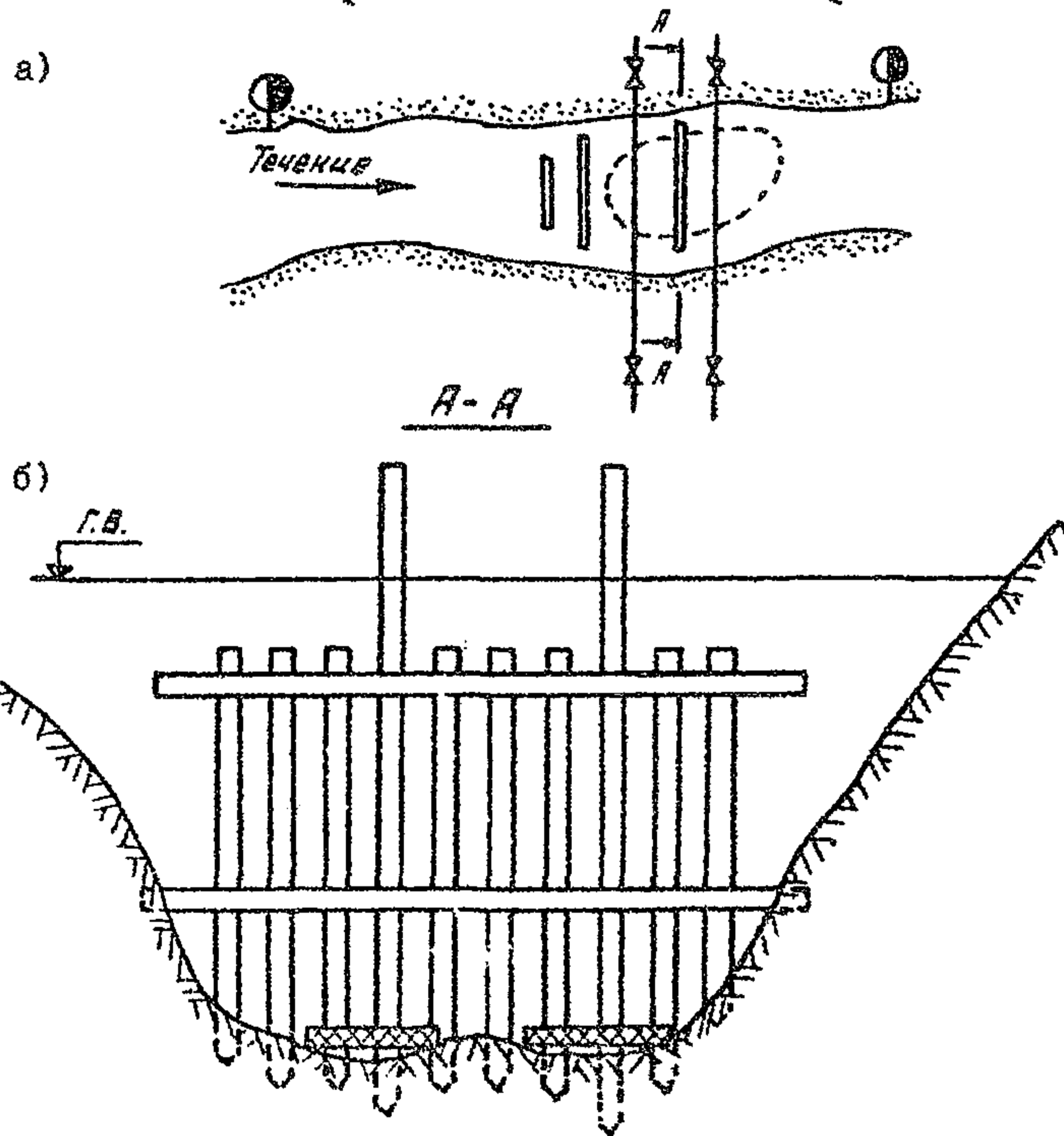
а) - расположение в плане; б) - конструкция сквозной шпору
