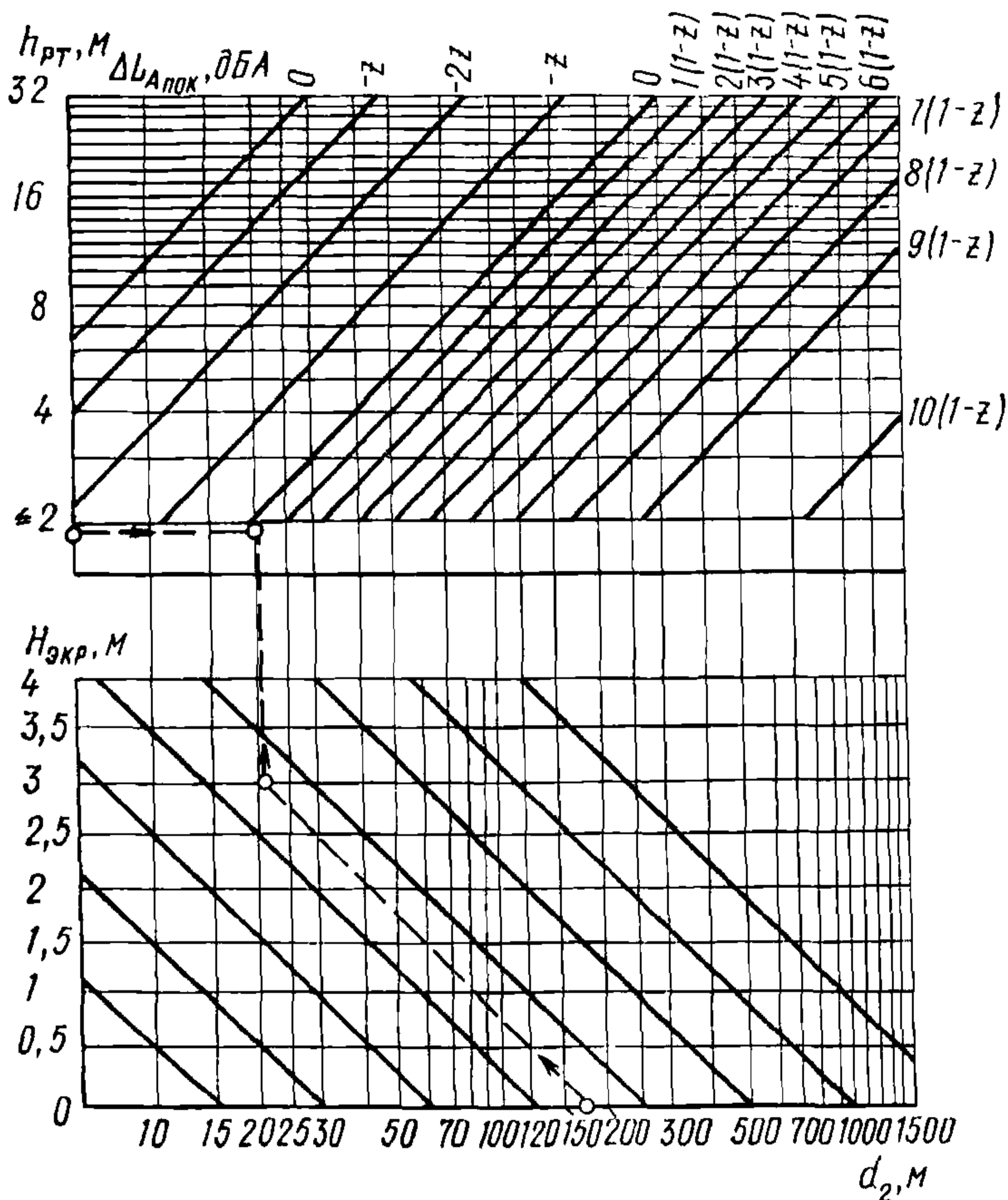
Рис. 9. Номограмма для определения снижения уровня звука вследствие его затухания над акустически мягким покрытием территории при распространении звуковых волн за экраном
