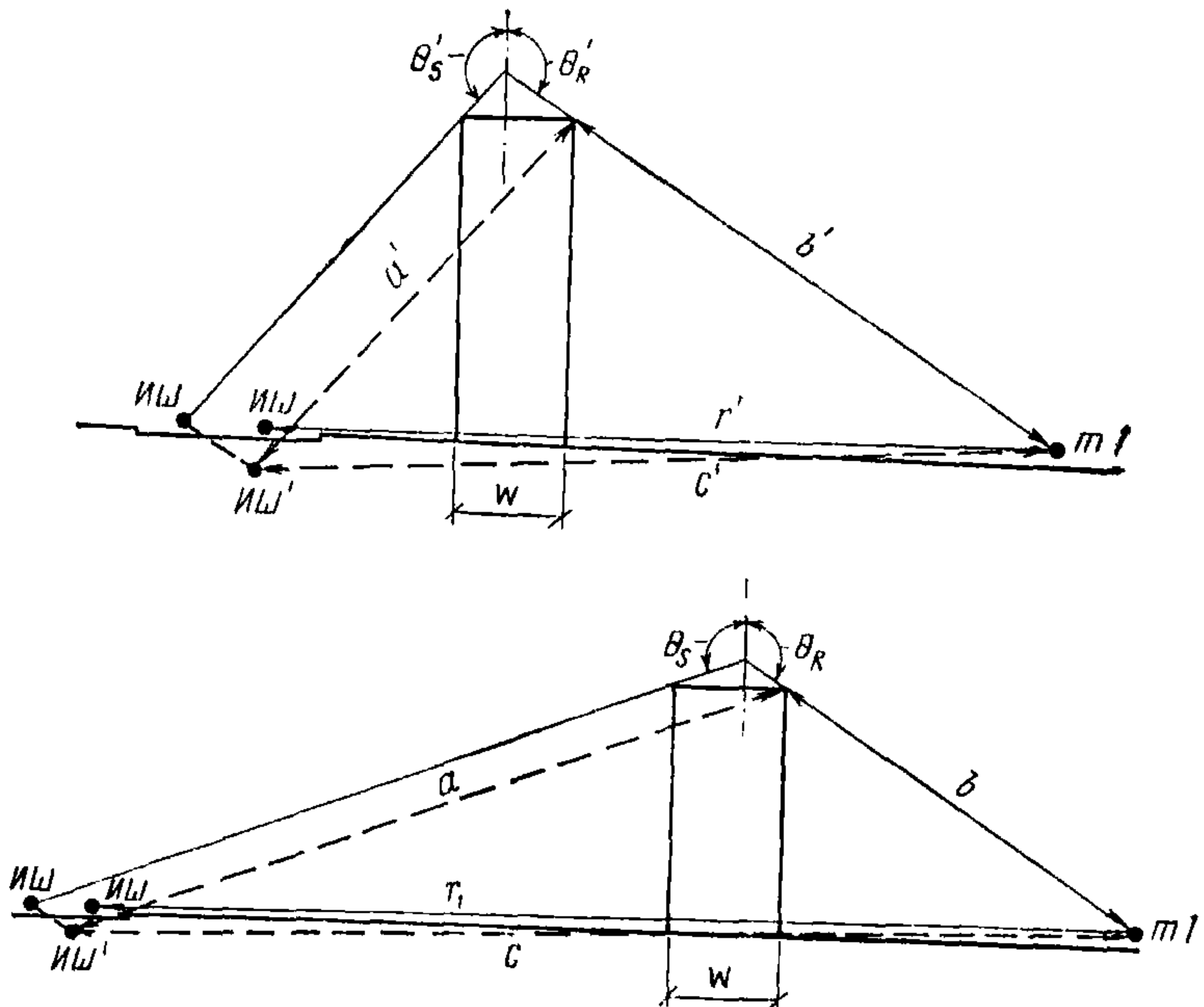
Рис. 15. Расчетные схемы для определения снижения уровня звука экранами-зданиями
