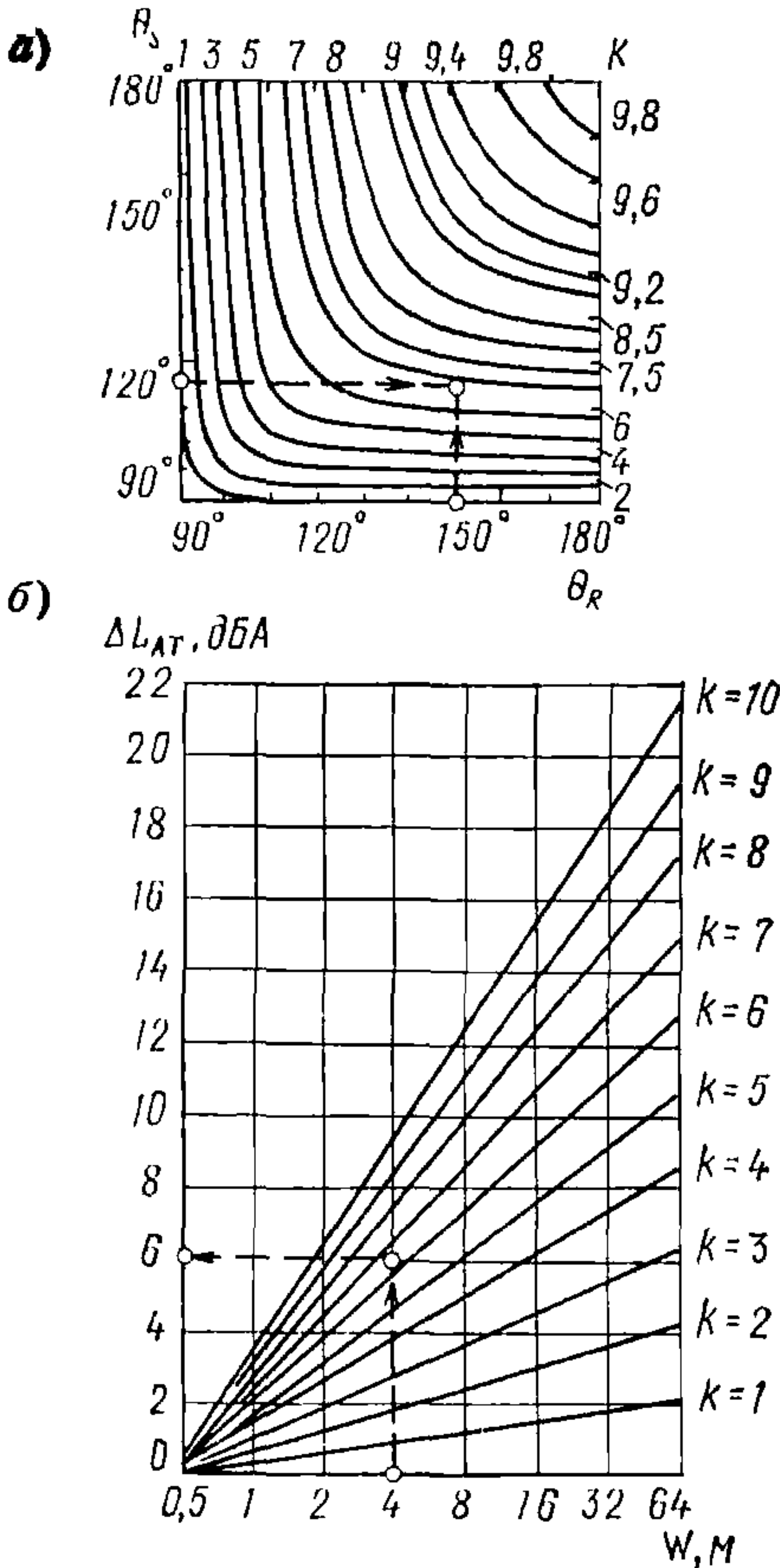
Рис. 8. Номограммы для определения дополнительного снижения уровня звука экраном большой толщины
