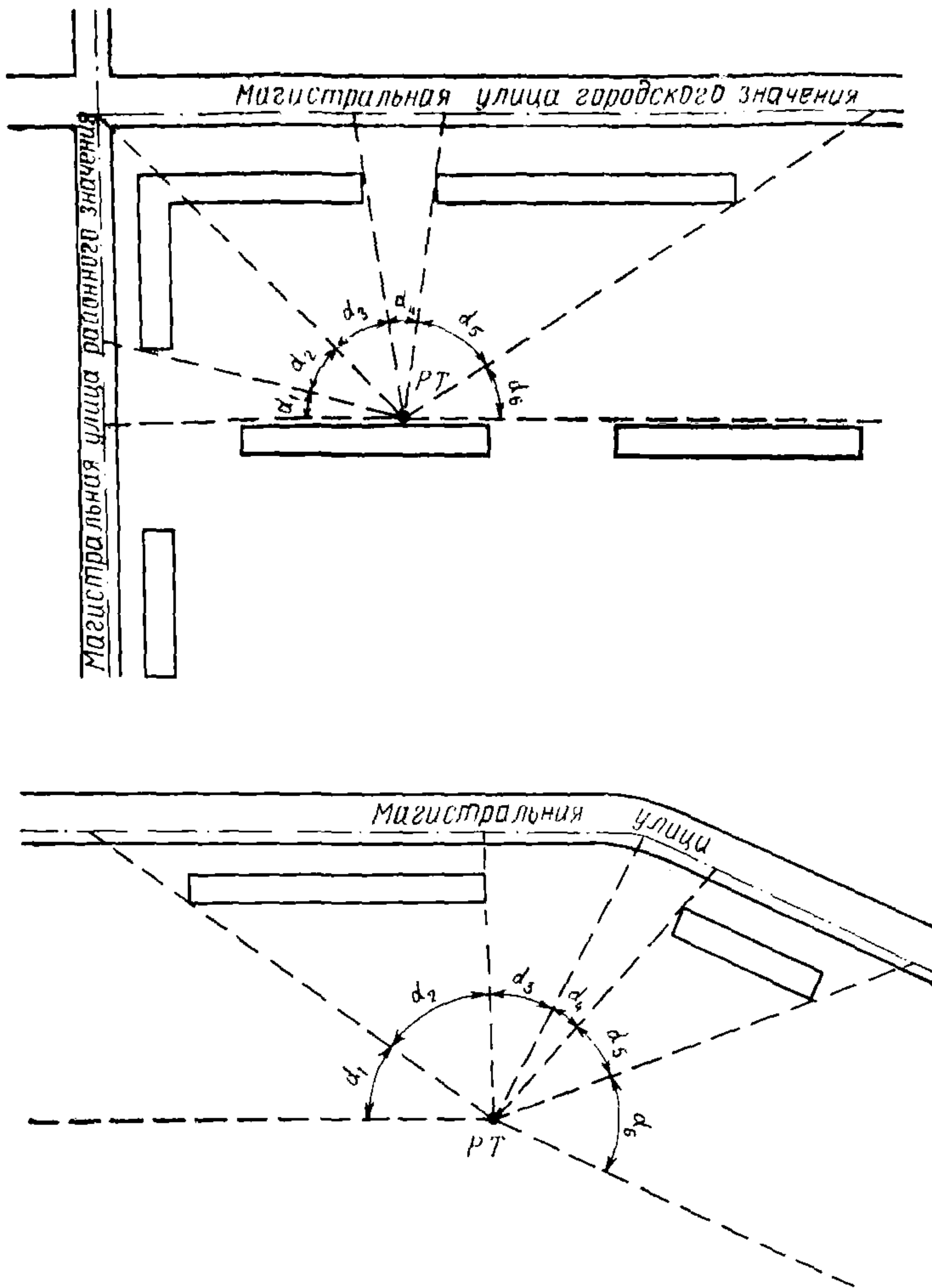
Рис. 1. Примеры разбивки примагистральной территории застройки на участки, отличающиеся по условиям распространения шума
