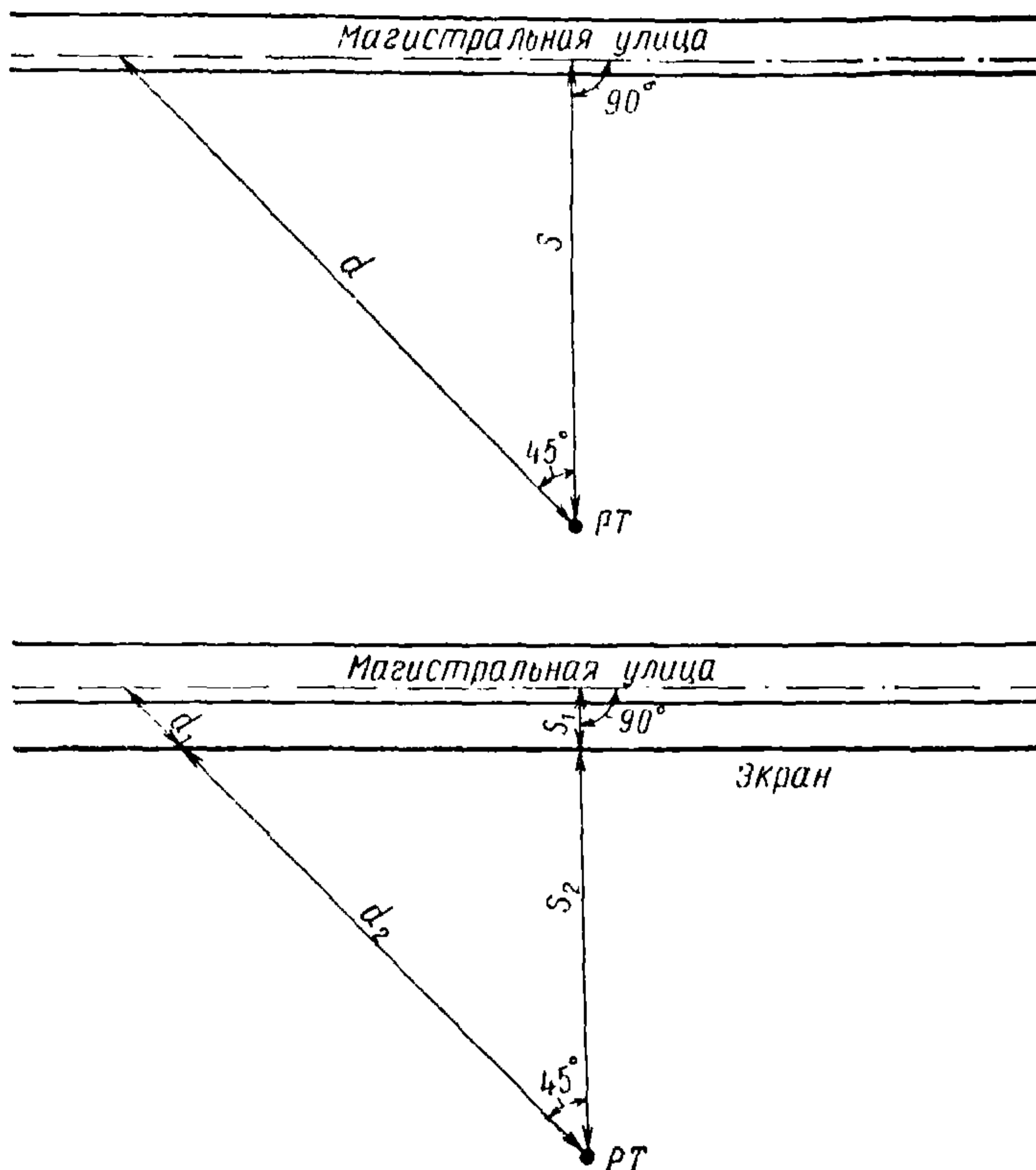
Рис. 5. Схемы для определения расчетных расстояний
