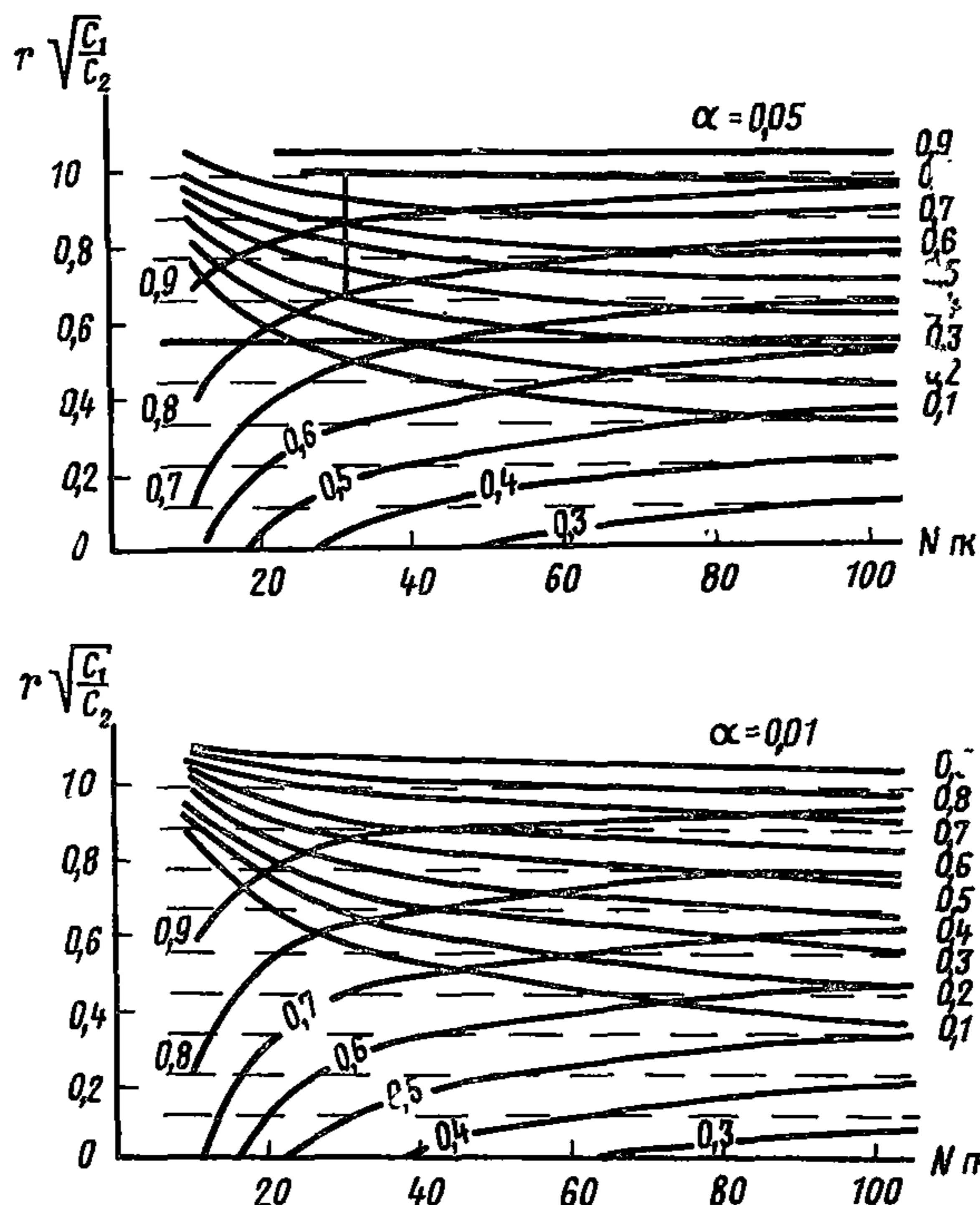
Рис. 1. Номограммы для выбора метода по критерию |r| \geq \sqrt{\frac{c_1}{c_2}} при 10 \leq N_{ПК} \leq 100 при уровнях значимости 0,05 и 0,01
