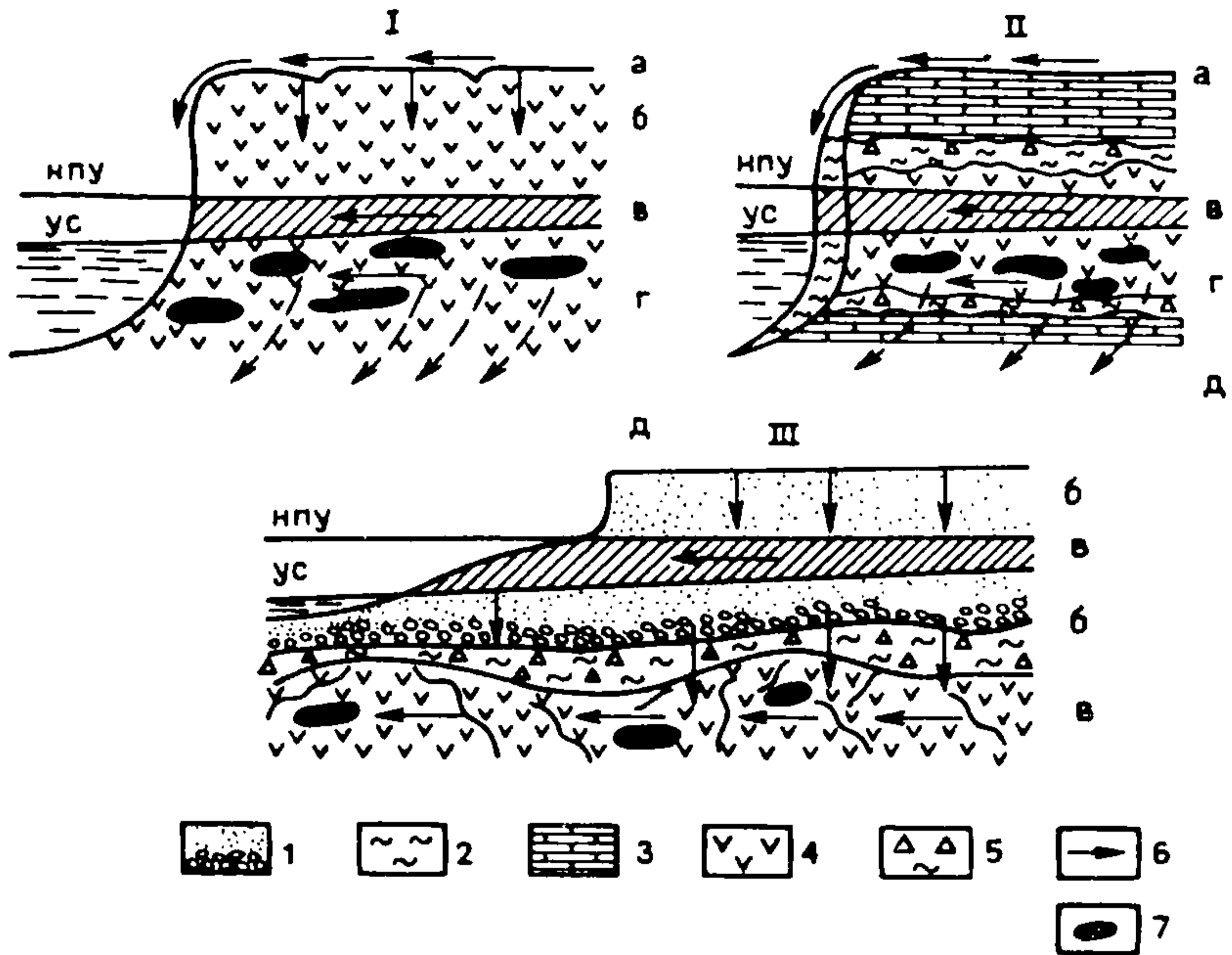
Рис. 5. Основные типы закарстованных берегов водохранилищ (по И.А.Печеркину)
