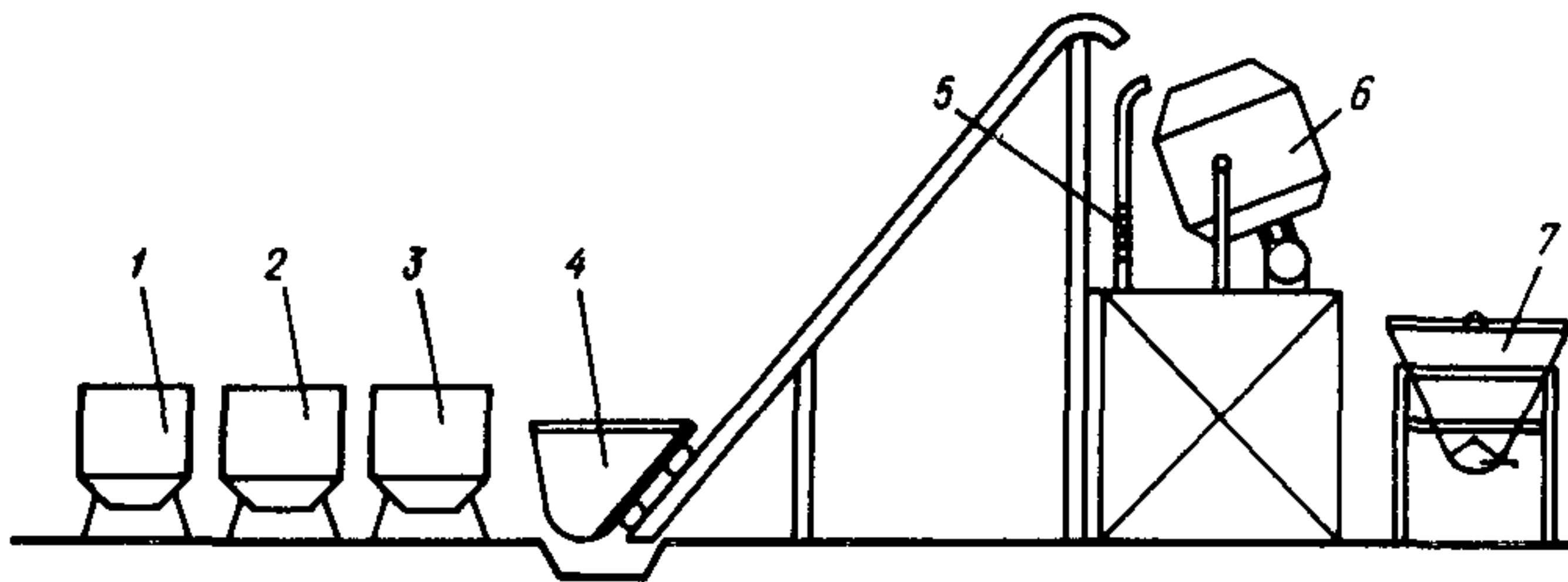
Рис.2. Пост приготовления декоративной бетонной смеси
