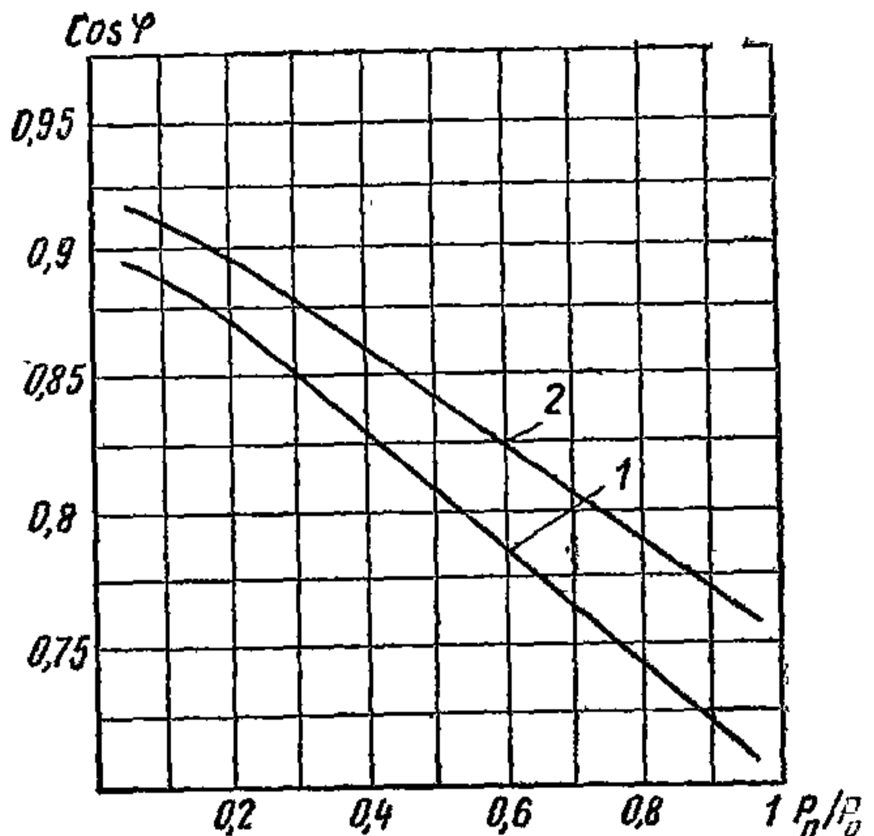
Рис. 1. Зависимость \cos \varphi от отношения \frac{P_{\text{п}}}{P_0} в максимуме нагрузок
