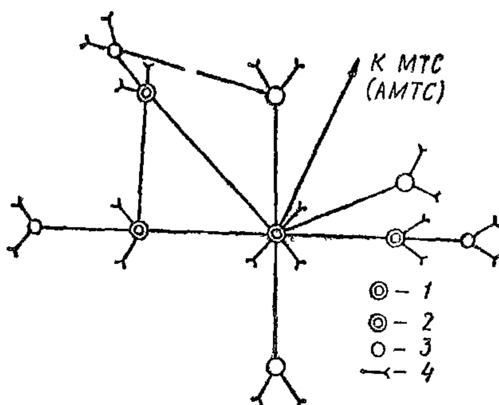
Рис. 3. Схема построения СТС
