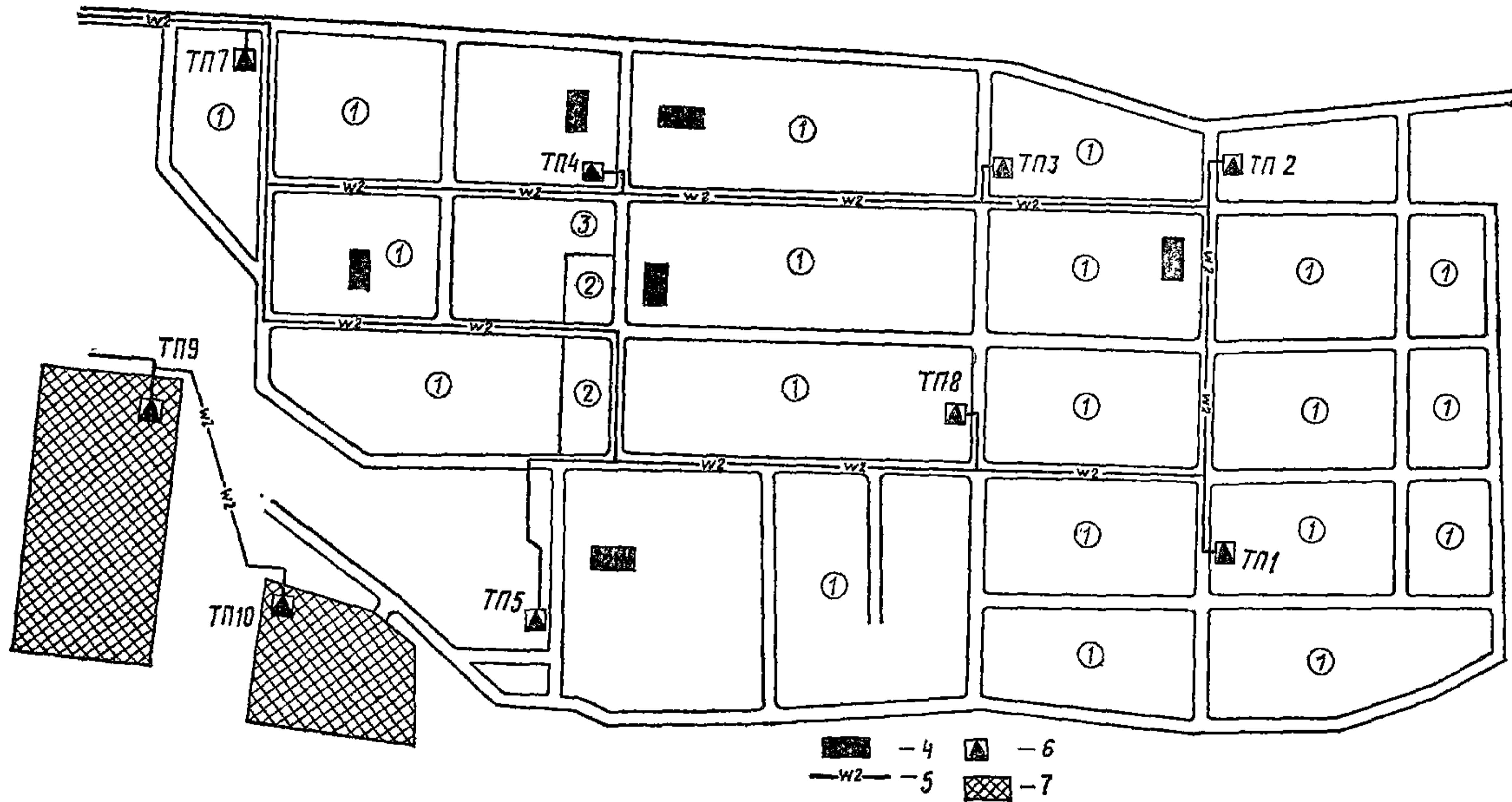
Рис. 6. План сети напряжением 10 кВ
