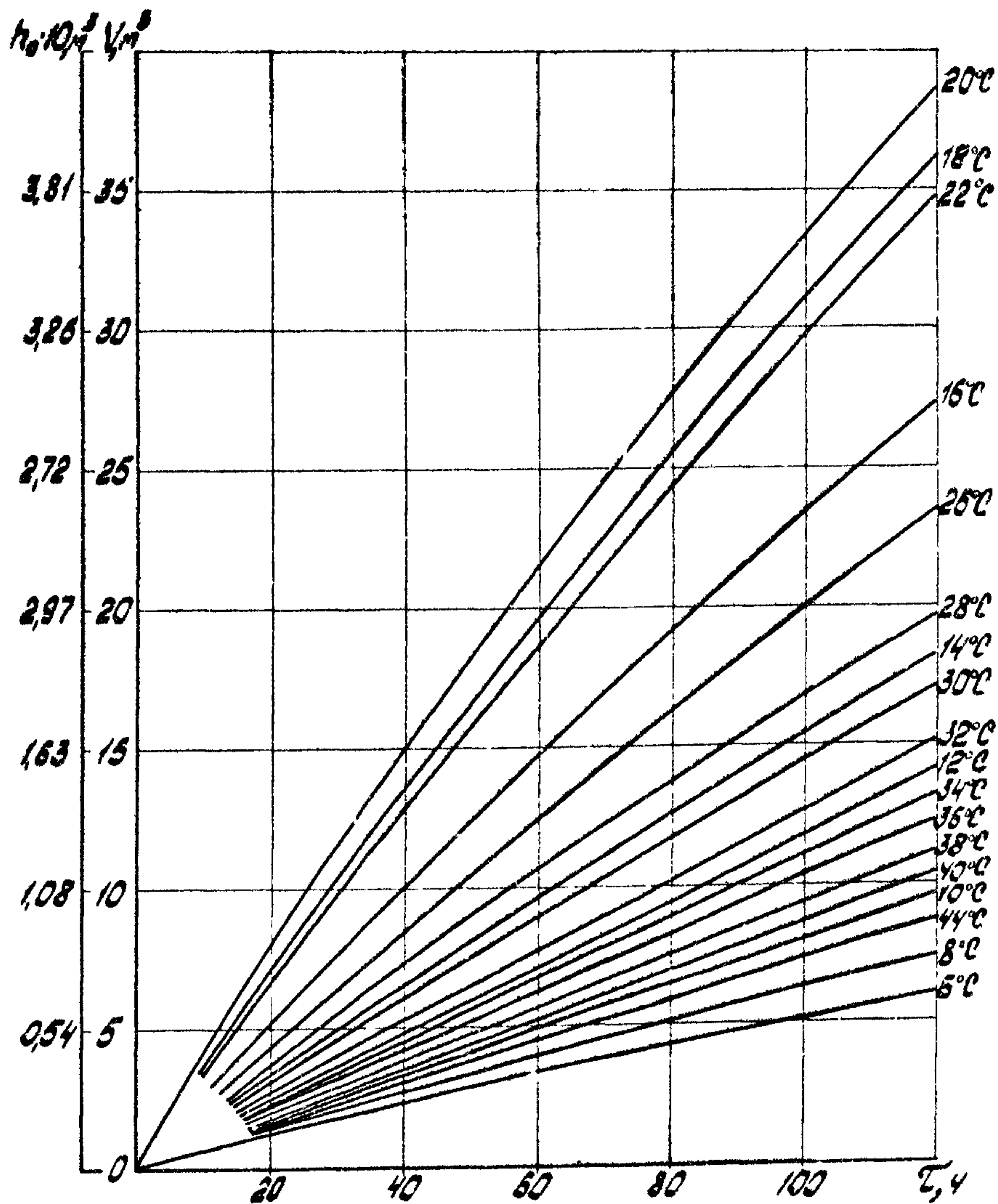
Рис. 24. Количество донного смоло-парафинового осадка, образующегося в резервуаре РВС-10000 в течение одного цикла заполнения-опорожнения его в зависимости от времени и температура хранения кулешовской нефти
