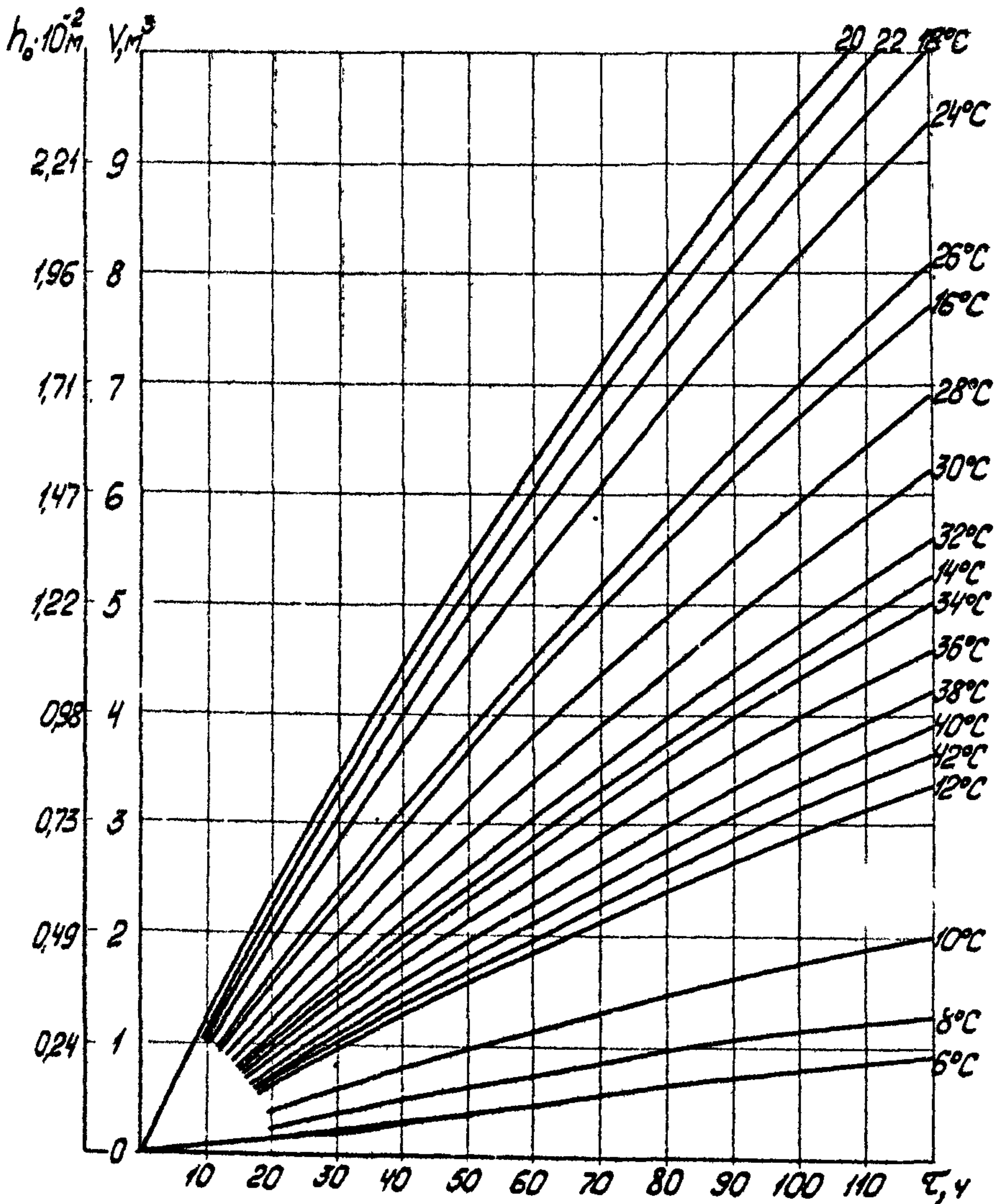
Рис. II. Количество донного смоло-парафинового осадка, образующегося в резервуаре РВС-5000 в течение одного цикла заполнения-опорожнения его в зависимости от времени и температуры хранения роштинской нефти
