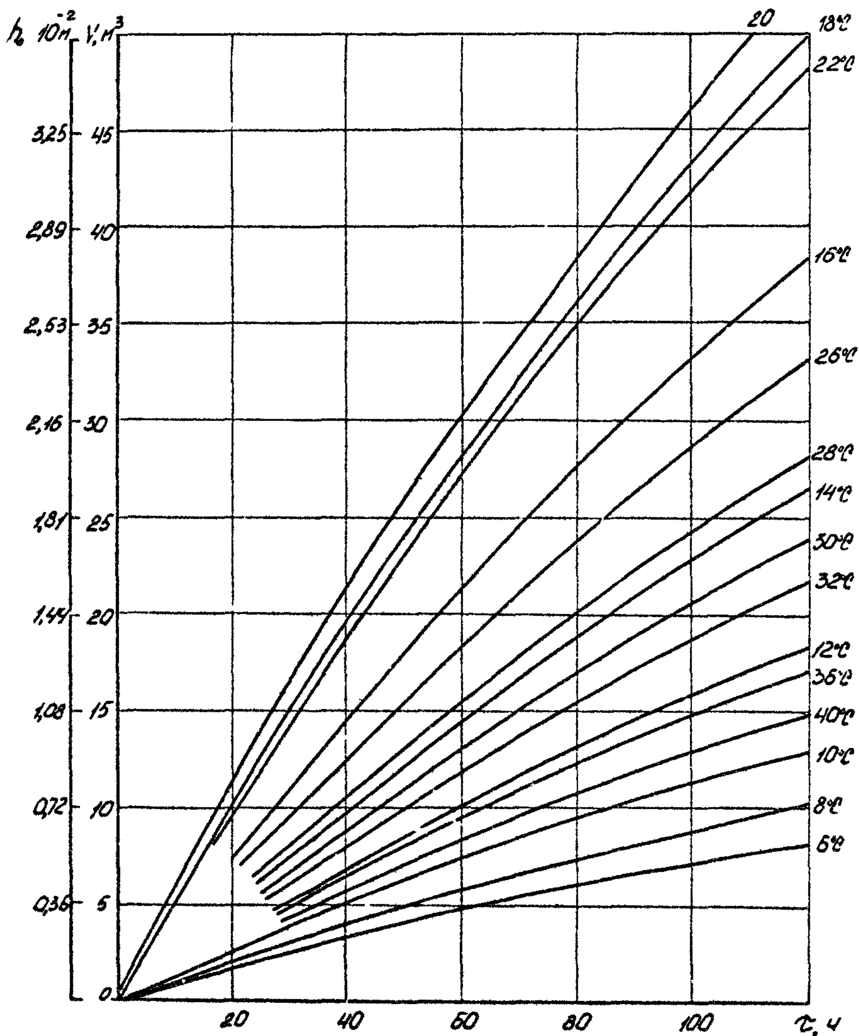
Рис.27. Количество донного смоло-парафинового осадка, образующегося в резервуаре ЖР-10000 в течение одного цикла заполнения-опорожнения его в зависимости от времени и температуры хранения кудловской нефти
