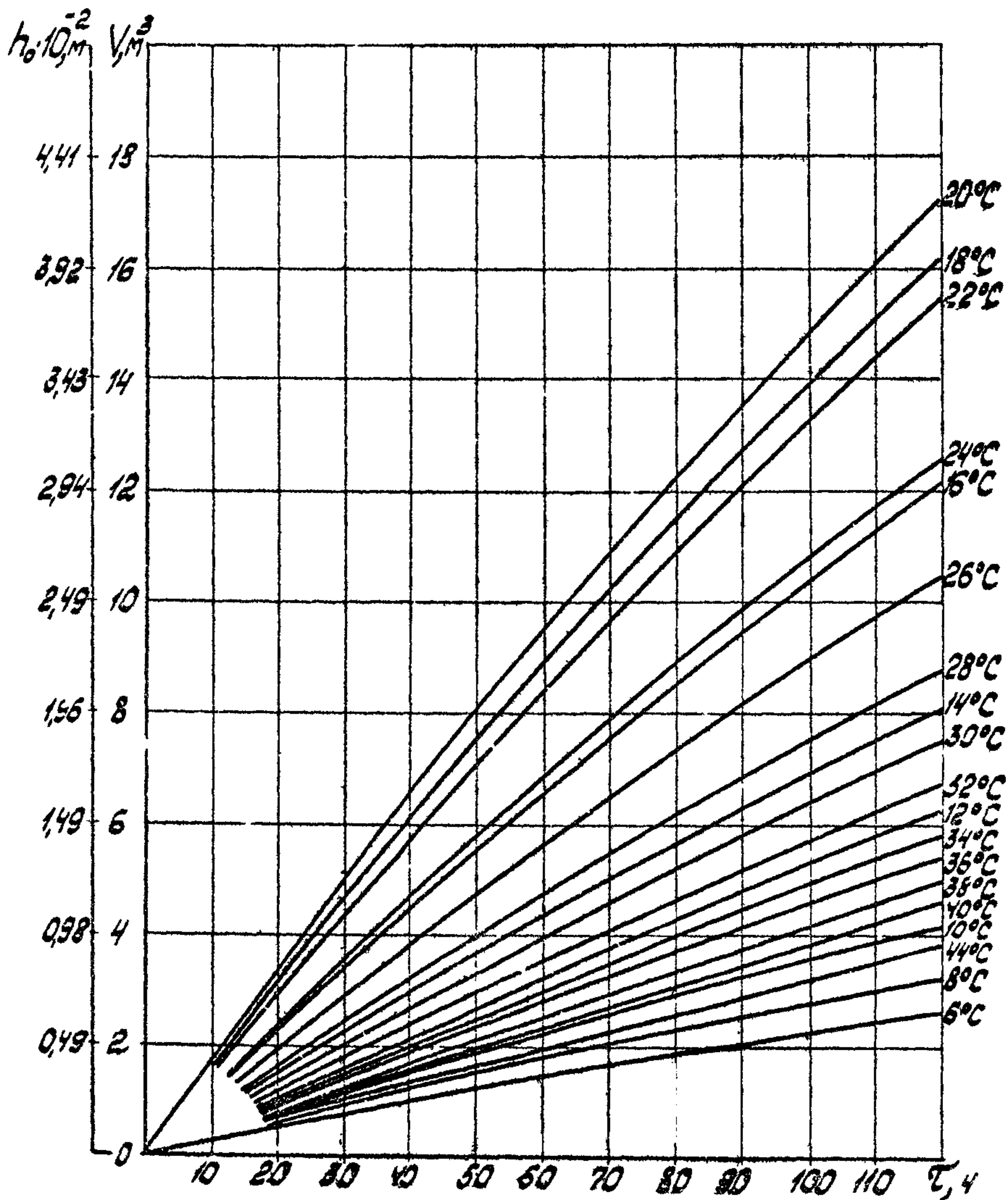
Рис. 23. Количество данного смоло-парафинового осадка, образующегося в резервуаре РВС-5000 в течение одного цикла заполнения-опорожнения его в зависимости от времени и температуры хранения кулешовской нефти
