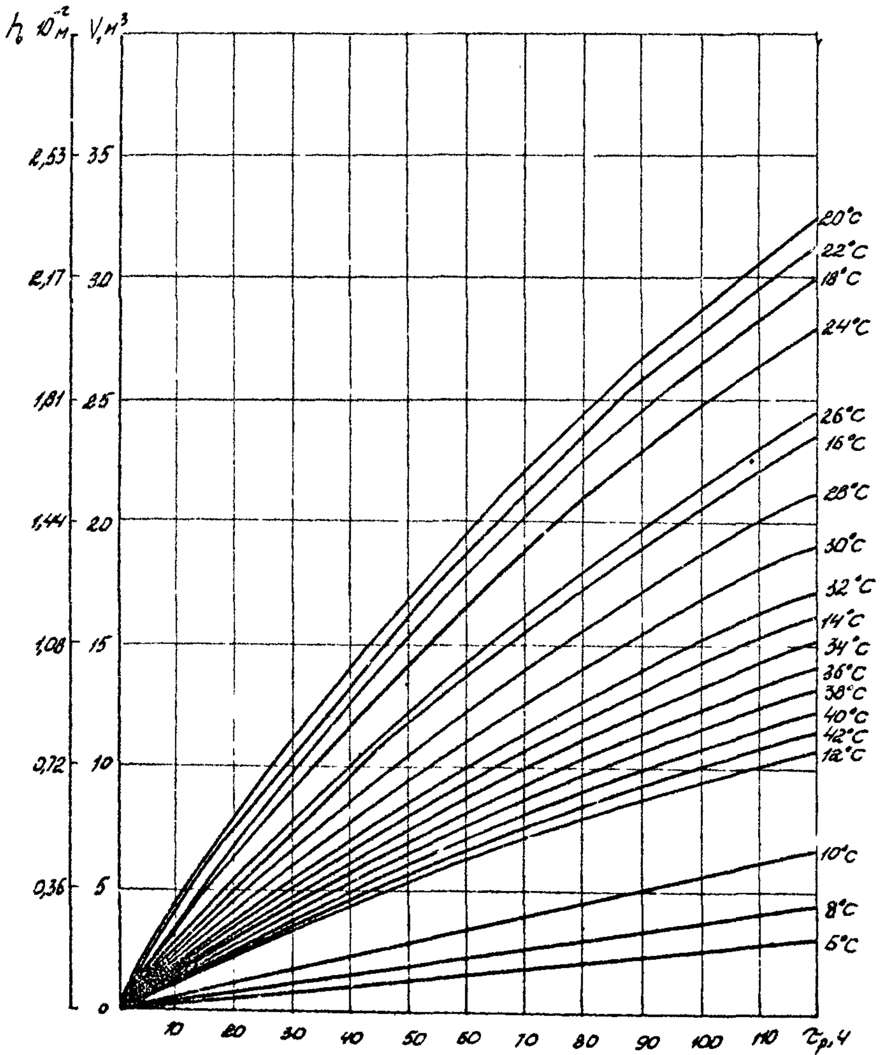
Рис. 15. Количество донного смоло-парафинового осадка, образующегося в резервуаре МБР-10000 в течение одного цикла заполнения-опорожнения его в зависимости от времени и температуры хранения ромашкинской нефти
