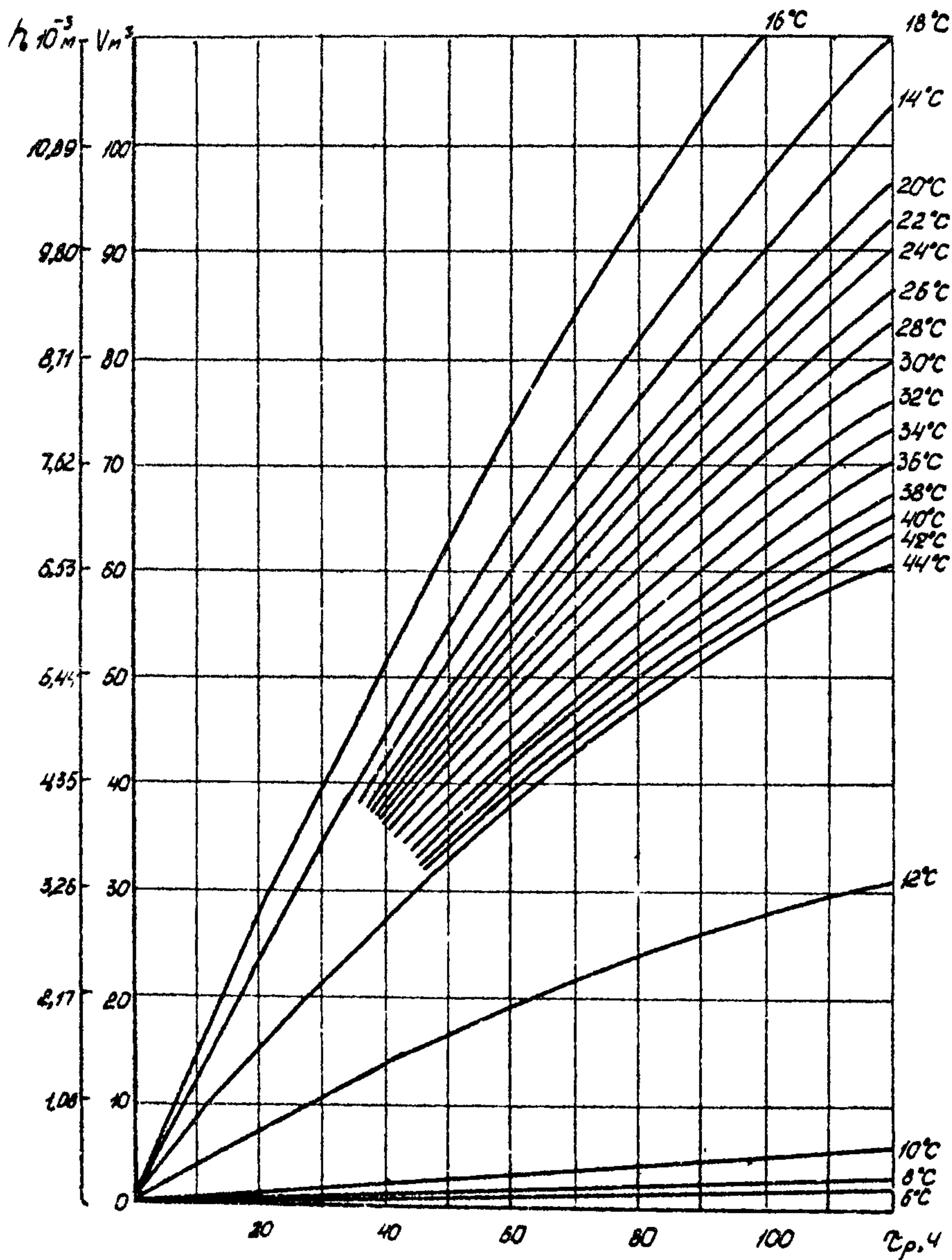
Рис. 18. Количество донного смоло-парафинового осадка, образующегося в резервуаре РВС-10000 в течение одного цикла заполнения-опорожнения его в зависимости от времени и температуры хранения кукуновской нефти
