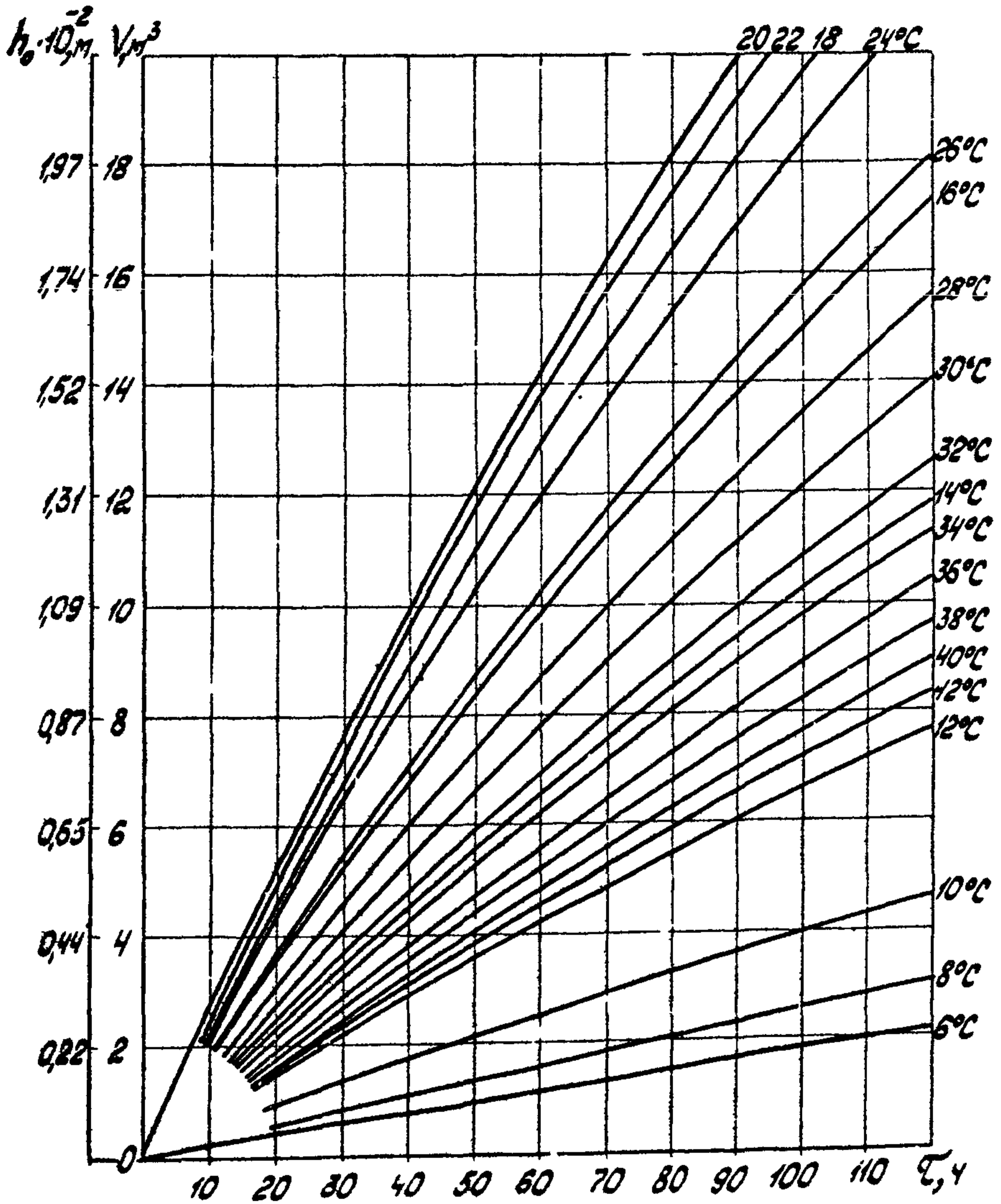
Рис. 12. Количество донного смоло-парафинового осадка, образующегося в резервуаре РВС-10000 в течение одного цикла заполнения-олорожнения его в зависимости от времени и температуры хранения ромашкинской нефти
