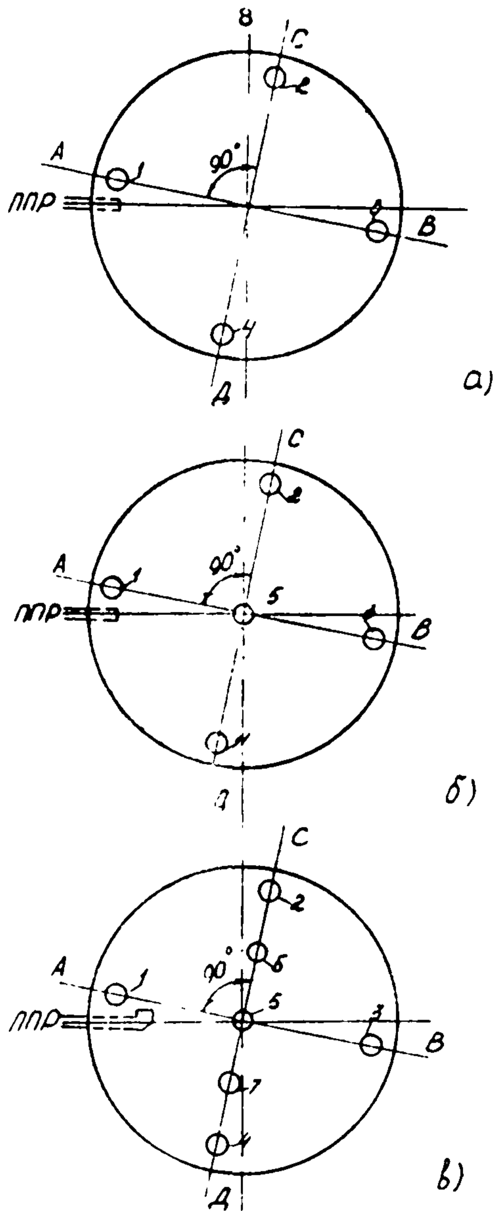
Рис. 2. Принципиальные схемы размещения люков для замера донных парафинистых отложений на перекрытии нефтяных резервуаров:
