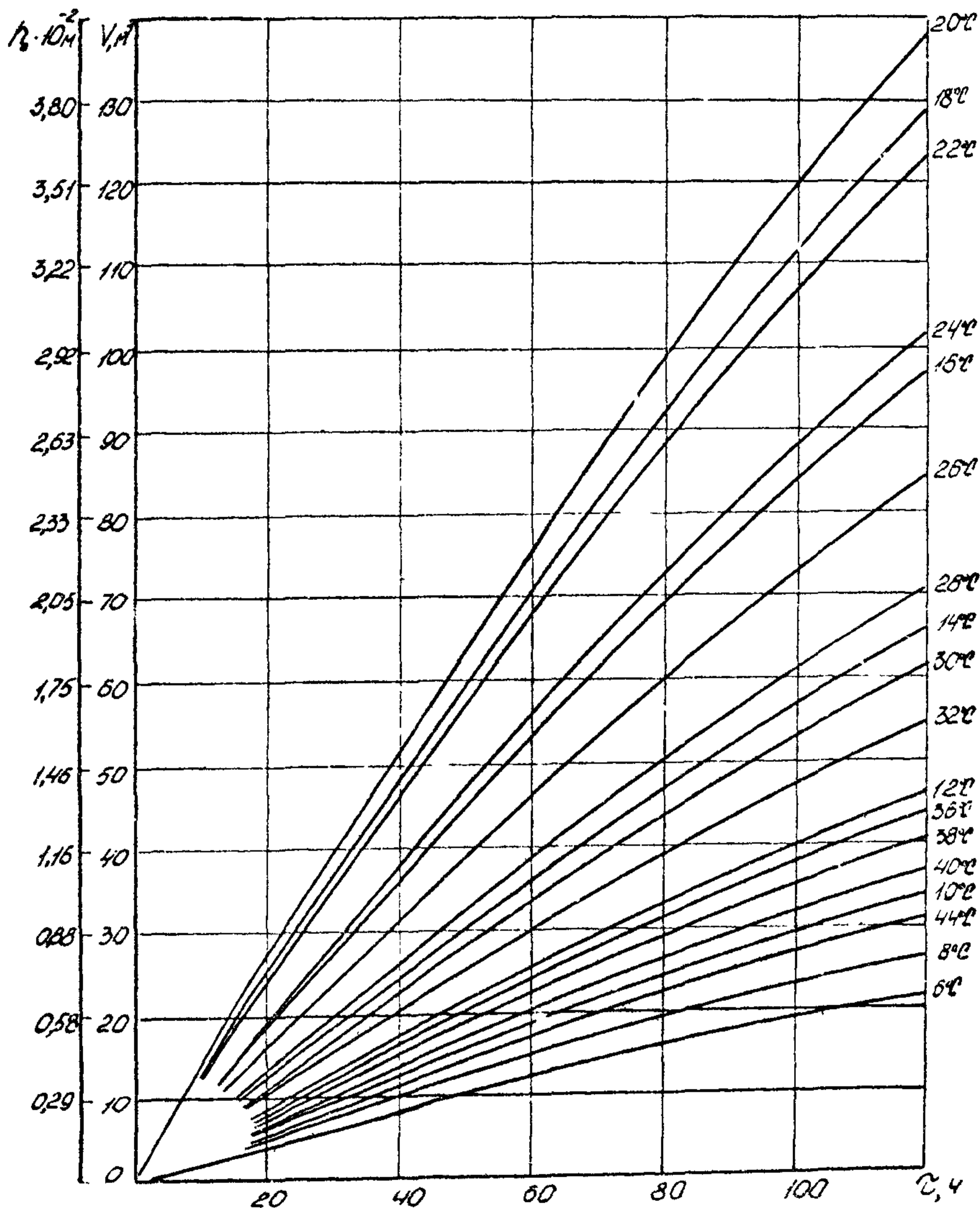
Рис.28. Количество донного смоло-парафинового осадка, образующегося в резервуаре КБР-30000 в течение одного цикла заполнения-опорожнения его в зависимости от времени и температуры хранения кузнецовской нефти
