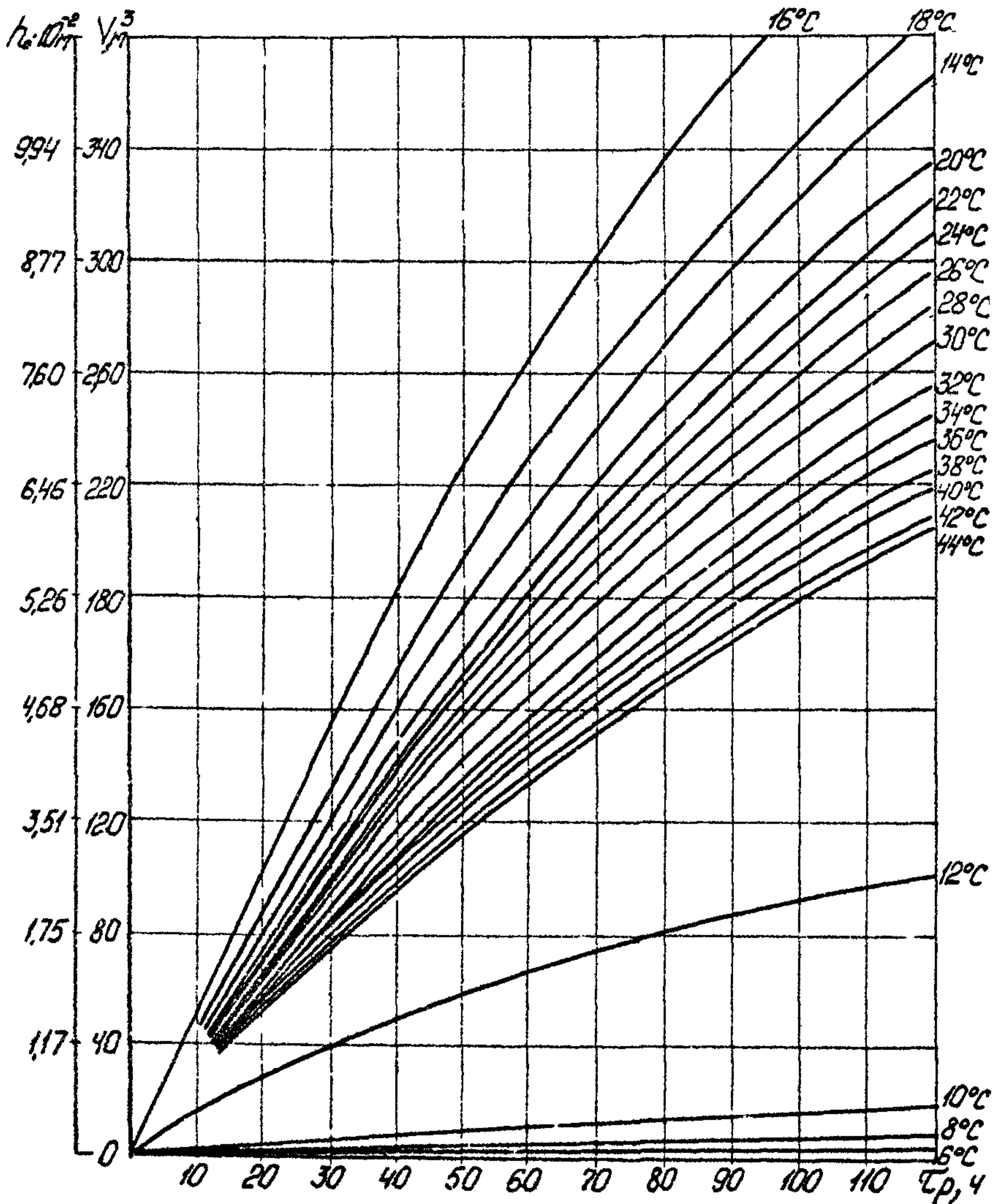
Рис. 22. Количество донного смоло-парафинового осадка, образующегося в резервуаре МБР-30000 в течение одного цикла заполнения-опорожнения его в зависимости от времени и температуры хранения мухановской нефти
