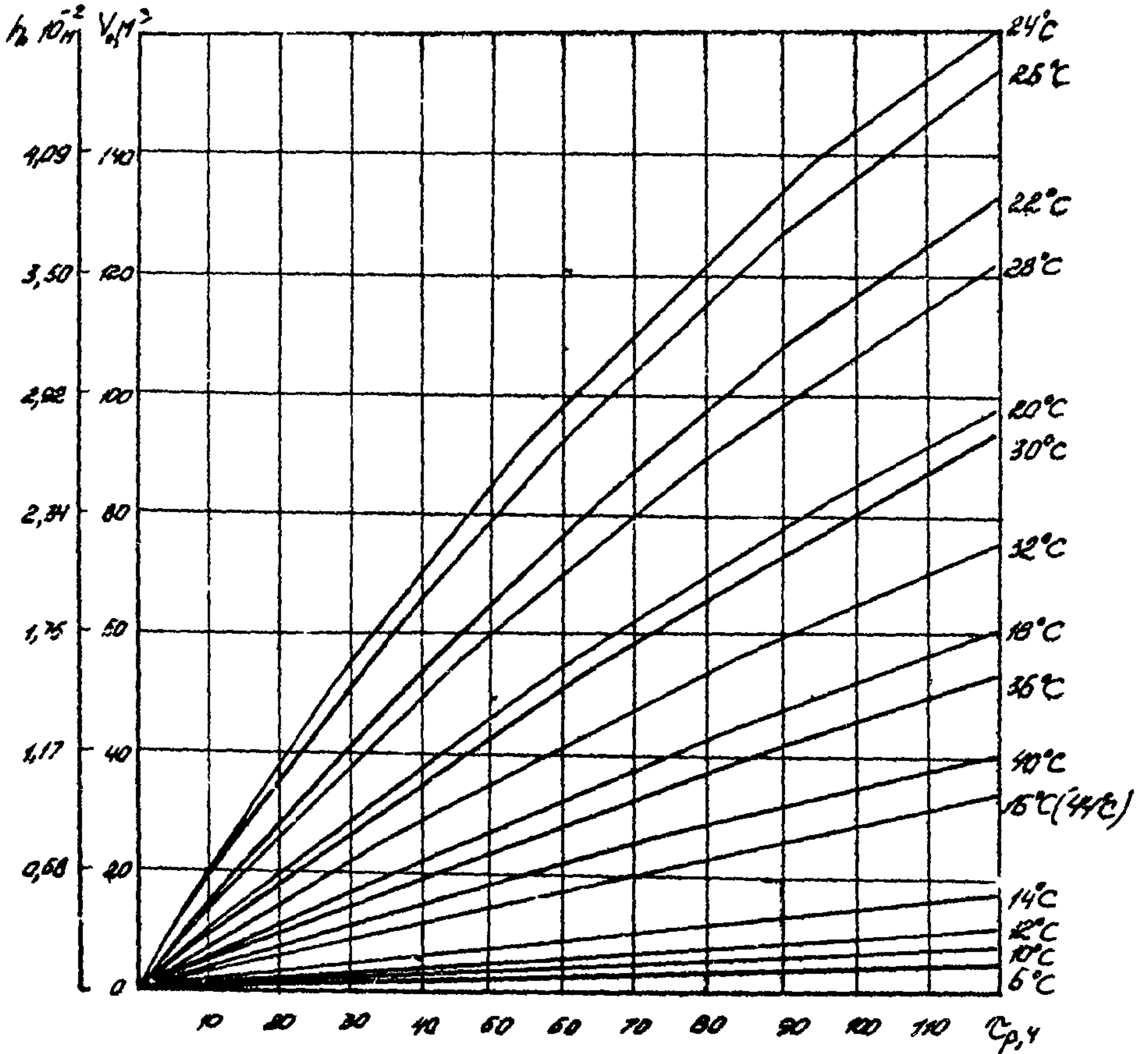
Рис. 10. Количество доплого смоло-парафинового осадка, образующегося в резервуаре ЖБР-30000 в течение одного цикла заполнения-опорожнения его в зависимости от времени и температуры хранения тменской нефти
