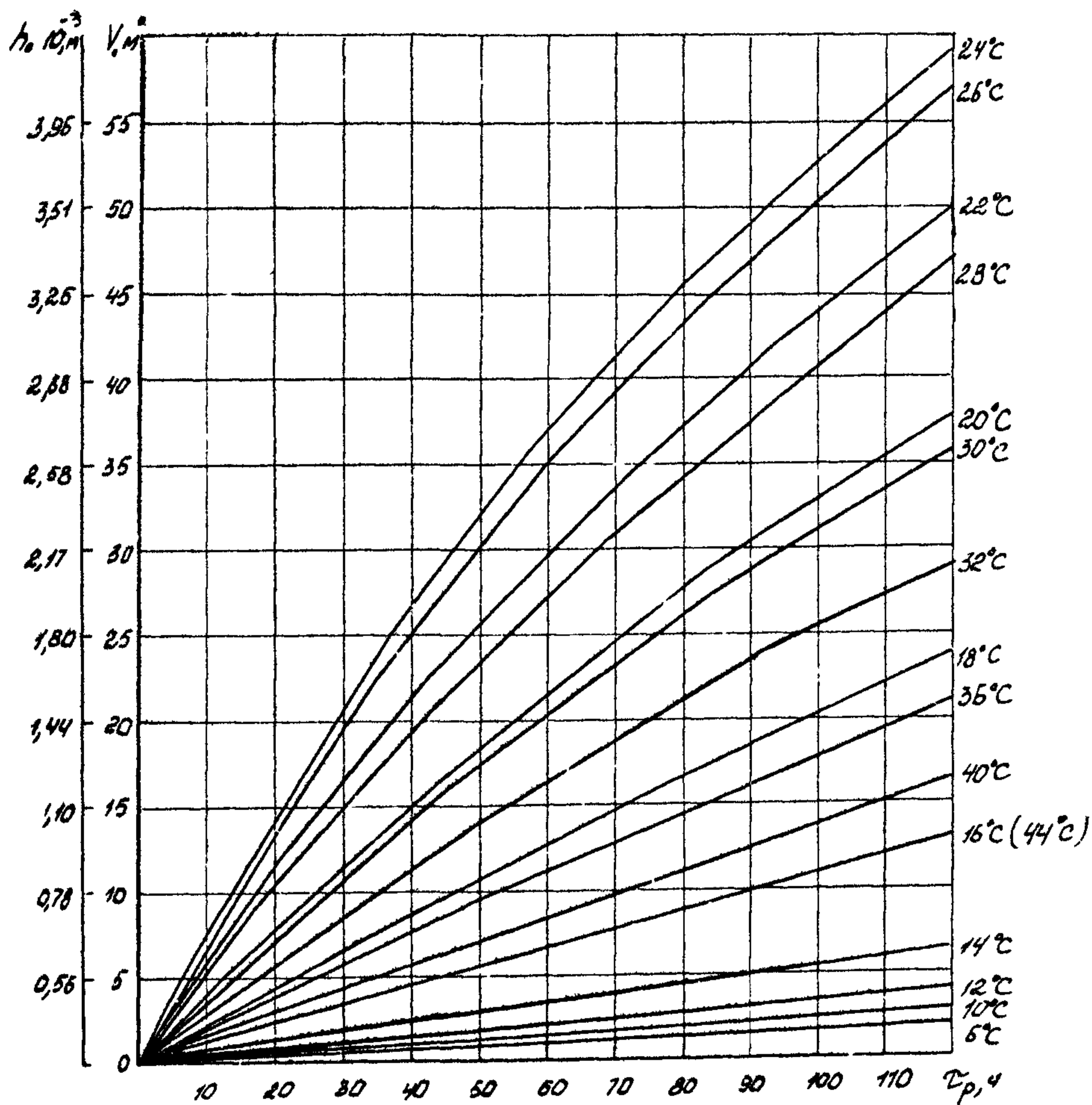
Рис. 9. Количество донного смоло-парафинового осадка, образующегося в резервуаре ЖБР-10000 в течение одного цикла заполнения-опорожнения его в зависимости от времени и температуры хранения томенской нефти
