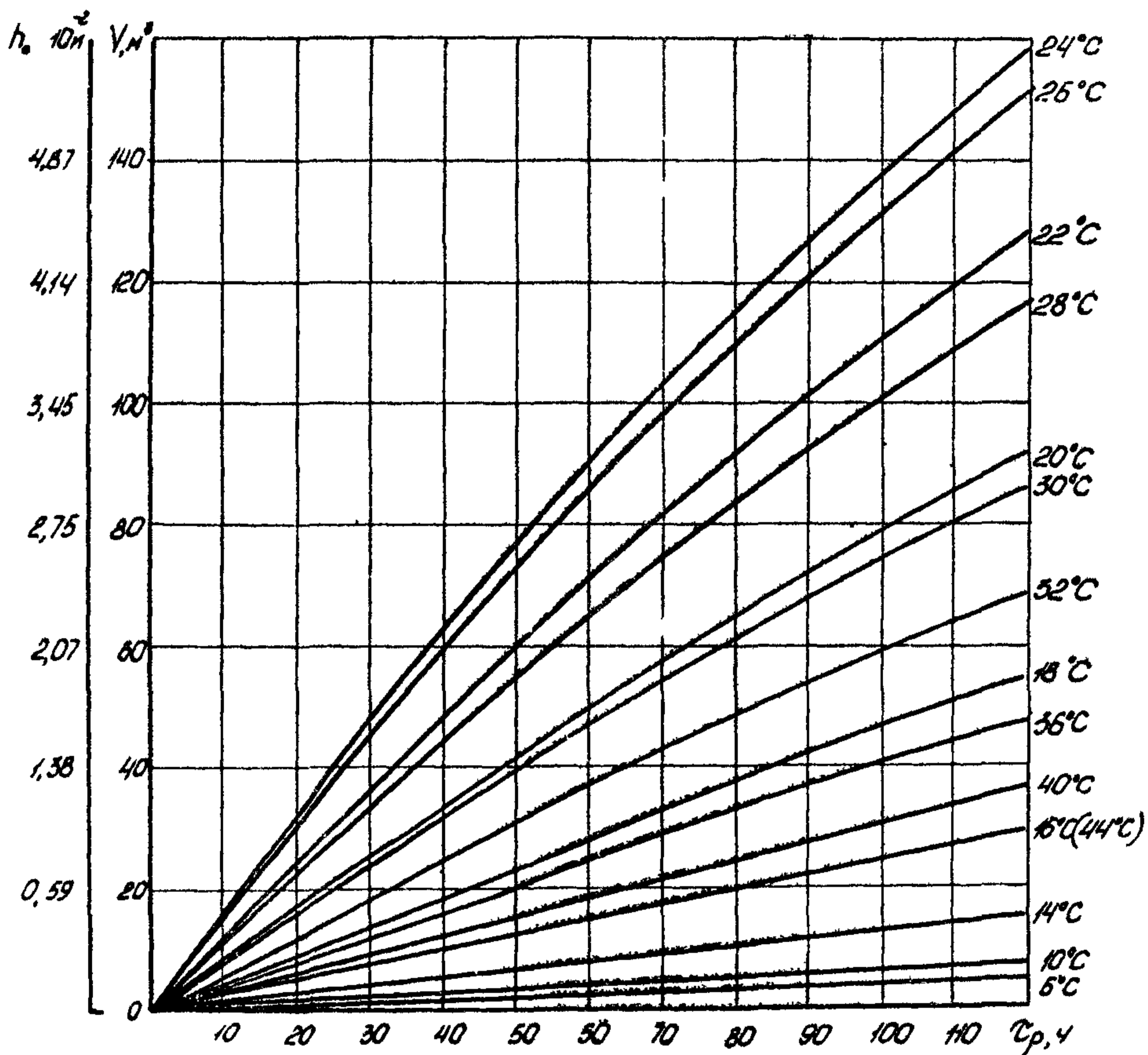
Рис. 8. Количество донного смоло-парафинового осадка, образующегося в резервуаре РВС-50000 в течение одного цикла заполнения-опорожнения его в зависимости от времени и температуры хранения тюменской нефти
