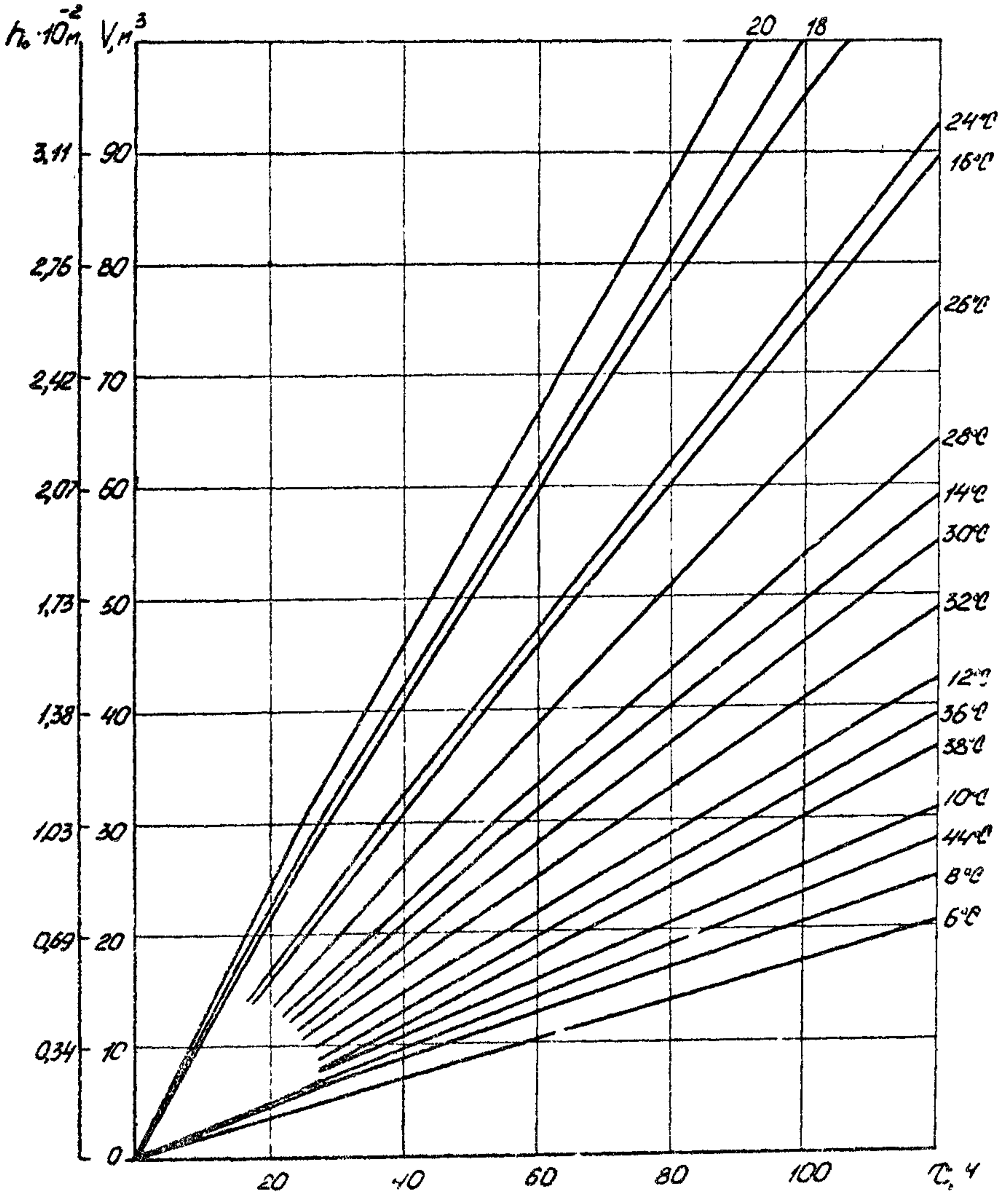
Рис. 26. Количество донного смоло-парафинового осадка, образующегося в резервуаре РС-50000 в течение одного цикла заполнения-опорожнения его в зависимости от времени и температуры хранения кудожовской нефти
