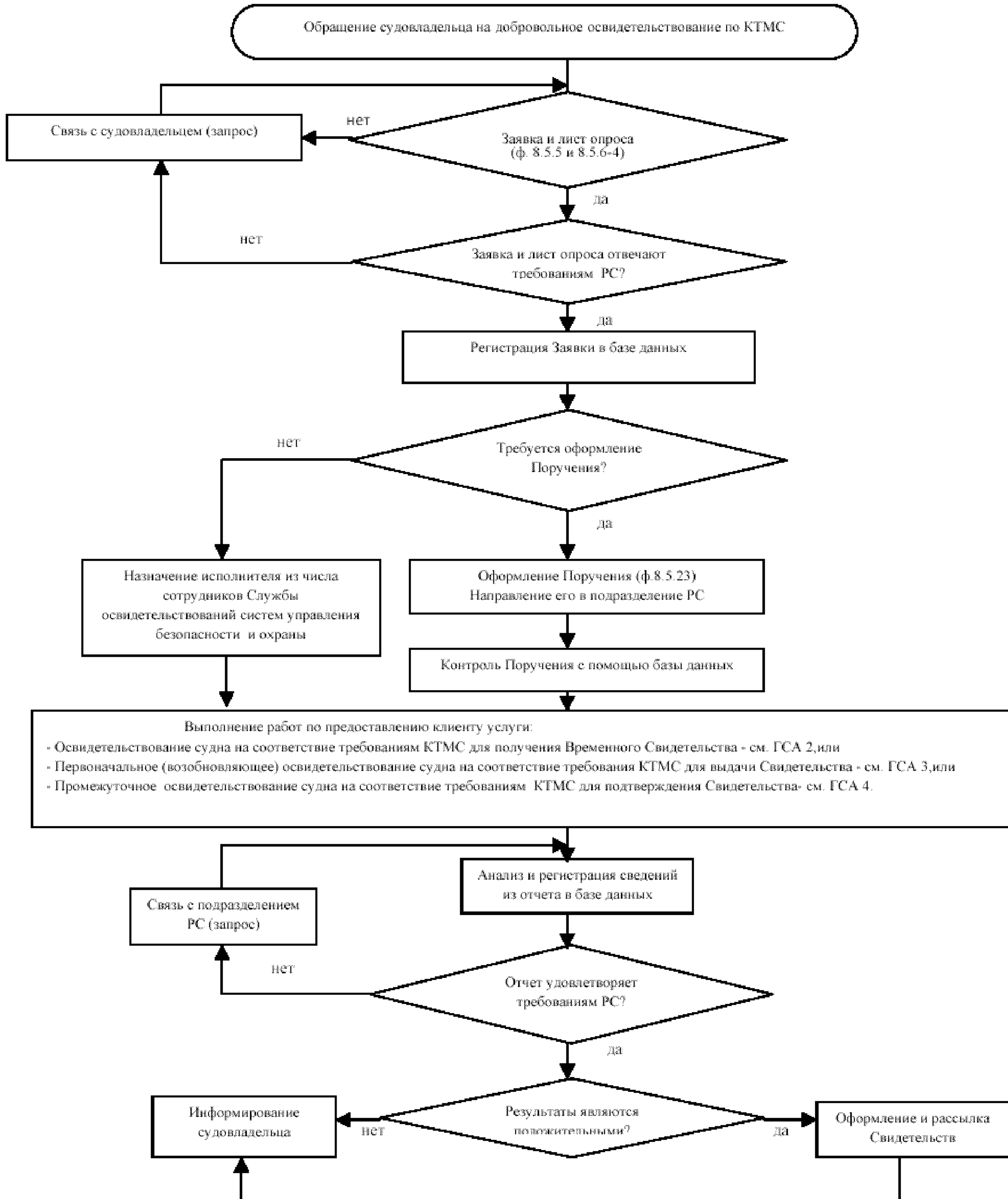
Граф-схема алгоритма общего взаимодействия РС с судовладельцем (ГСА 1)
