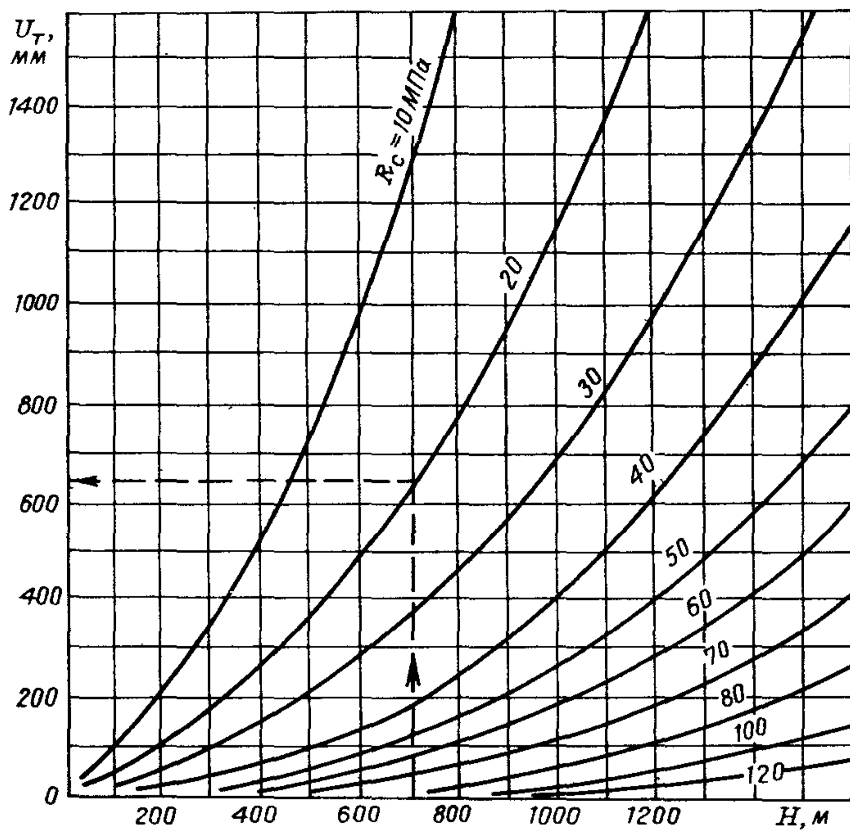
Рис. 2. Графики для определения типового смещения пород
