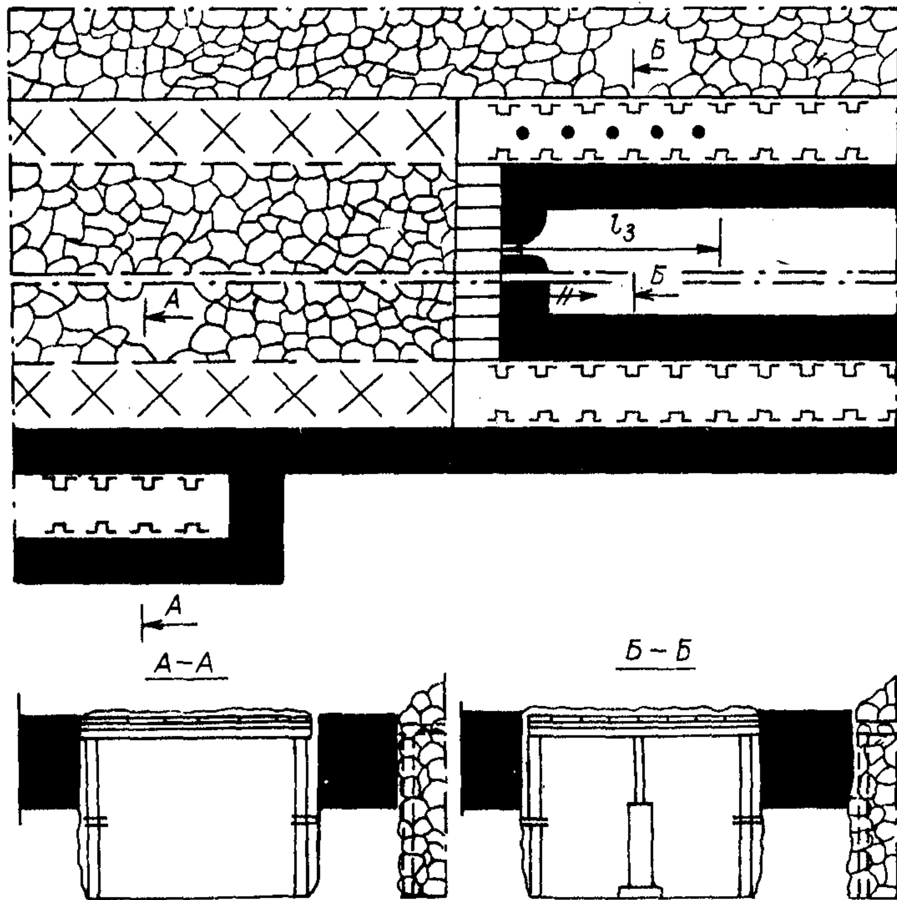
Рис. 25. Схема проведения выработок вприсечку к выработанному пространству
