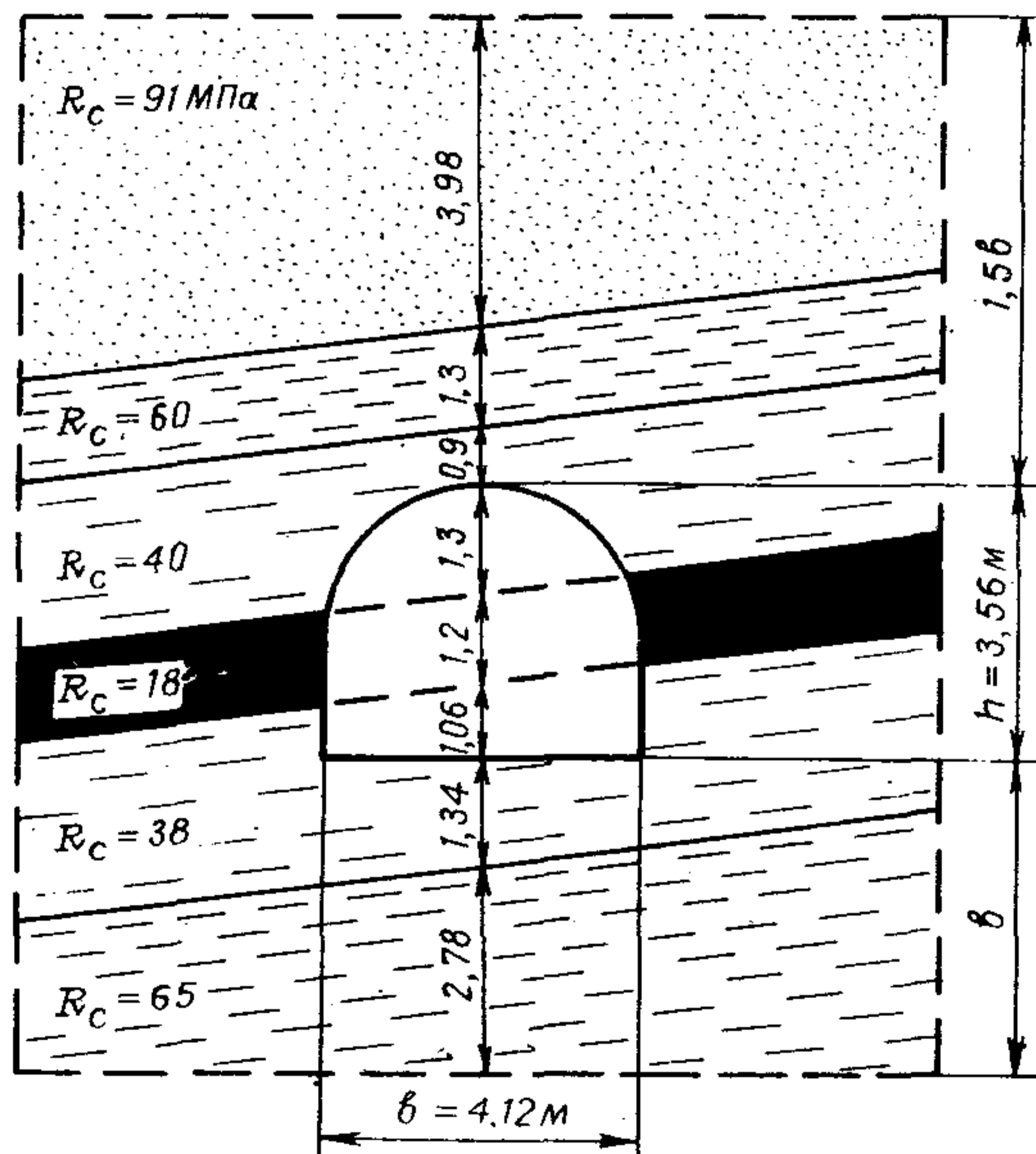
Рис. 23. Расчетная схема к примеру 1
