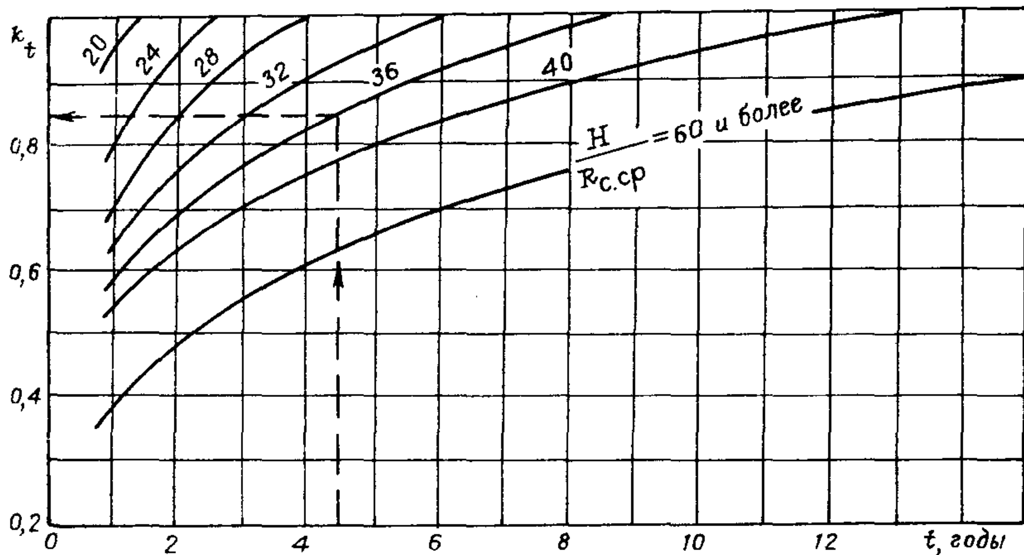
Рис. 3. График для определения k_t
