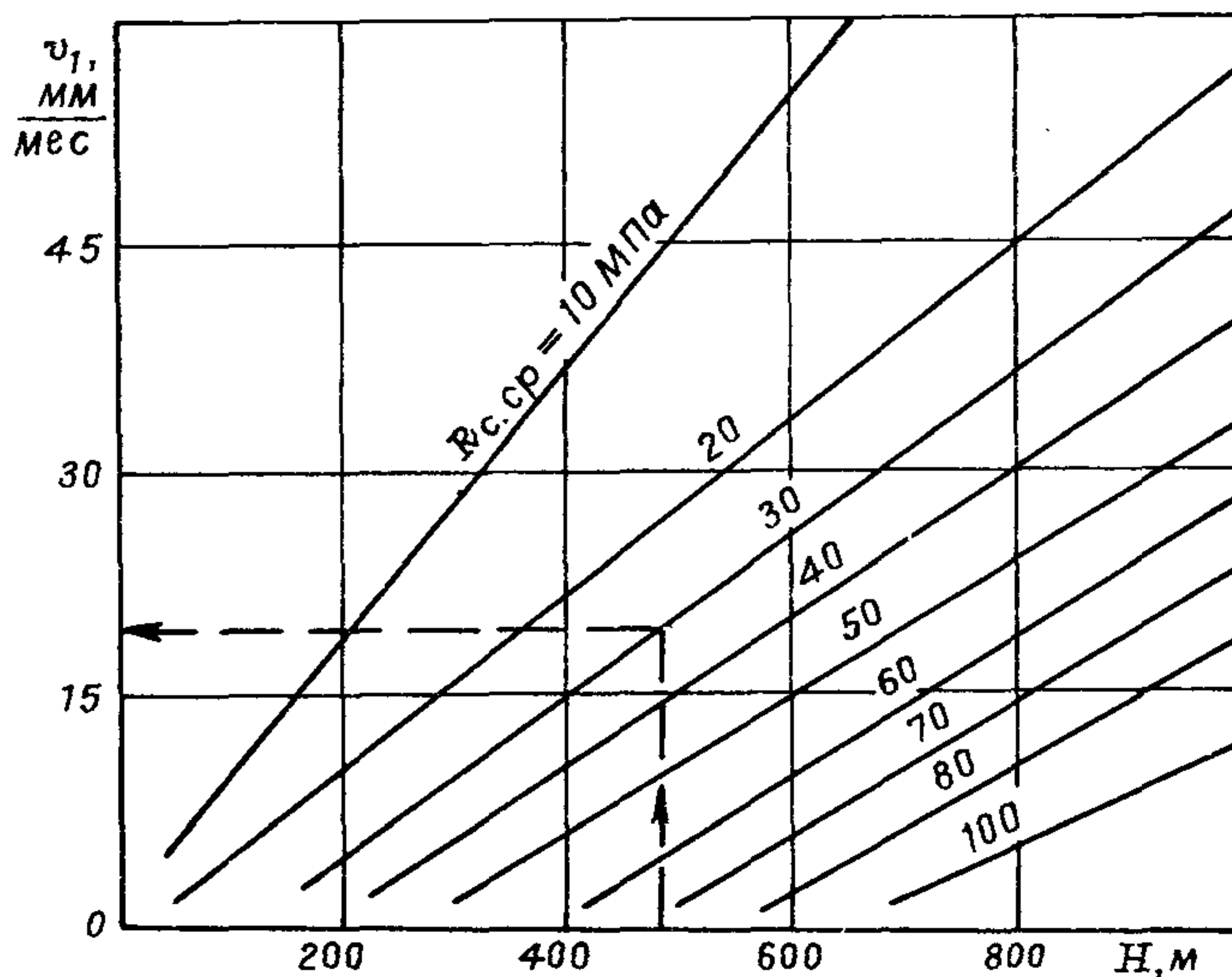
Рис. 12. Скорость смещений пород позади очистного забоя
