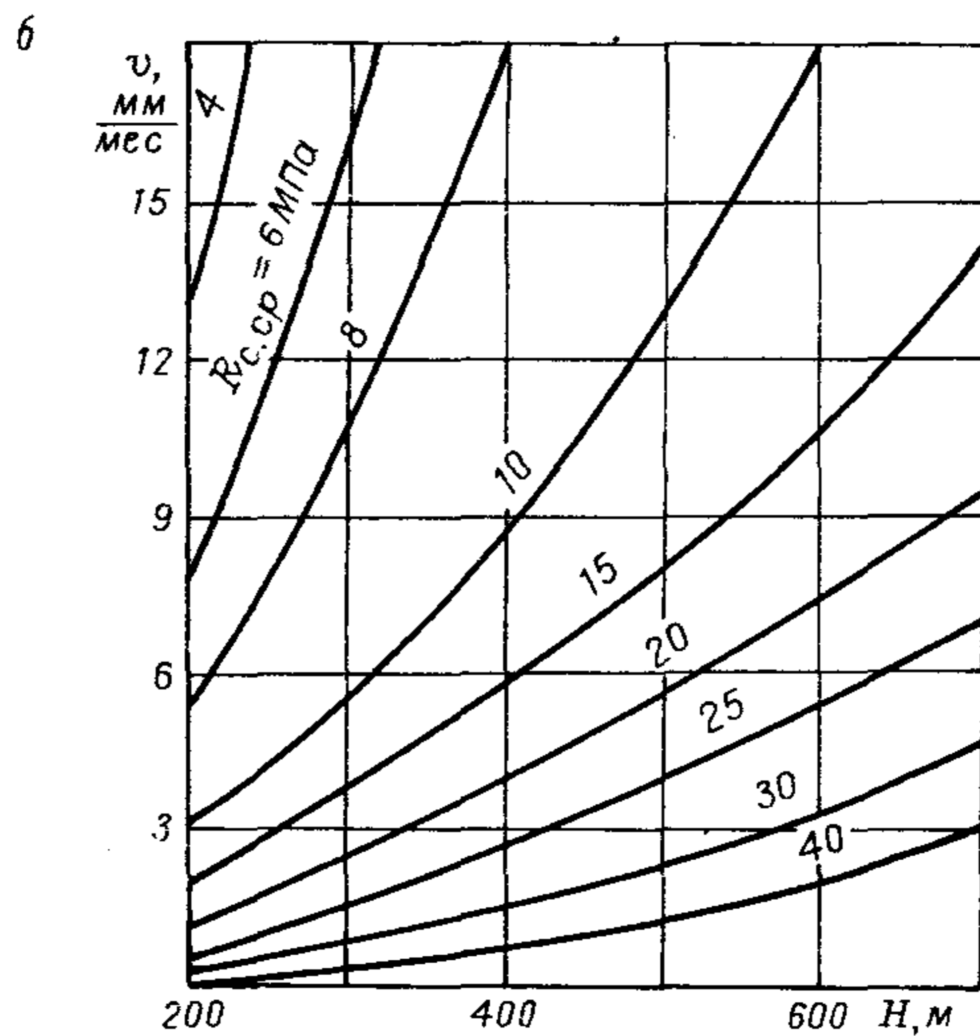
Рис. 17. Скорость смещения пород месторождений на глубинах: а — каменноугольных, до 200 м, б — 200—700 м
