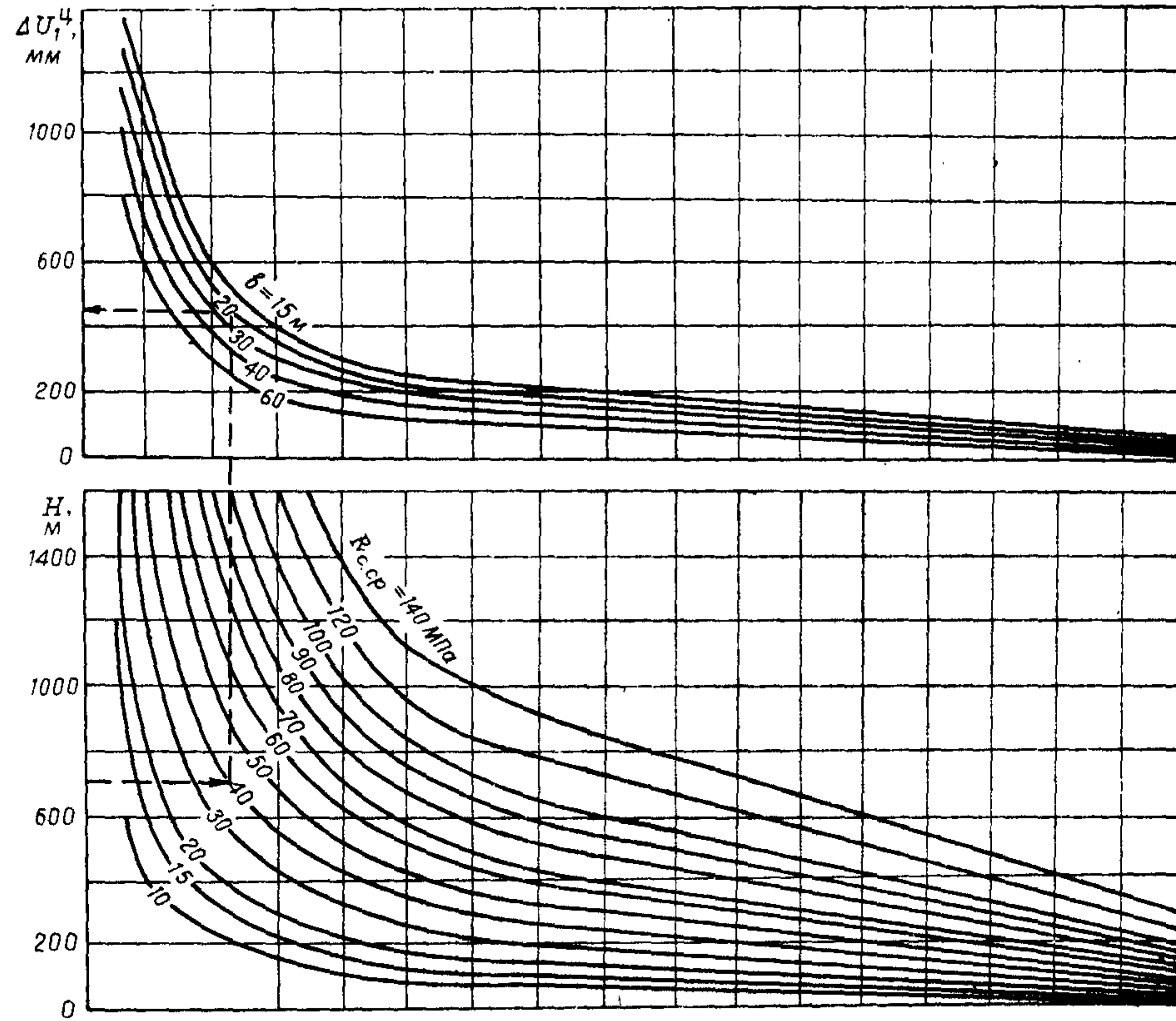
Рис. 10. Номограмма для определения \Delta U_1^4
