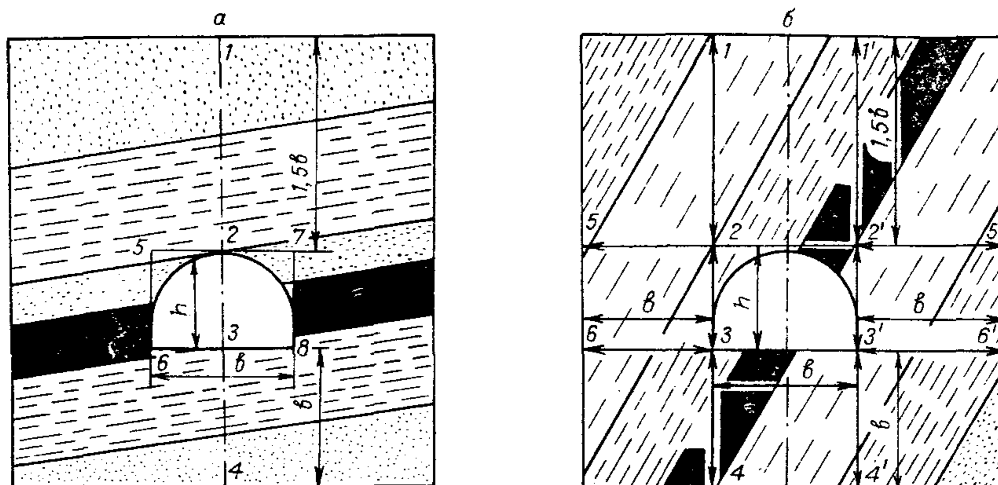
Рис. 1. Схемы к определению расчетного сопротивления пород сжатию:
