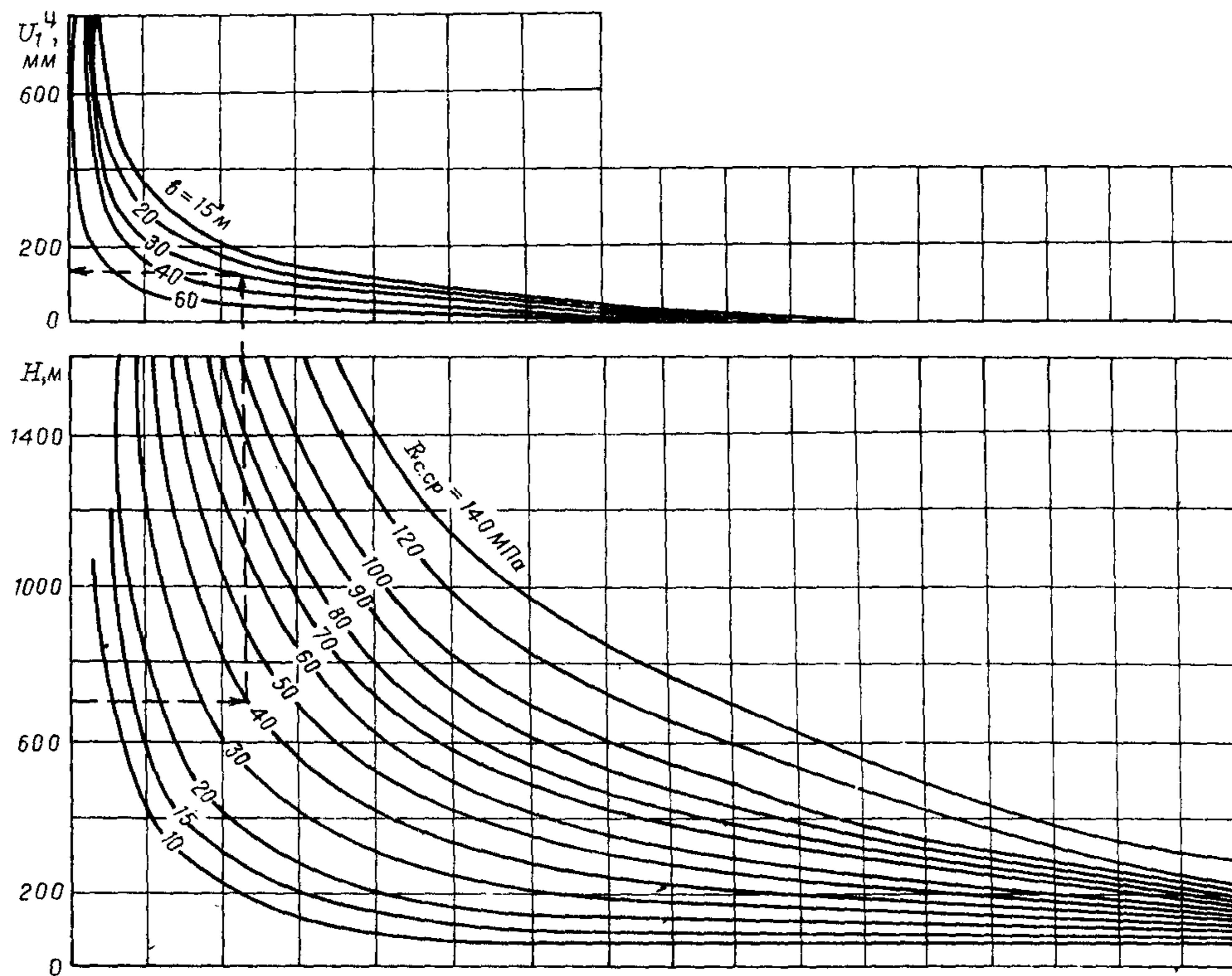
Рис. 9. Номограмма для определения U_1^{II}
