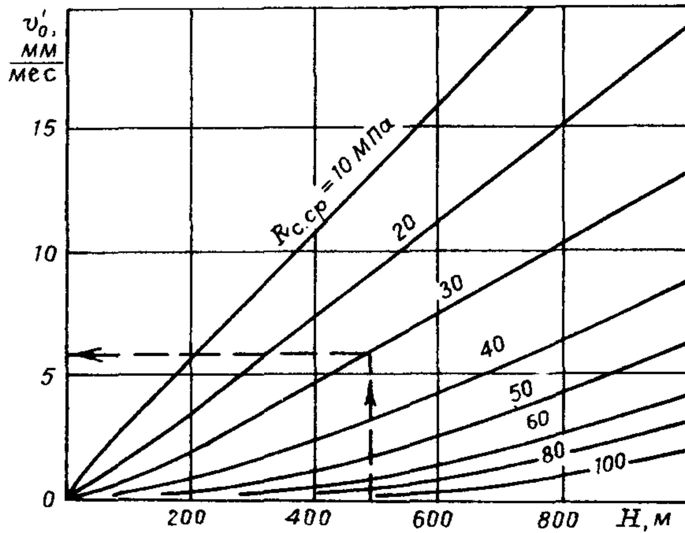
Рис. 14. Скорости смещений пород кровли в присечных выработках
