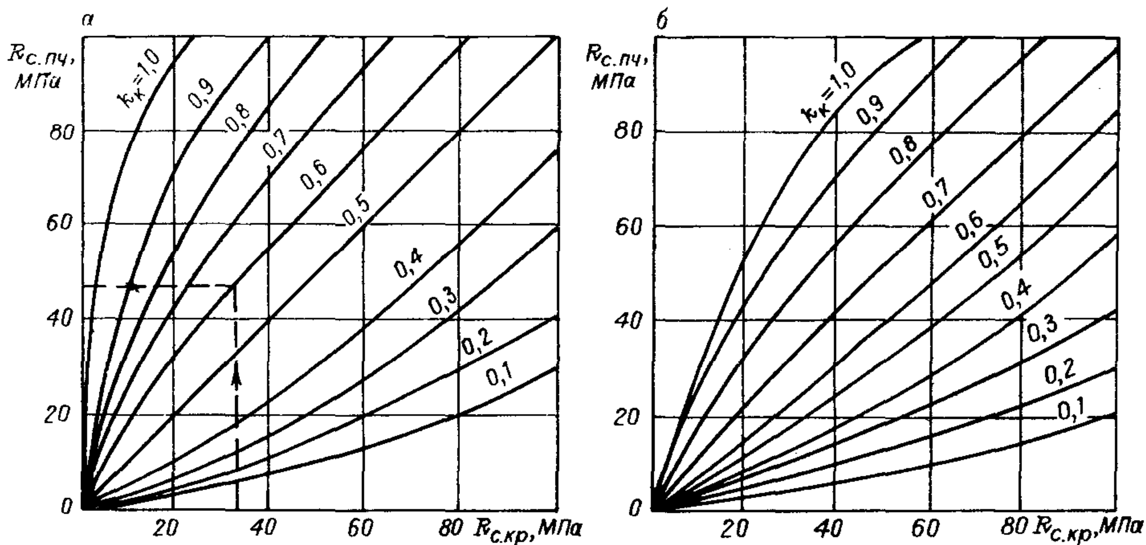
Рис. 5. Графики для определения коэффициента k_k :
