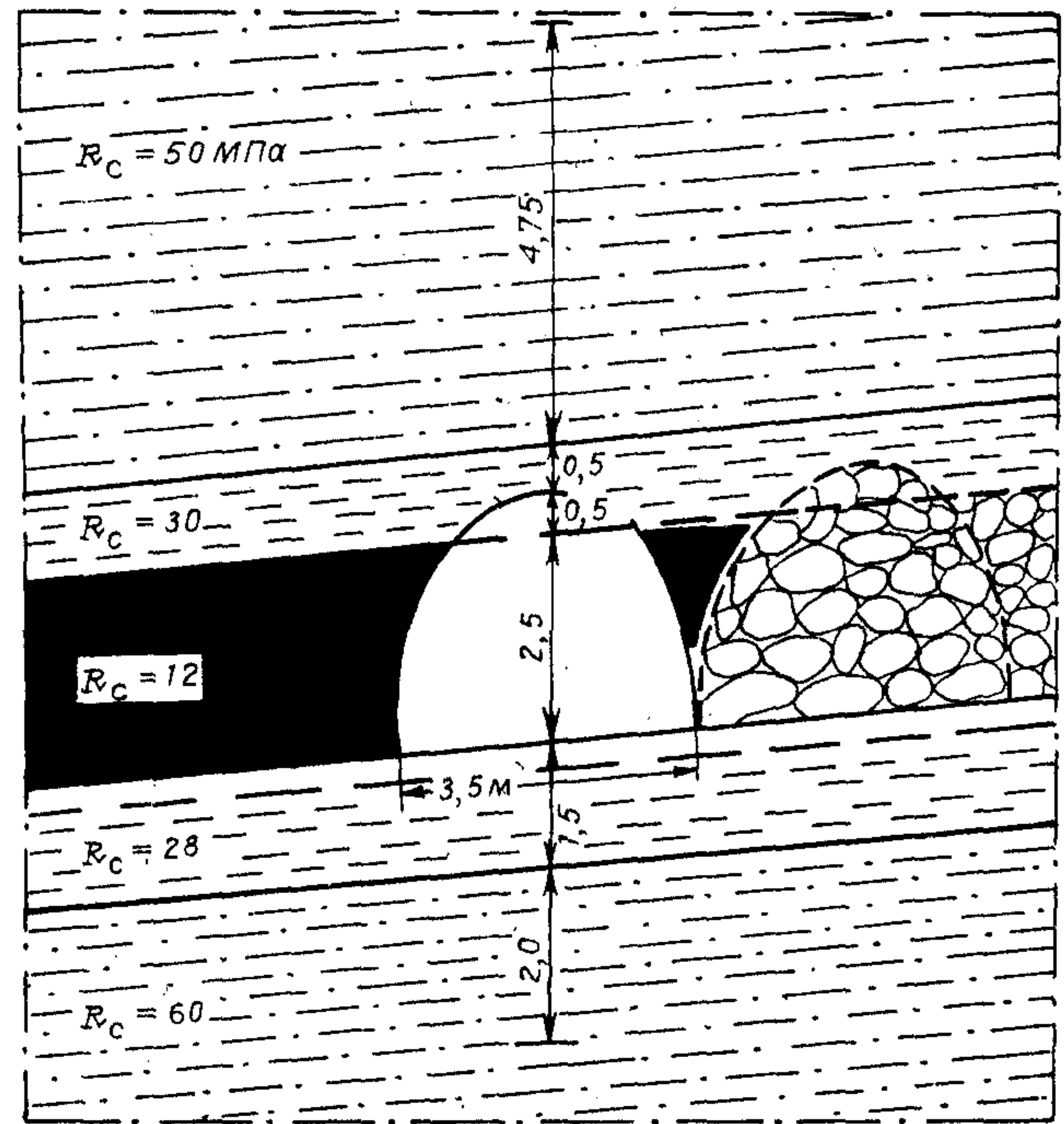
Рис. 26. Расчетная схема к примеру 4
