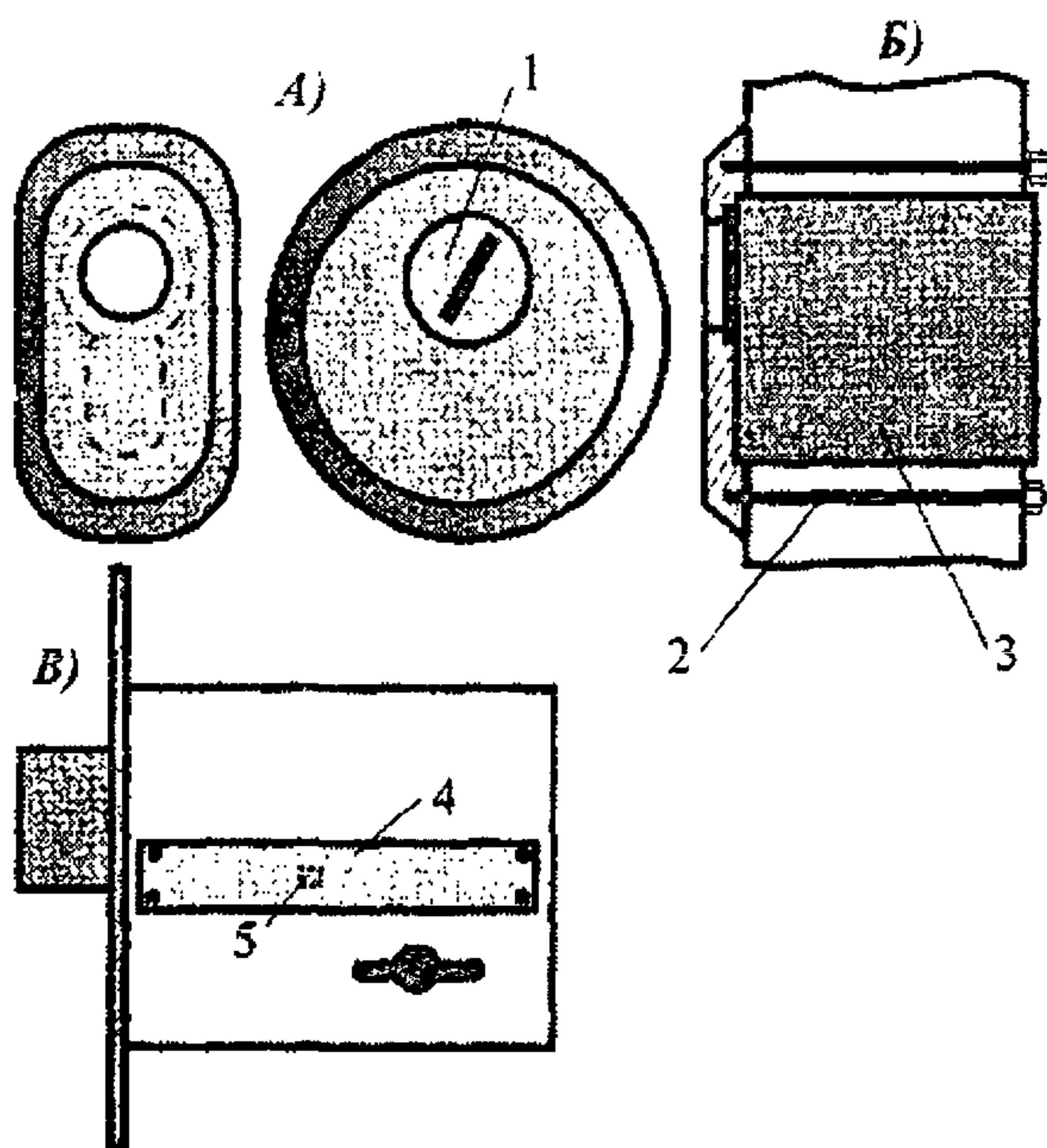
Рисунок 8 - Примеры защитных накладок от высверливания и сворачивания А) - типы защитных накладок для цилиндрических механизмов секретности; Б) - крепление защитной пластины к дверному полотну; В) - сувальдный замок с защитой стойки хвостовика засова 1 - свободно вращающаяся пластина из термообработанной стали; 2 - штифта с резьбой М5 или более; 3- цилиндрический МС; 4 - свободно вращающаяся шайба из термообработанной стали; 5 - стойка хвостовика засова
