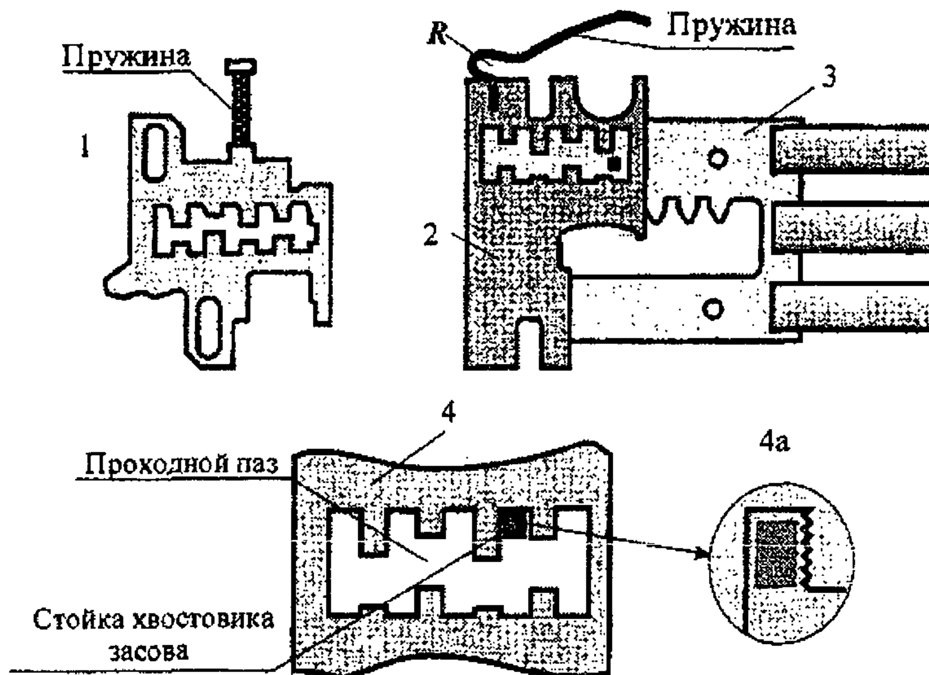
Рисунок 9 - Элементы сувальдных МС:
