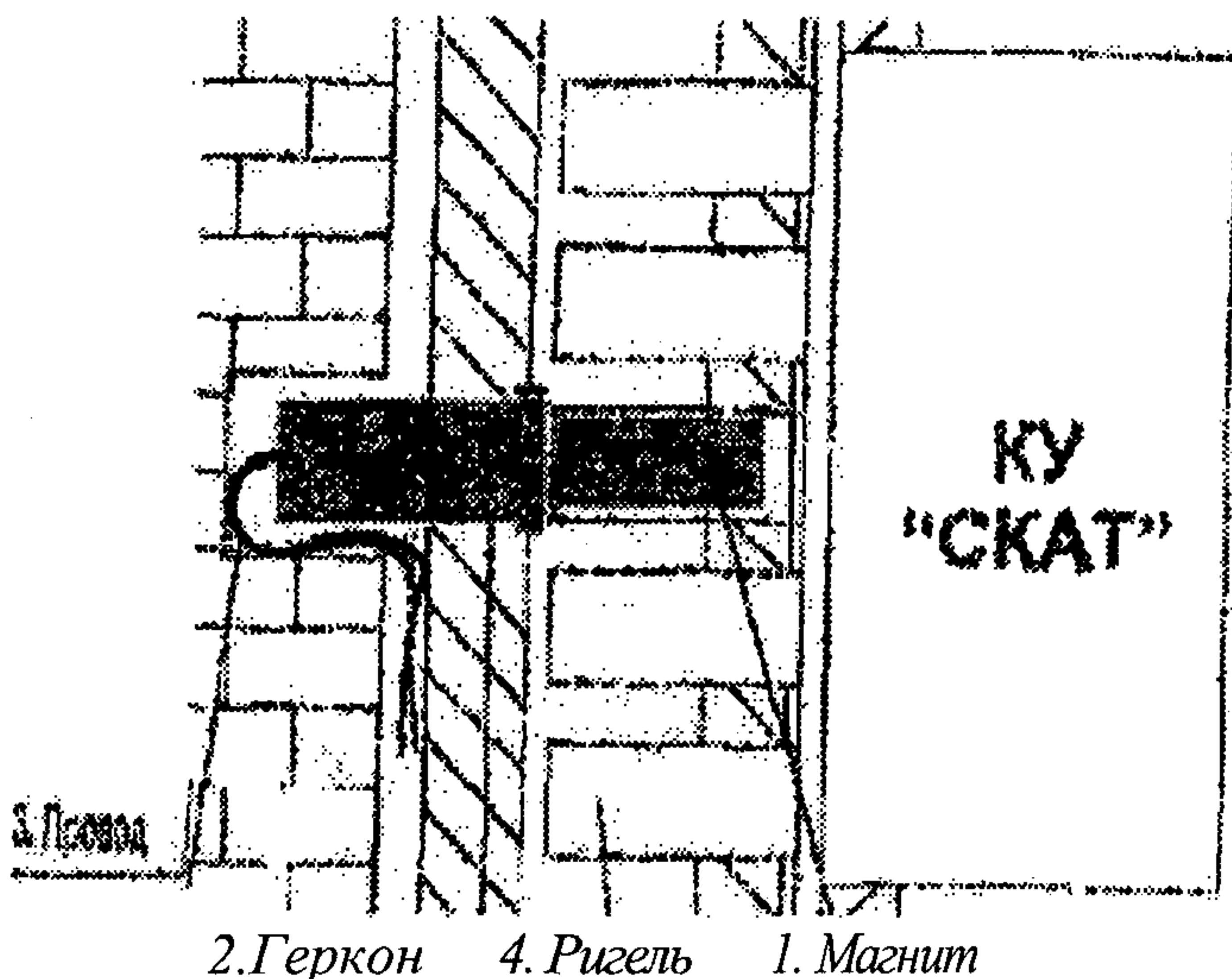
Рисунок 14-1 – Пример установки КУ «СКАТ»
