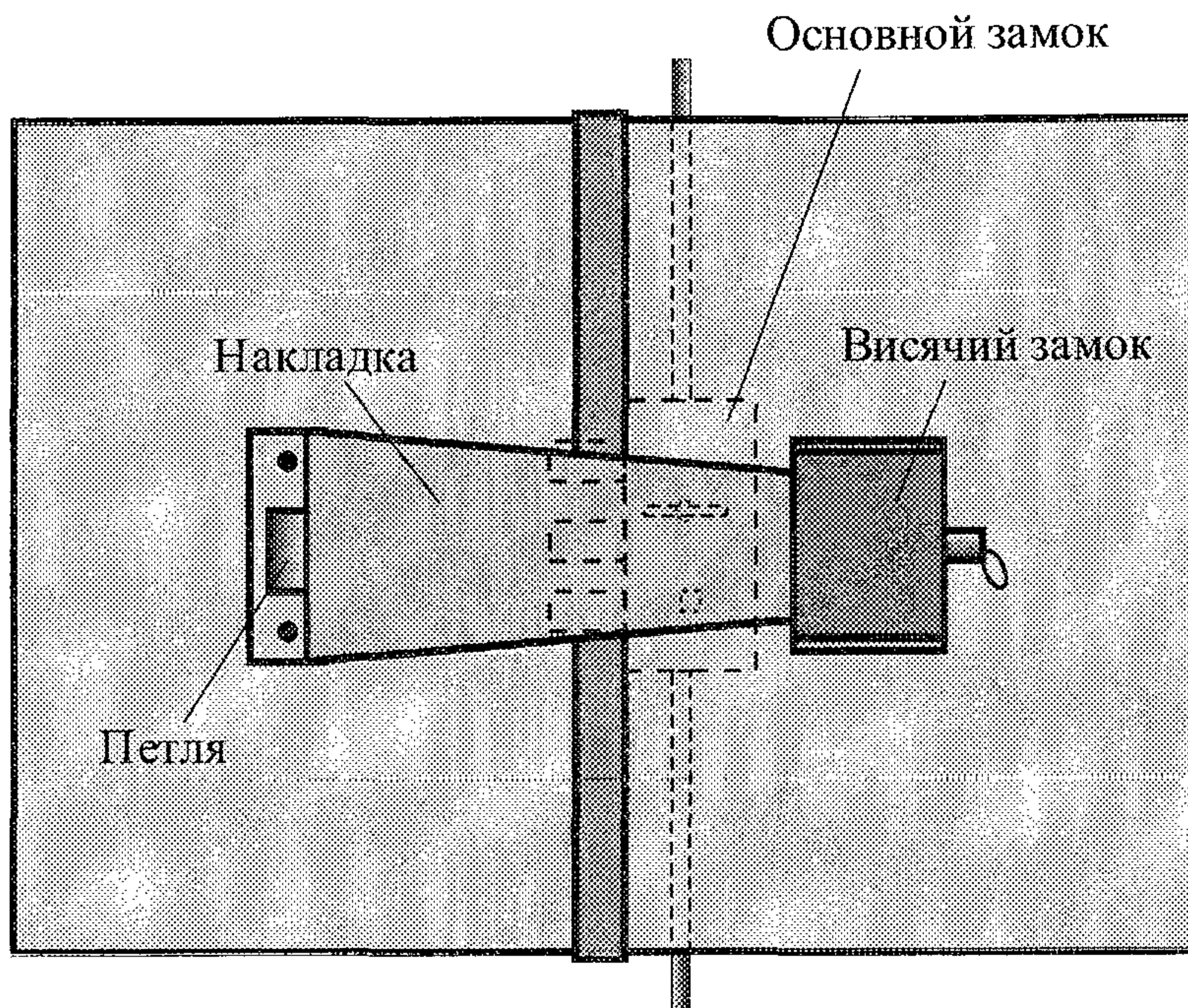
Рисунок 19 – Блокировка гаражных ворот
