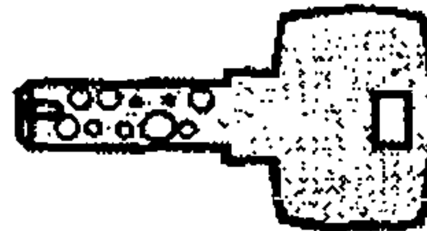
Рисунок 6 - Примеры ключей для штифтовых МС с "перфорацией": 1 - однорядного; 2 - двухрядного
