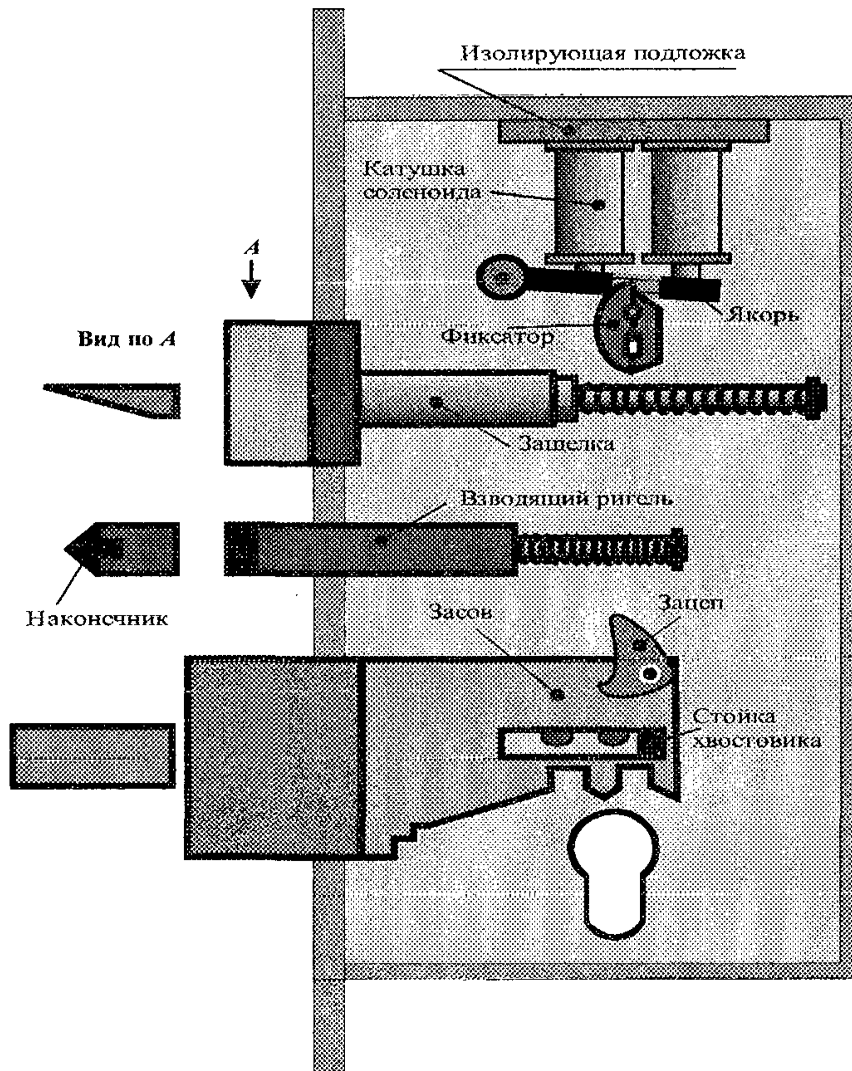
Рисунок 13 - Замок с электроблокировкой (рычаги и тяги не показаны)
