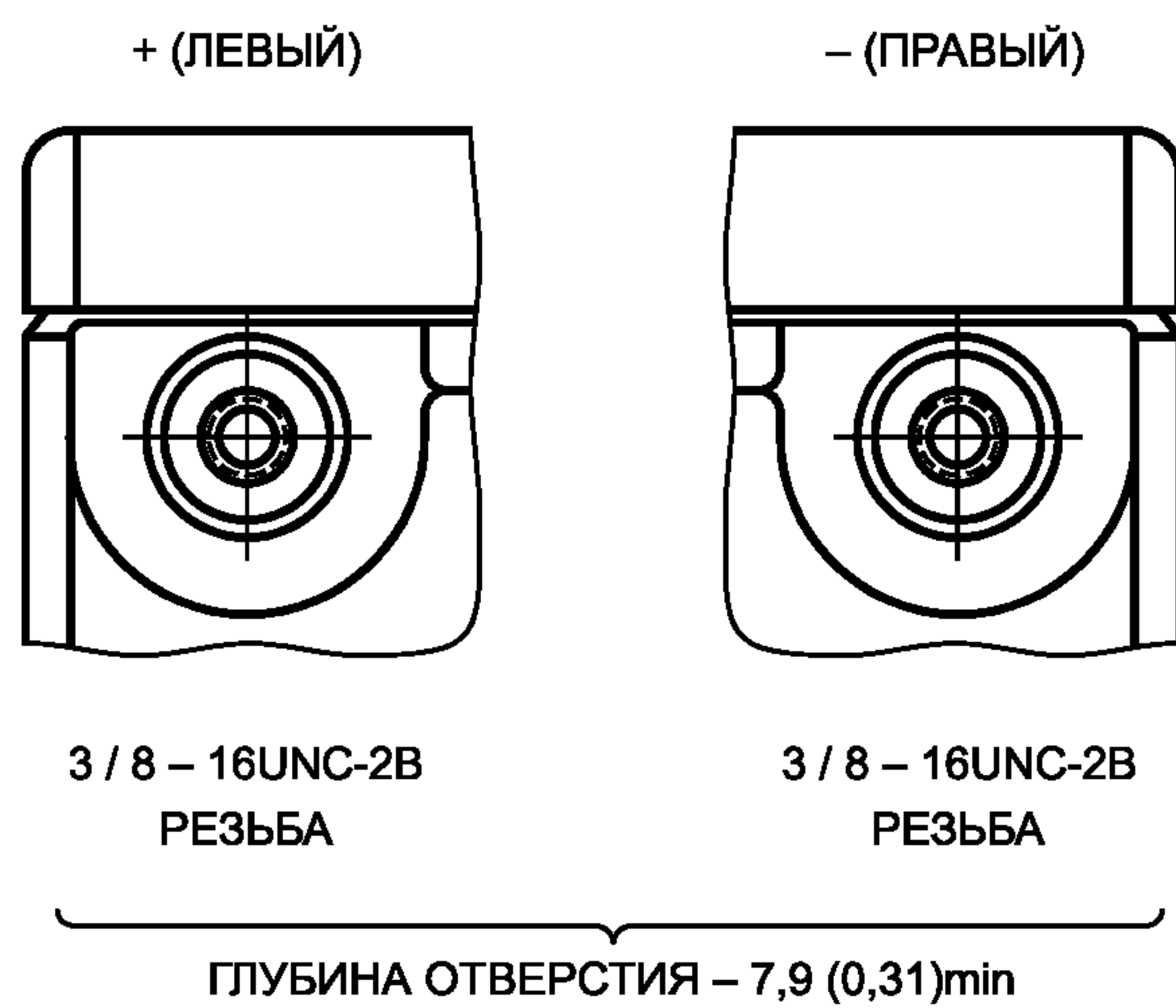
Рисунок 13 — Углубления боковых выводов
