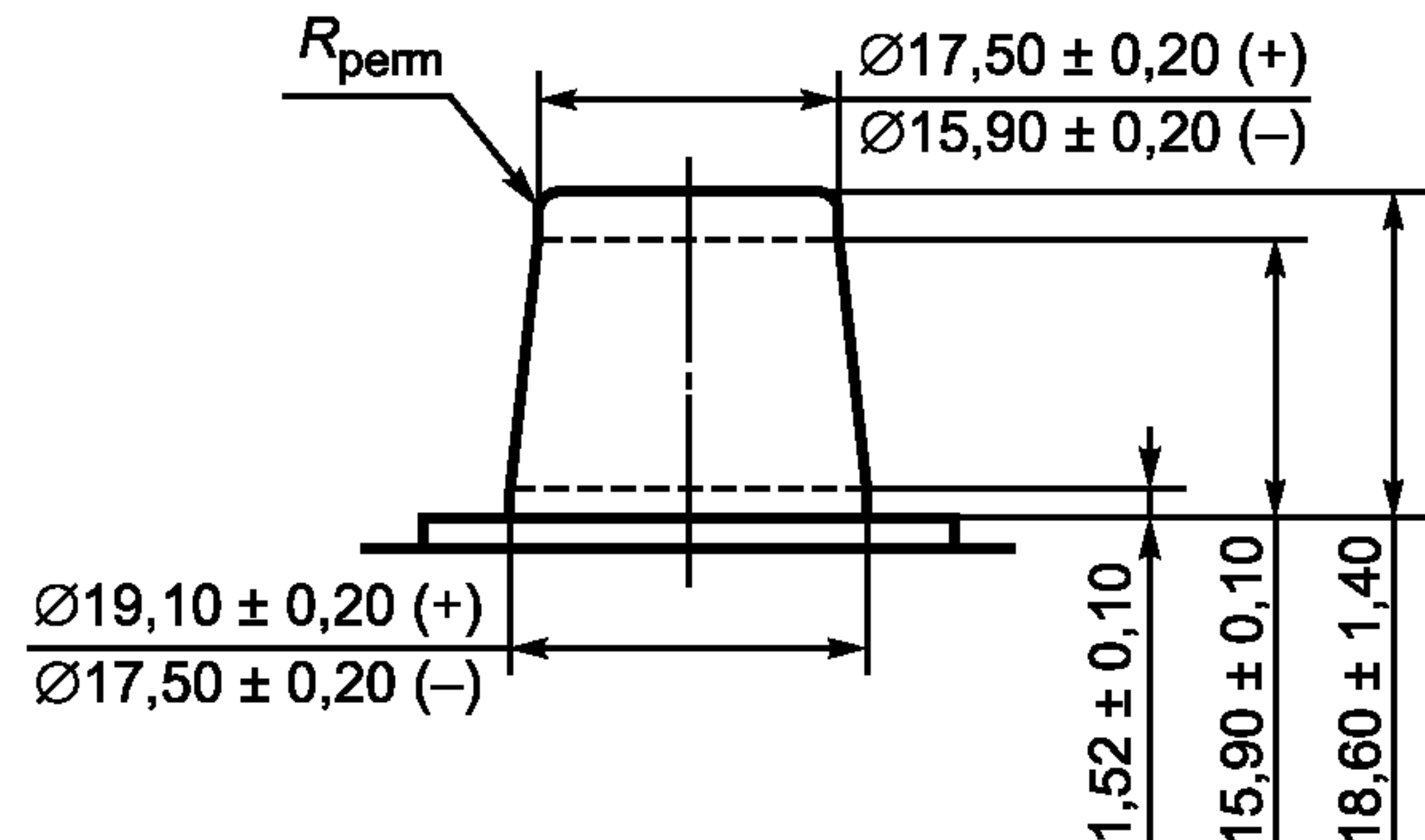
Рисунок 12 — Размеры выводов, мм (1:9 конусность)
