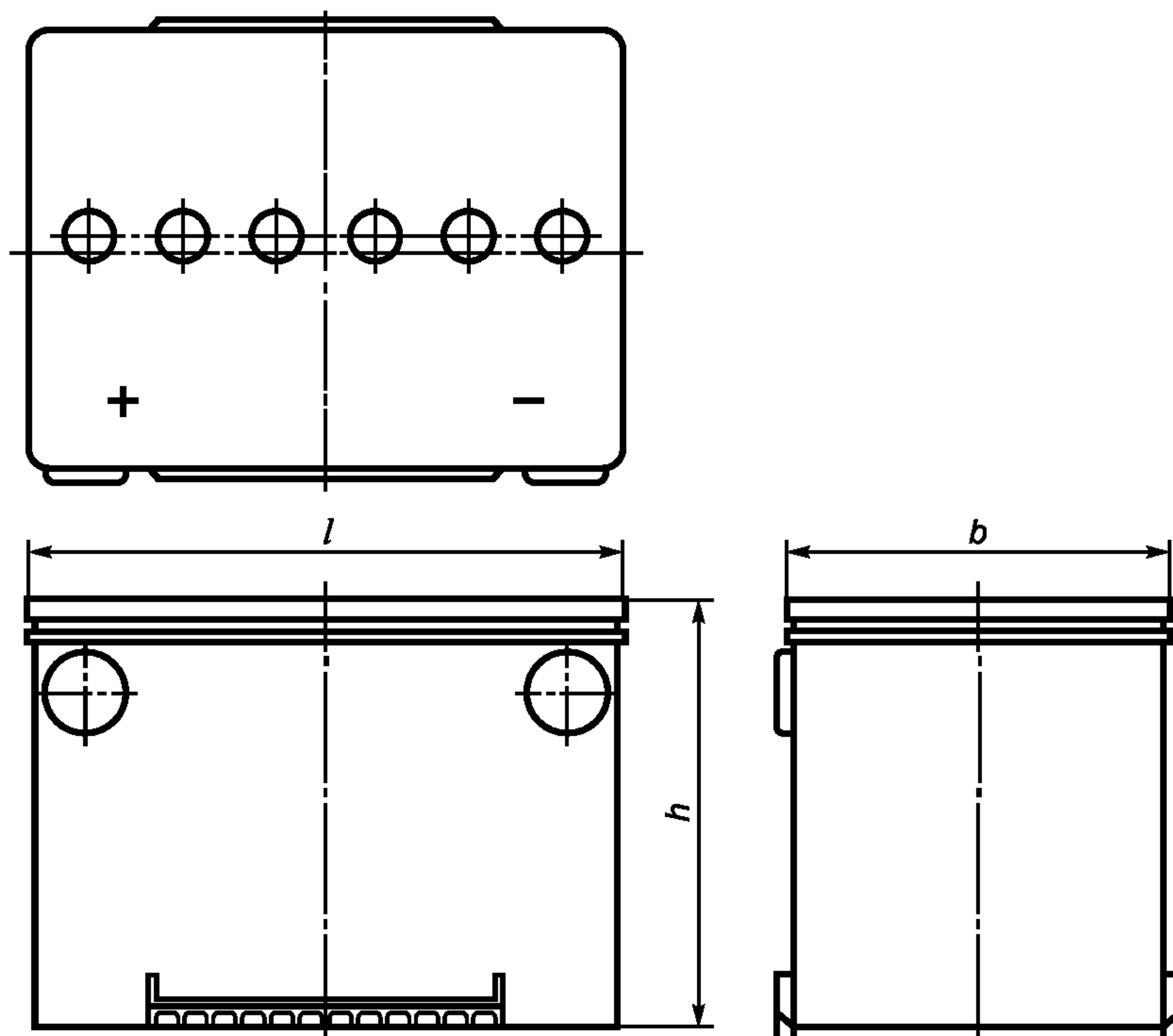
Рисунок 22 — Размеры типов 78, 100
