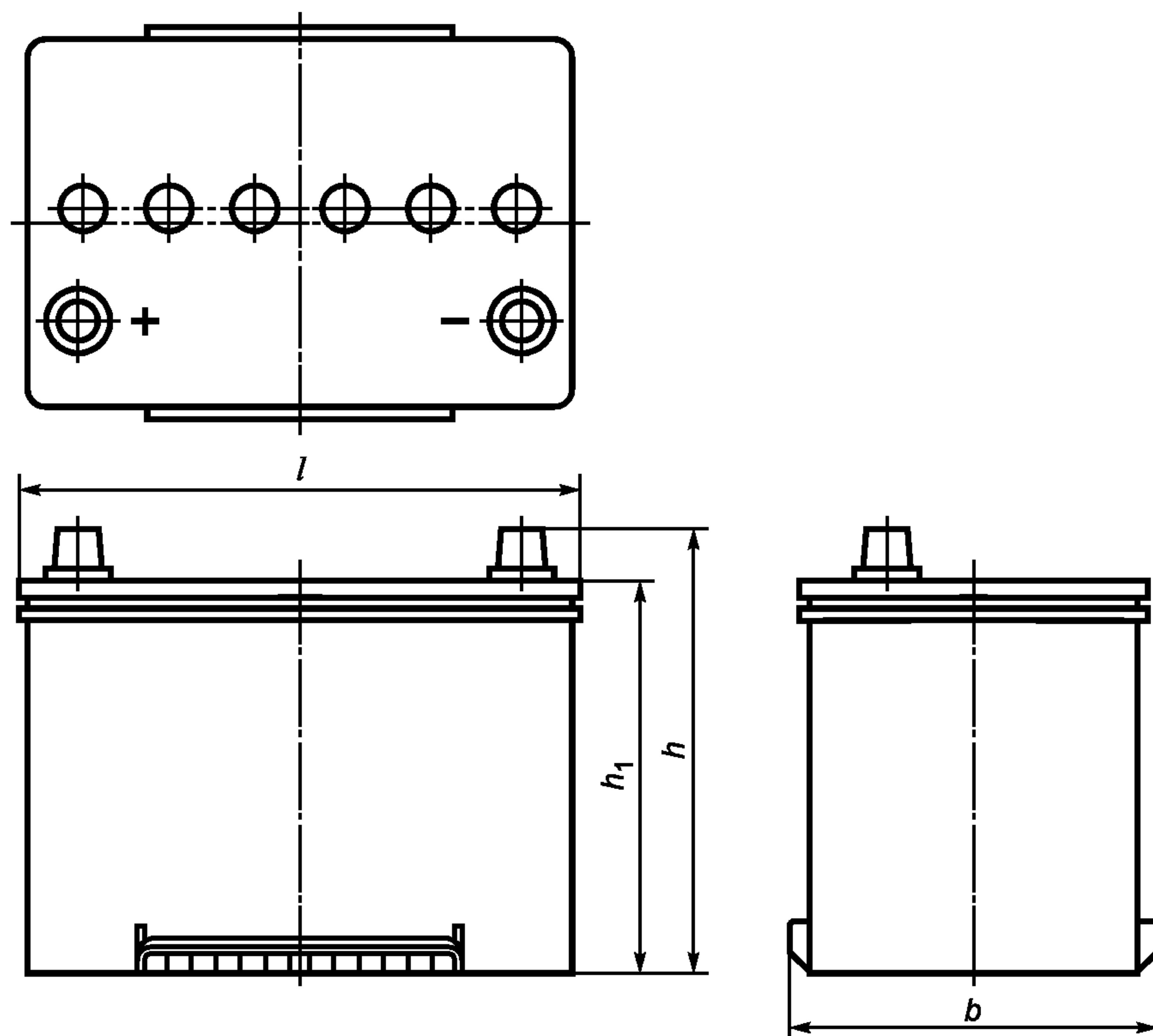
Рисунок 18 — Размеры типов 27, 34, 86
