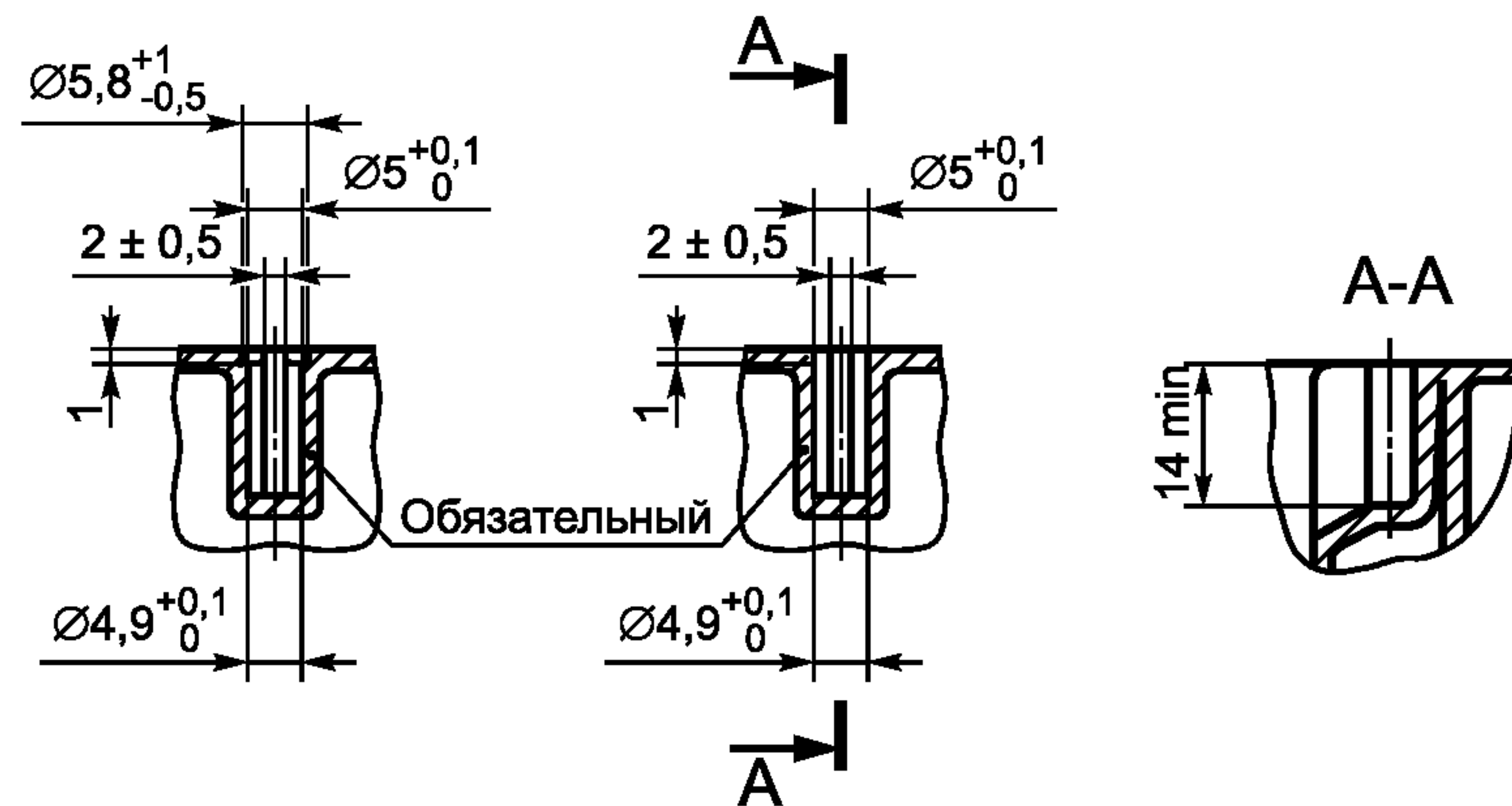
Рисунок 9 — Глухие отверстия защитной оболочки выводов (деталь К)
