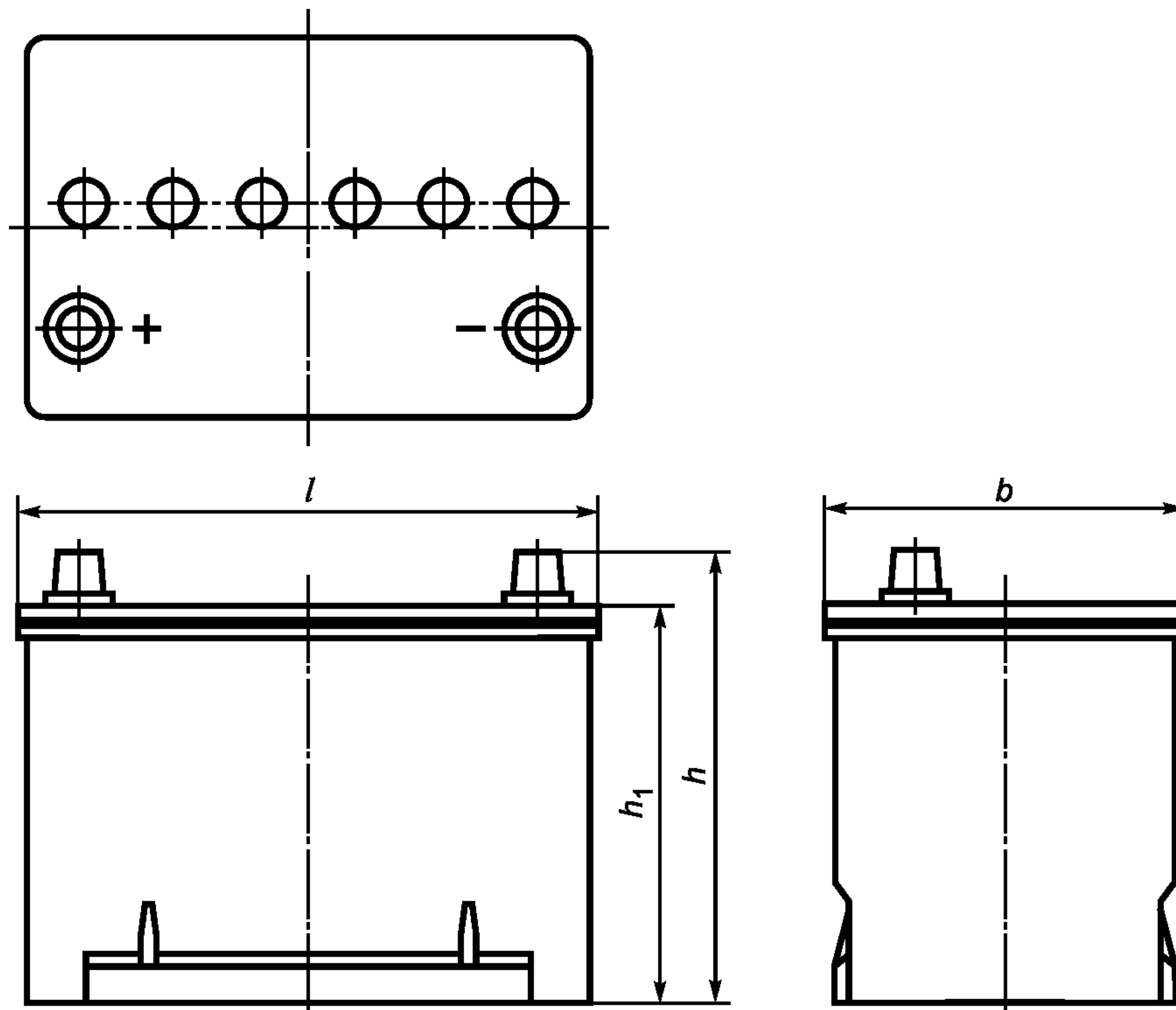
Рисунок 20 — Размеры типов 59, 65
