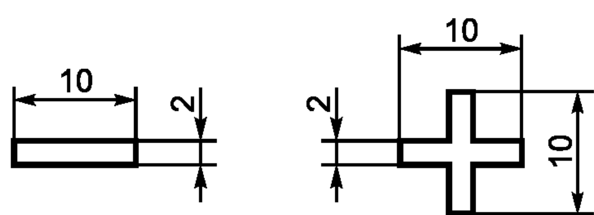
Рисунок 1 — Маркировка полярности
