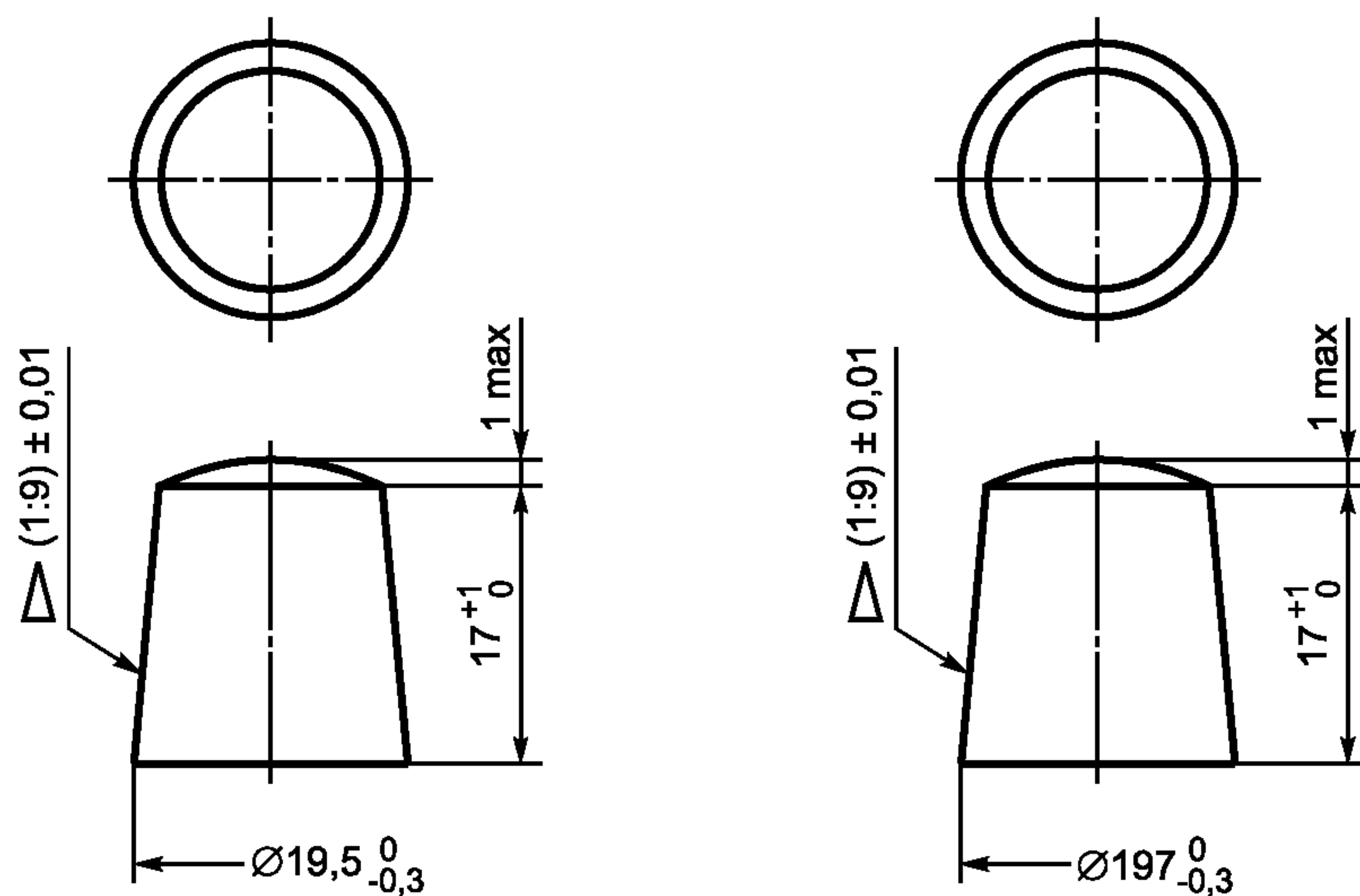
Рисунок 28а — Положительный вывод
