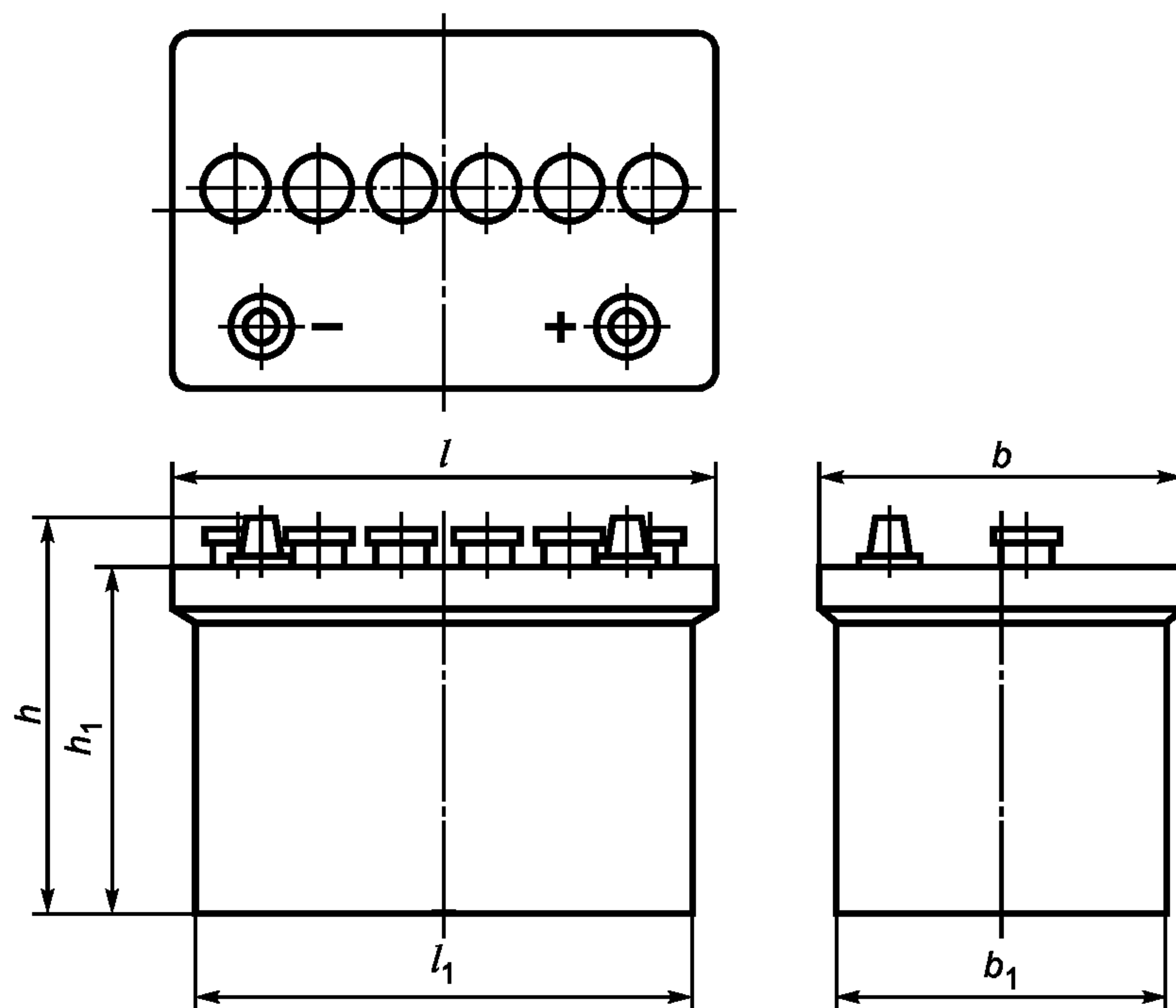
Рисунок 24 — Основные размеры батарей
