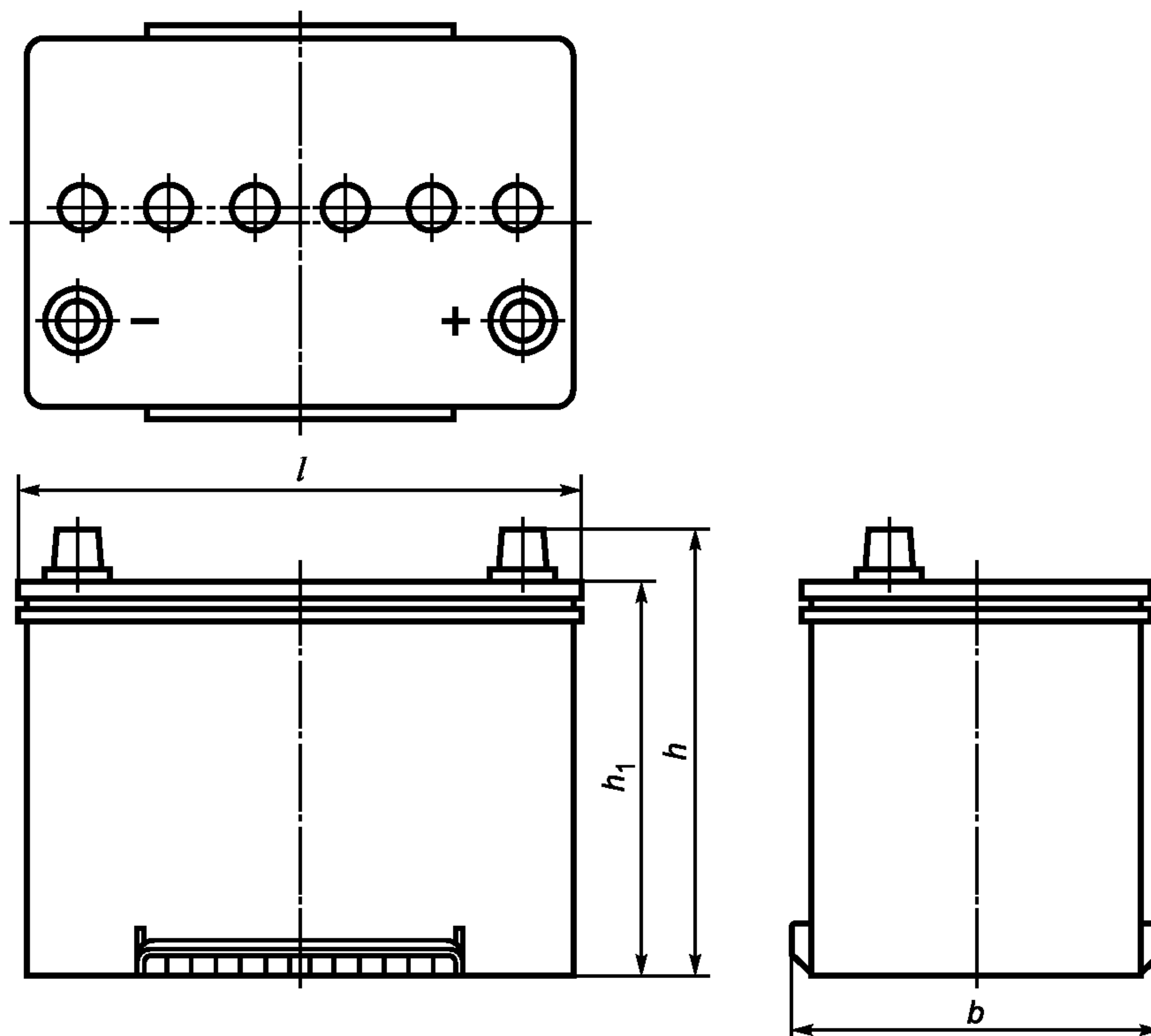
Рисунок 17 — Размеры типов 26R, 85
