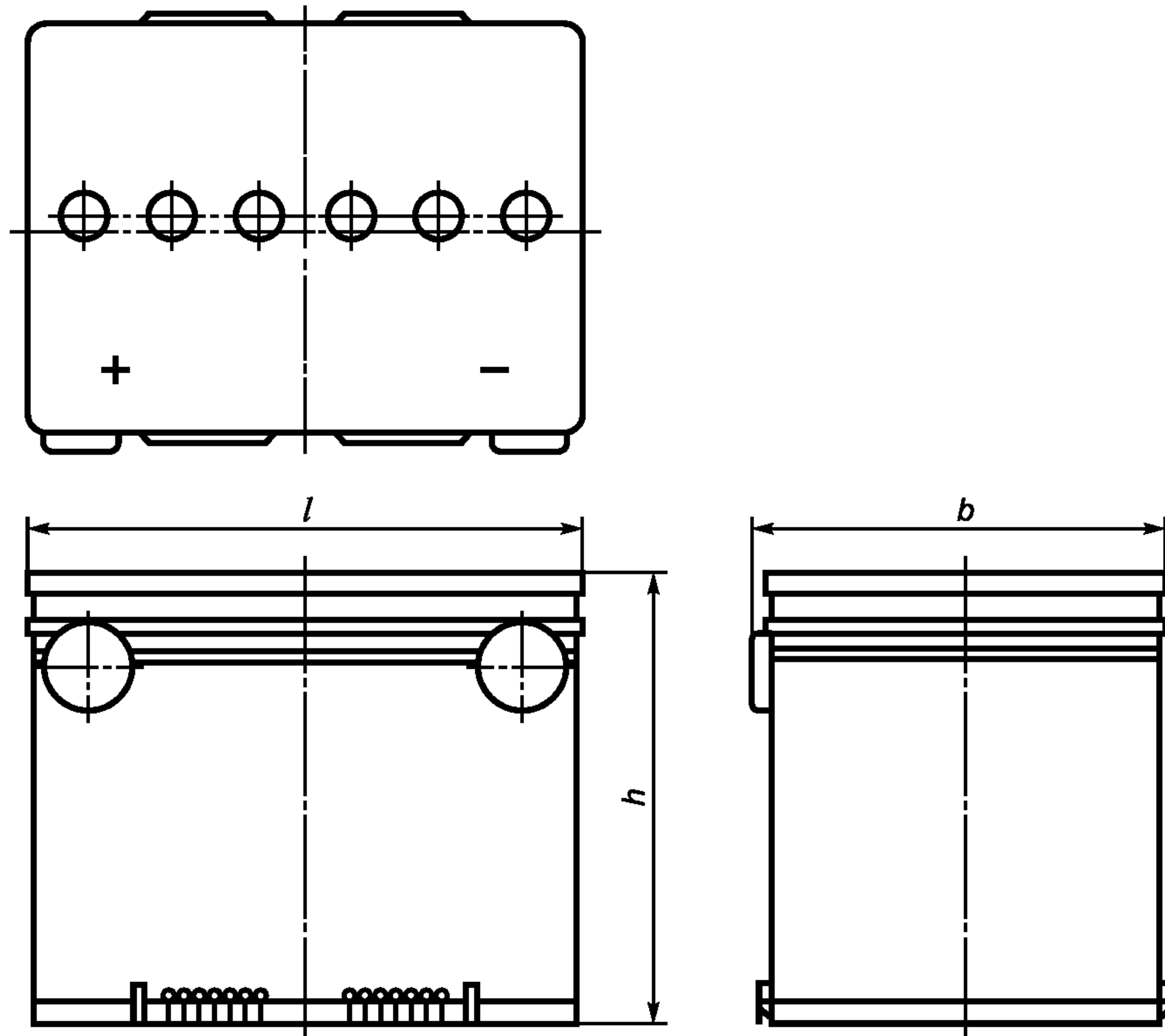
Рисунок 21 — Размеры типа 75
