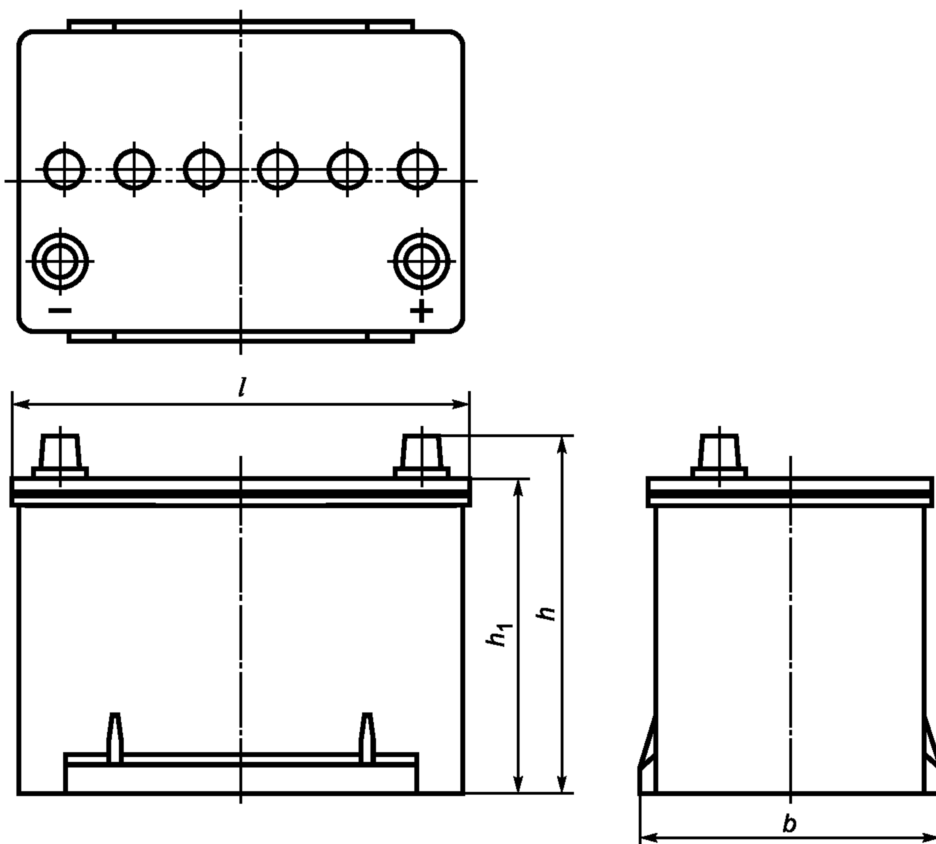
Рисунок 19 — Размеры типа 36R
