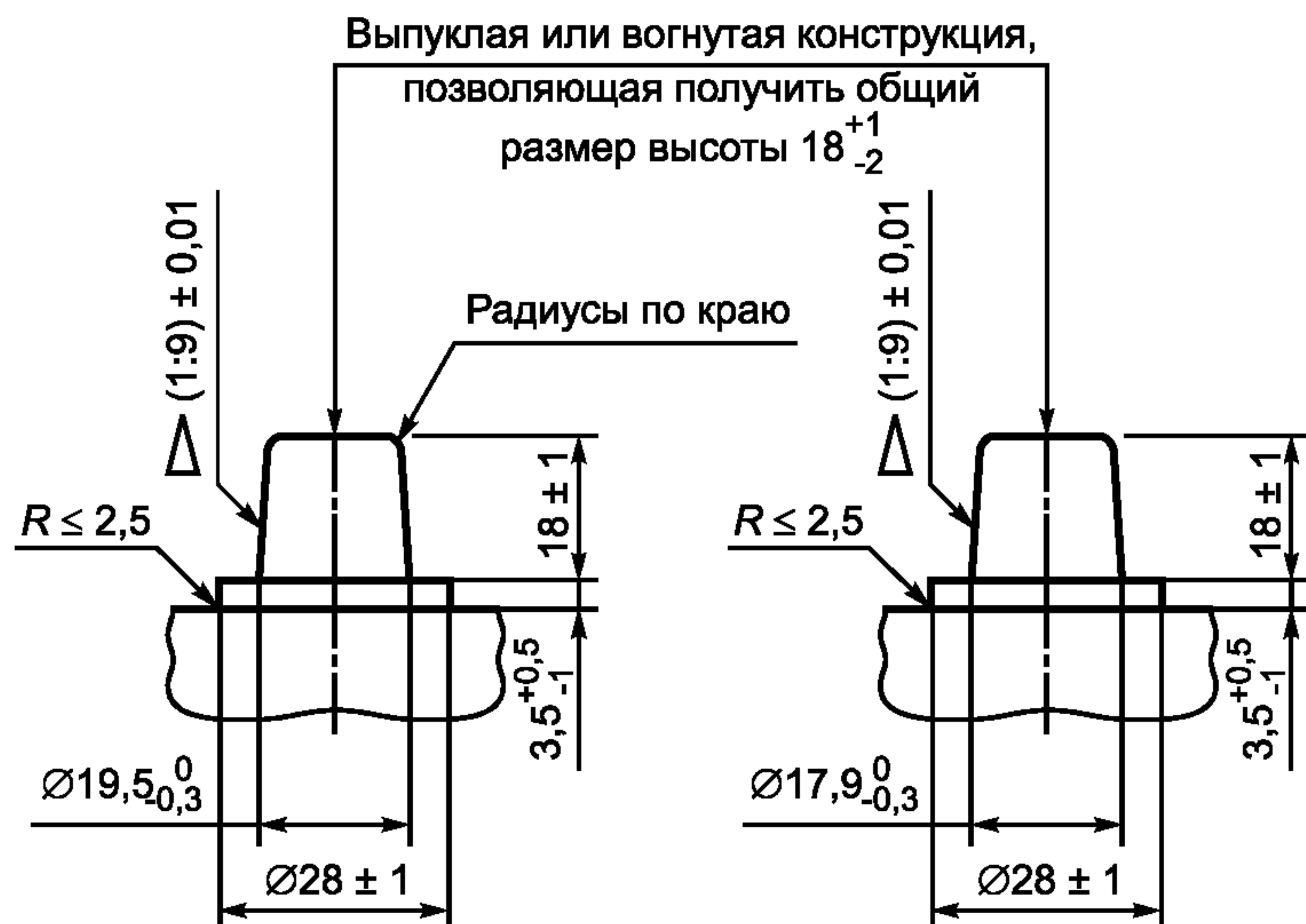
Рисунок 7а — Положительный вывод Рисунок 7b — Отрицательный вывод
