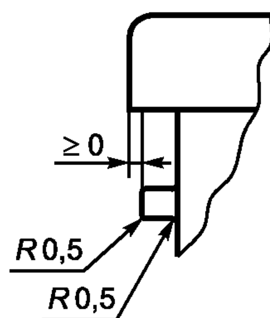
Рисунок 30 — Захваты для роботов, деталь X
