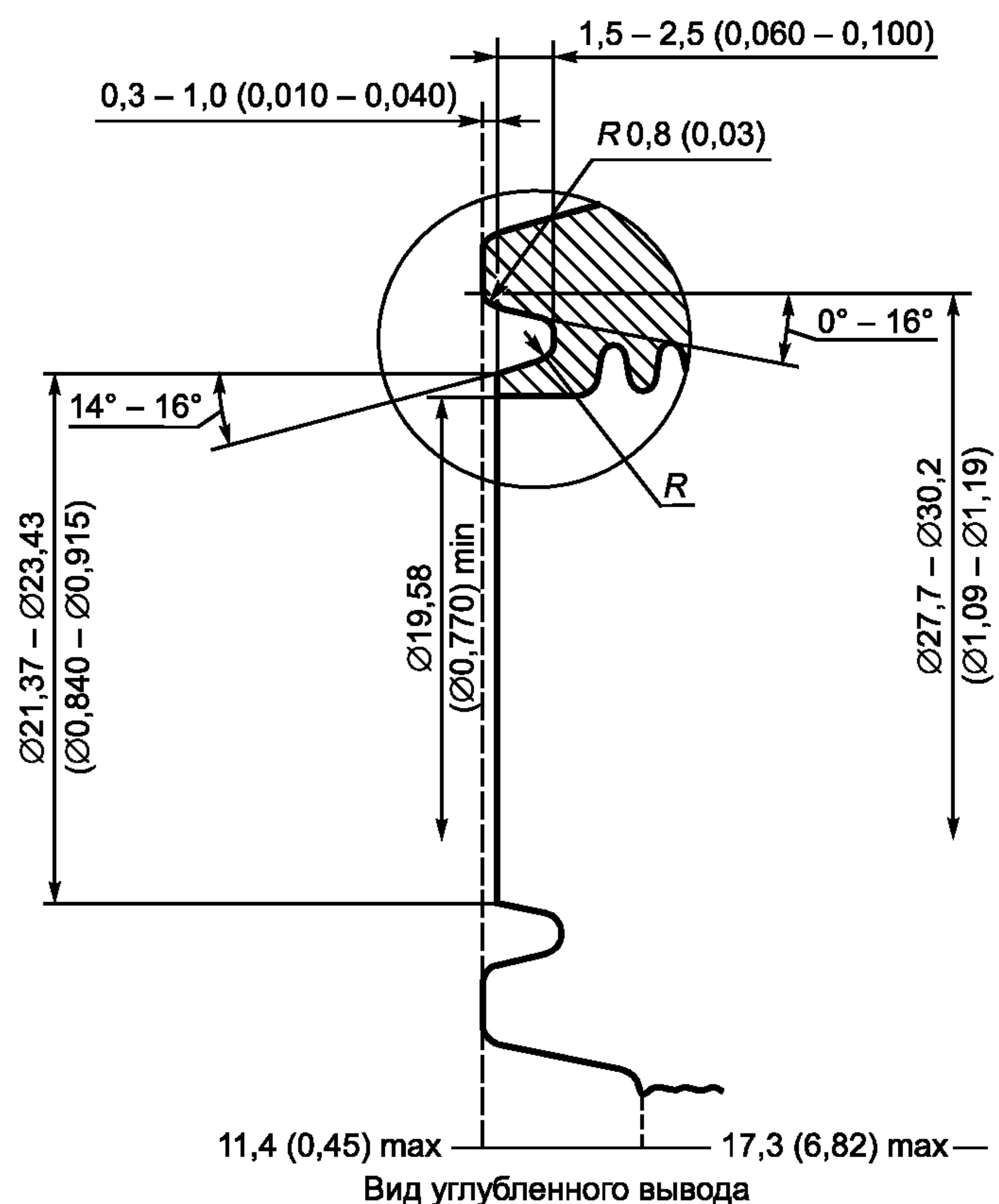
Рисунок 14 — Размеры углублений боковых выводов, мм (дюйм)
