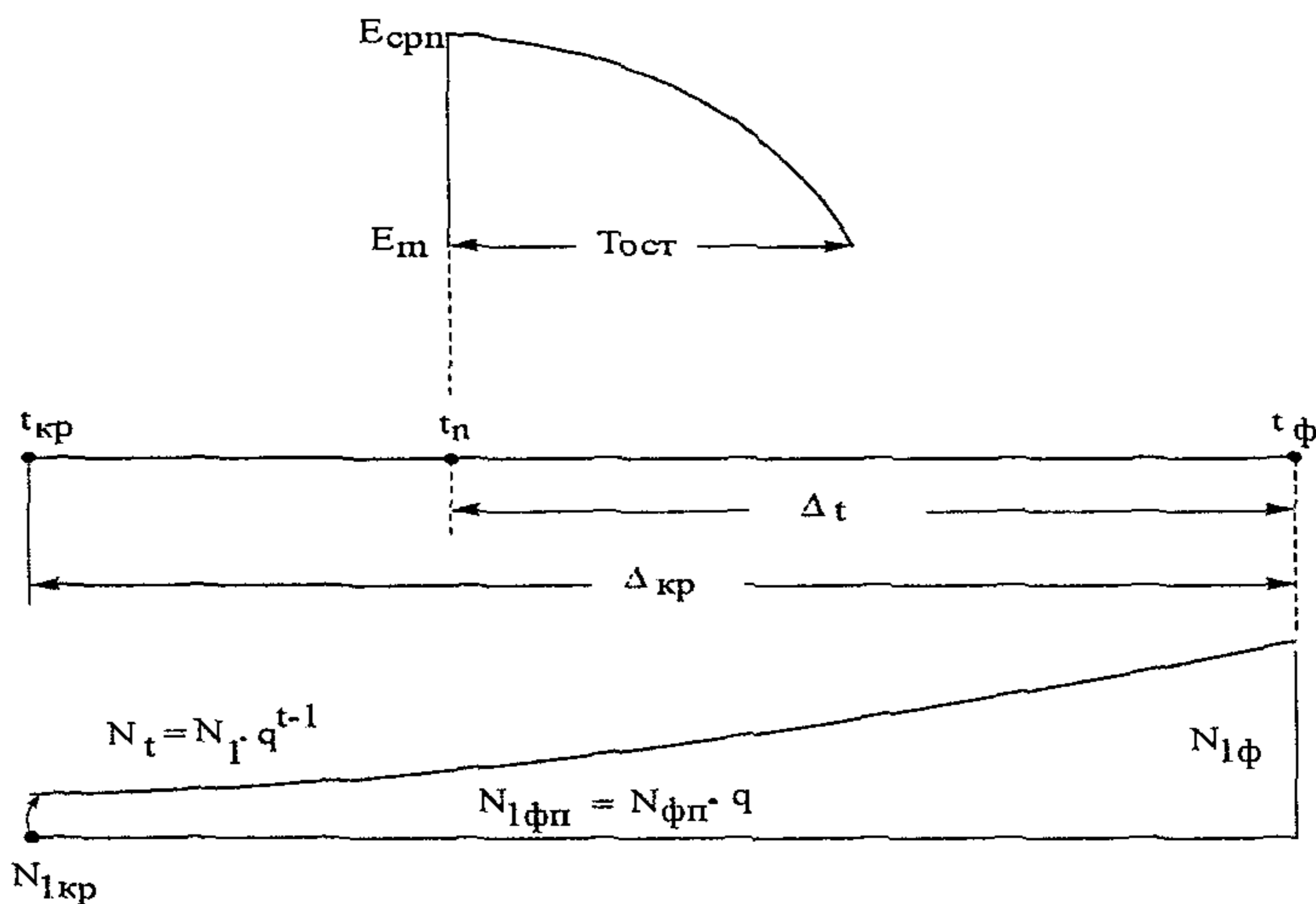
Рис. 1. Расчетная схема для прогнозирования коэффициента прочности
