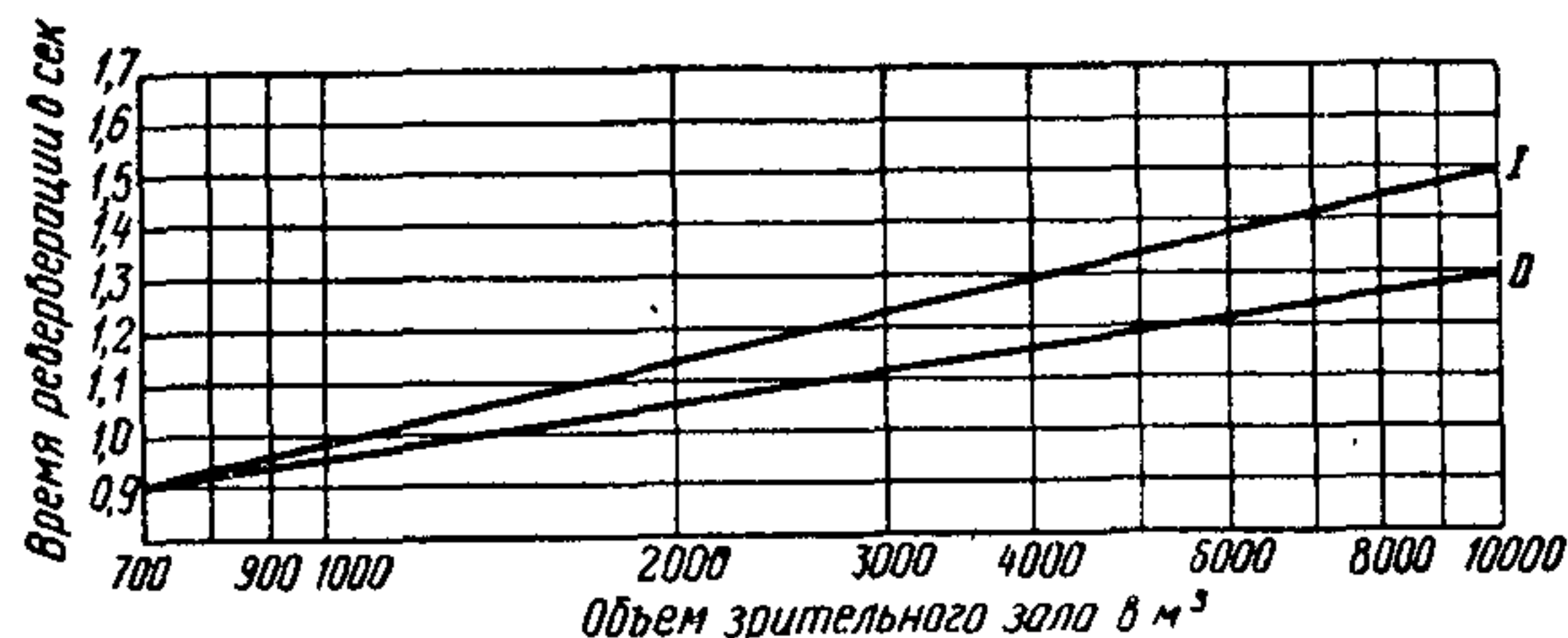
Рис. 4. График времени реверберации
