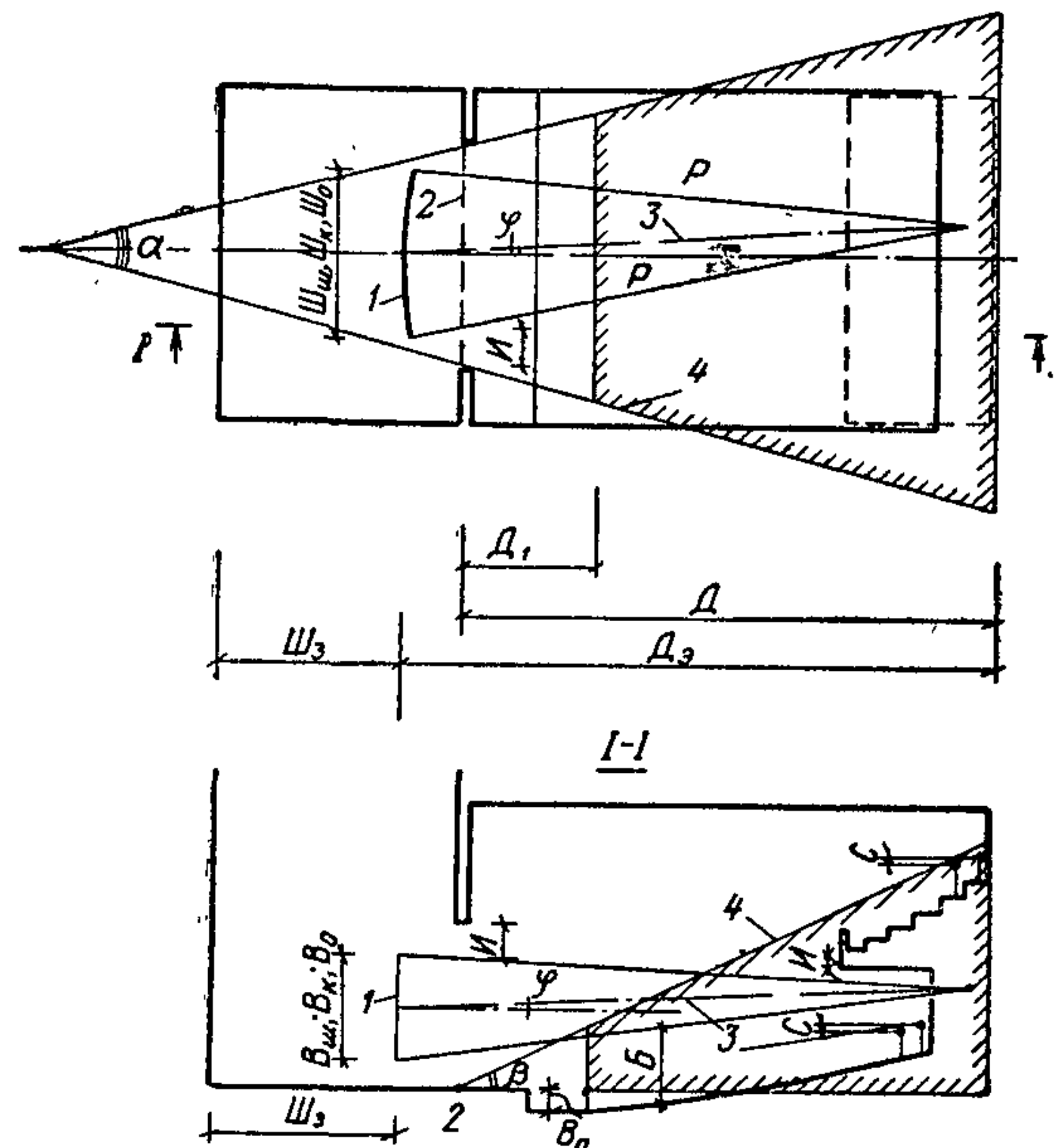
Рис. 1. Размещение зрительских мест, расположение и размеры экрана
