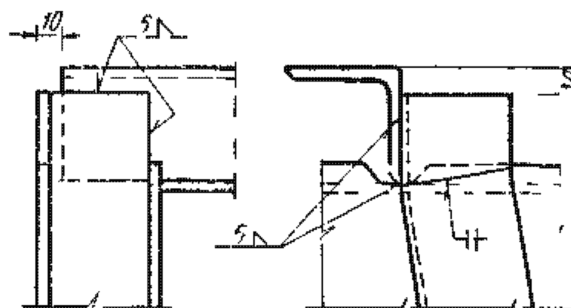
Ребра жесткости из угловой стали
