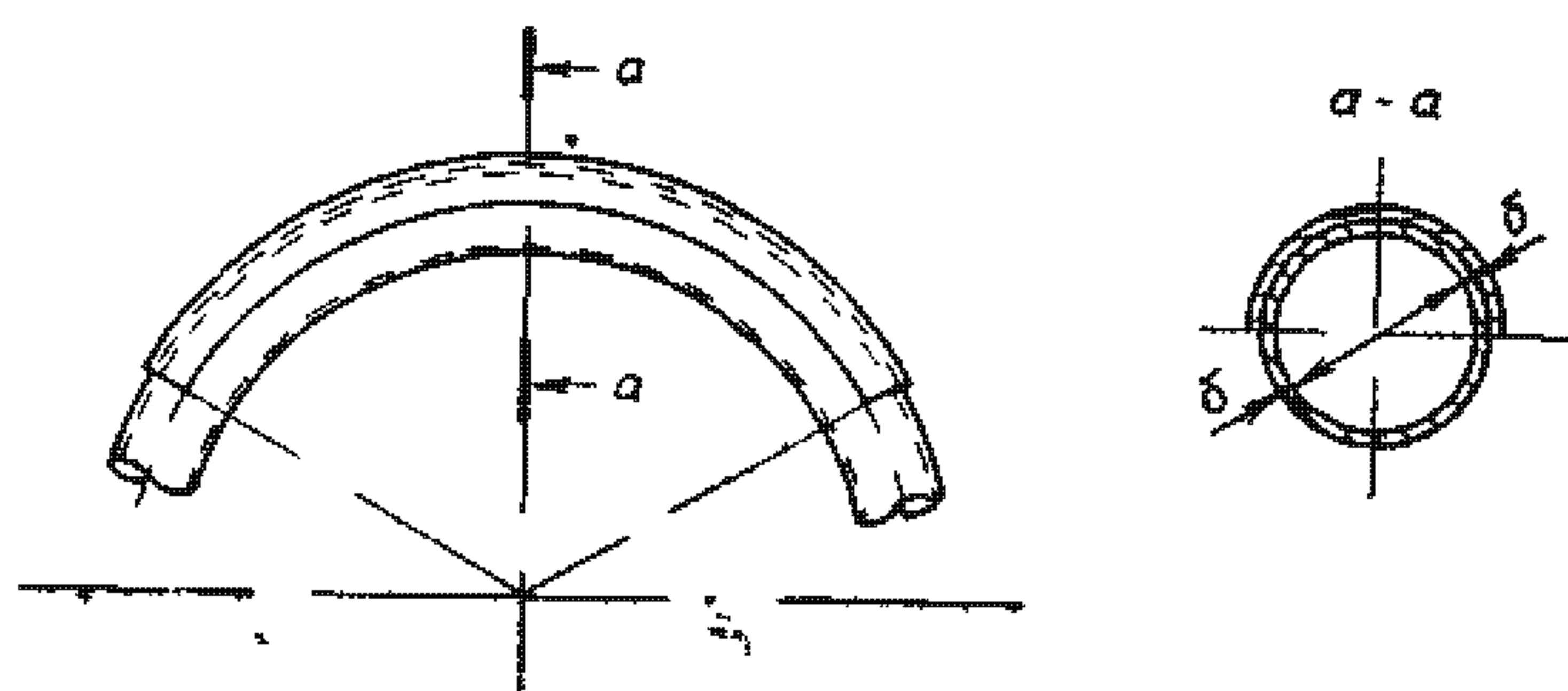
Рис.1. Расположение противоизносной накладки
