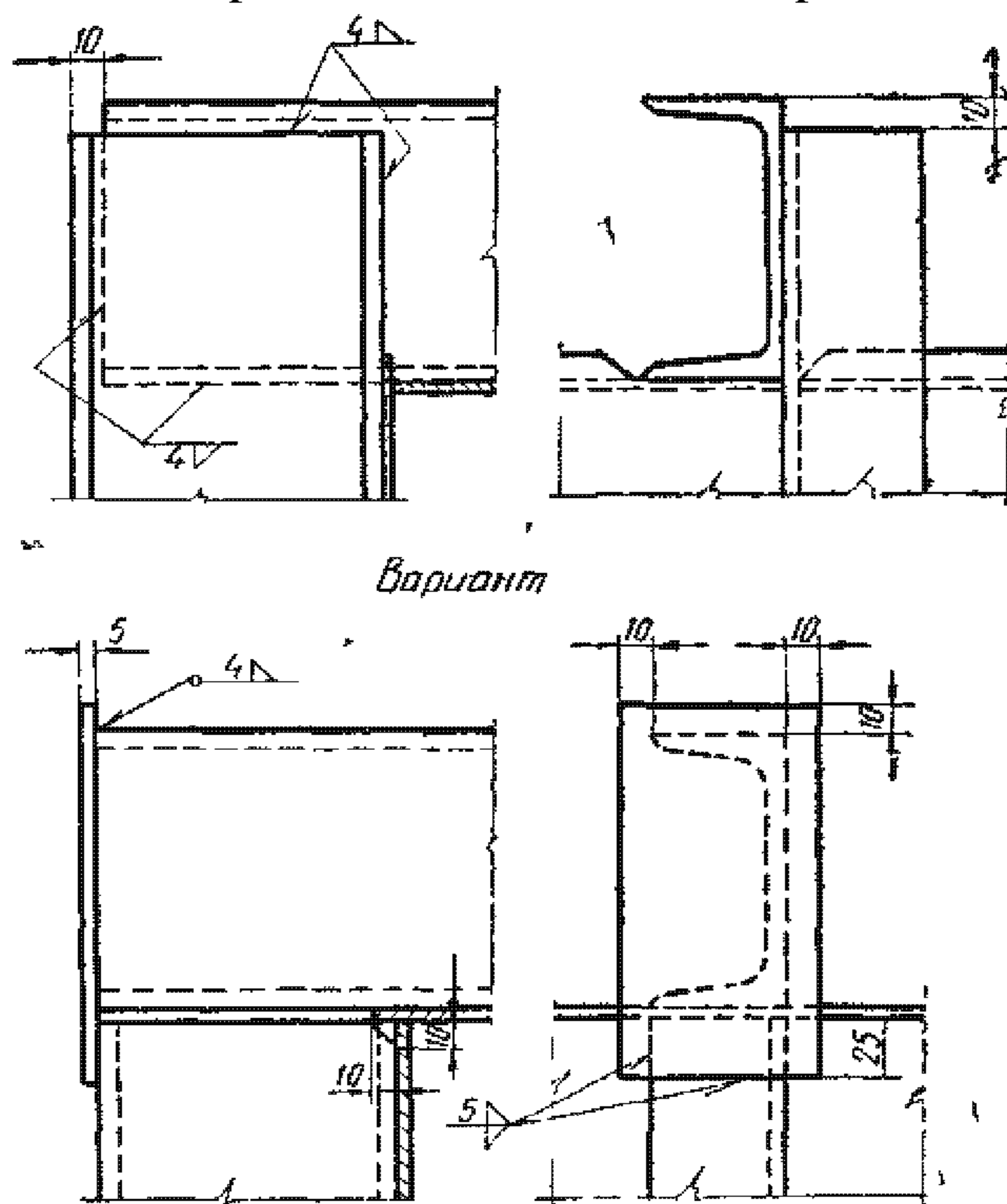
Ребра жесткости из швеллеров
