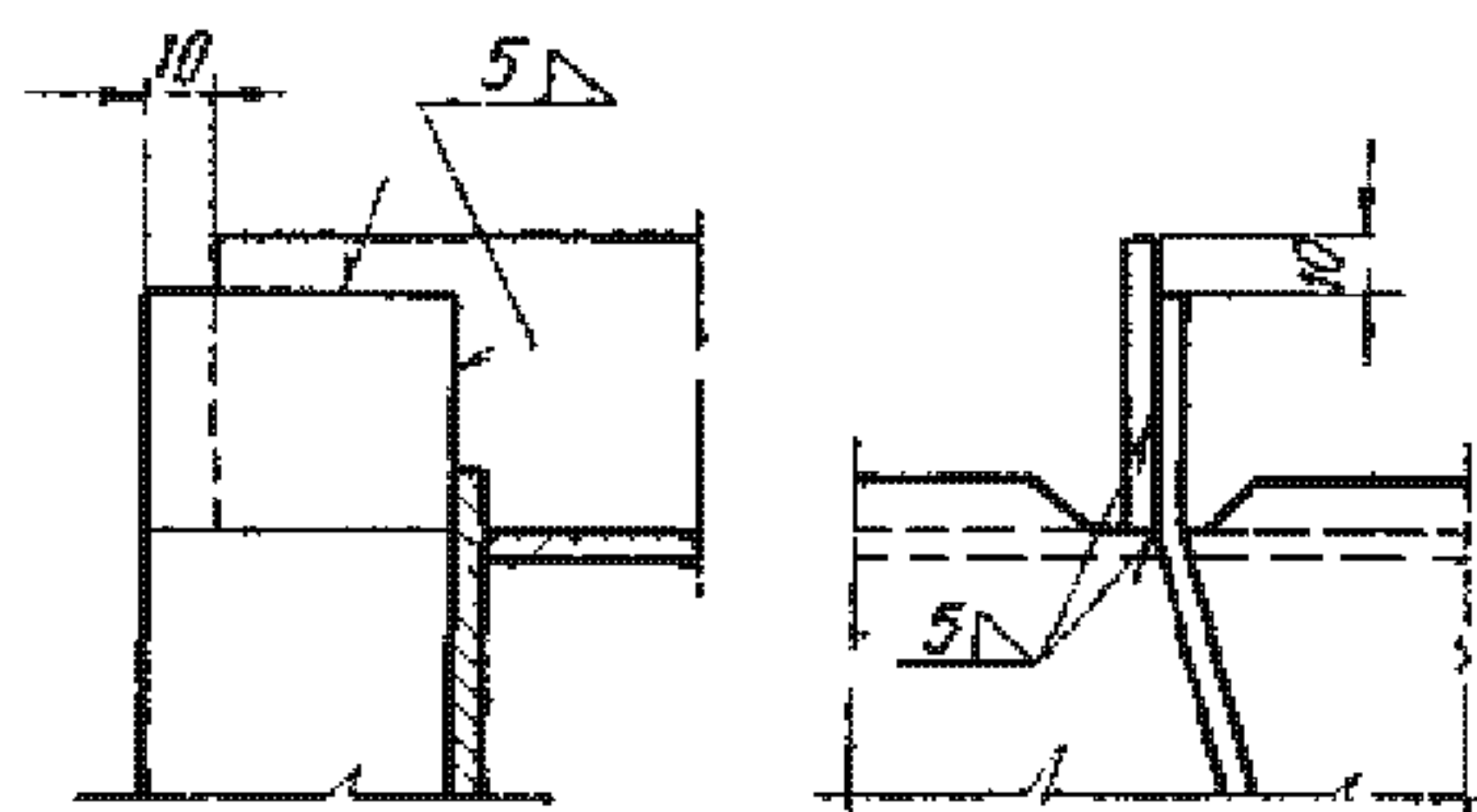
Ребра жесткости из угловой стали
