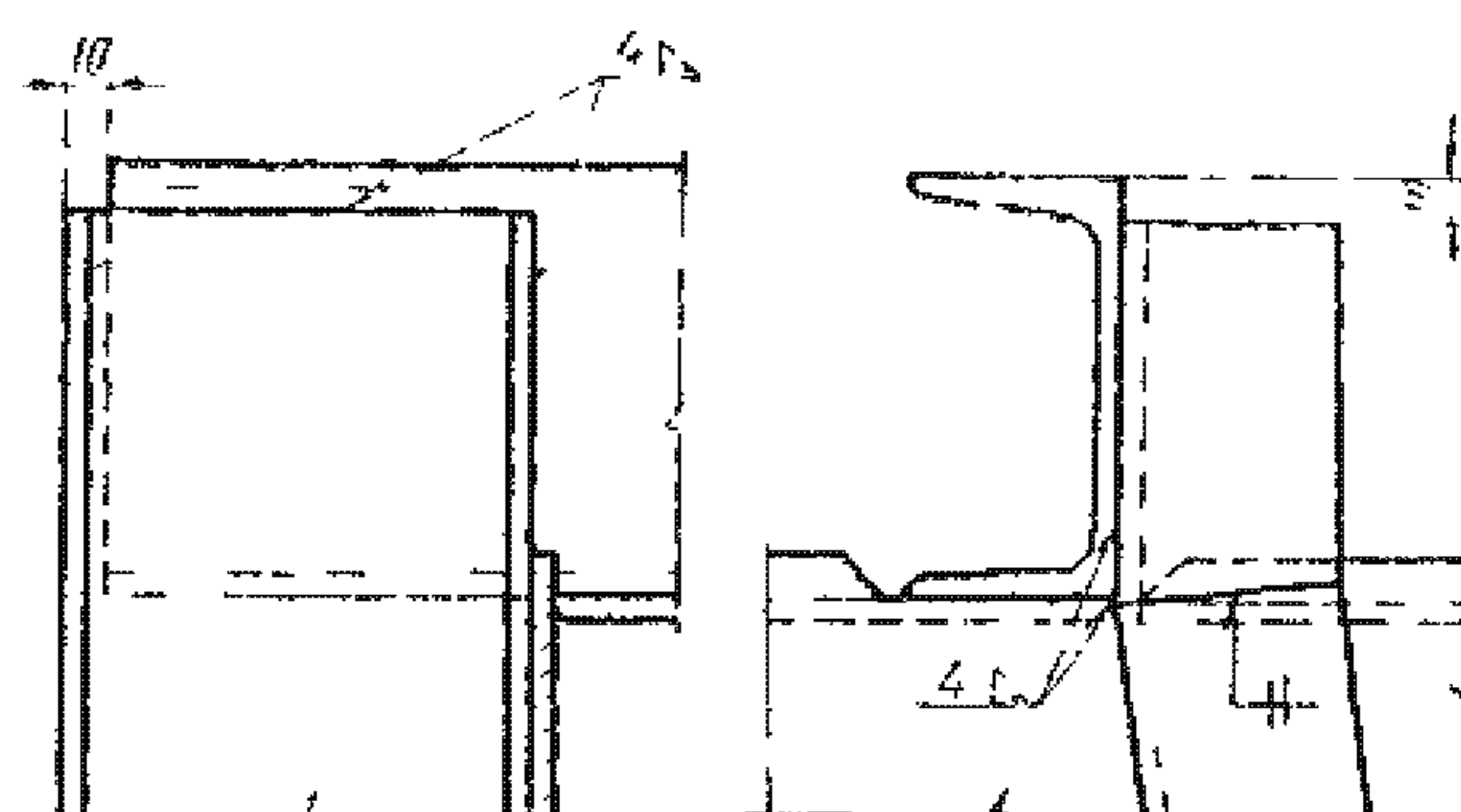
Ребра жесткости из швеллеров
