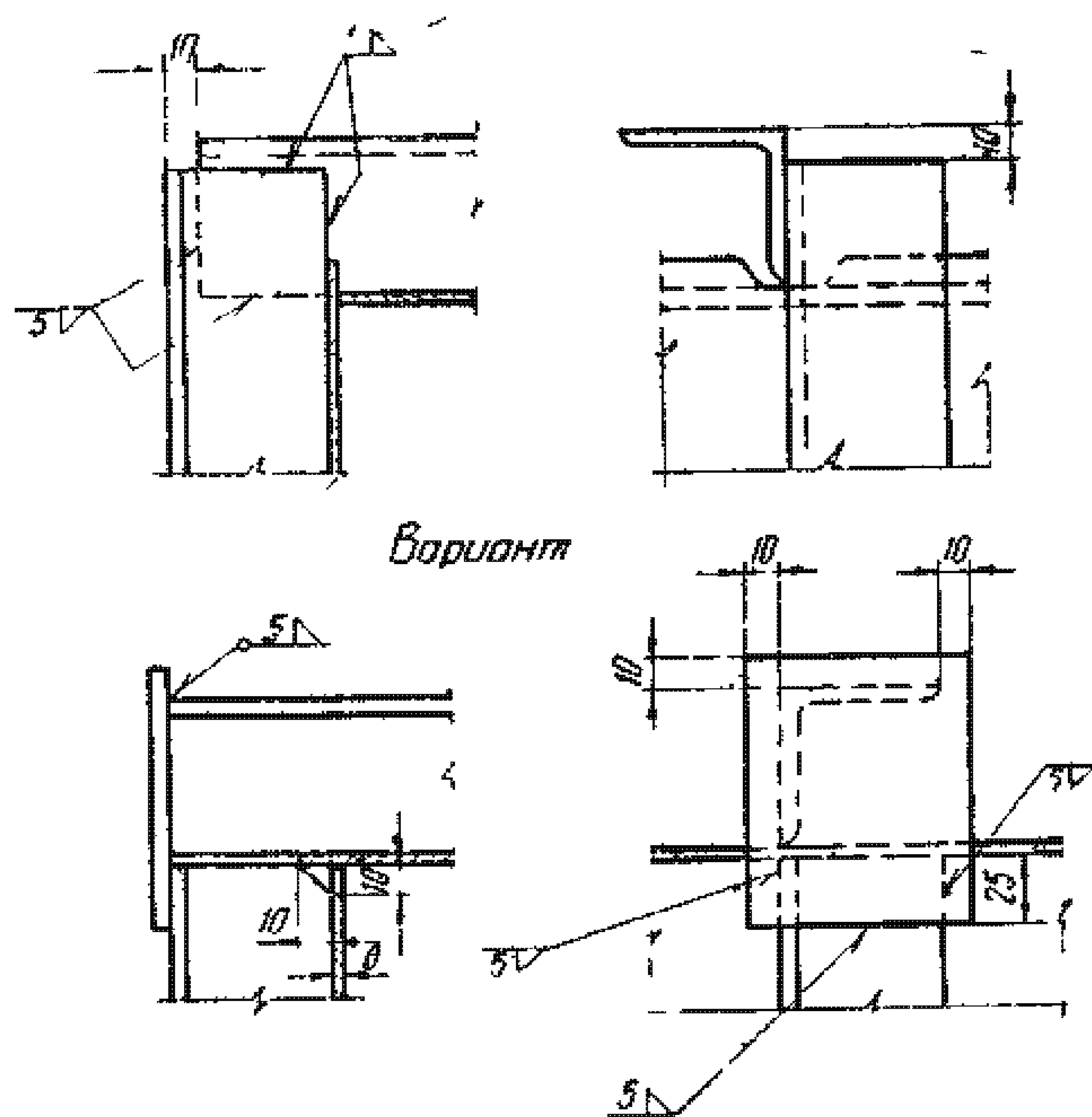
Ребра жесткости из швеллеров
