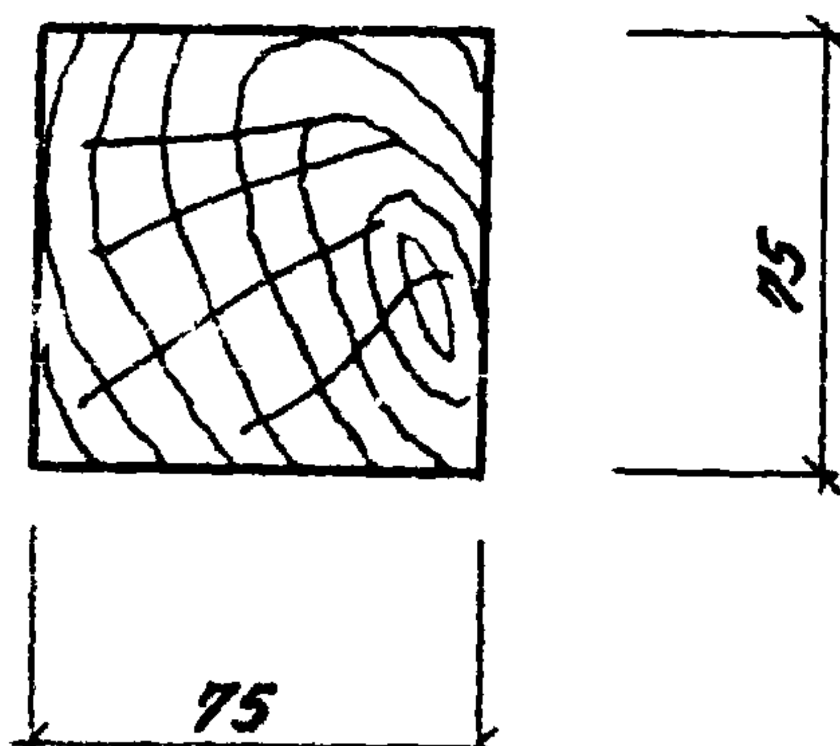
A-A M 1:2
