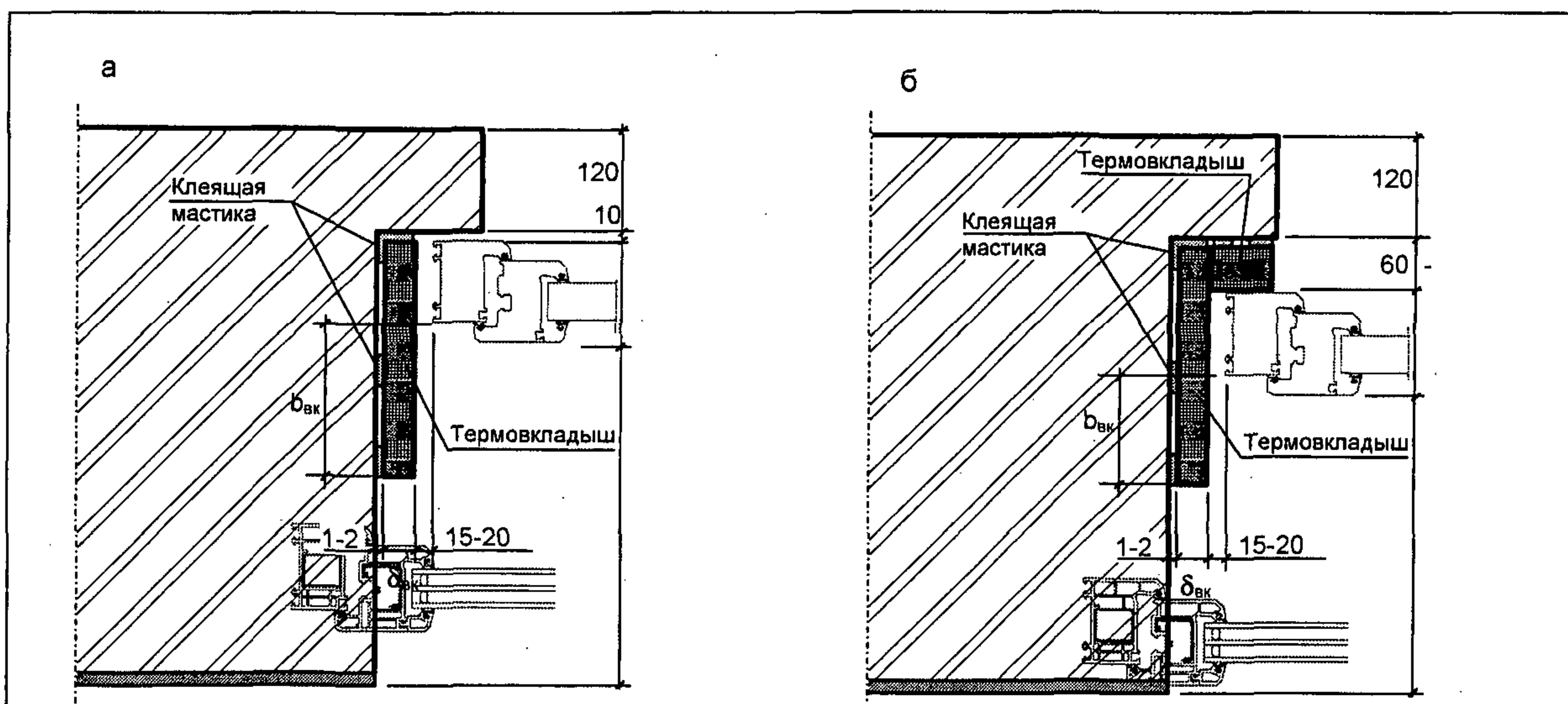
Рис.7.5. Примеры расположения утепляющих вкладышей в монтажных зазорах: а – при расположении оконного блока у оконной четверти; б – при смещении оконного блока от четверти стены
