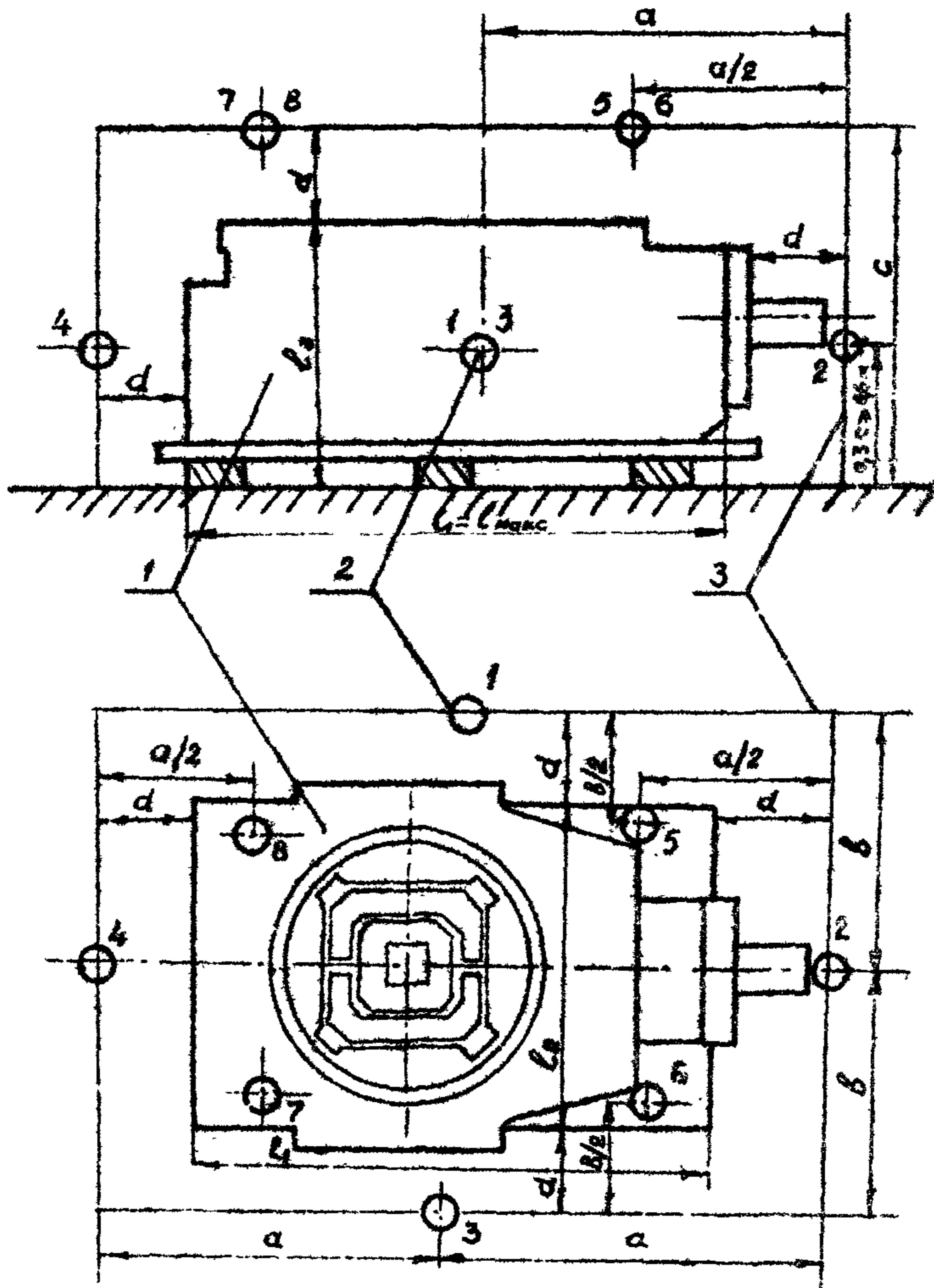
Рис. I. I. Расположение измерительных точек 1 - ротор, 2 - измерительные точки, 3 - измерительная поверхность.
