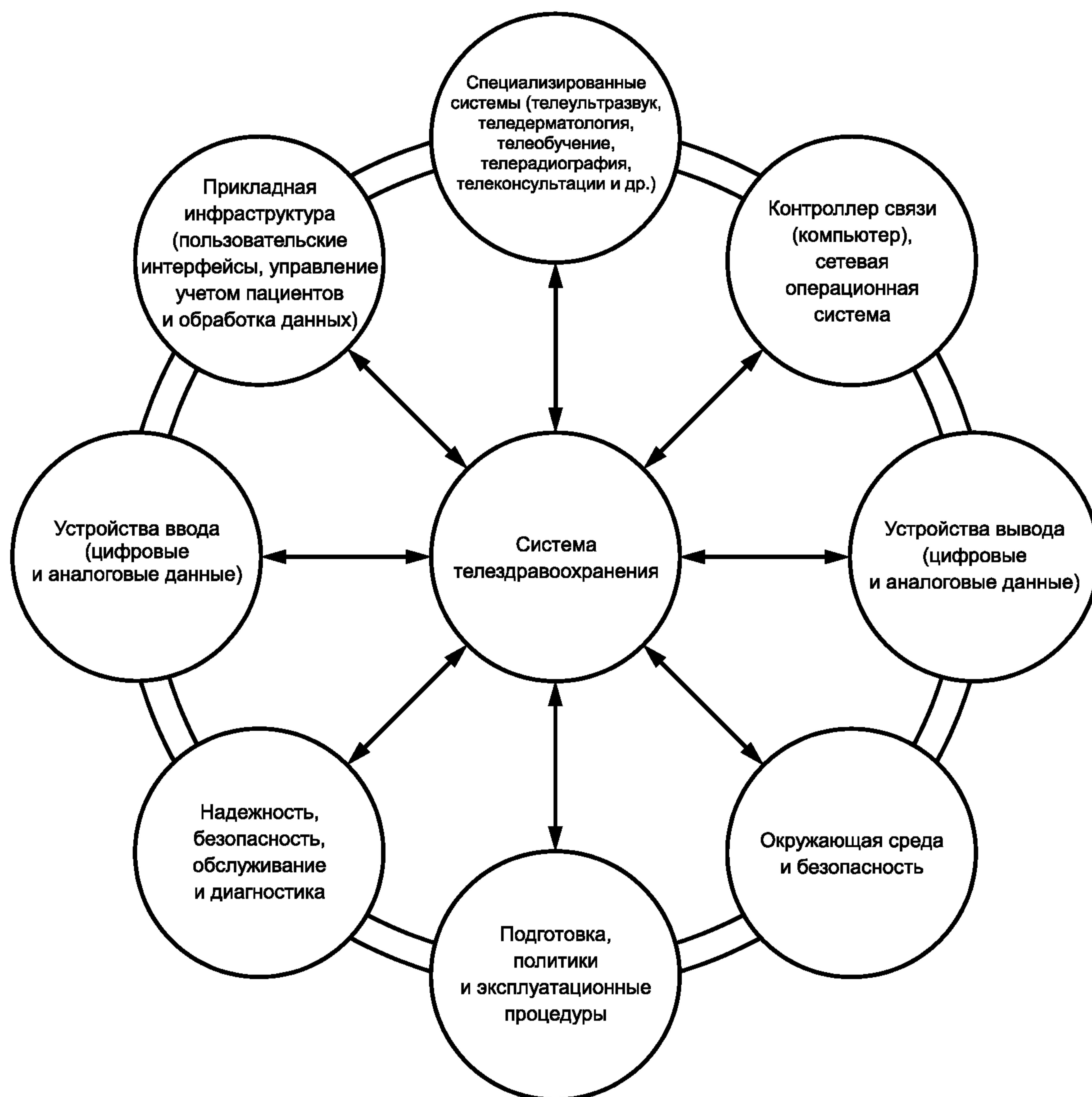
Рисунок А.1 — Техническая эталонная архитектура системы телездравоохранения
