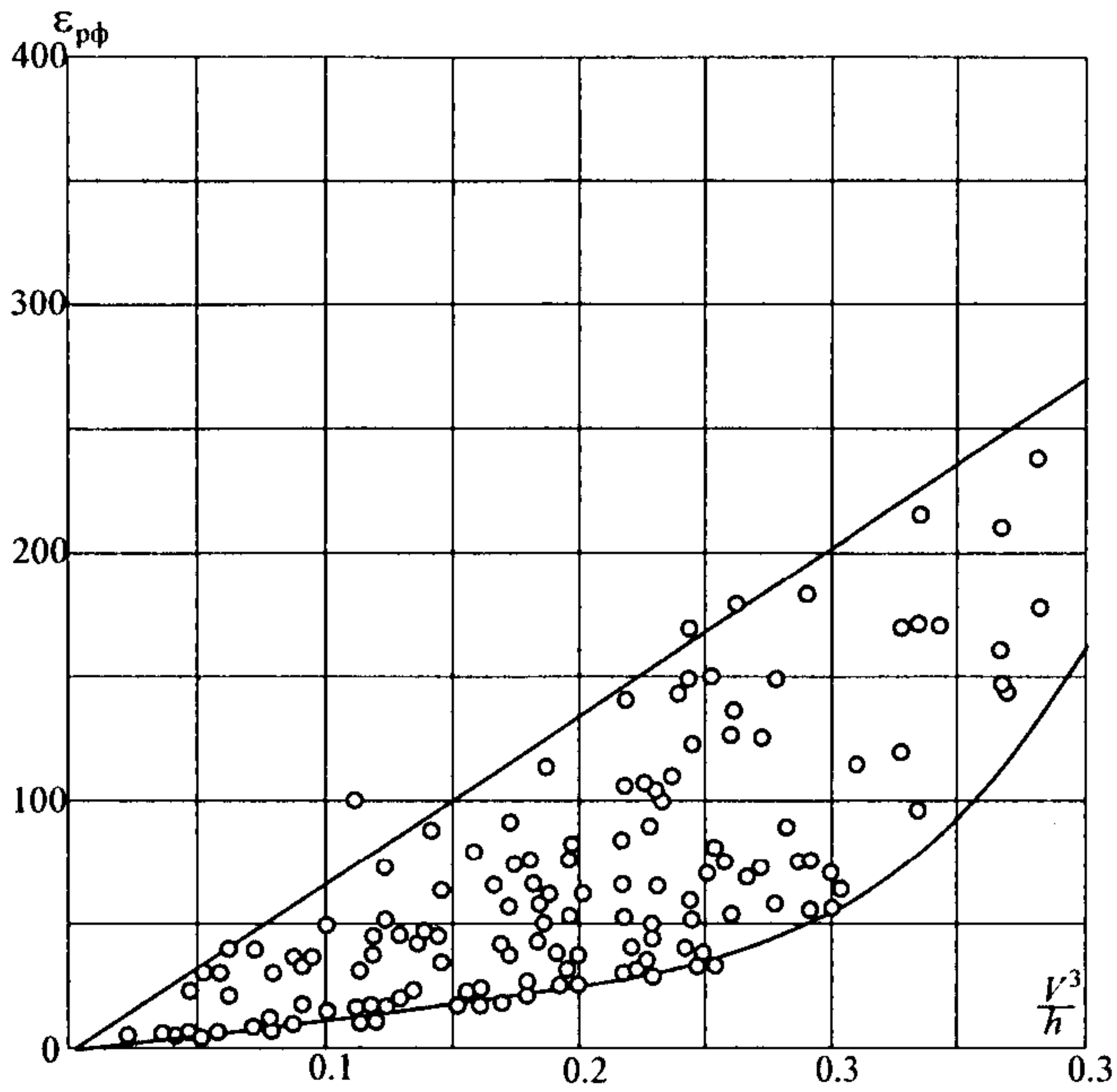
Рис. П2.1. Зависимость \epsilon_{\rho\phi} = f(V^3/h)
