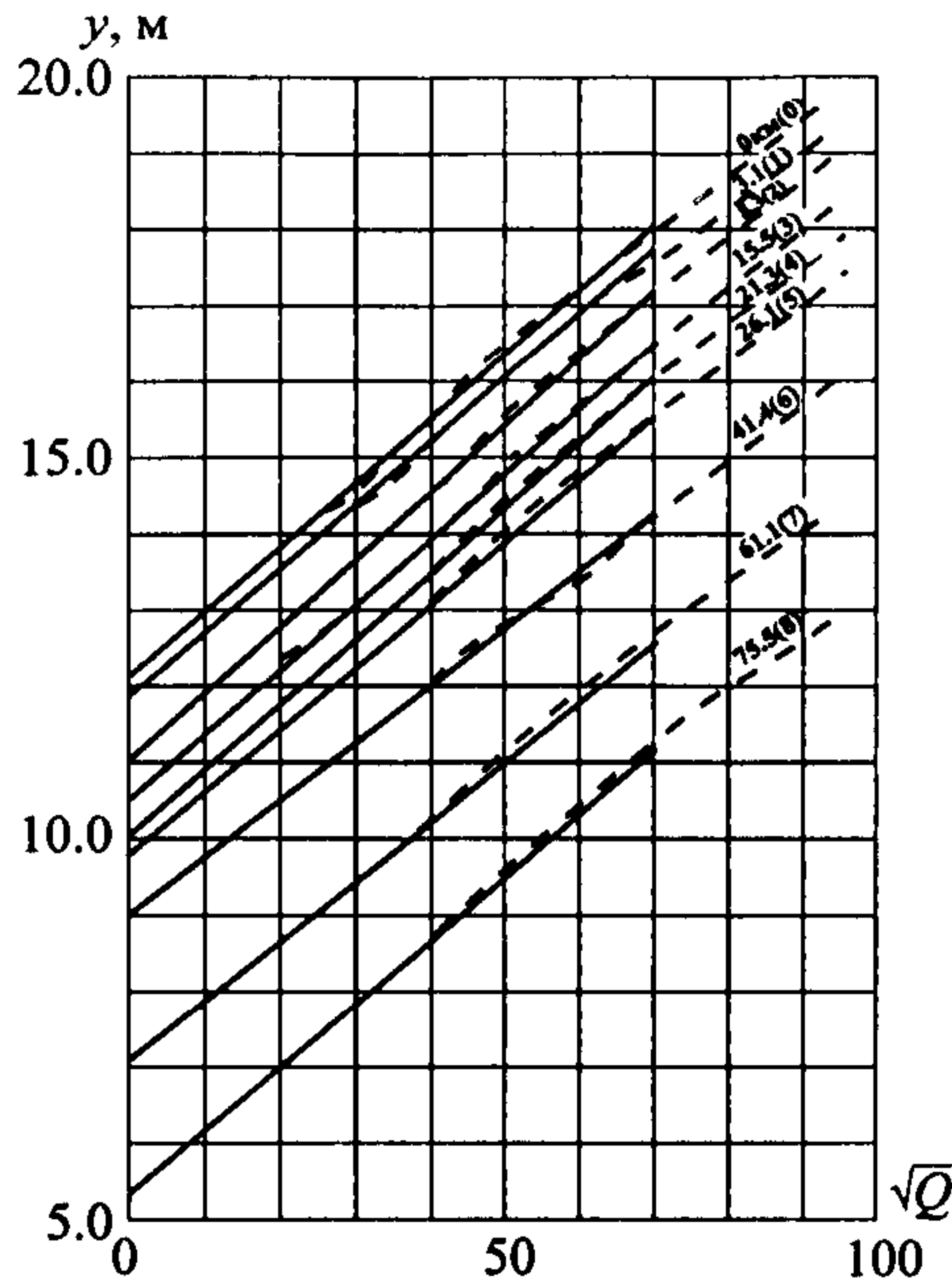
Рис. П1.3. Аппроксимация кривых Q = f(H) прямыми \sqrt{Q} = \sqrt{k}(y - y_0) в расчетных створах: числа на кривых указывают расстояние от створа ГЭС в км и номер расчетного створа; — — — кривые расходов в различных створах; ————— линейная аппроксимация
