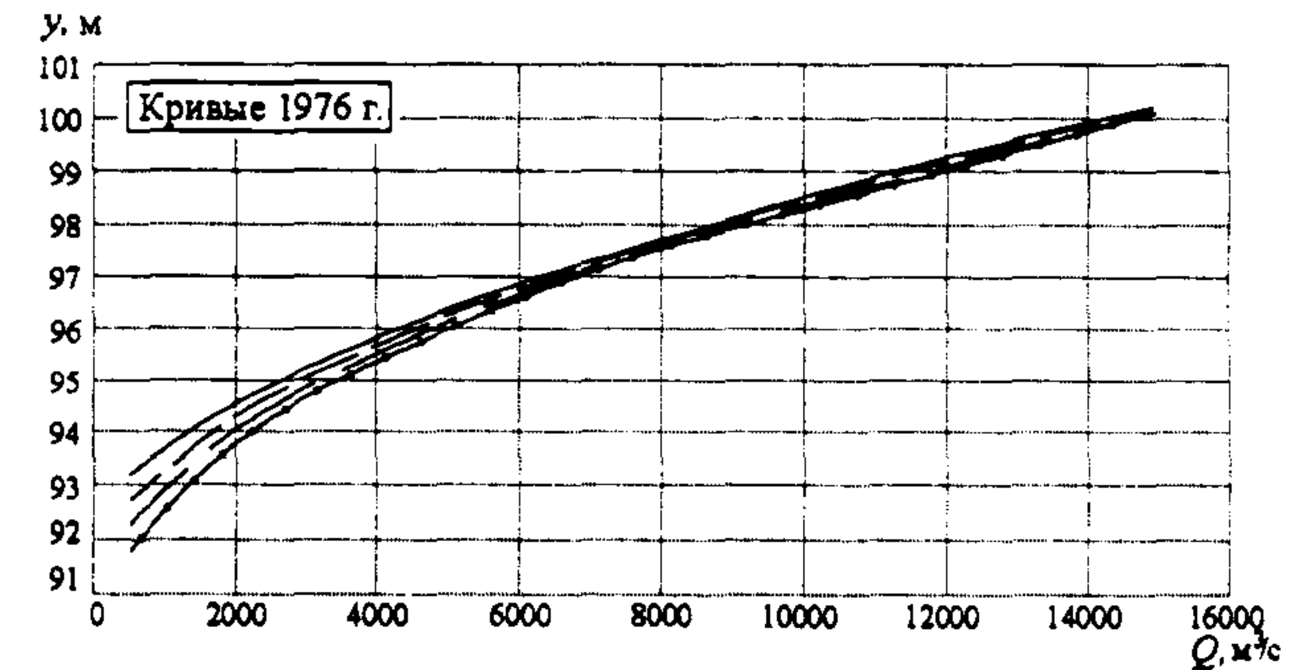
Рис.П4.4. Кривые связи расходов и уровней Q = f(y) и изменение уровней u в створе 15 при различных расходах притока Q_n на участке 18: а – пример 1; б – пример 2
