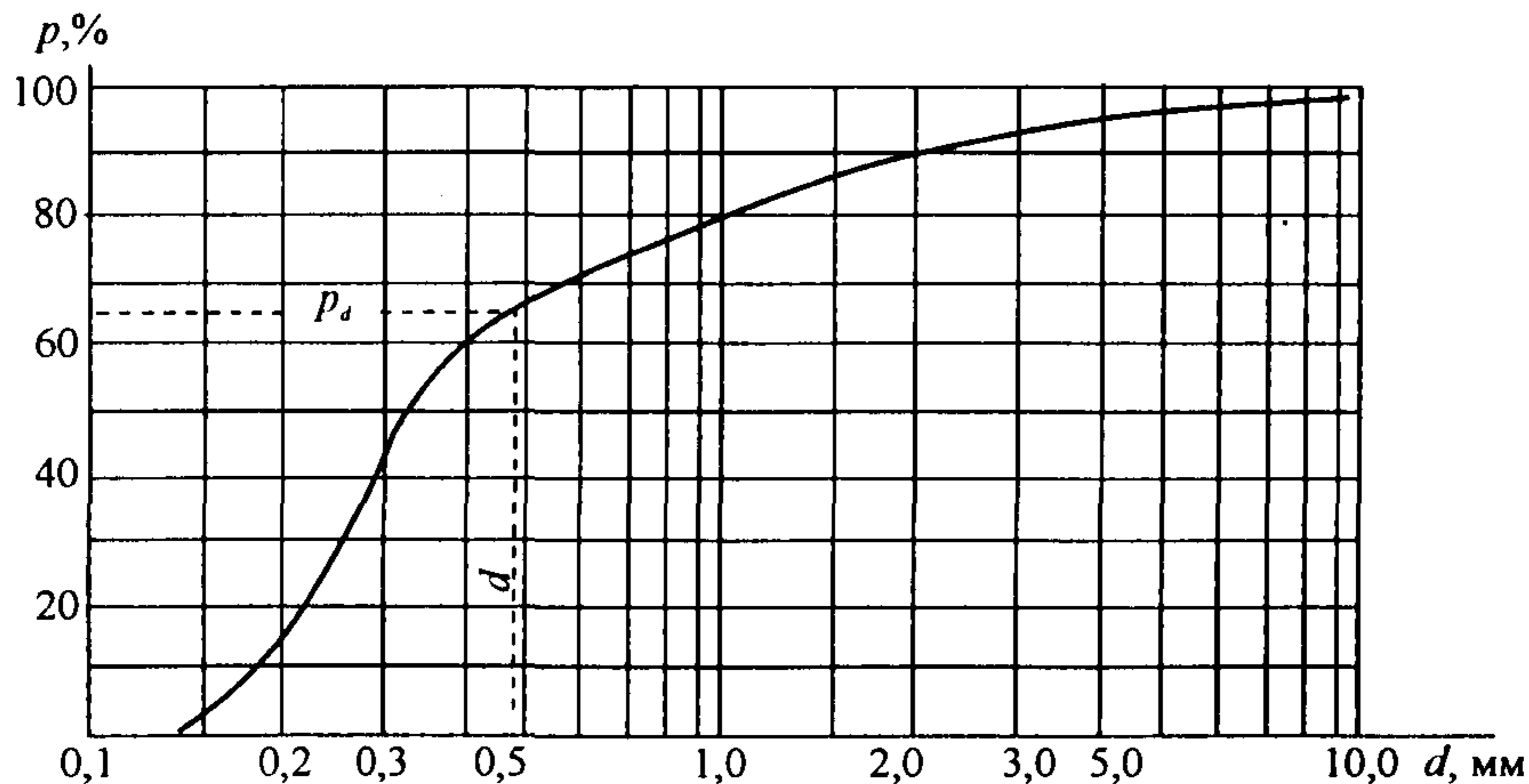
Рис. 1. Кривая гранулометрического состава наносов
