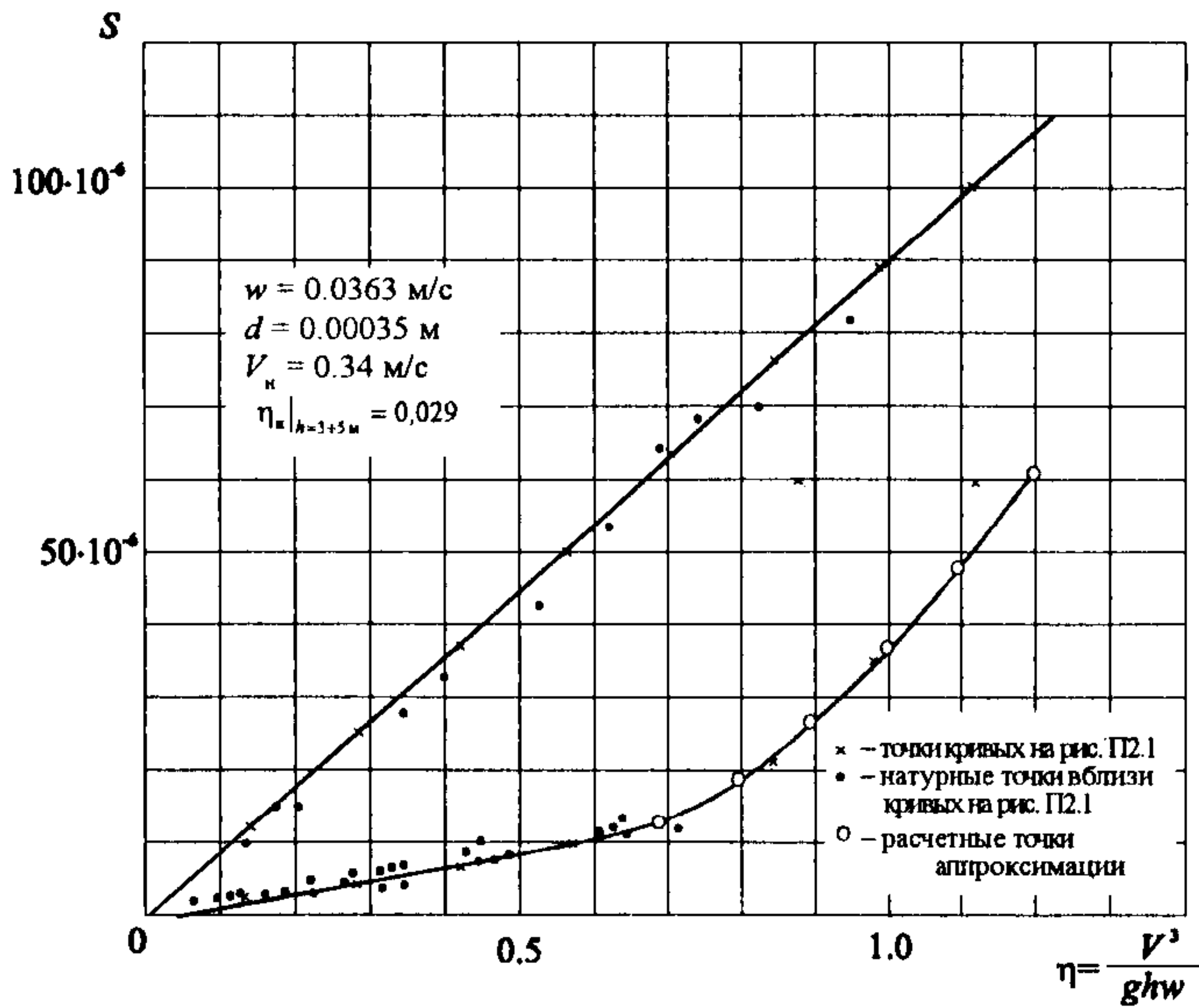
Рис. П2.2. Зависимость S = f(\eta)
