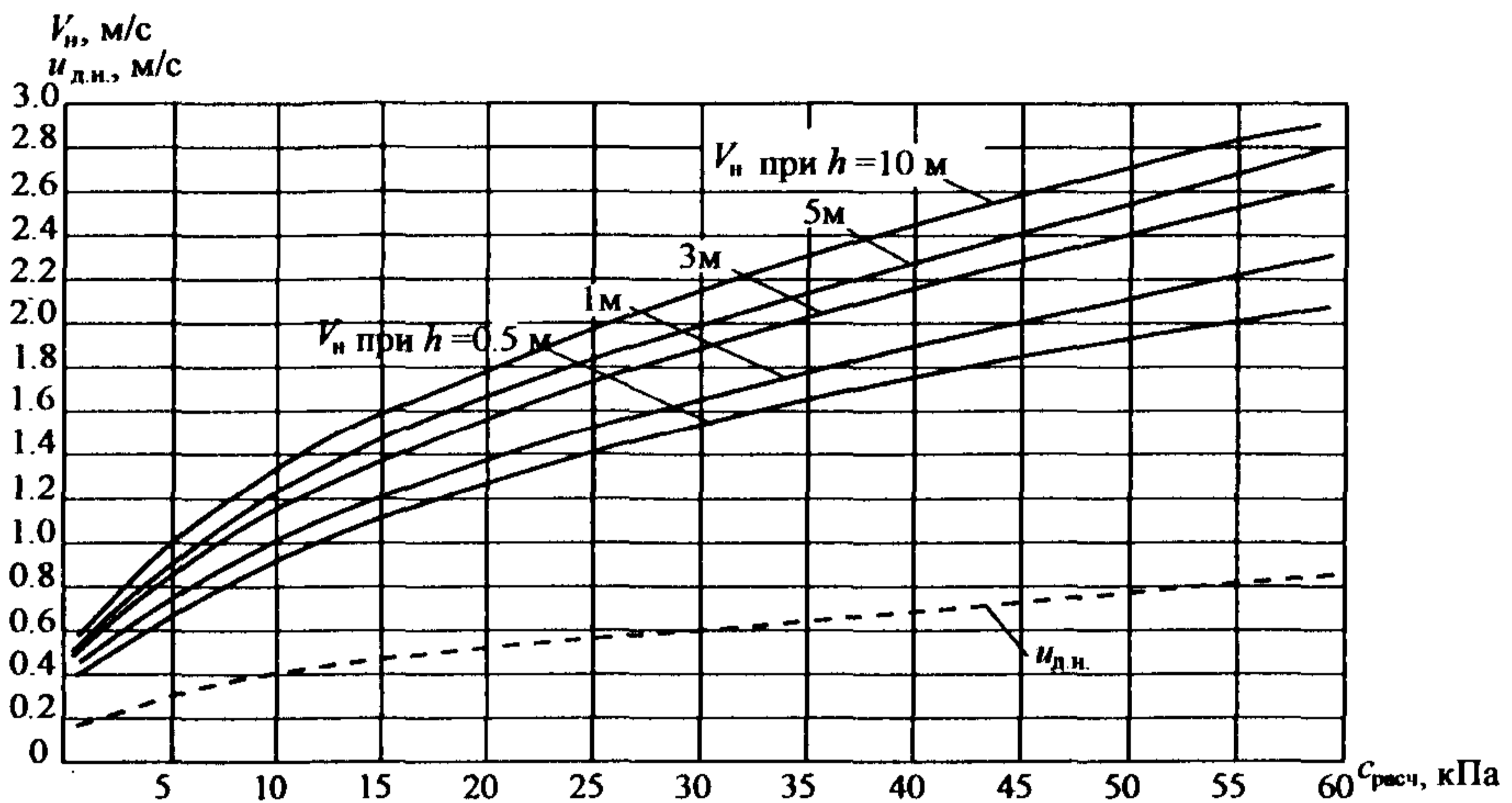
Рис. 6. Зависимость неразмывающих скоростей V_n связных грунтов от расчетного значения сцепления c_{расч.} = c_n / K_c при плотности \rho_s = 2650 \text{ кг/м}^3 и коэффициенте m_m = 1
