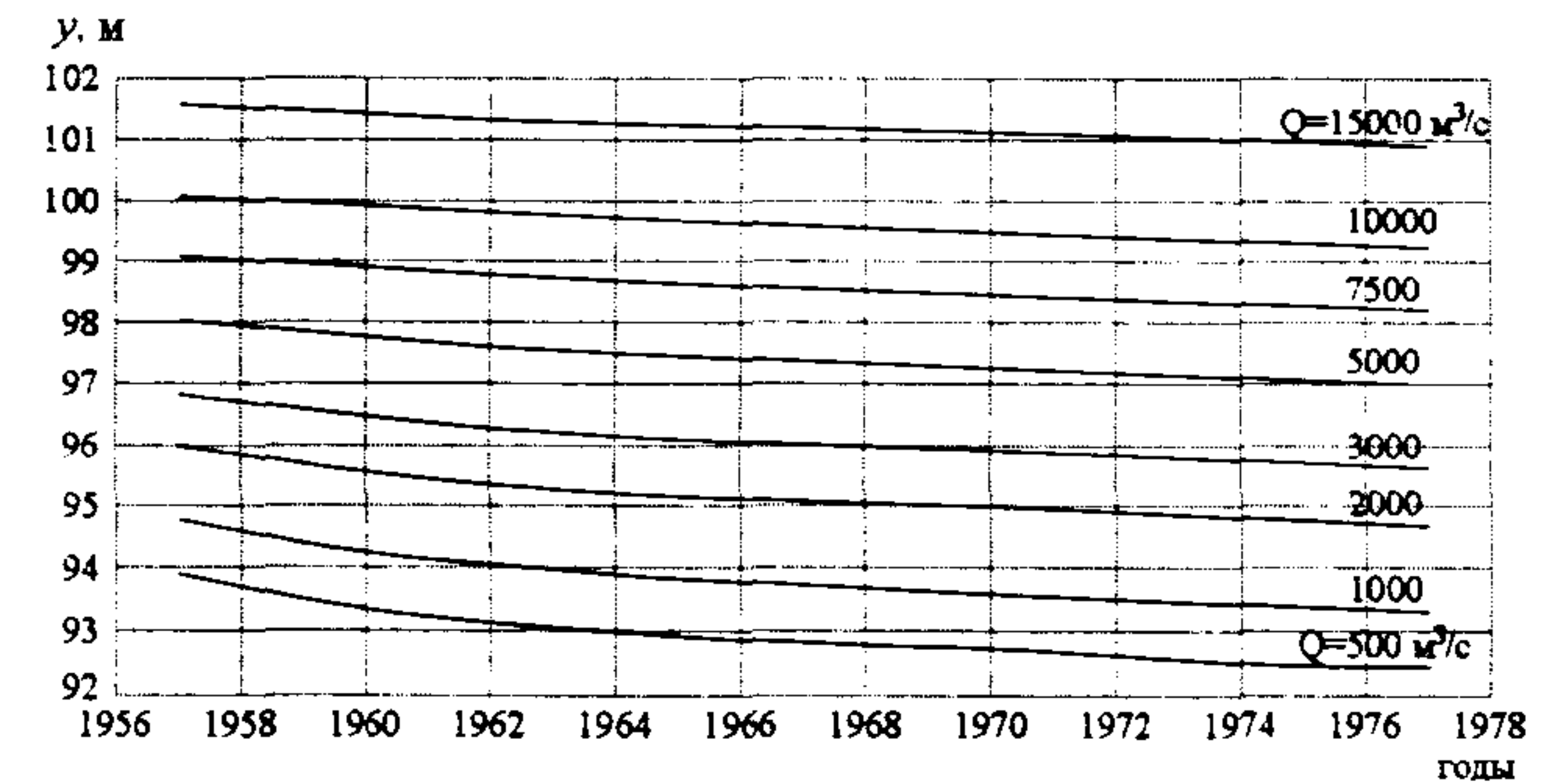
Рис.П4.2. Кривые связи расходов и уровней Q = f(y) и изменение уровней y в створе 1 при различных расходах Q : а – пример 1; б – пример 2
