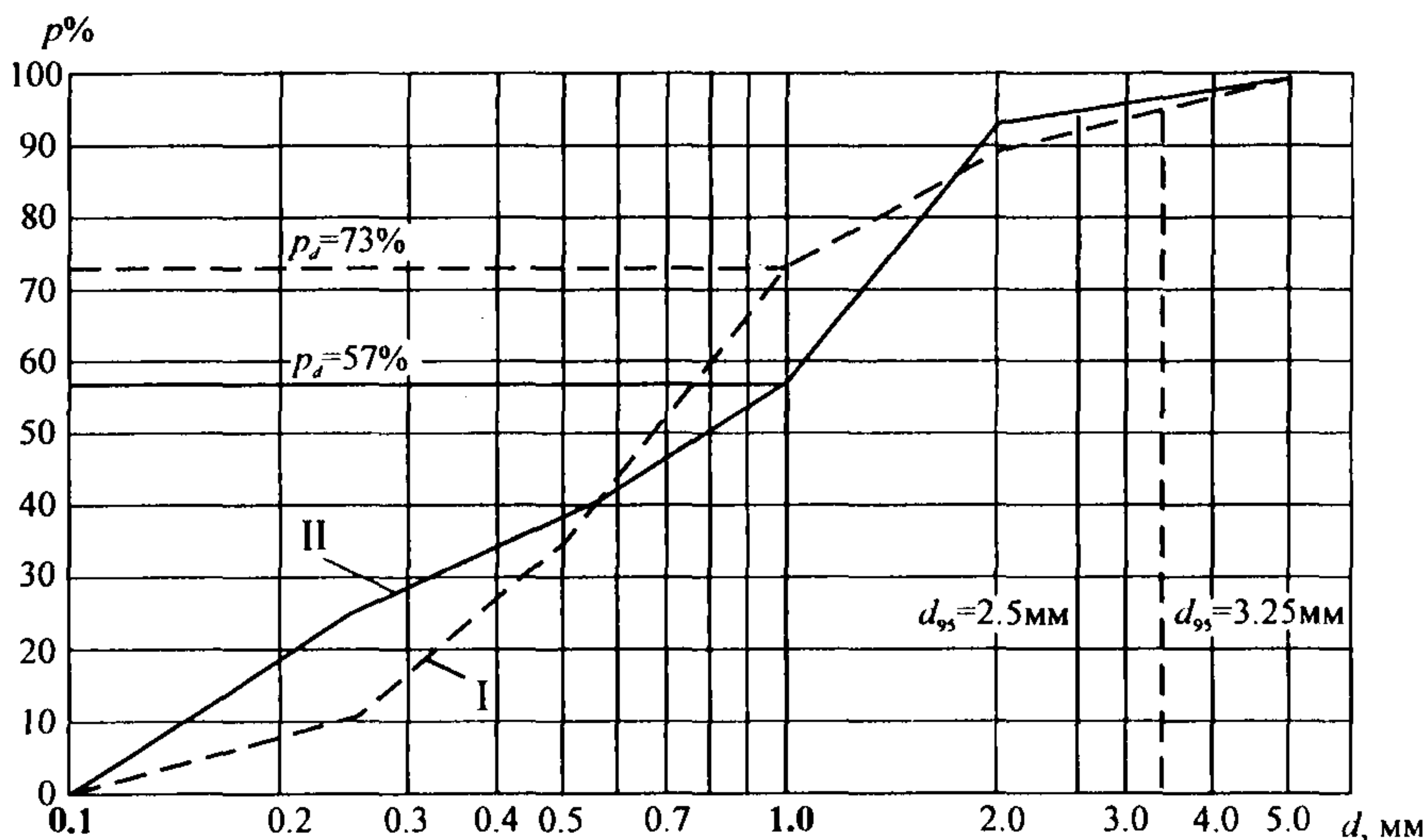
Рис. П5.1. Кривые гранулометрического состава разнозернистого грунта: I, II – номера составов по табл. П5.2
