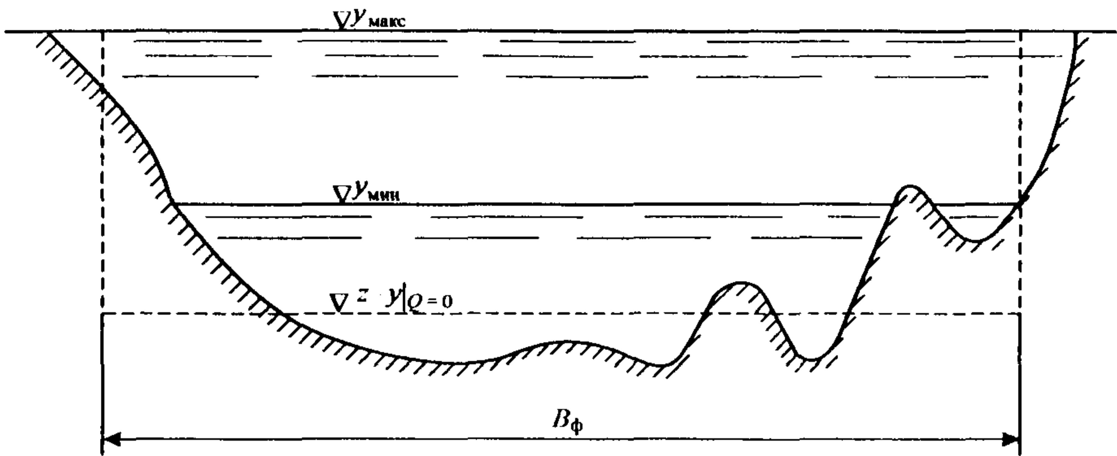
Рис.8. Схематизация живого сечения потока
