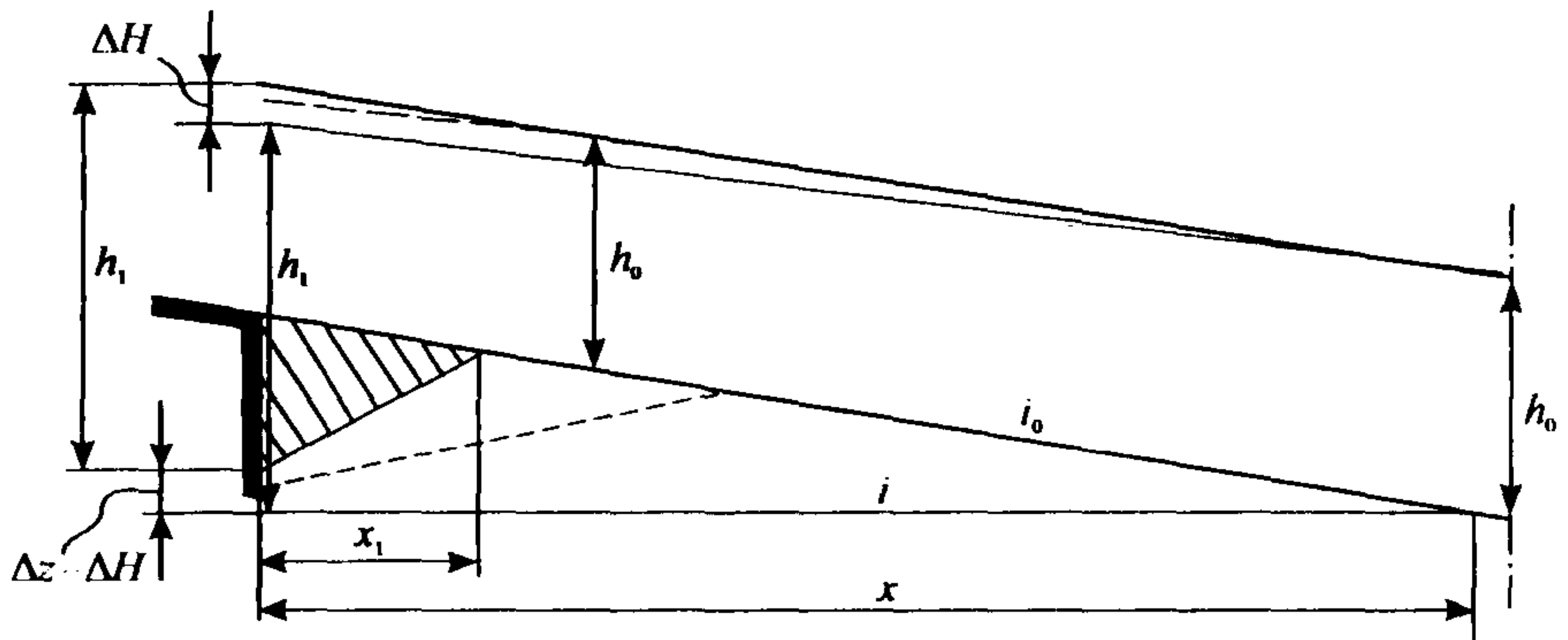
Рис.13. Схема расчета общего размыва по приближенному методу
