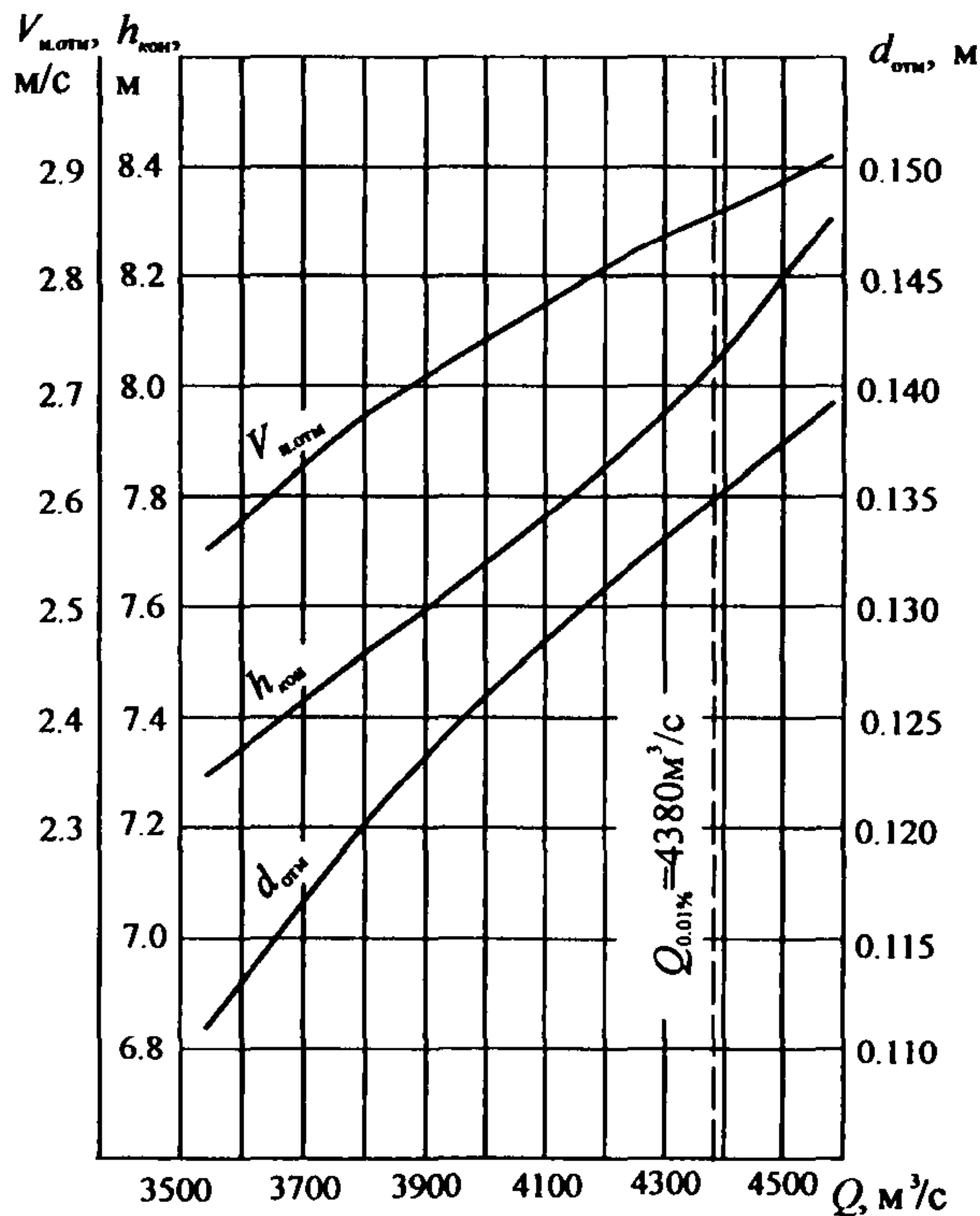
Рис. ПЗ.2. Графики для нахождения параметров самоотмоности русла
