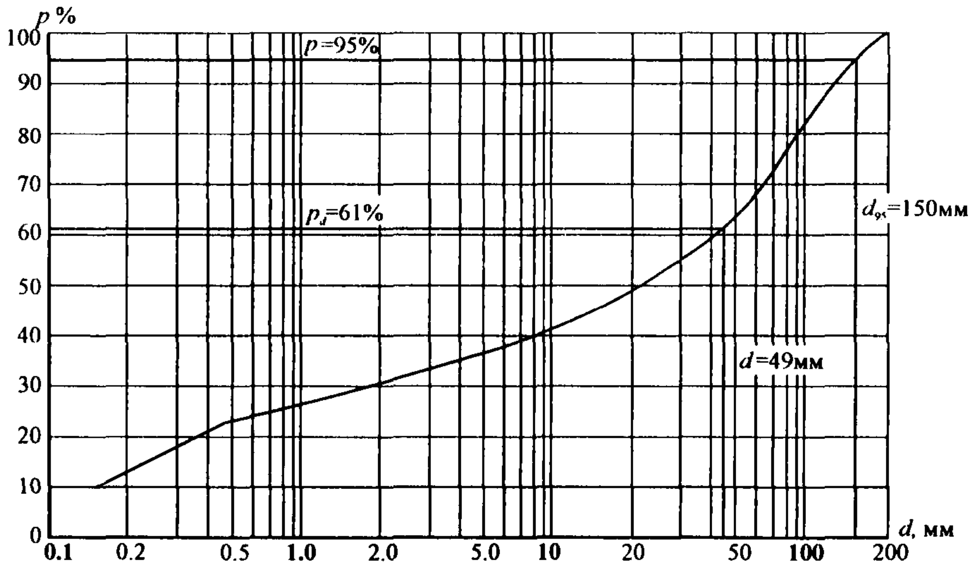
Рис. ПЗ.1. Кривая гранулометрического состава наносов
