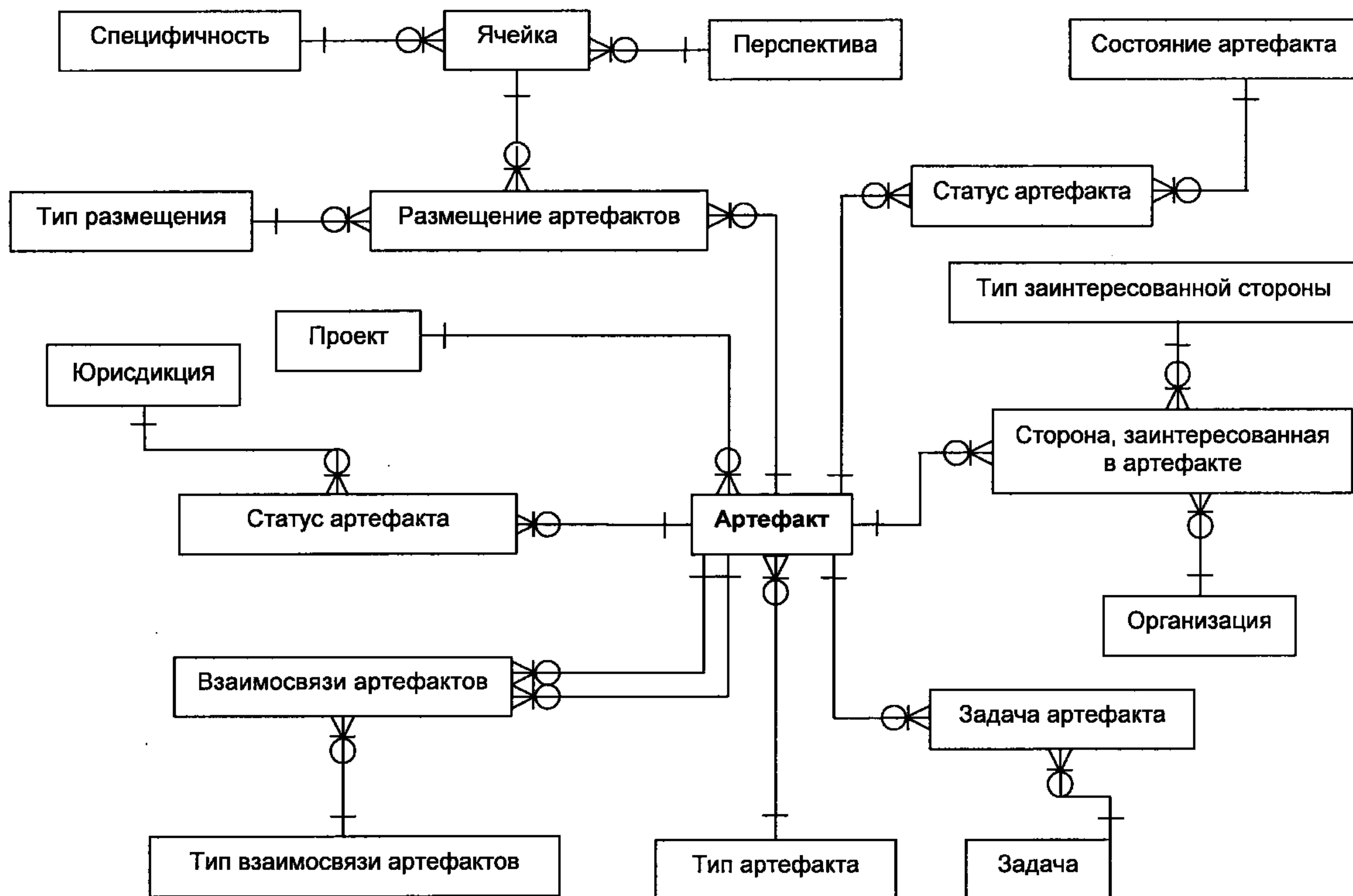
Рисунок В.1 — Диаграмма метамодели СПРИЗ
