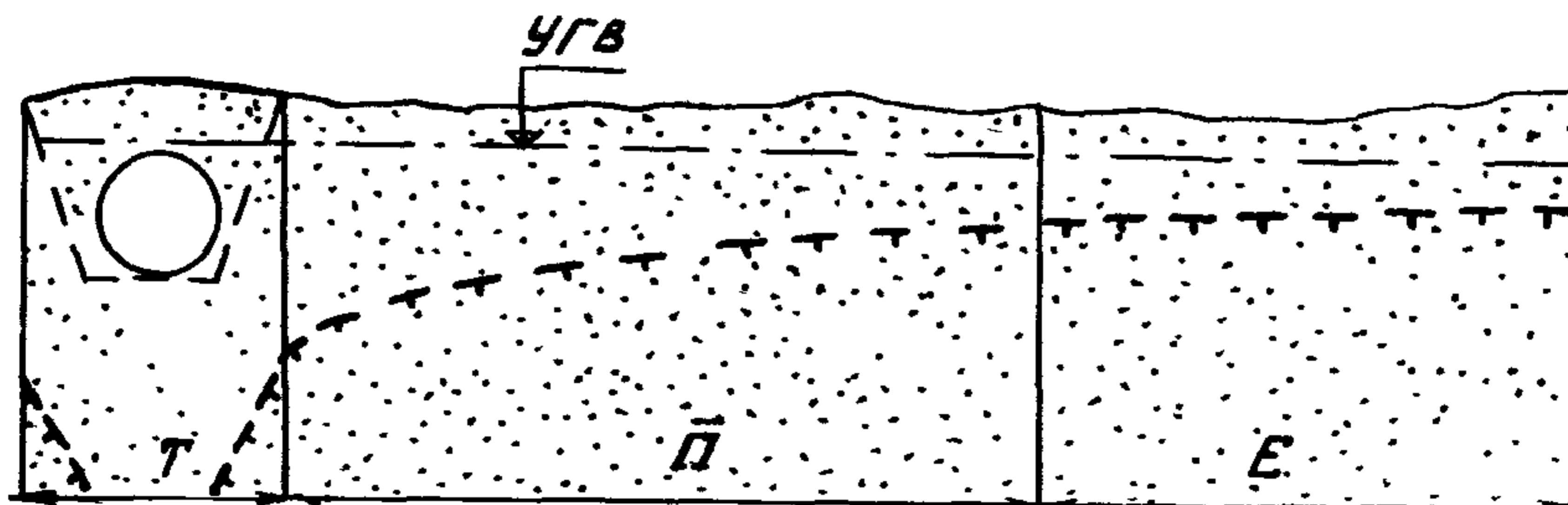
Рис.6. Зоны режима грунтовых вод по трассе трубопровода:
