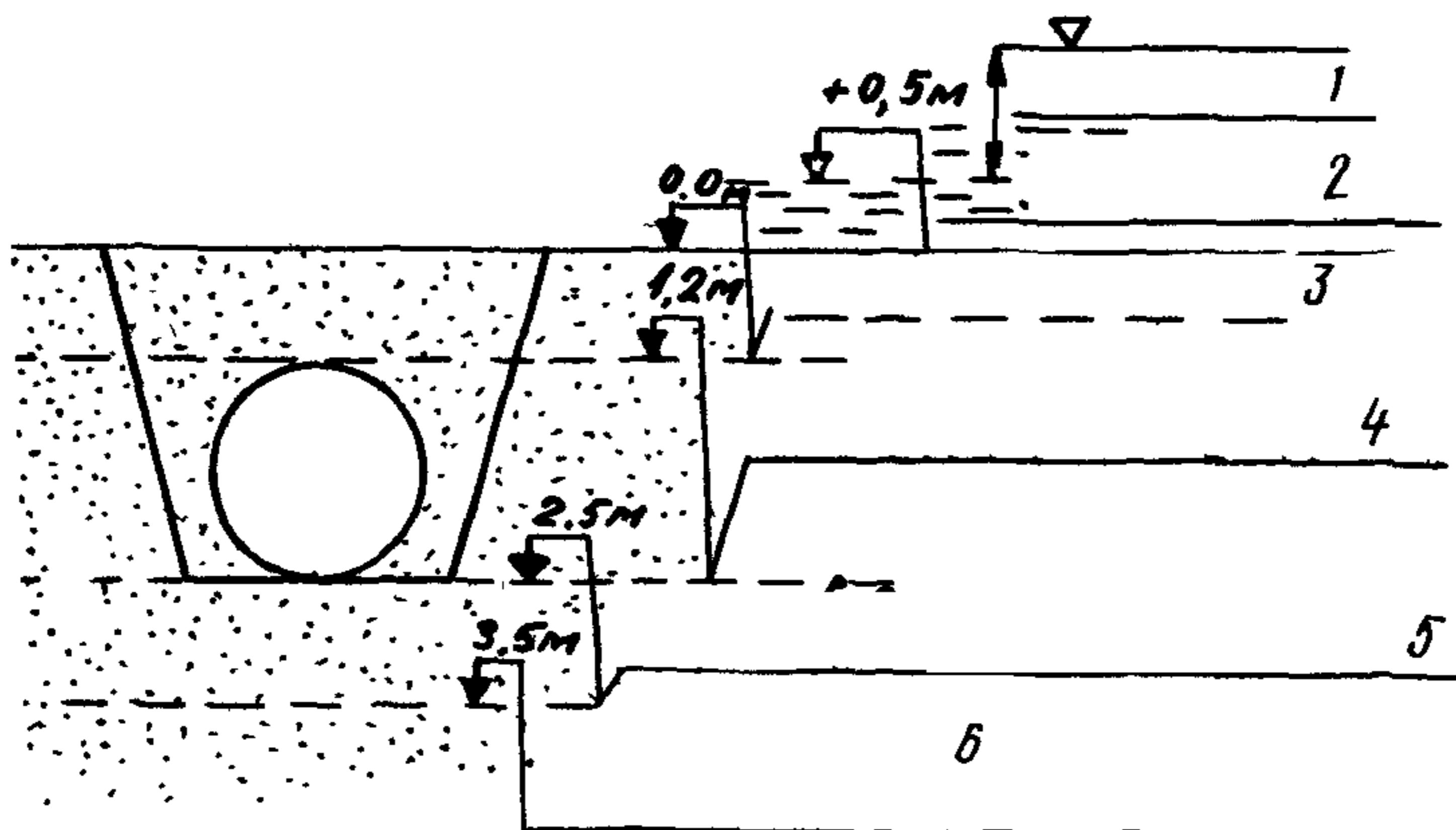
Рис.4. Типы участков по степени обводнения :
