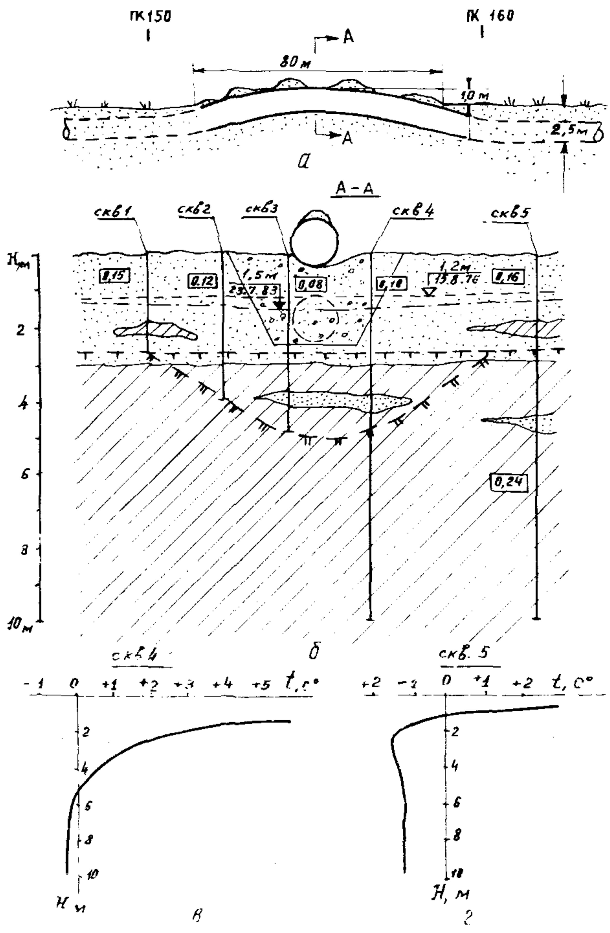
Схема (а), инженерно-геологический разрез (б) и температурные графики по скважинам (в, г) к акту обследования трубопровода: [пунктир] -пески; [штриховка] -суглинки; [шестиугольник] -грунты обратной засыпки; [0,15] -влажность весовая, ед.; - - - -верхняя граница многолетней мерзлоты до строительства; - - - -верхняя граница многолетней мерзлоты на момент обследования; - - - -уровень грунтовых вод до строительства; - - - -уровень грунтовых вод на момент обследования; ○ положение газопровода на момент обследования; ⊙ положение газопровода по проекту
