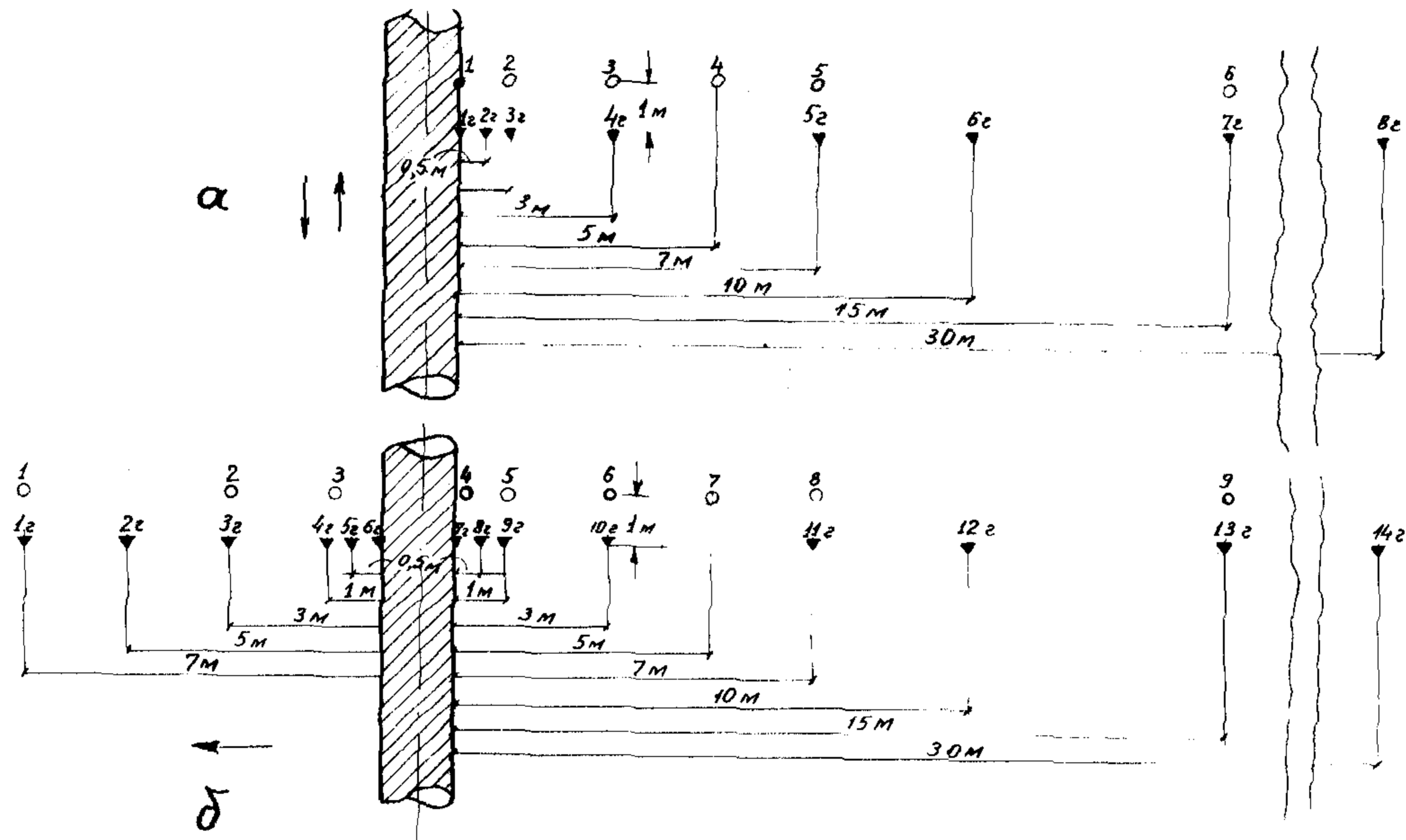
Схема расположения наблюдательных скважин на инженерно-геологическом поперечнике при различных видах прокладки трубопровода (виды прокладки трубопровода по рис.5): а-равнинная, продольносклоновая; б-поперечносклоновая, поперечностоковая; \nabla - гидрогеологическая скважина и ее номер; \circ - термометрическая скважина и ее номер; \downarrow - направление стока грунтовых вод в естественных условиях; \text{▨} - трубопровод
