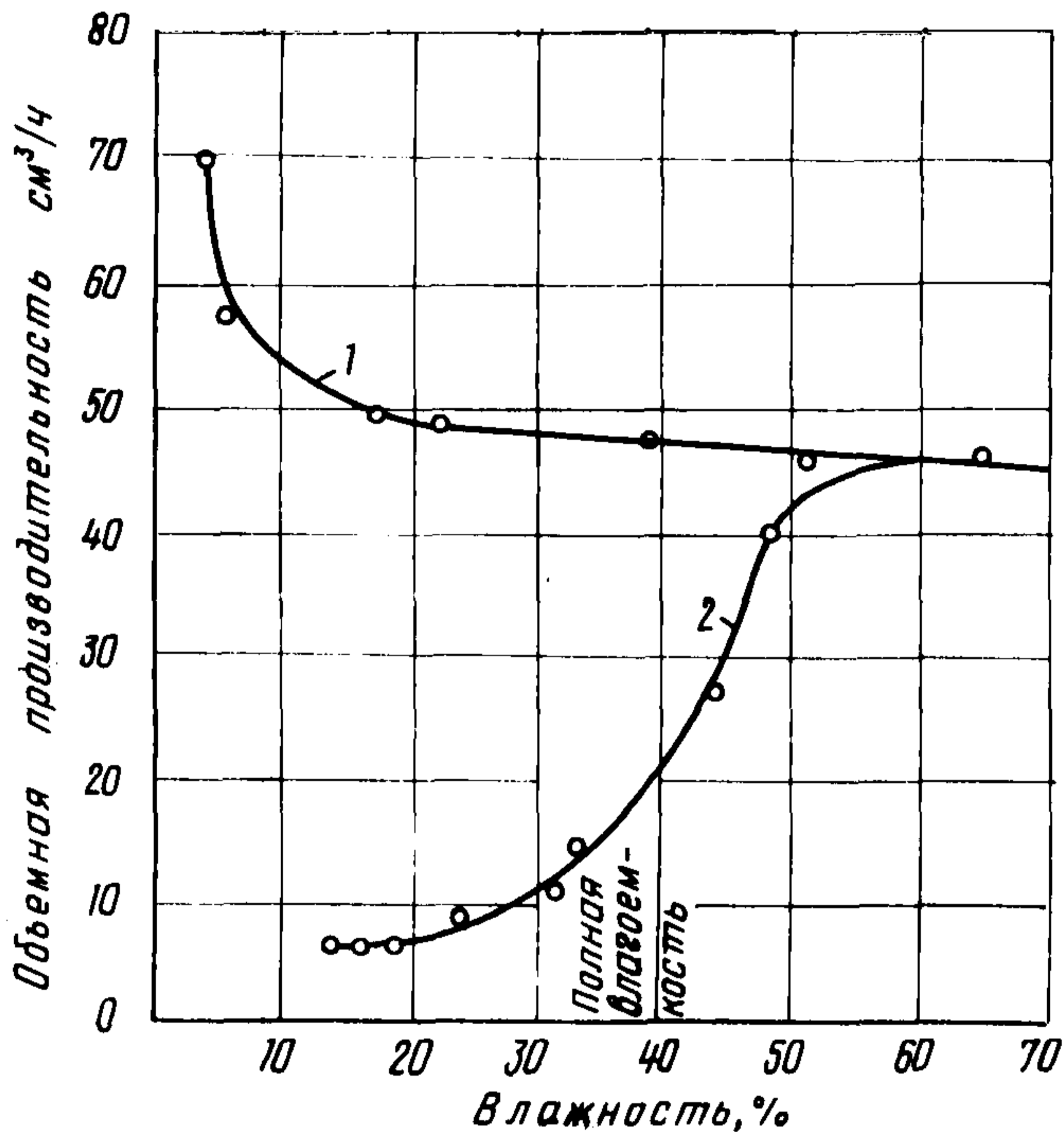
Рис. 3. Влияние влажности грунта на скорость бурения скважин:
