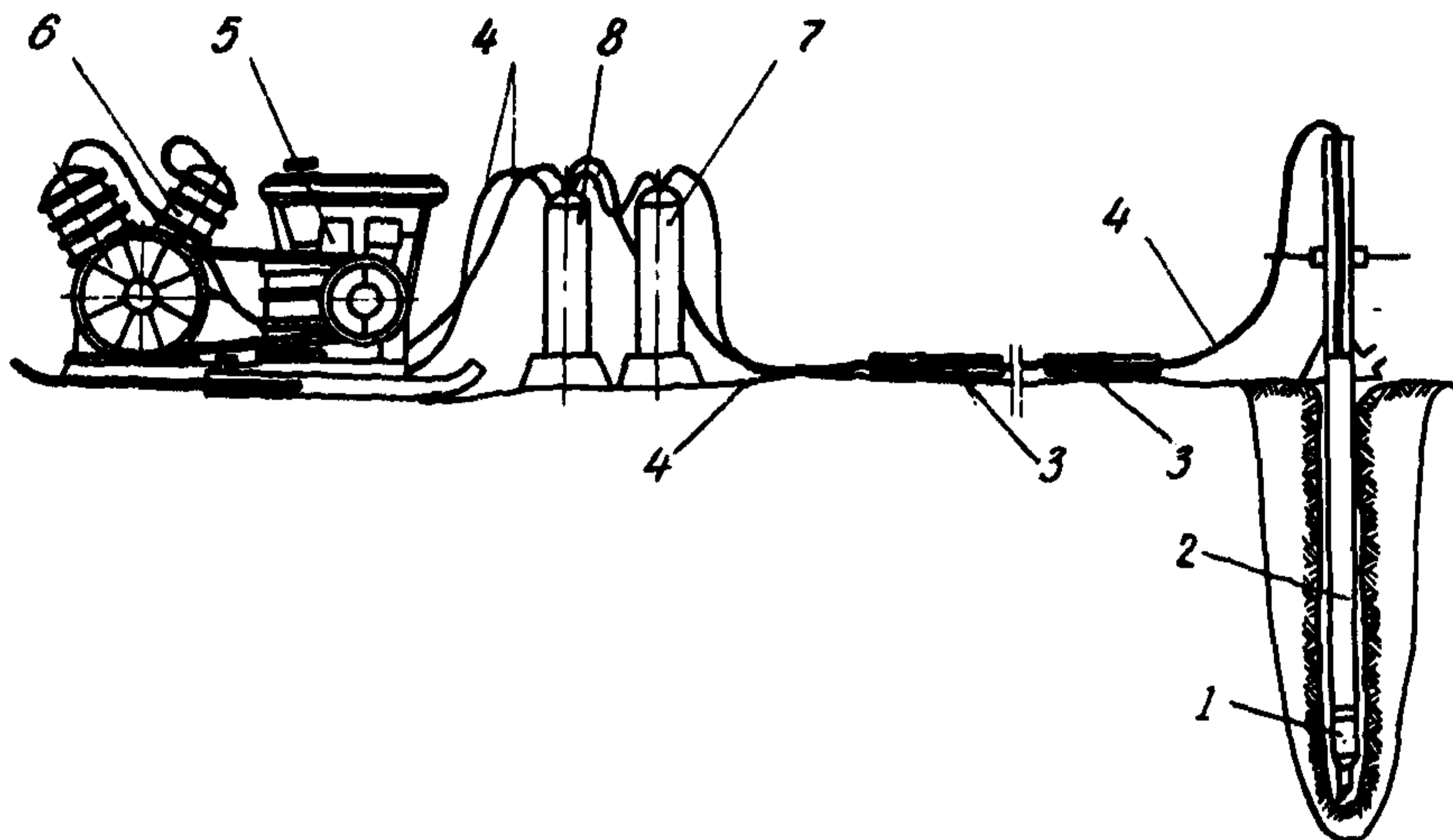
Рис.1. Принципиальная схема малогабаритной установки МТБУ-Д для огнеструйного бурения скважин:
