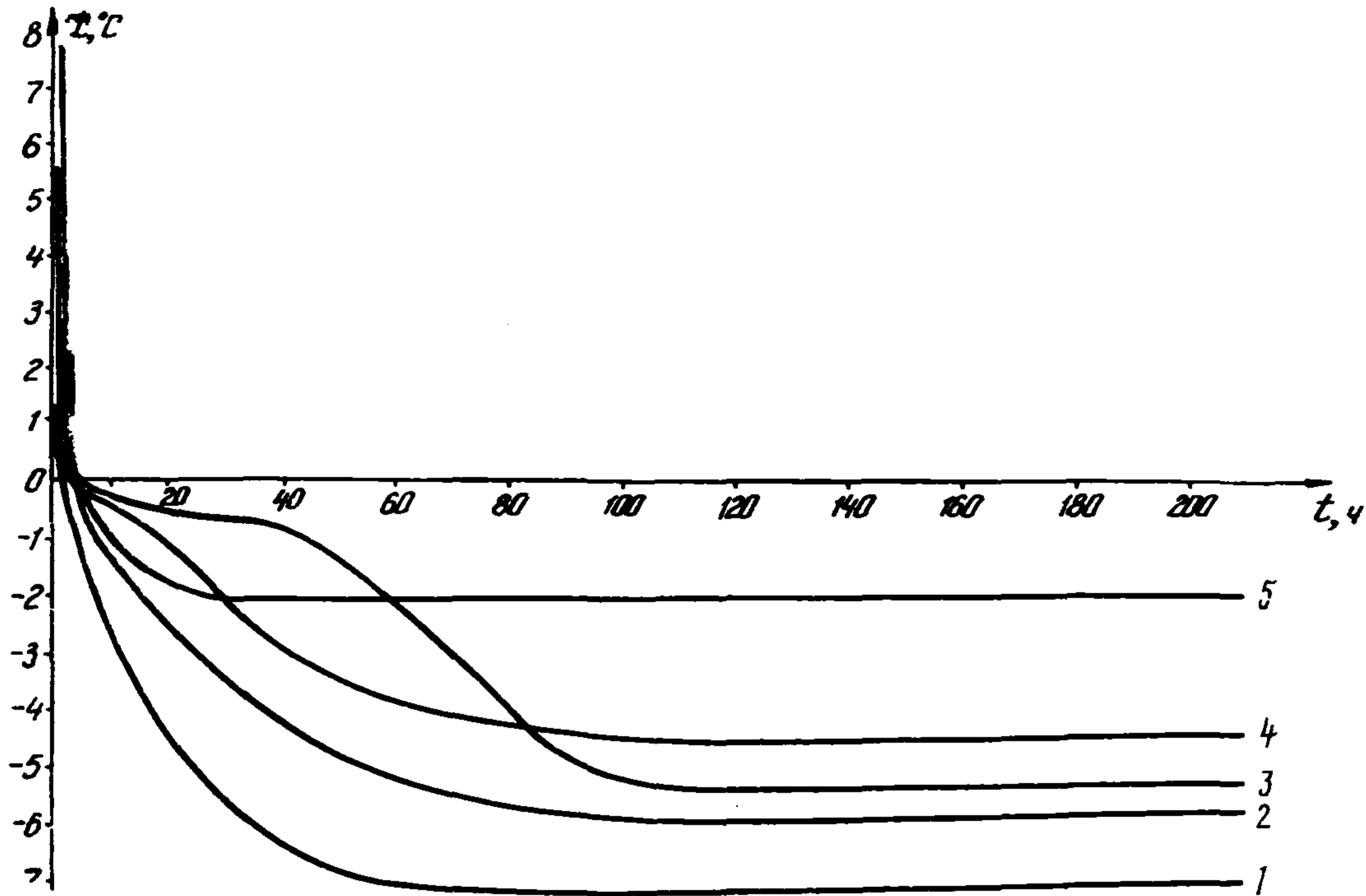
Рис. 13. Изменение температур на различных горизонтах скважины № 2 ( l_{скв} ) г. Норильска: 1 - l_{скв} = 3,0 м; 2 - l_{скв} = 2,5 м; 3 - l_{скв} = 2,0 м; 4 - l_{скв} = 1,0 м; 5 - l_{скв} = 0,5 м
