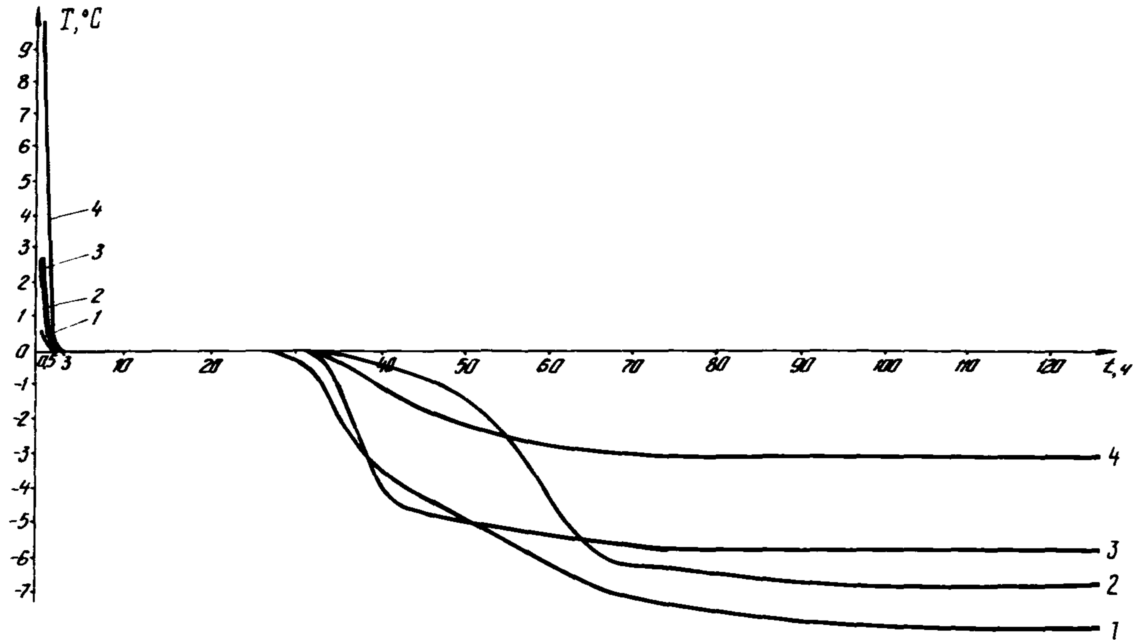
Рис. II. Изменение температур на различных горизонтах скважины № 2 ( l_{скв} ) пос. Малая Хета: 1 - l_{скв} = 5,0 м; 2 - l_{скв} = 4,5 м; 3 - l_{скв} = 3,5 м; 4 - l_{скв} = 2,0 м
