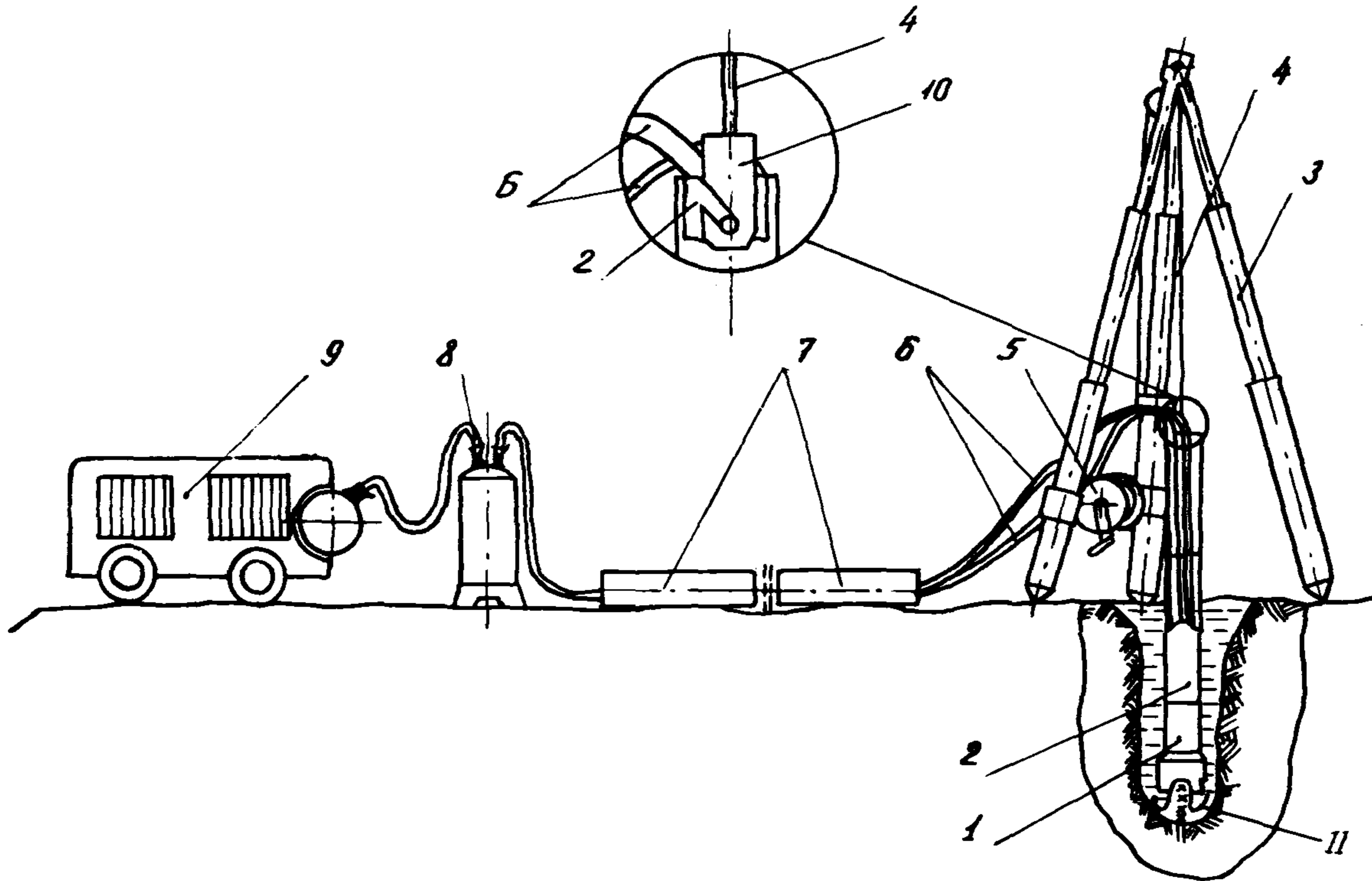
Рис.4. Схема подвески термобура ТВД-107м:
