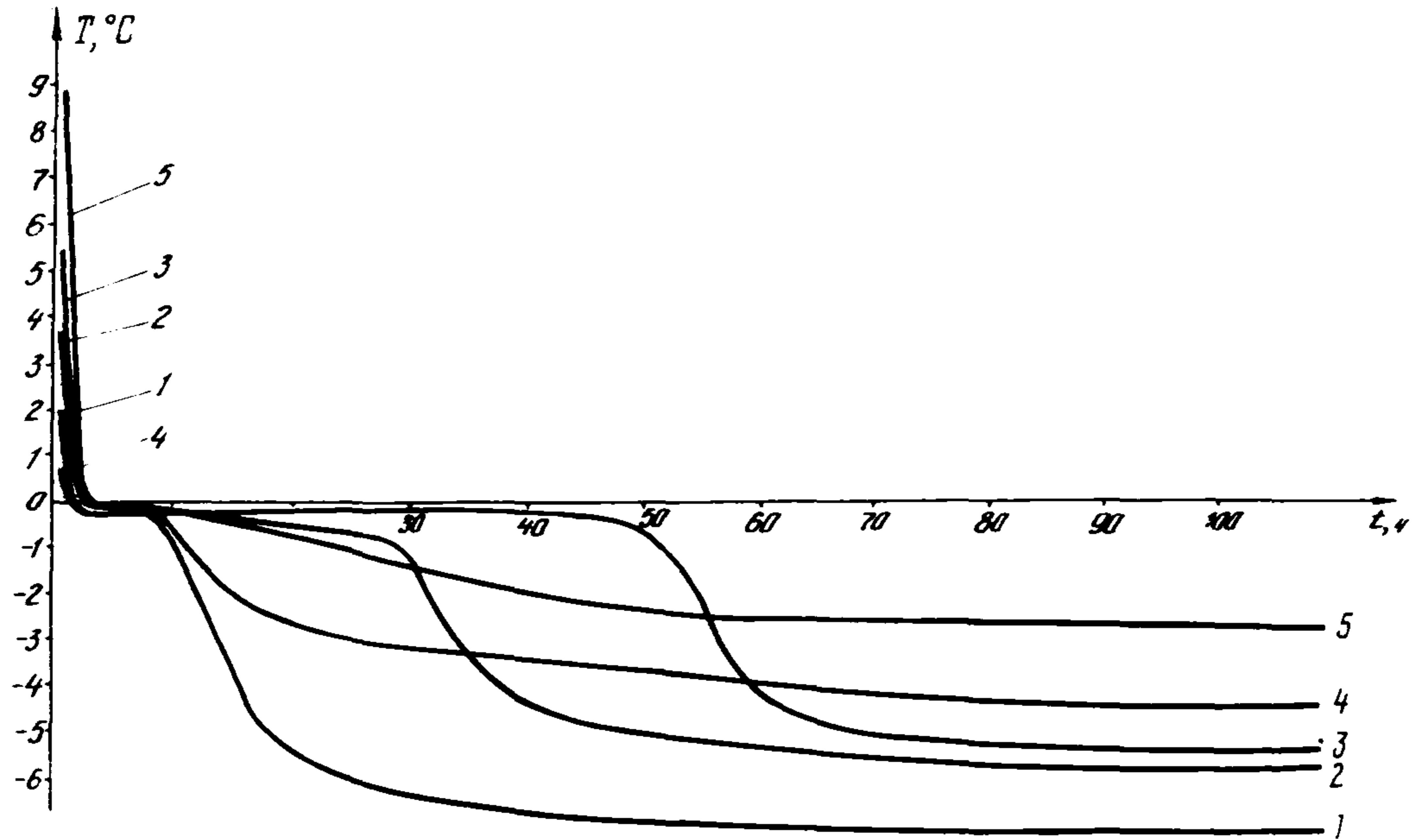
Рис. 12. Изменение температур на различных горизонтах скважины № 3 ( l_{\text{скв}} ) пос. Малая Хета: 1 - l_{\text{скв}} = 3,0 м; 2 - l_{\text{скв}} = 2,5 м; 3 - l_{\text{скв}} = 2,0 м; 4 - l_{\text{скв}} = 1,0 м; 5 - l_{\text{скв}} = 0,5 м
