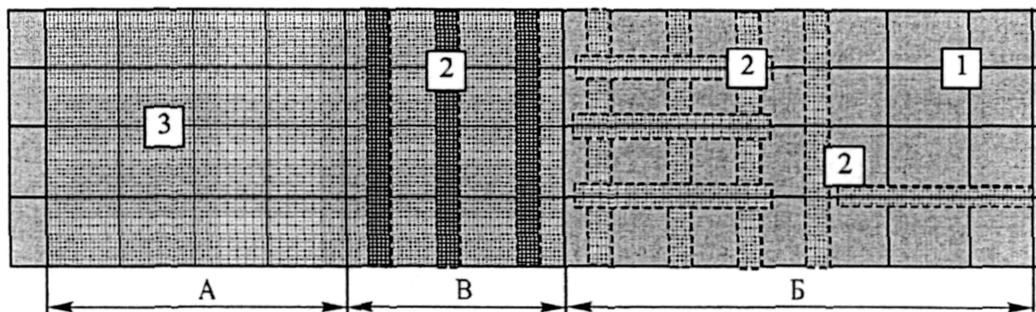
Рисунок 2. Схемы укладки геосетки (геокомпозита): A – сплошная; Б – участковая; В – комбинированная; 1 – «старое» покрытие со швами (трещинами); 2 – полосы геосетки; 3 – полотно геосетки
