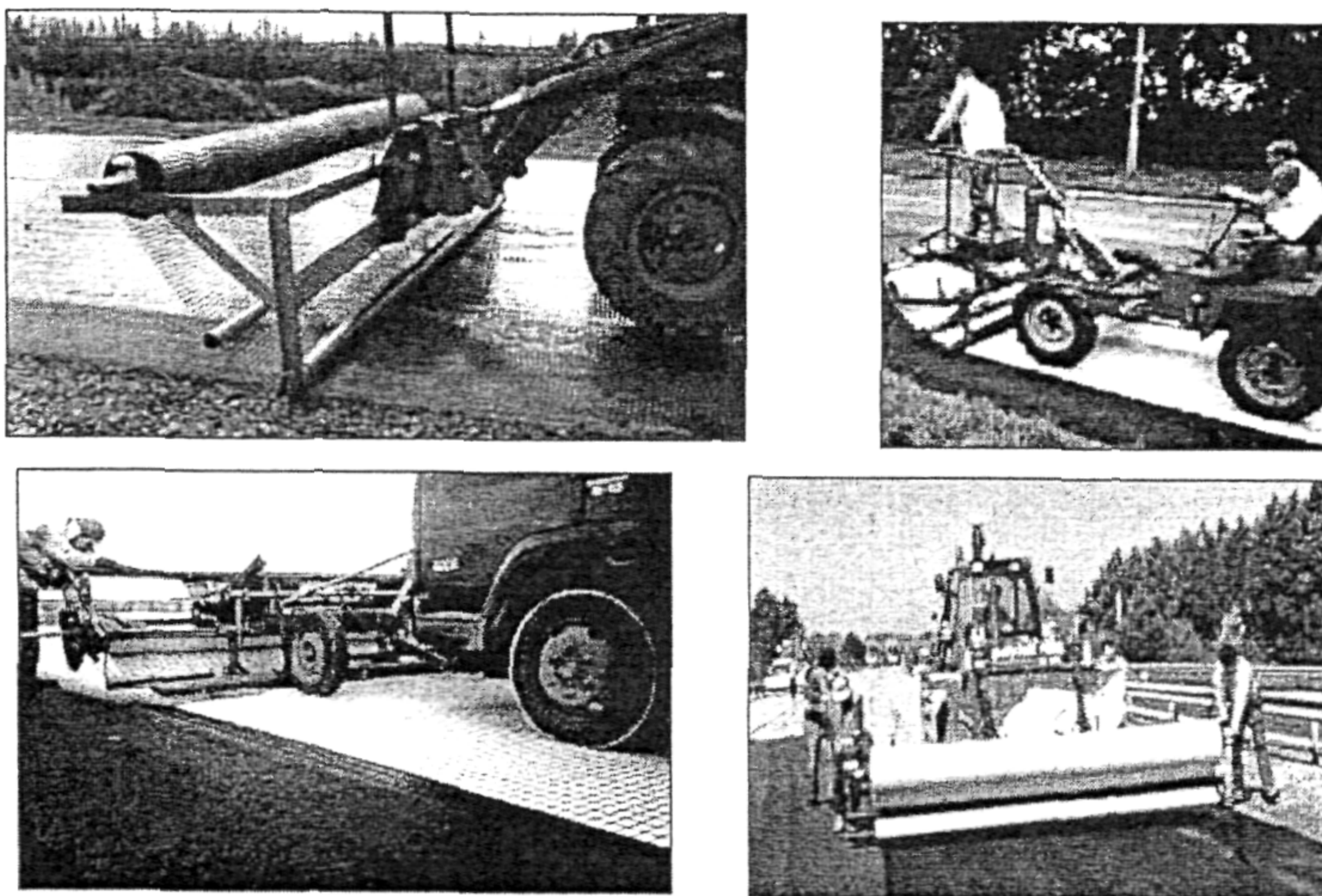
Рисунок 6 . Навесные механизмы для раскладки армирующих материалов
