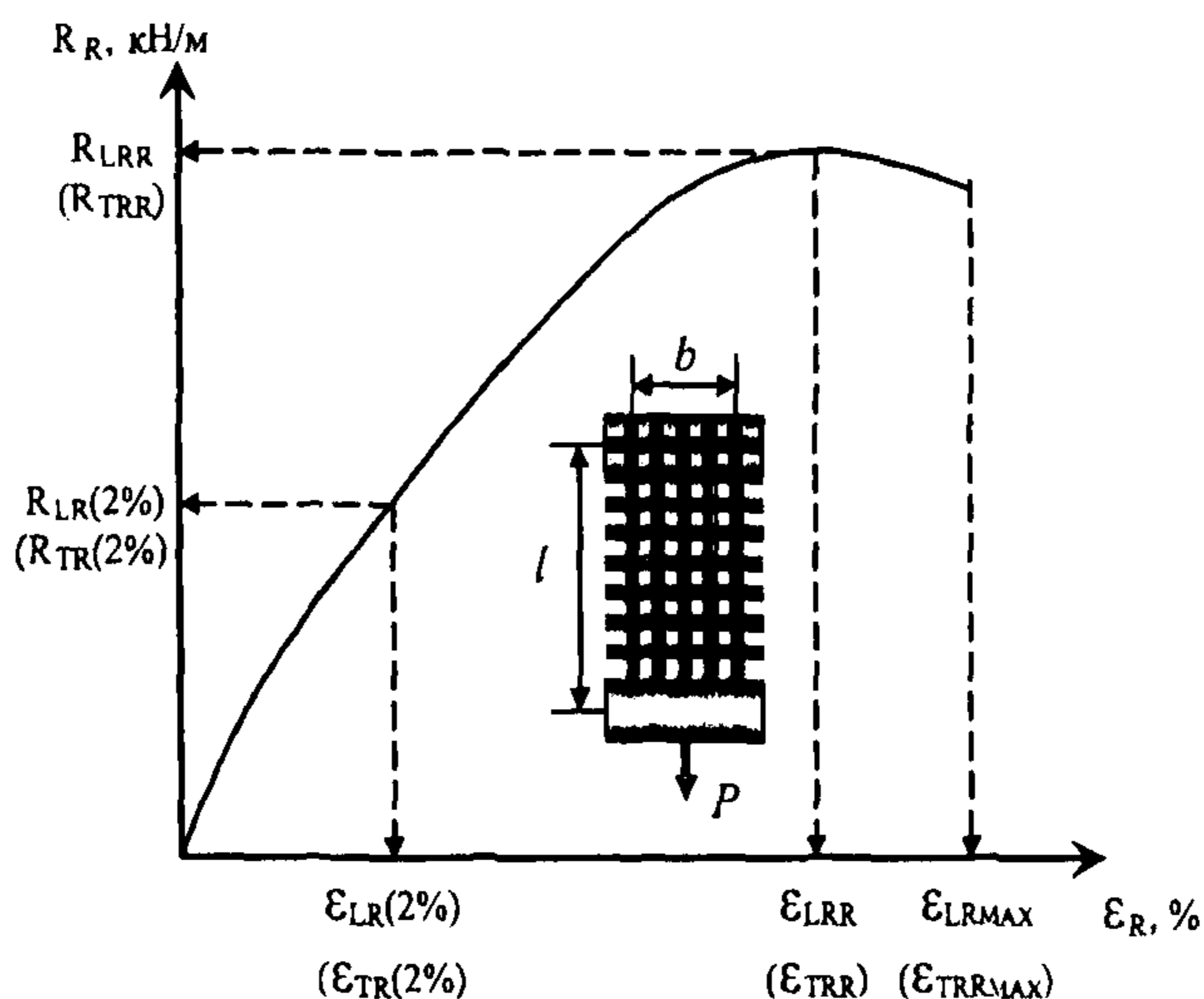
Рисунок Б 1.2 . График зависимости деформации от нагрузки
