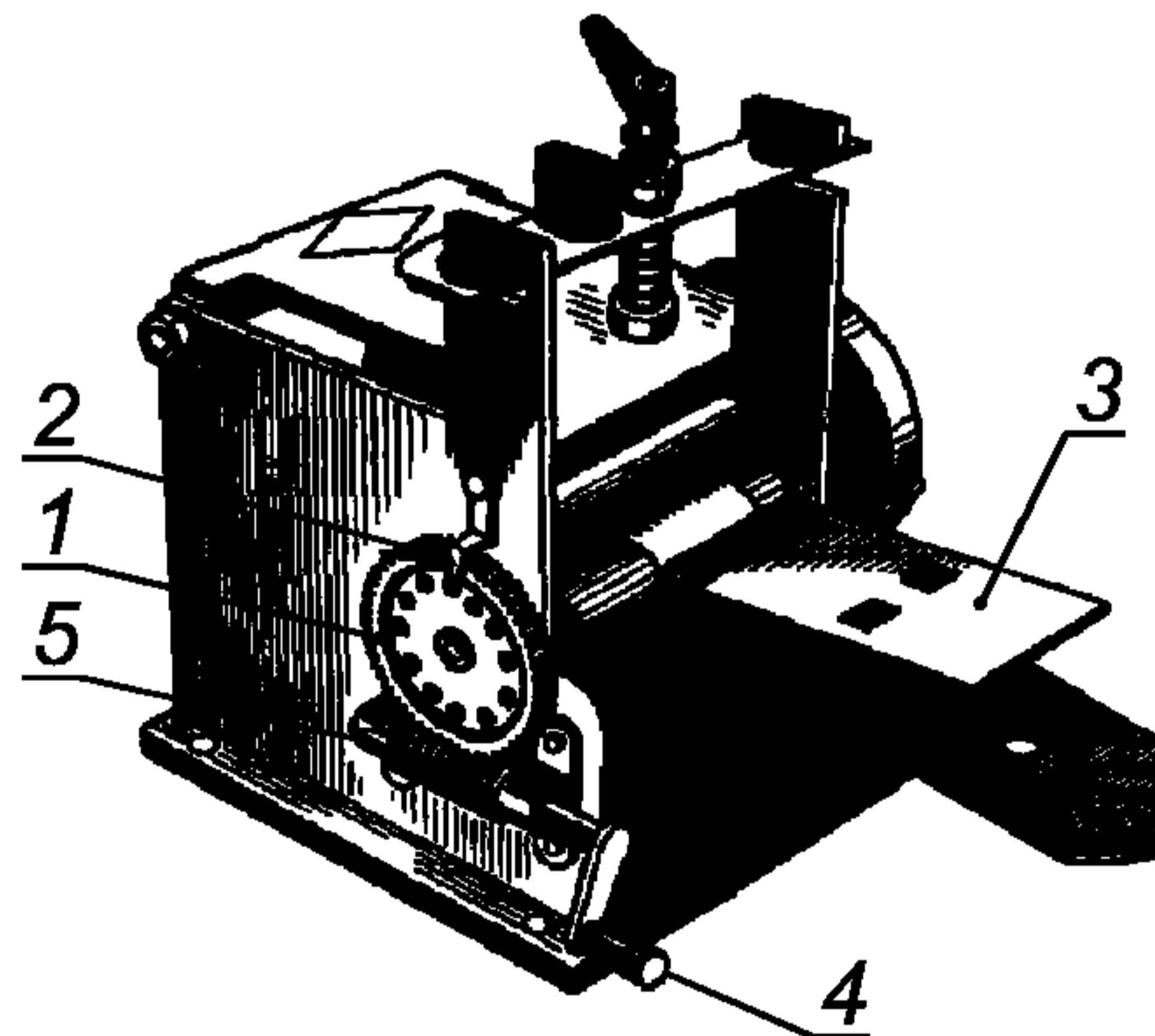
1 — червячное колесо; 2 — указатель; 3 — зажим № 2; 4 — рукоятка червяка; 5 — червяк
