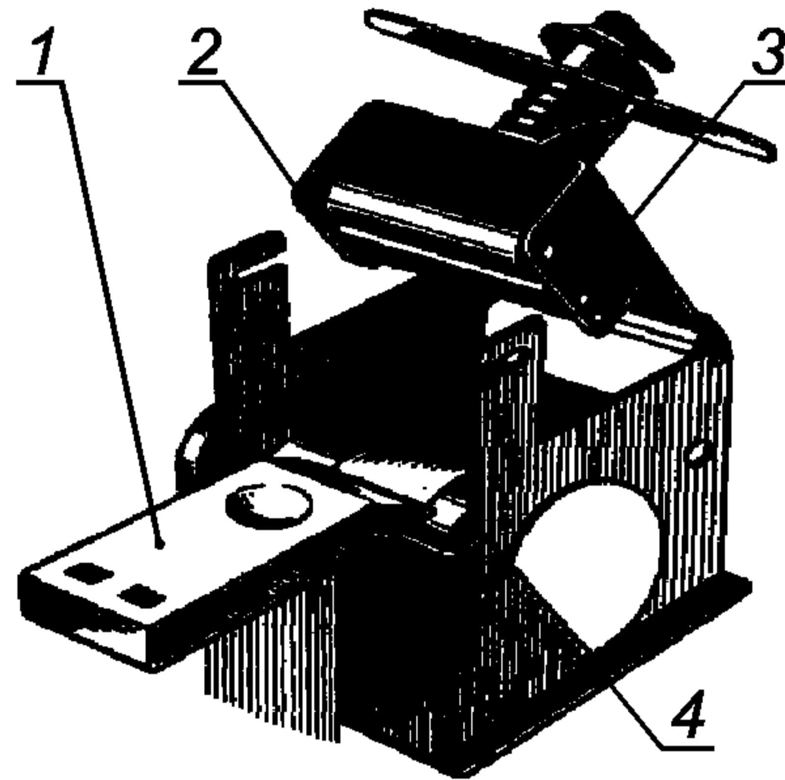
1 — зажим № 1; 2 — валик; 3 — крышка; 4 — фартук
