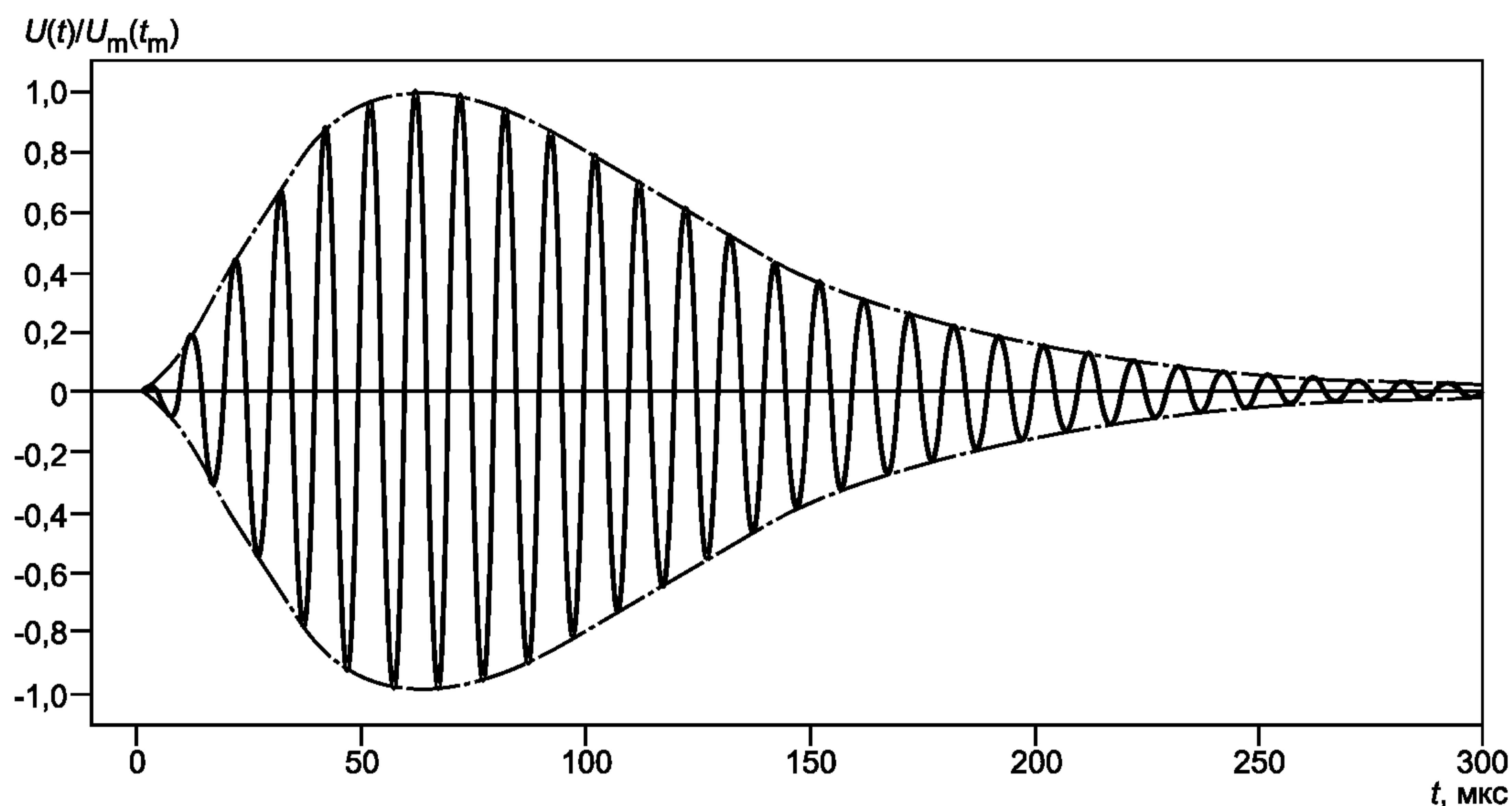
Рисунок 2 — Типичная форма радиоимпульса с экспоненциально-степенной огибающей.
