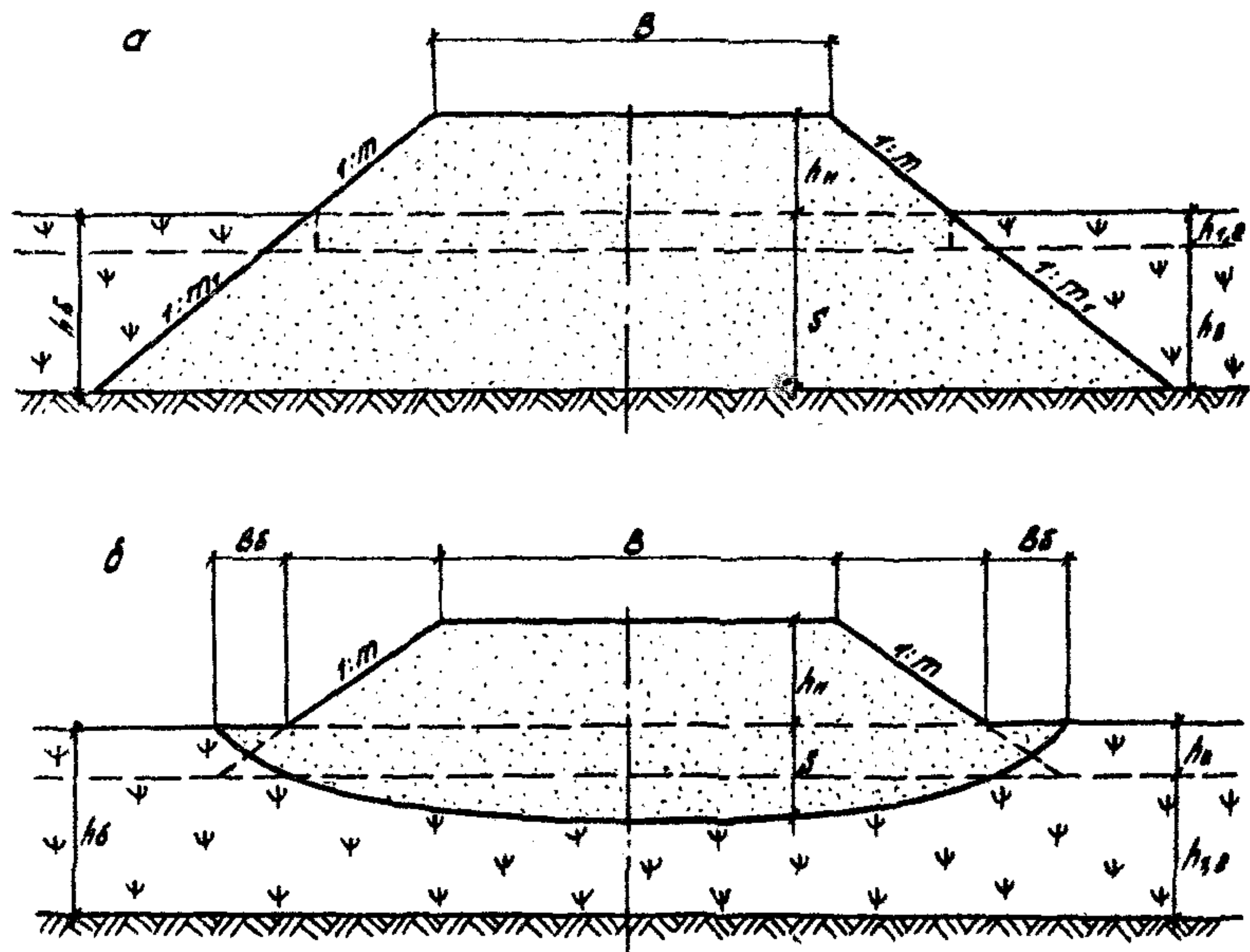
Рис. 3.5. Поперечные профили земляного полотна на болотах I, III типов без вырезки торфа: а - на болоте III типа со слявиной сверху; б - на болоте III типа с торфом I, II типов внизу
