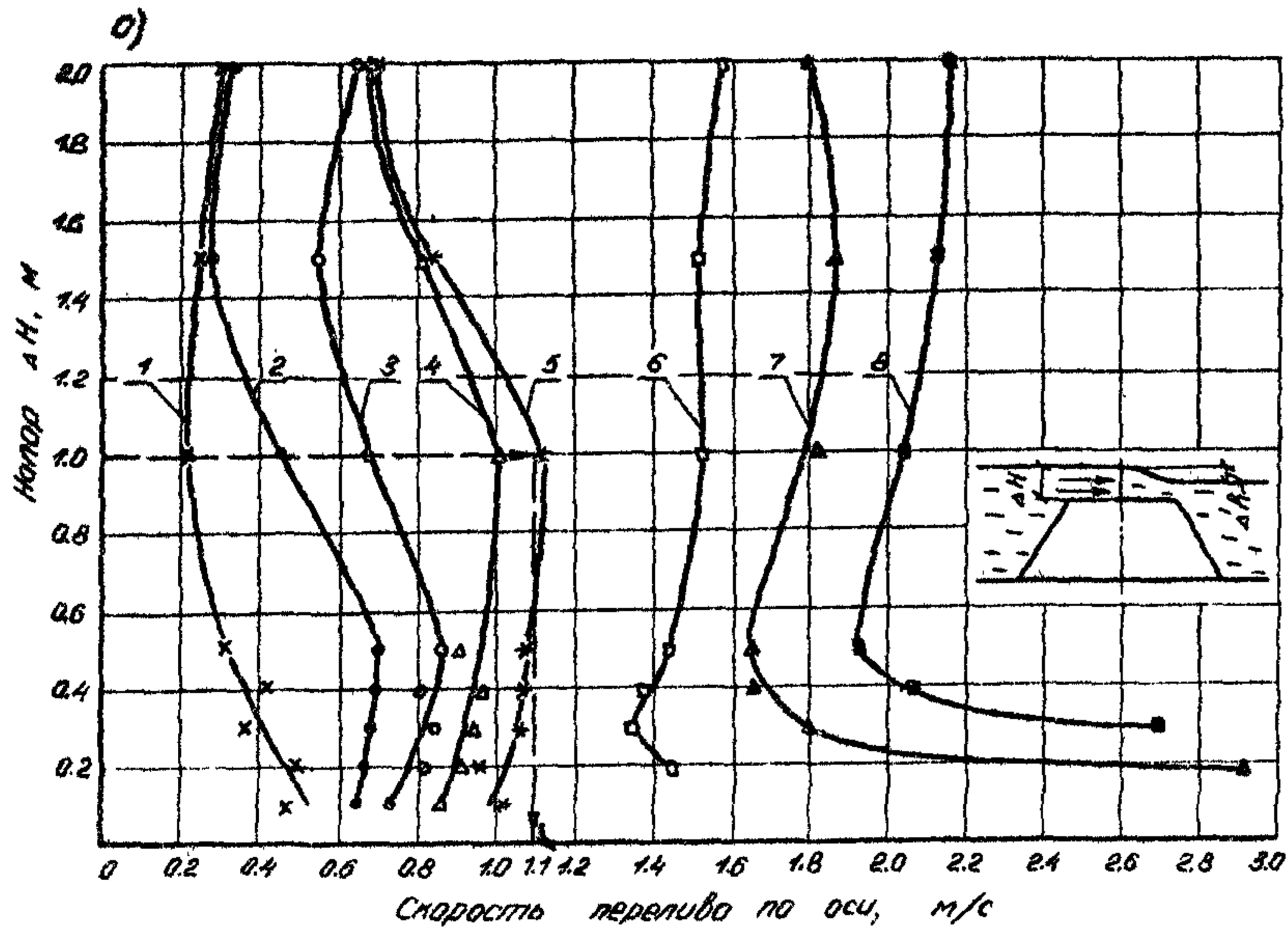
Рис. 4.14. График для определения скоростей перелива по оси (а) и на бровке (б) затопленной насыпи при подпоре ( \Delta h ), равном: 1-1 см; 2-2 см; 3-3 см; 4-4 см; 5-5 см; 6-10 см; 7-15 см; 8-20 см
