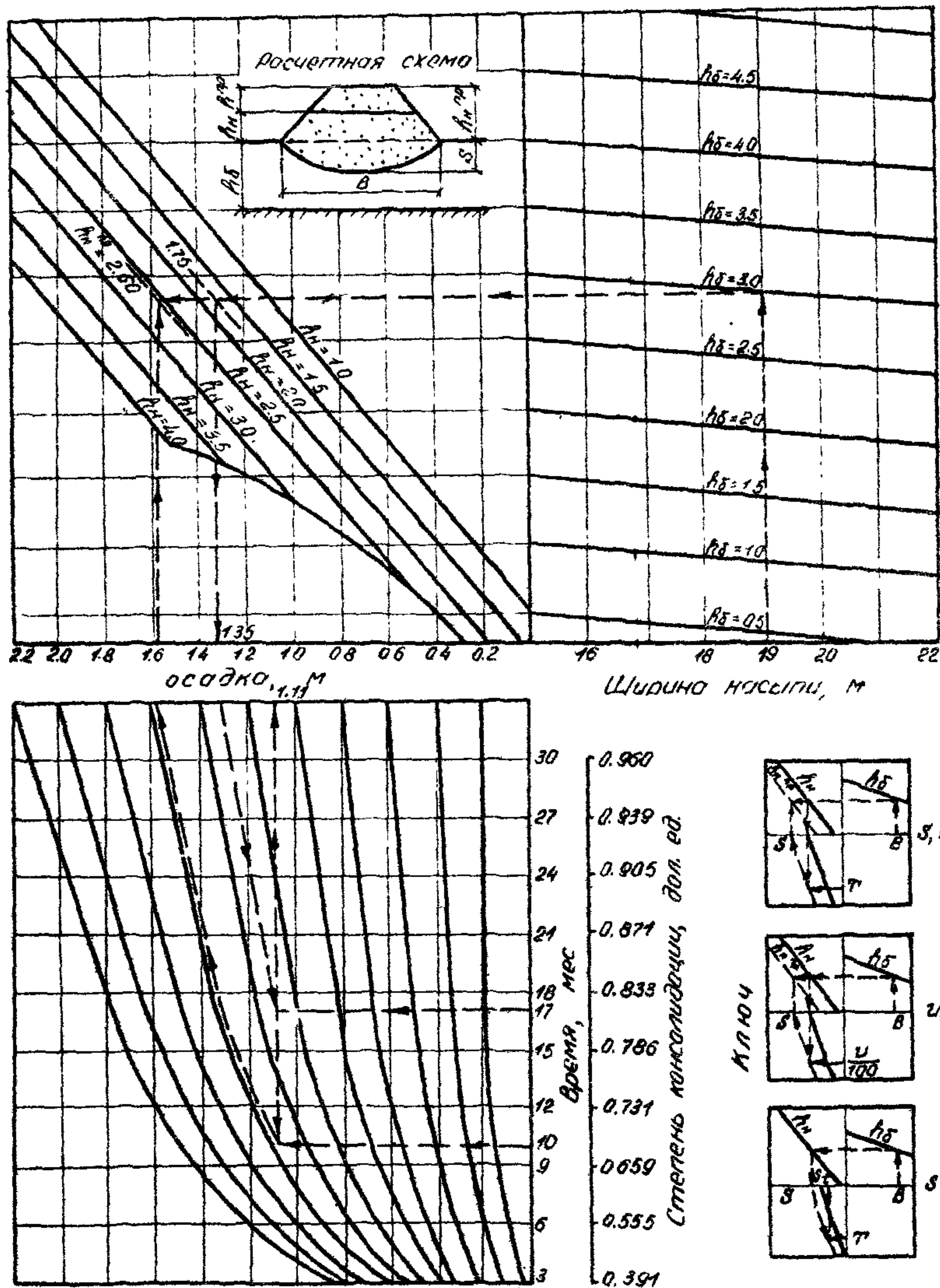
Рис. 3.10. Номограмма для определения осадки ( S ), консолидации ( U ), времени консолидации ( T ) торфяного основания и высоты временной пригрузки насыпи на болоте II типа
