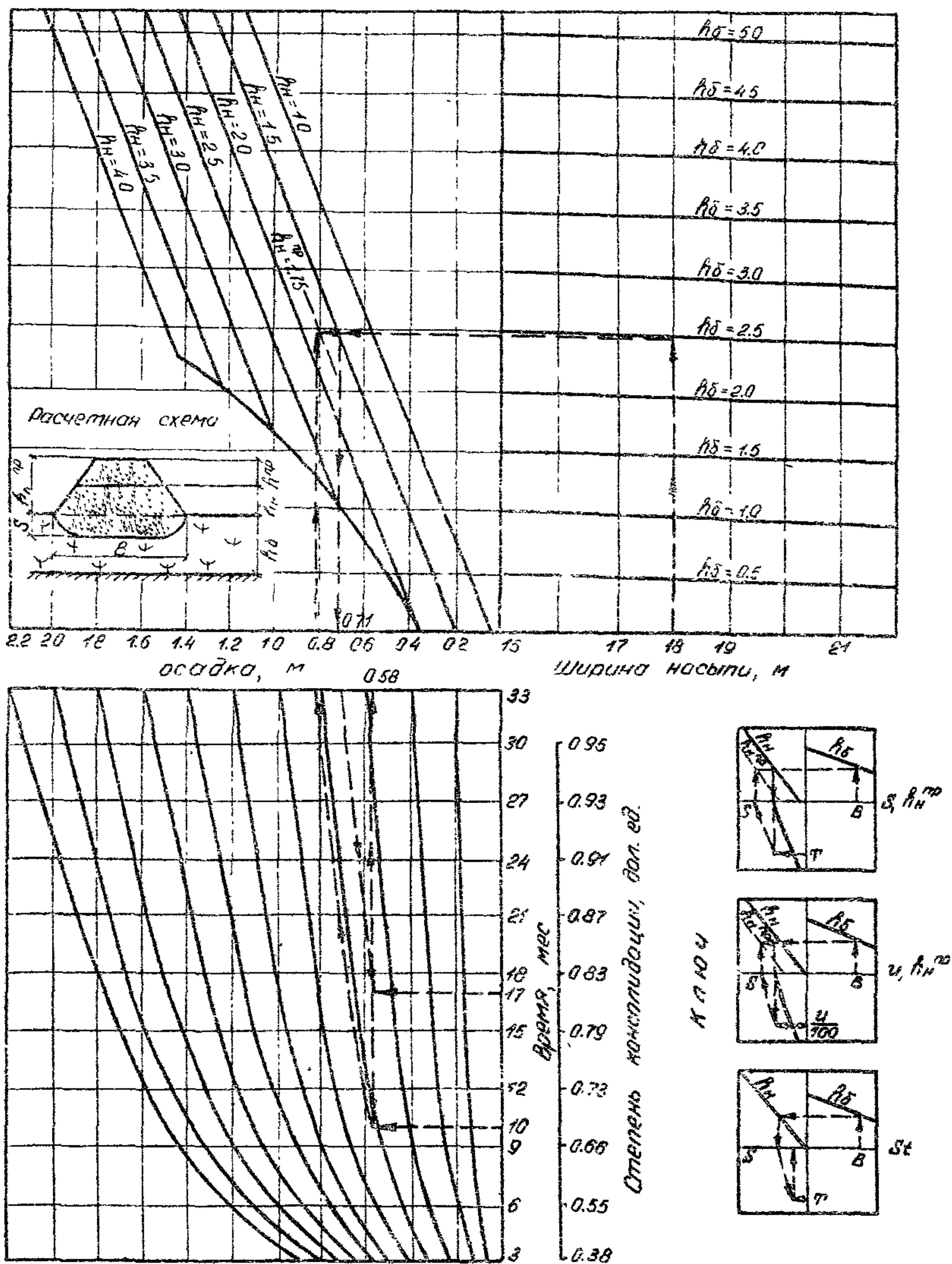
Рис. 3.9. Номограмма для определения осадки ( S ), консолидации ( U ), времени консолидации ( T ) торфяного основания и высоты временной пригрузки насыпи на болоте I типа
