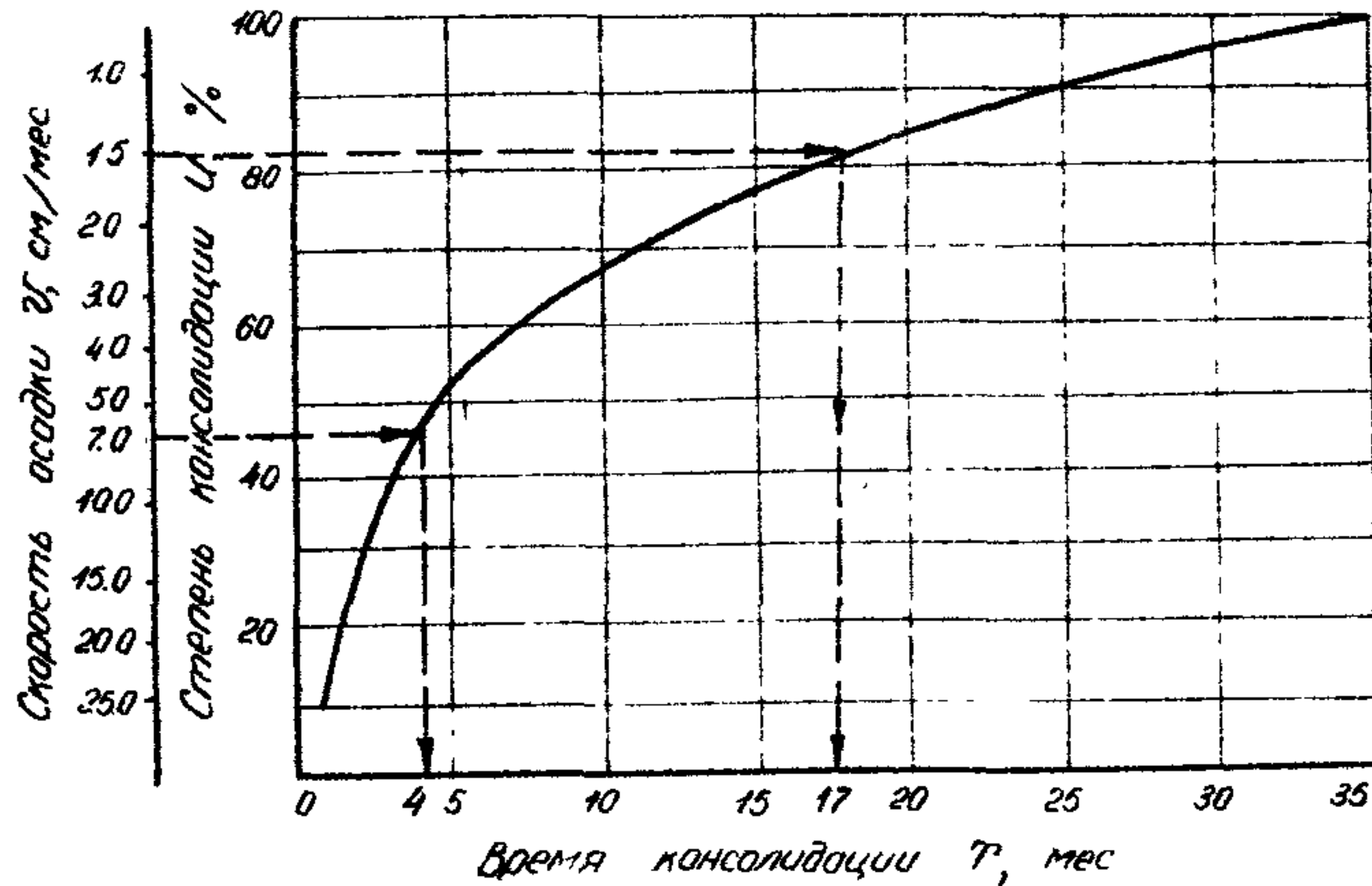
Рис. 3. II. Зависимости степени консолидации ( U ) и скорости осадки ( V ) насыпи на торфе от времени ( T ).
