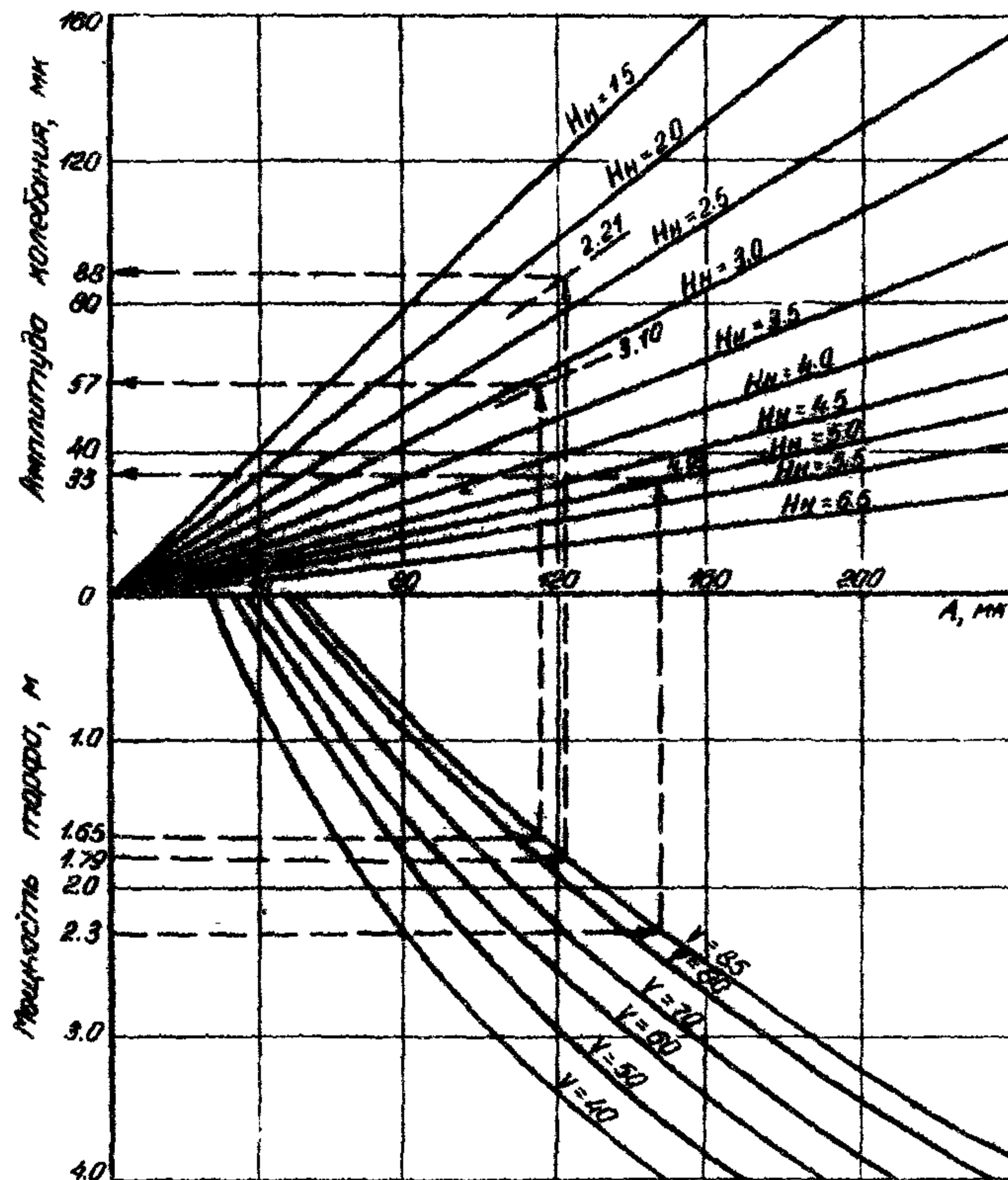
Рис. 3.14. Зависимость амплитуды колебаний от A , V_x , H_n
