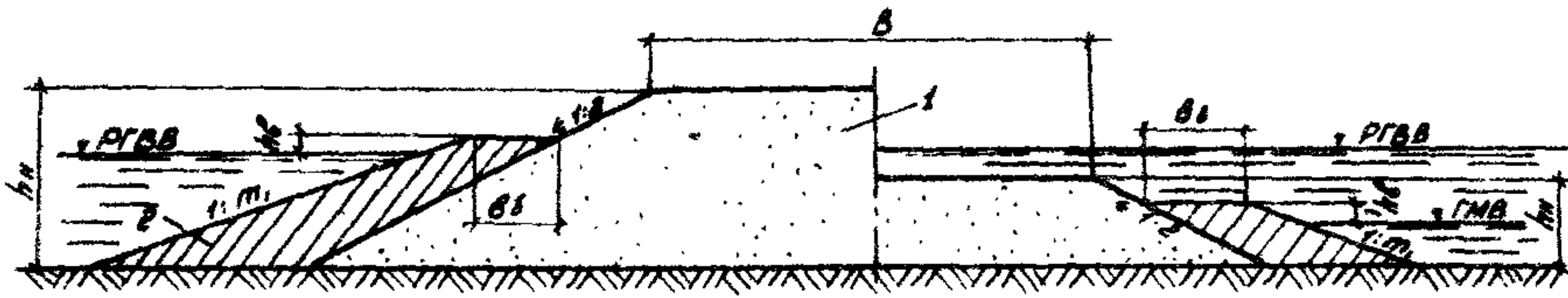
Рис. 4.6. Насыпи из песка и глинистого грунта в откосной части на старицах и озерах: 1 - песок; 2 - глинистый грунт
