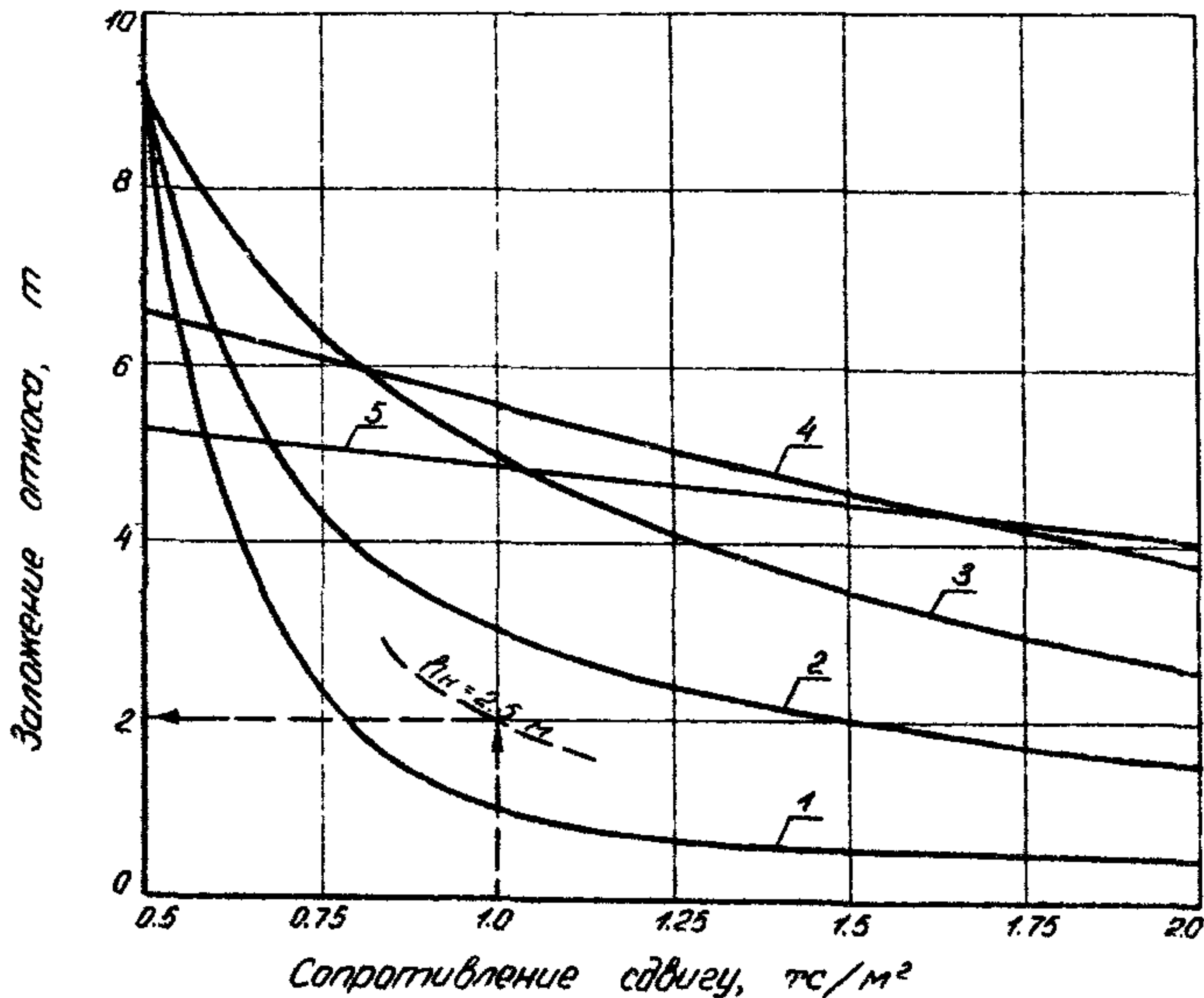
Рис. 4.12. Зависимость требуемого заложения откоса насыпи из мелкозернистого песка от сопротивления сдвигу грунта основания: 1 - h_H = 2 м; 2 - h_H = 3 м; 3 - h_H = 4 м; 4 - h_H = 8 м; 5 - h_H = 12 м
