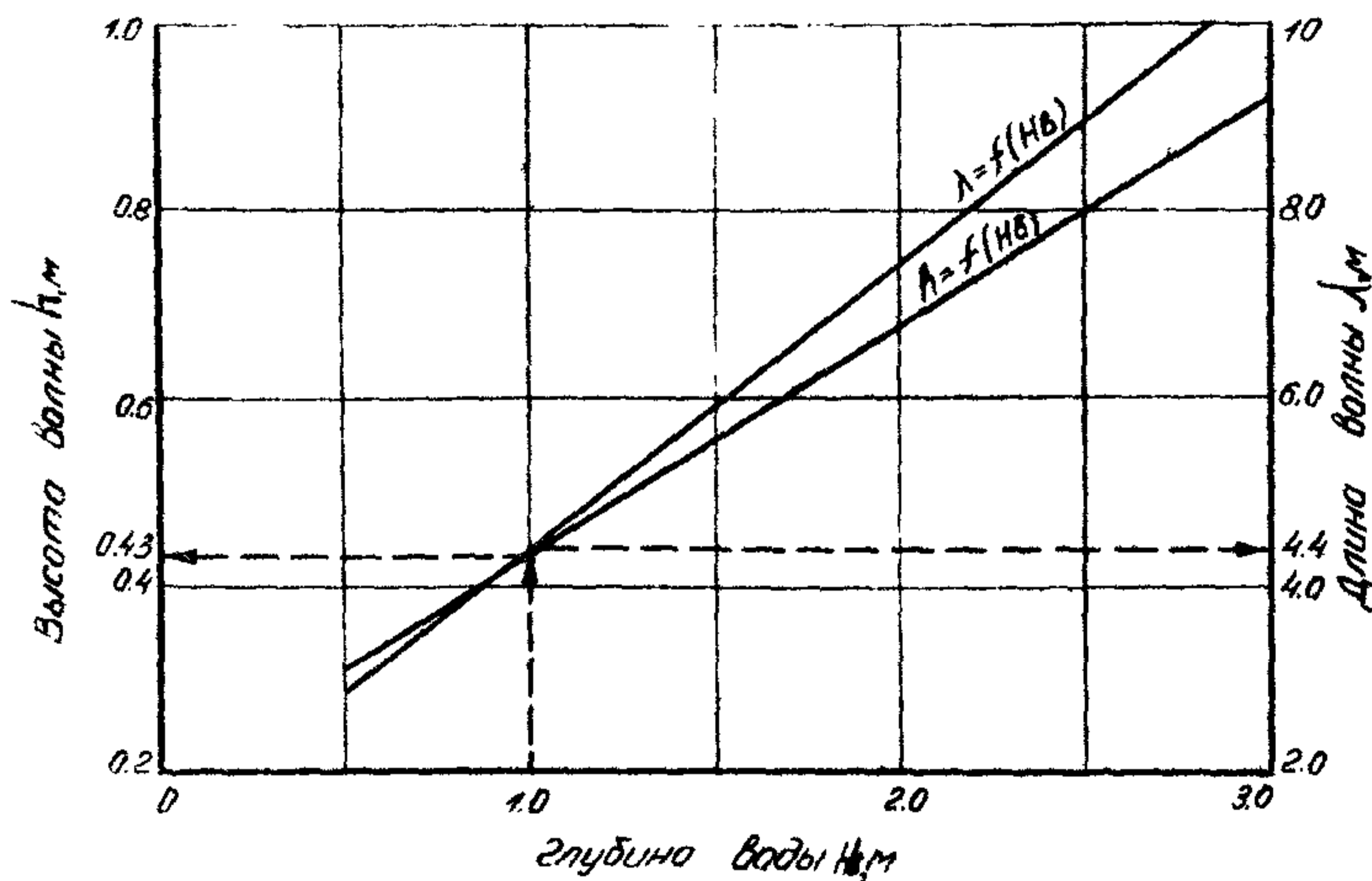
Рис. 4.13. Номограмма для определения высоты и длины волны в зависимости от глубины водоема
