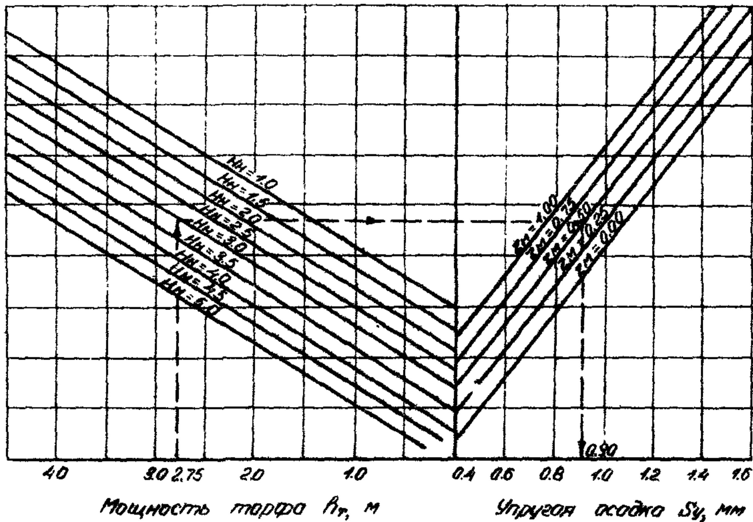
Рис. 3.13. Зависимость величины упругой осадки ( S_y ) от мощности насыпи ( H_n ), торфа ( h_T ) и мерзлого перелетка ( Z_m ) в основании
