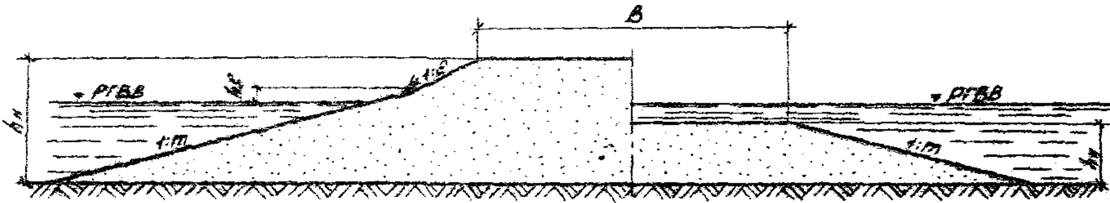
Рис. 4.1. Насыпи из песка на поймах рек
