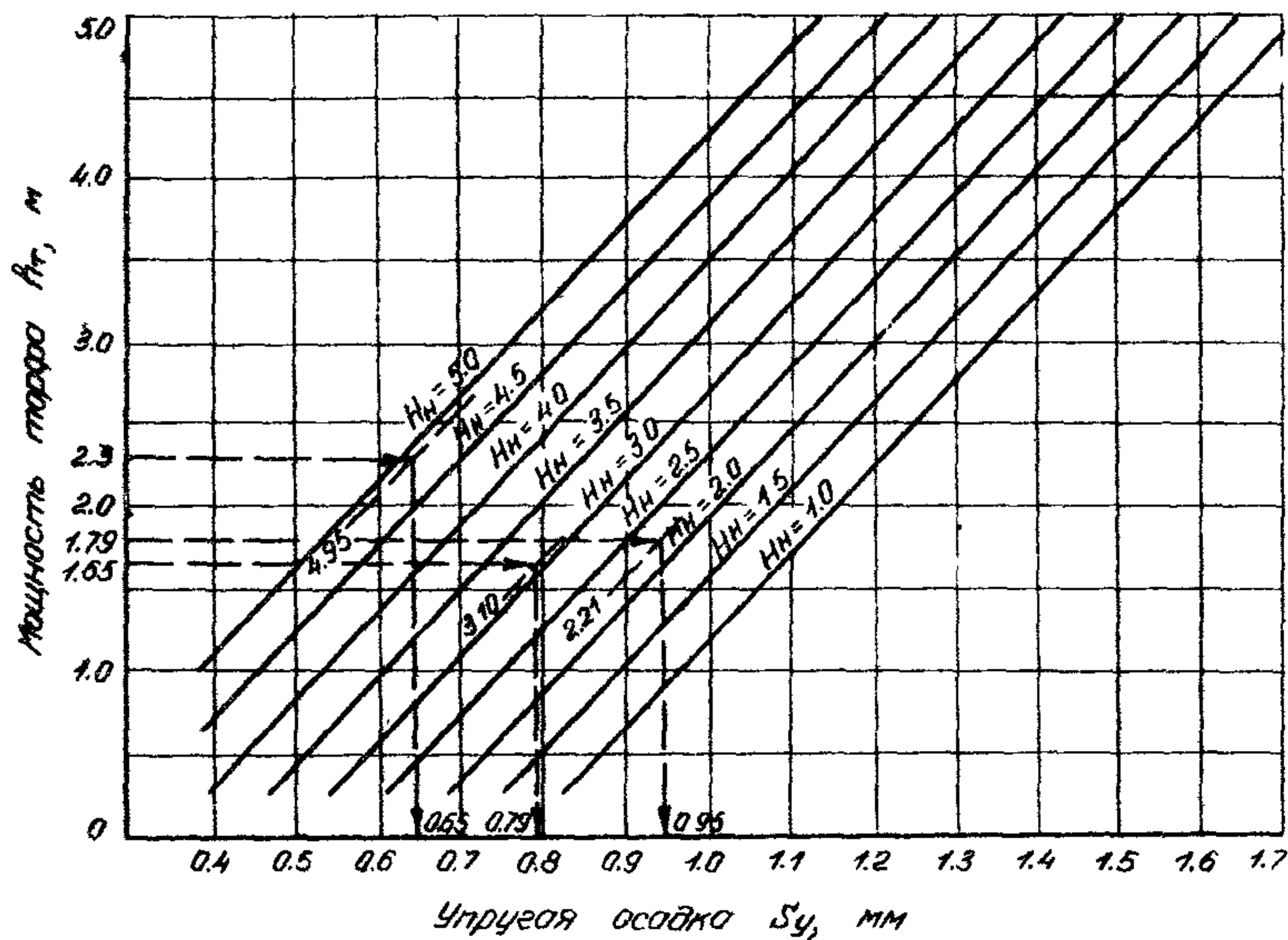
Рис. 3.12. Зависимость величины упругой осадки ( S_y ) от мощности насыпи ( H_H ) и торфа ( h_T ) в основании
