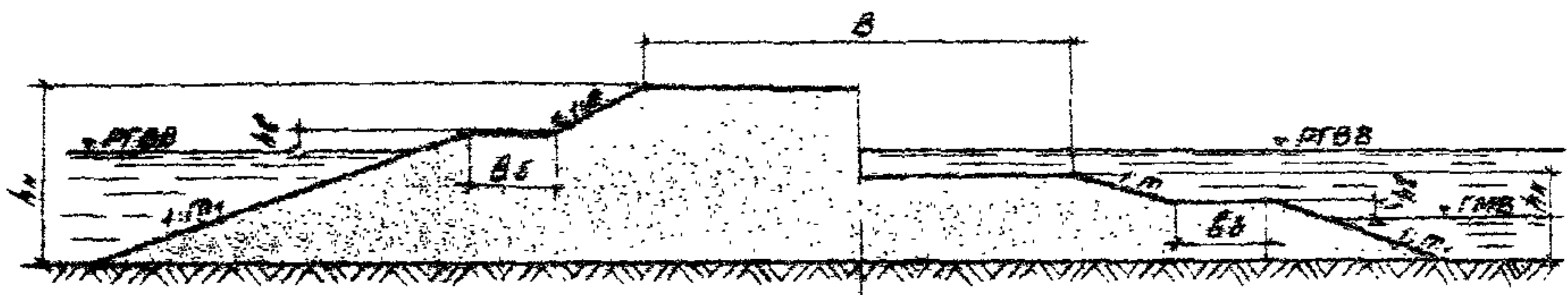
Рис. 4.5. Насыпи из песка на старицах и озерах
