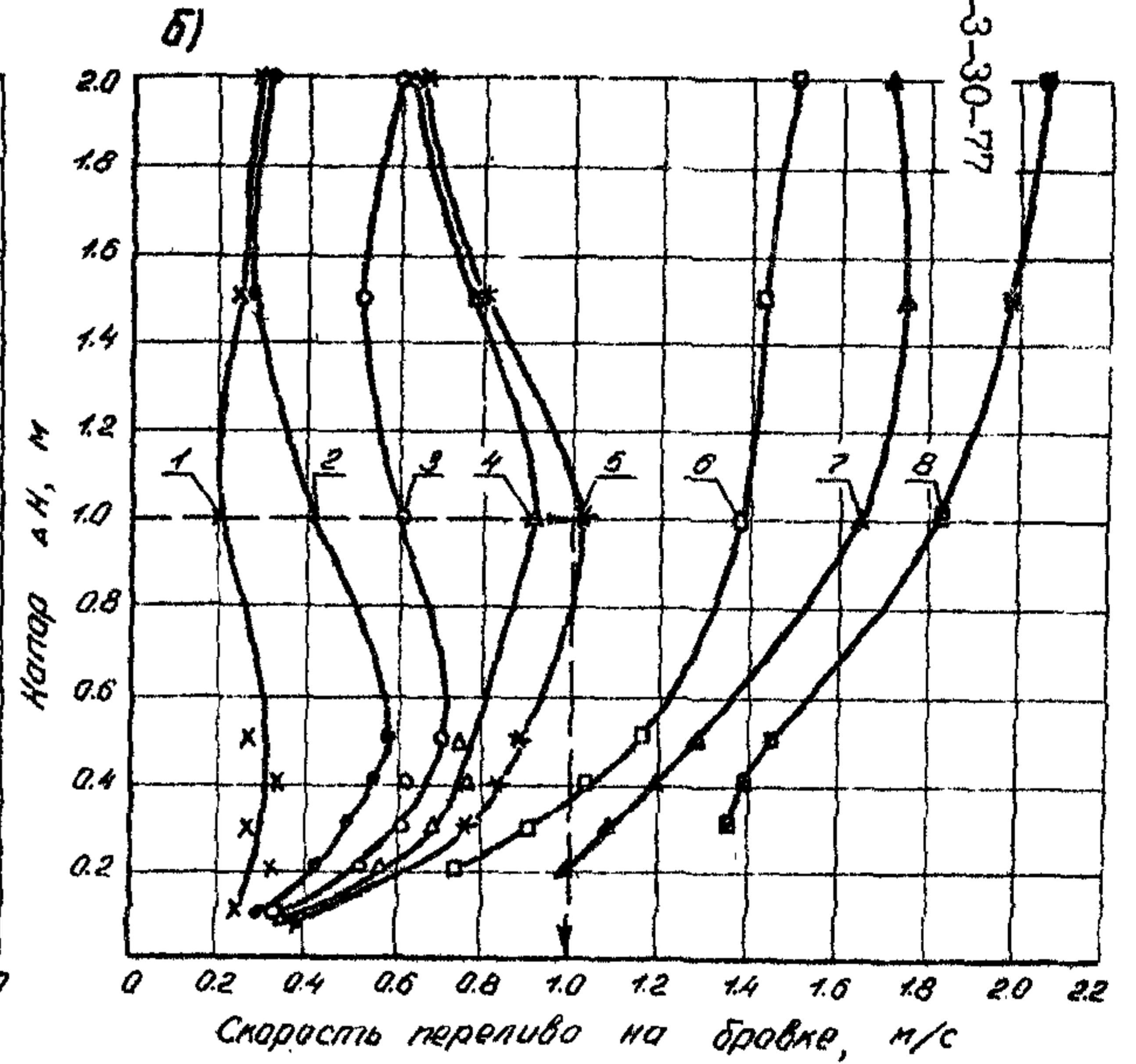
Рис. 4.14. График для определения скоростей перелива по оси (а) и на бровке (б) затопленной насыпи при подпоре ( \Delta h ), равном: 1-1 см; 2-2 см; 3-3 см; 4-4 см; 5-5 см; 6-10 см; 7-15 см; 8-20 см
