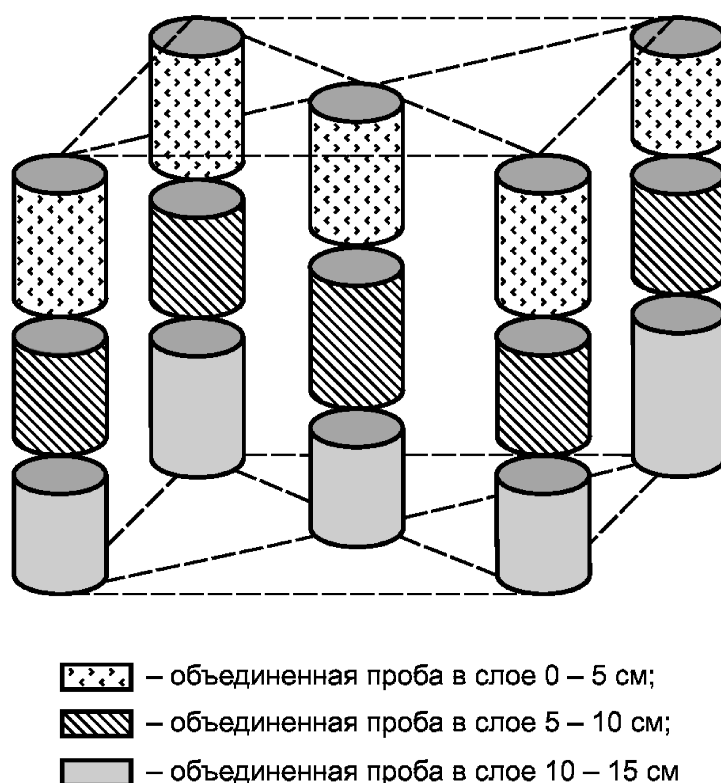
Рисунок 2 — Схема отбора объединенной пробы
