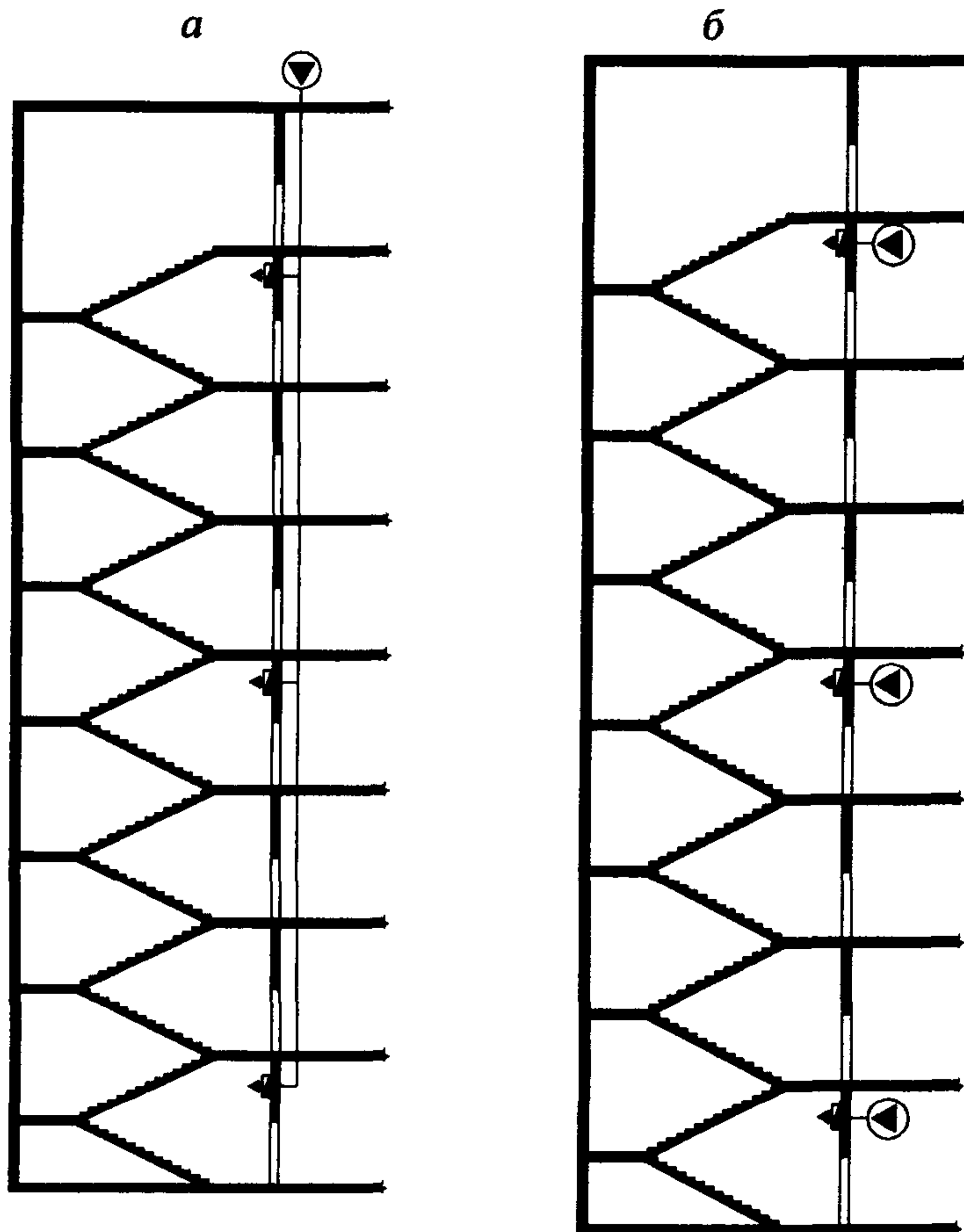
Рис. 4. Схема распределенной подачи воздуха в лестничную клетку:
