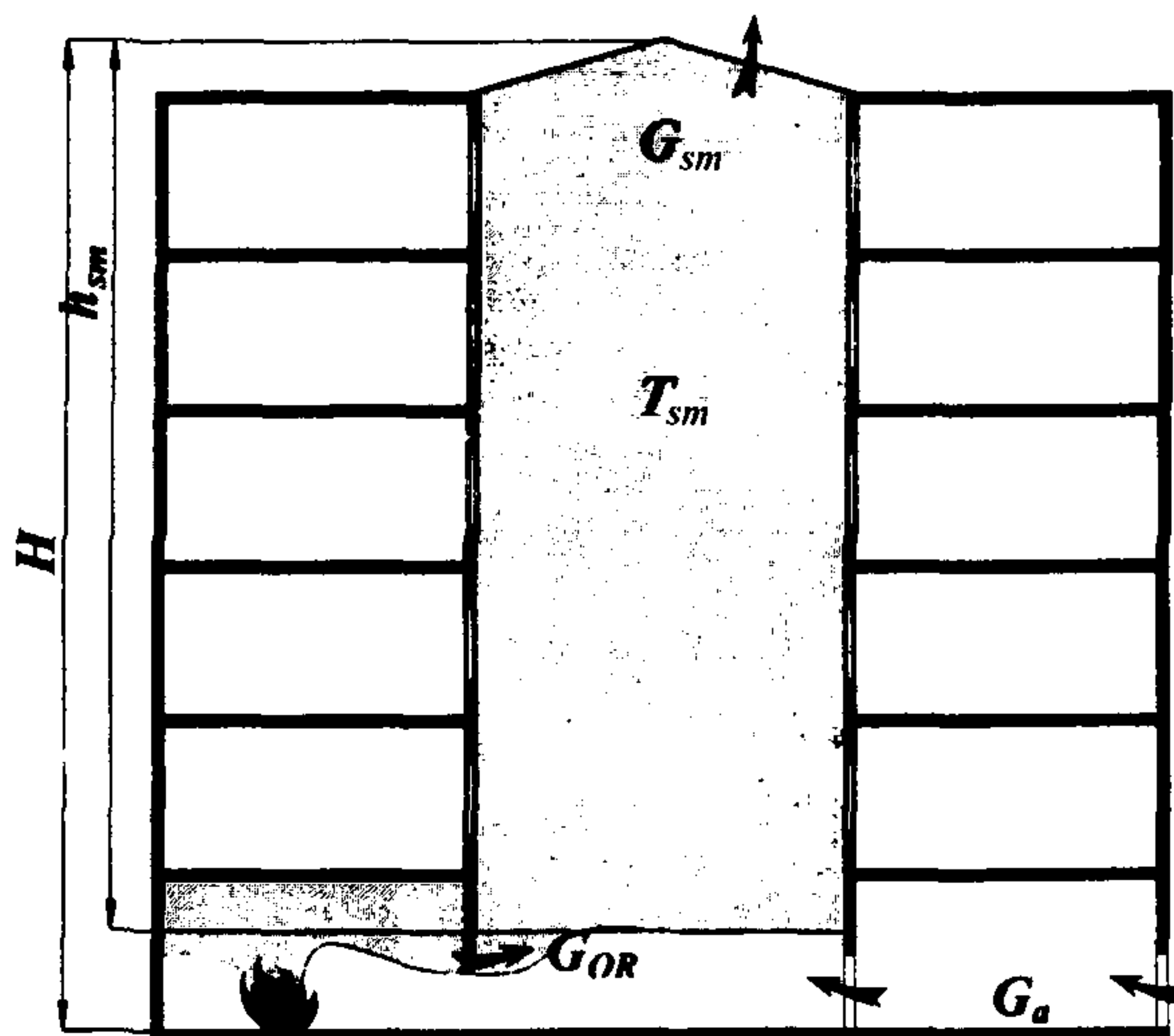
Рис. 2. Расчетная схема газообмена при пожаре в атриуме с конструктивно неотделенными галереями (а) и с конструктивно отделенными этажами (б)
