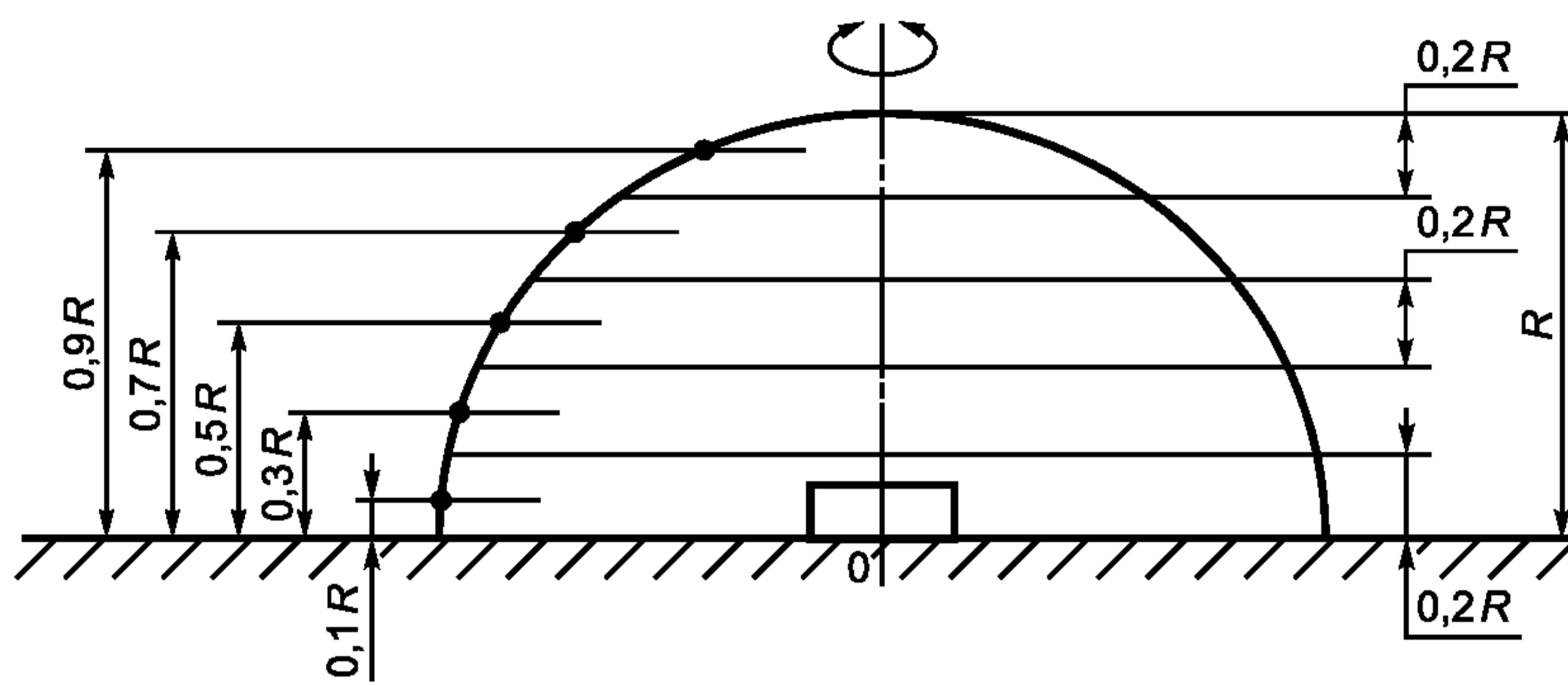
Рисунок А.2 — Соосные круговые траектории микрофона
