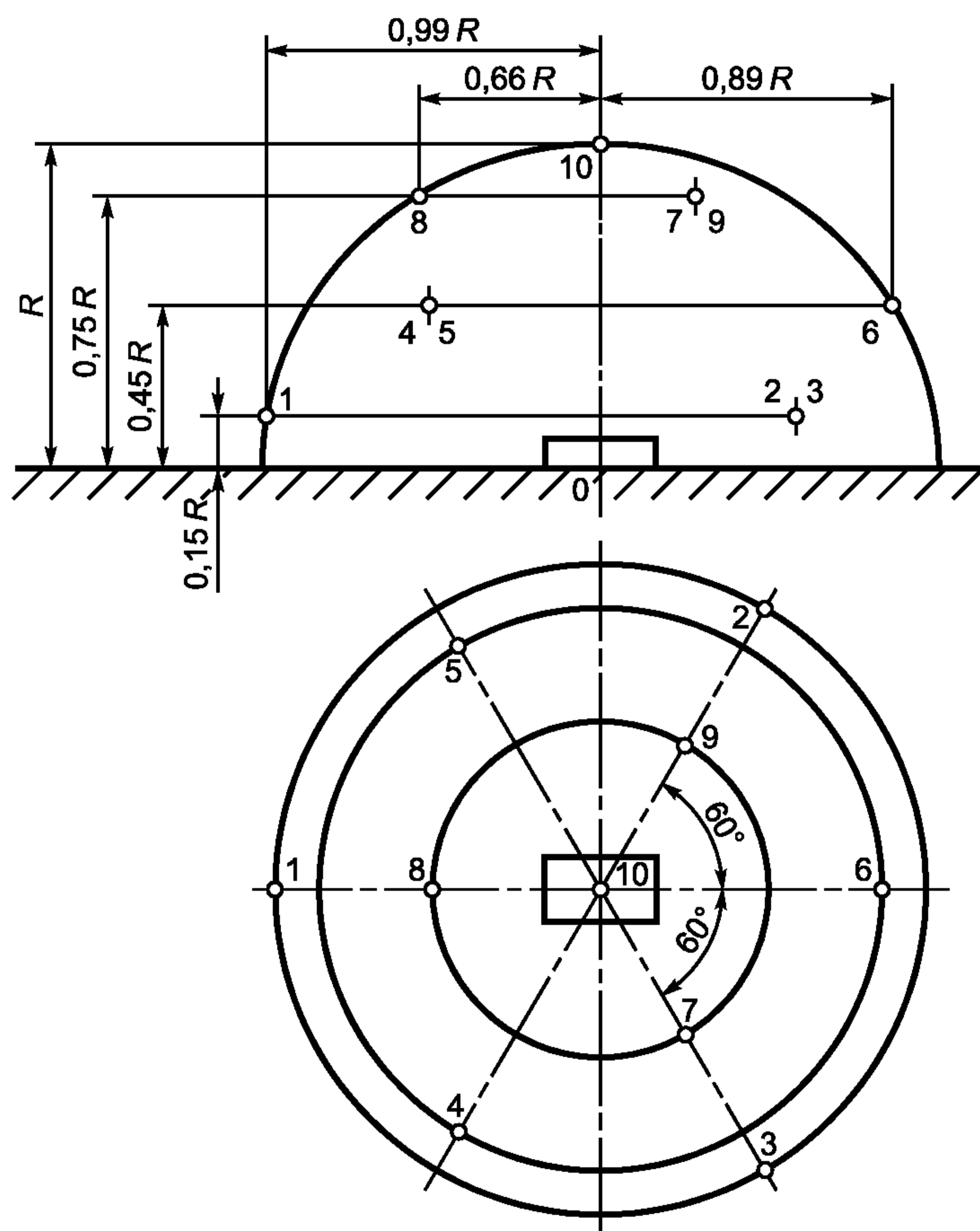
Рисунок А.1 — Положение микрофонов на полусфере
