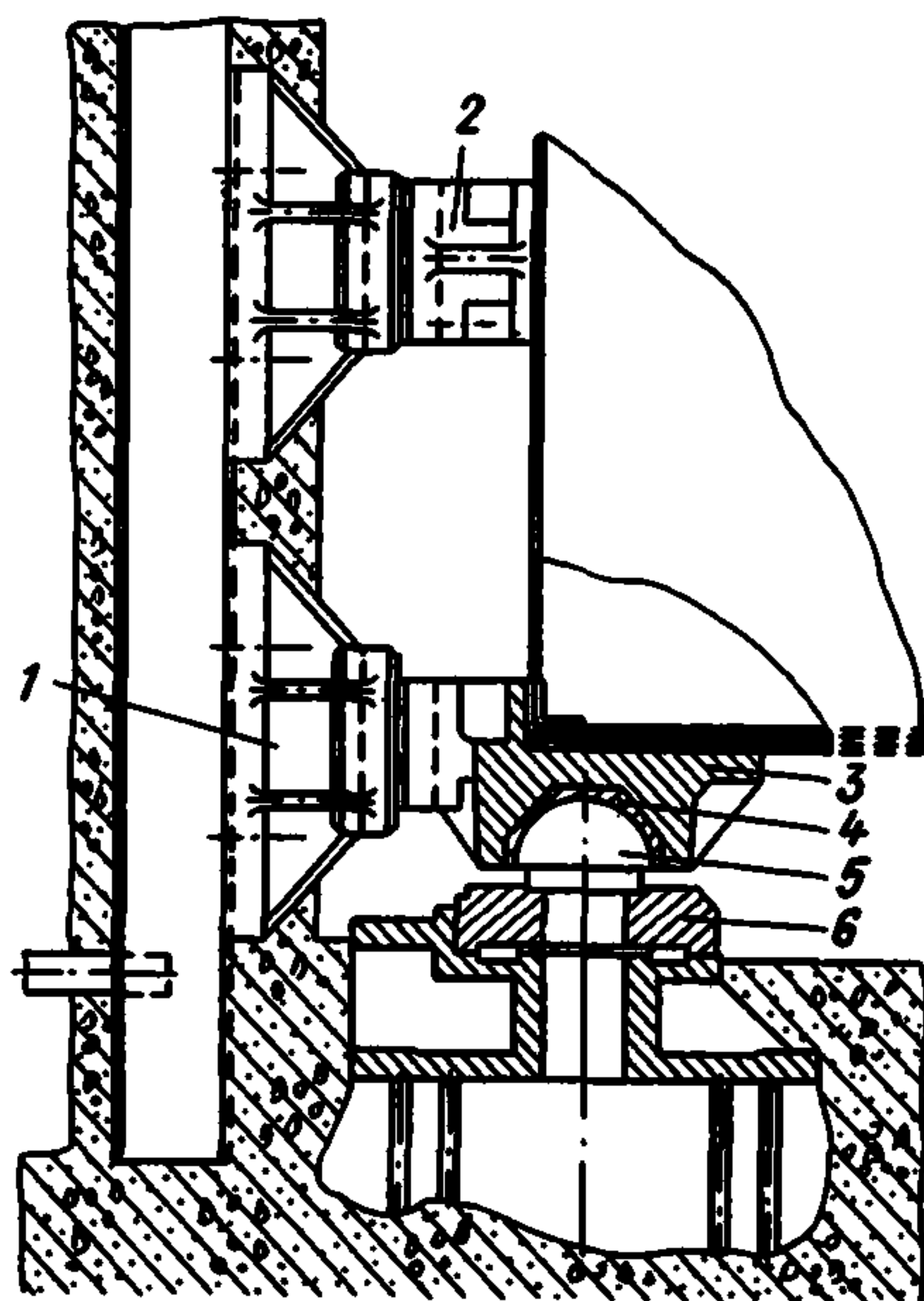
Рис. 2. Пятавое устройство ворот шлюза
