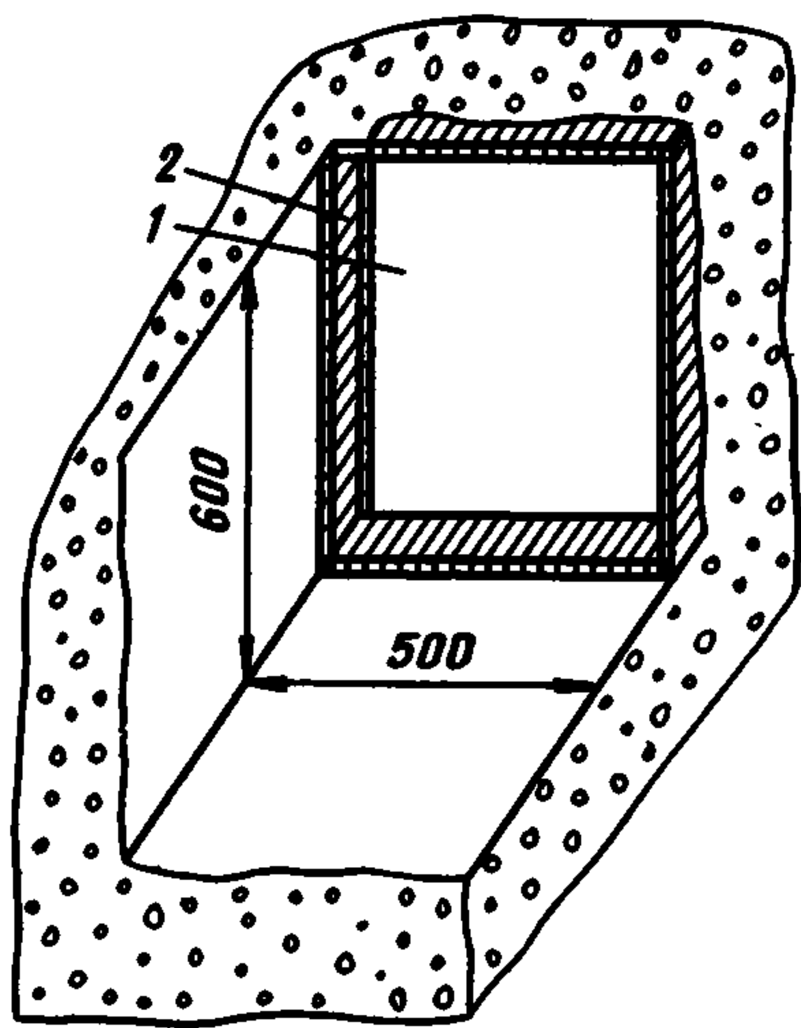
Рис. 11. Схема шпонок водопроводной галереи
