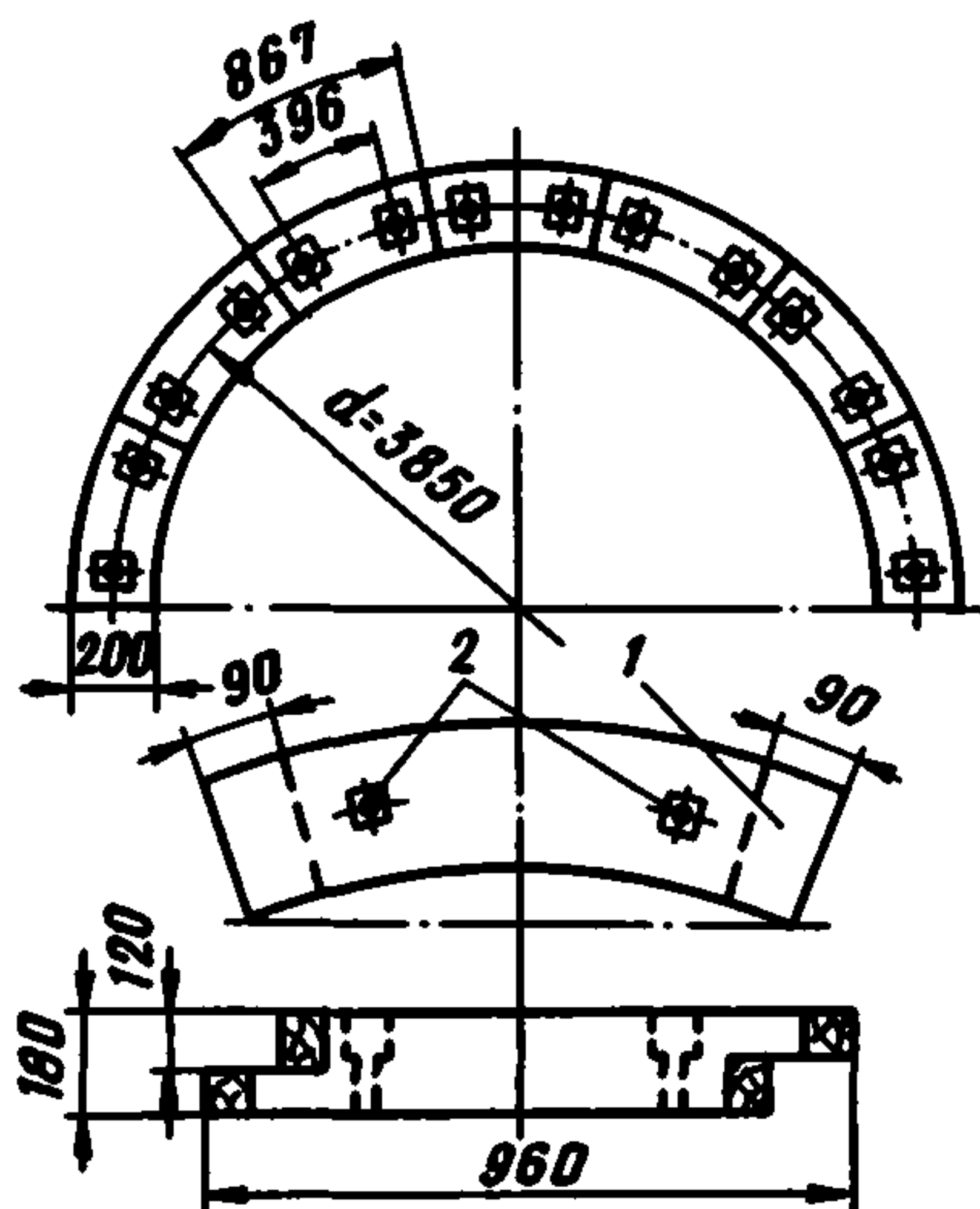
Рис. 9. Дубовое кольцо уплотнения
