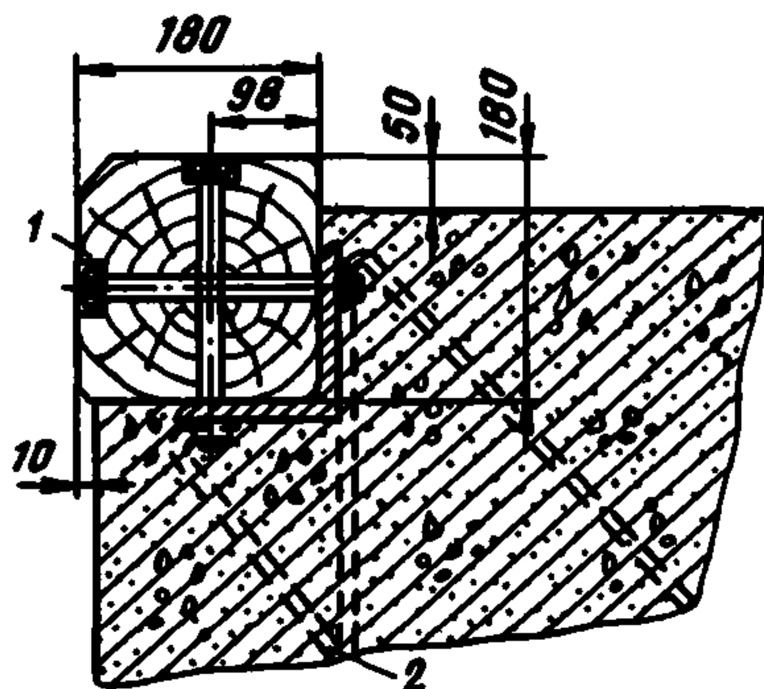
Рис. 7. Брус уплотнения порога короля
