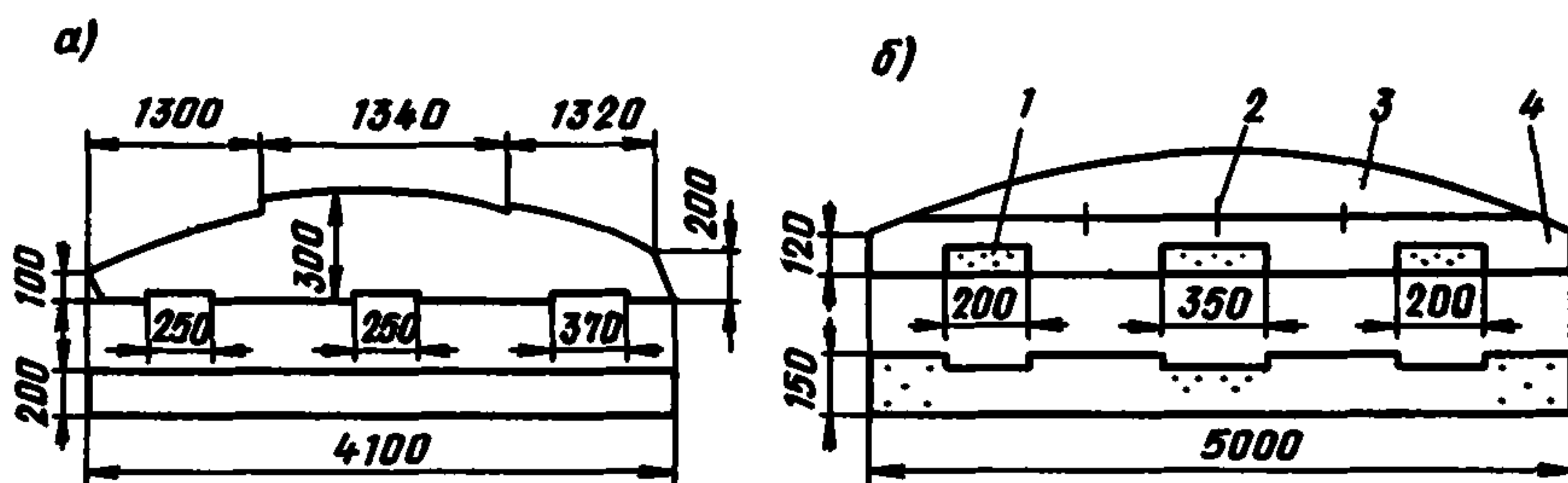
Рис. 6. Схемы шпангоутов. а — верхнего яруса; б — нижнего яруса: 1 — отверстия под заклепки, 2 — скобы для крепления брусьев, 3 — верхний брус, 4 — нижний брус
