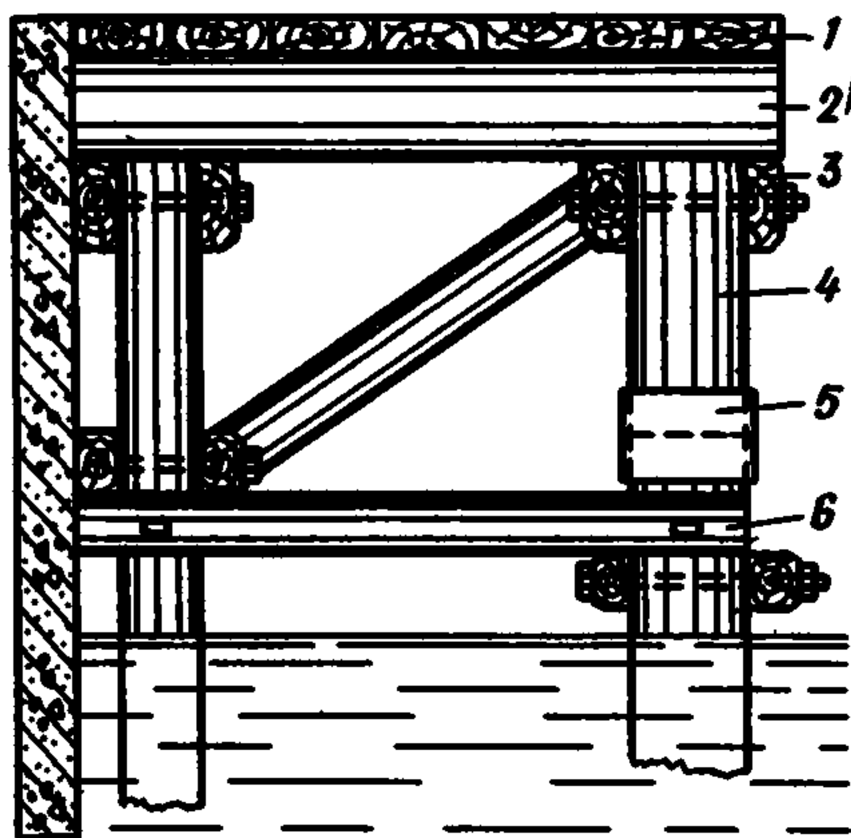
Рис. 28. Схема верхнего строения
