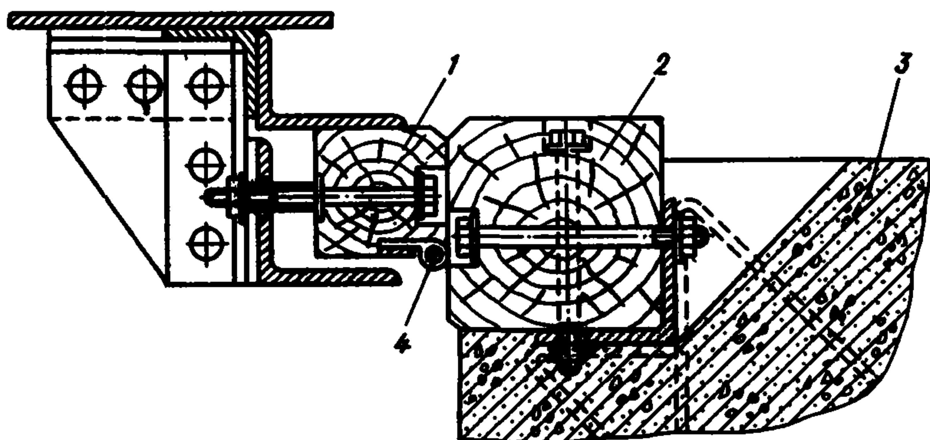
Рис. 4 Схема донного уплотнения
