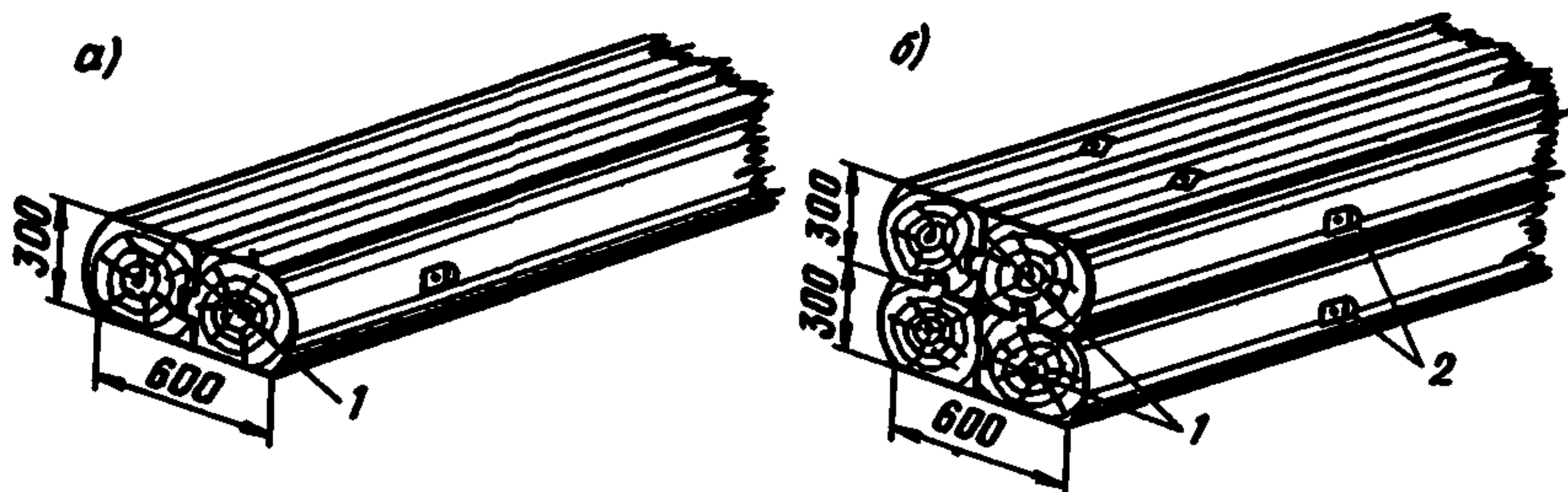
Рис. 17. Конструкции колод
