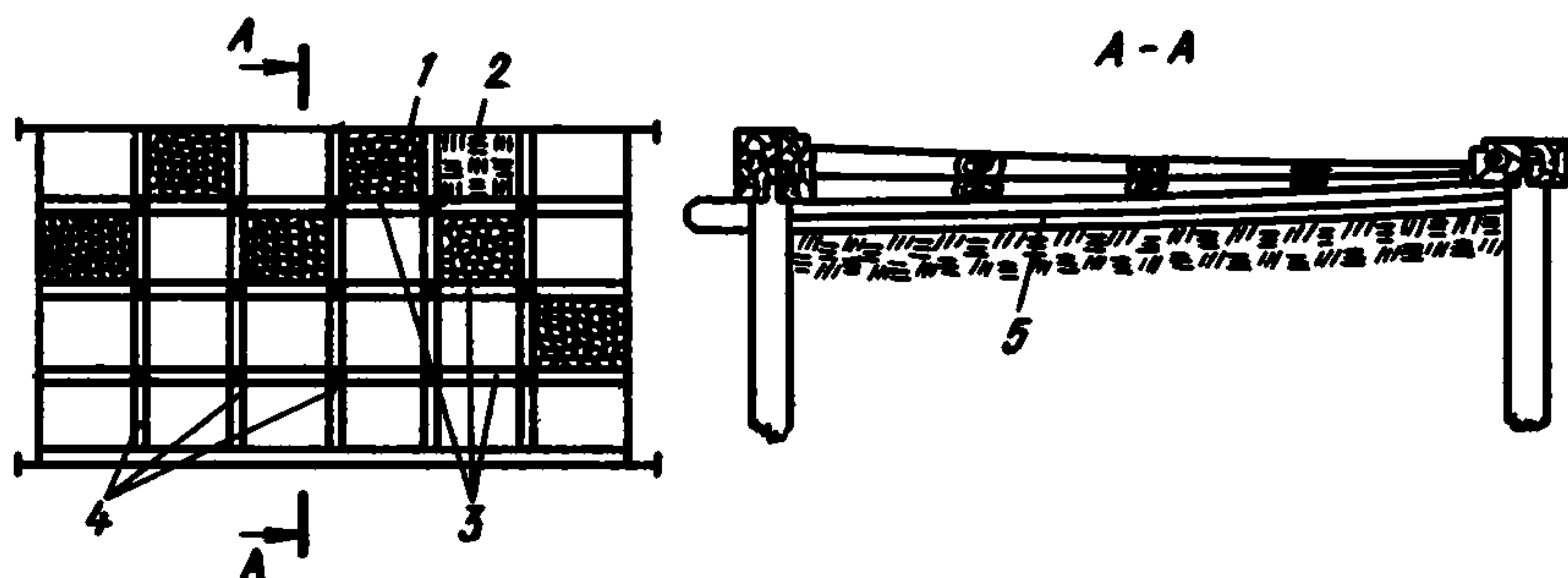
Рис. 24. Схема-ростверка
