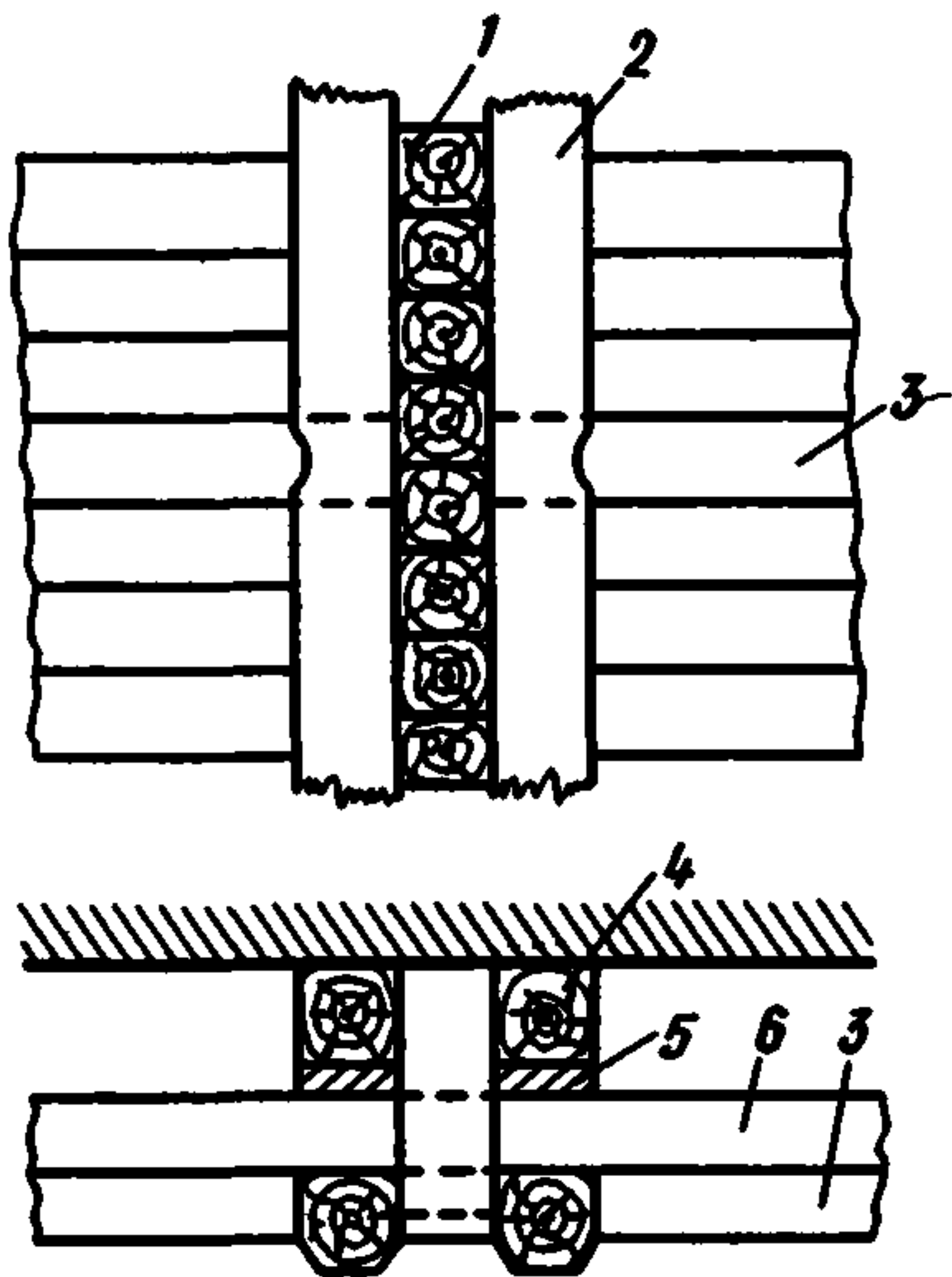
Рис. 22. Отбойная система, тип I
