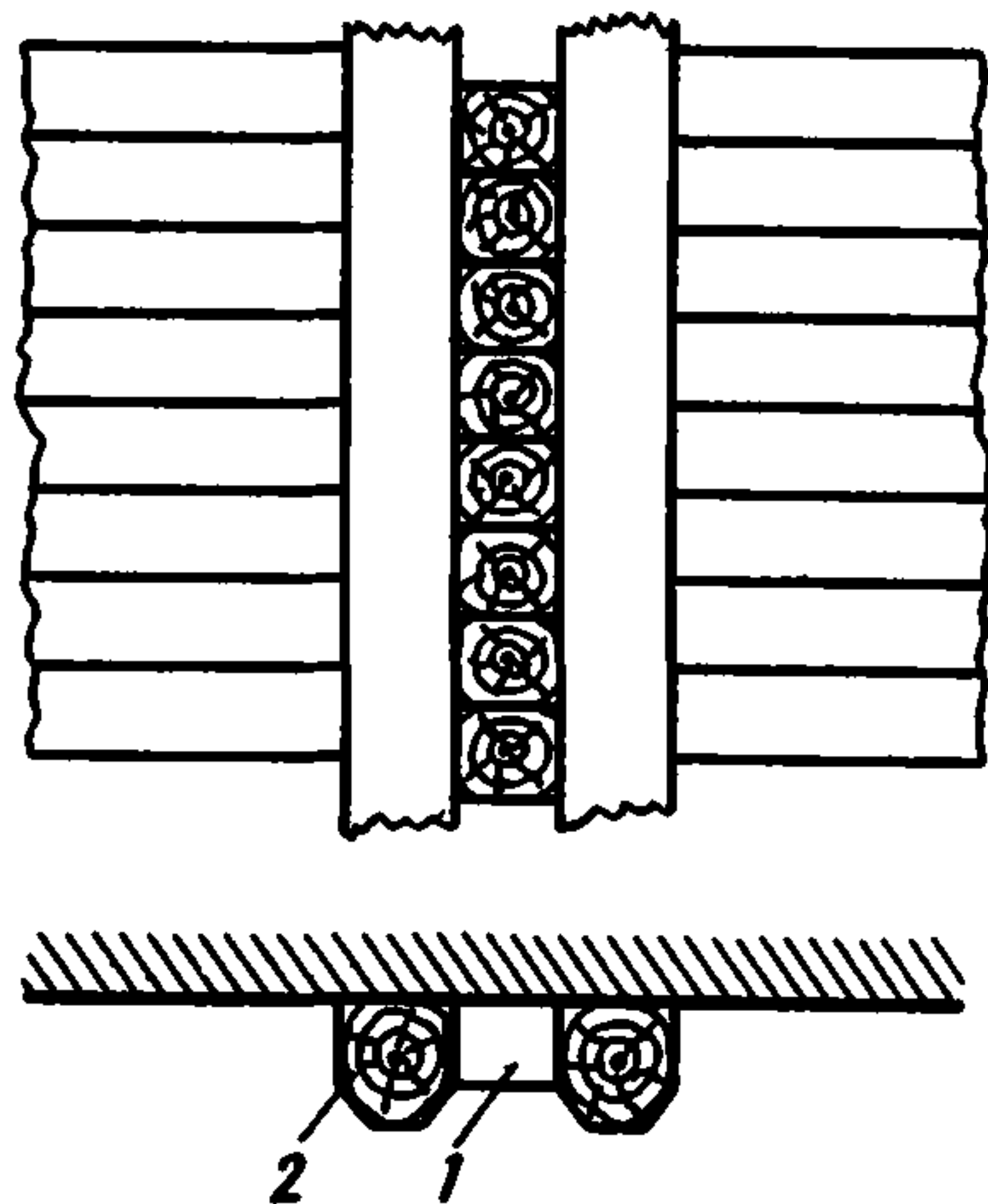
Рис. 23. Отбойная система, тип II
