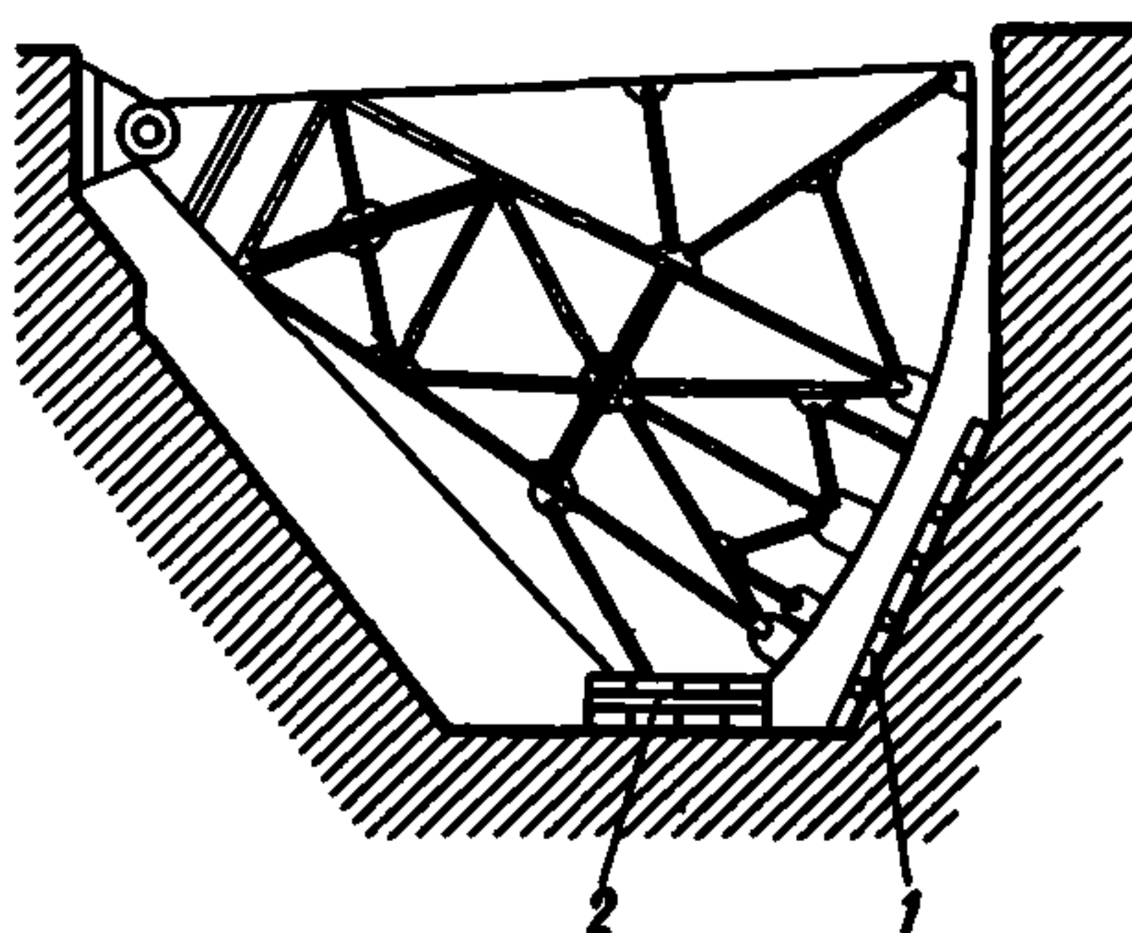
Рис 5. Схема рабочей зоны 1 — лестница; 2 — опорные клетки
