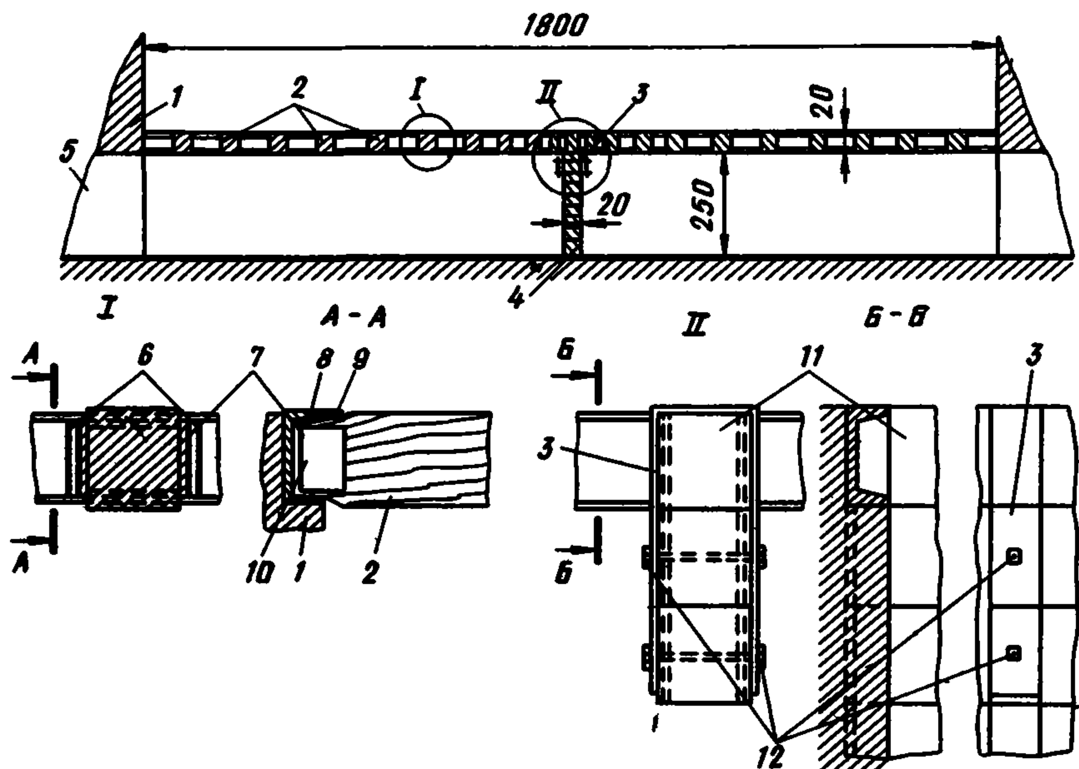
Рис. 10. Схема ниши гашения (разрезы)
