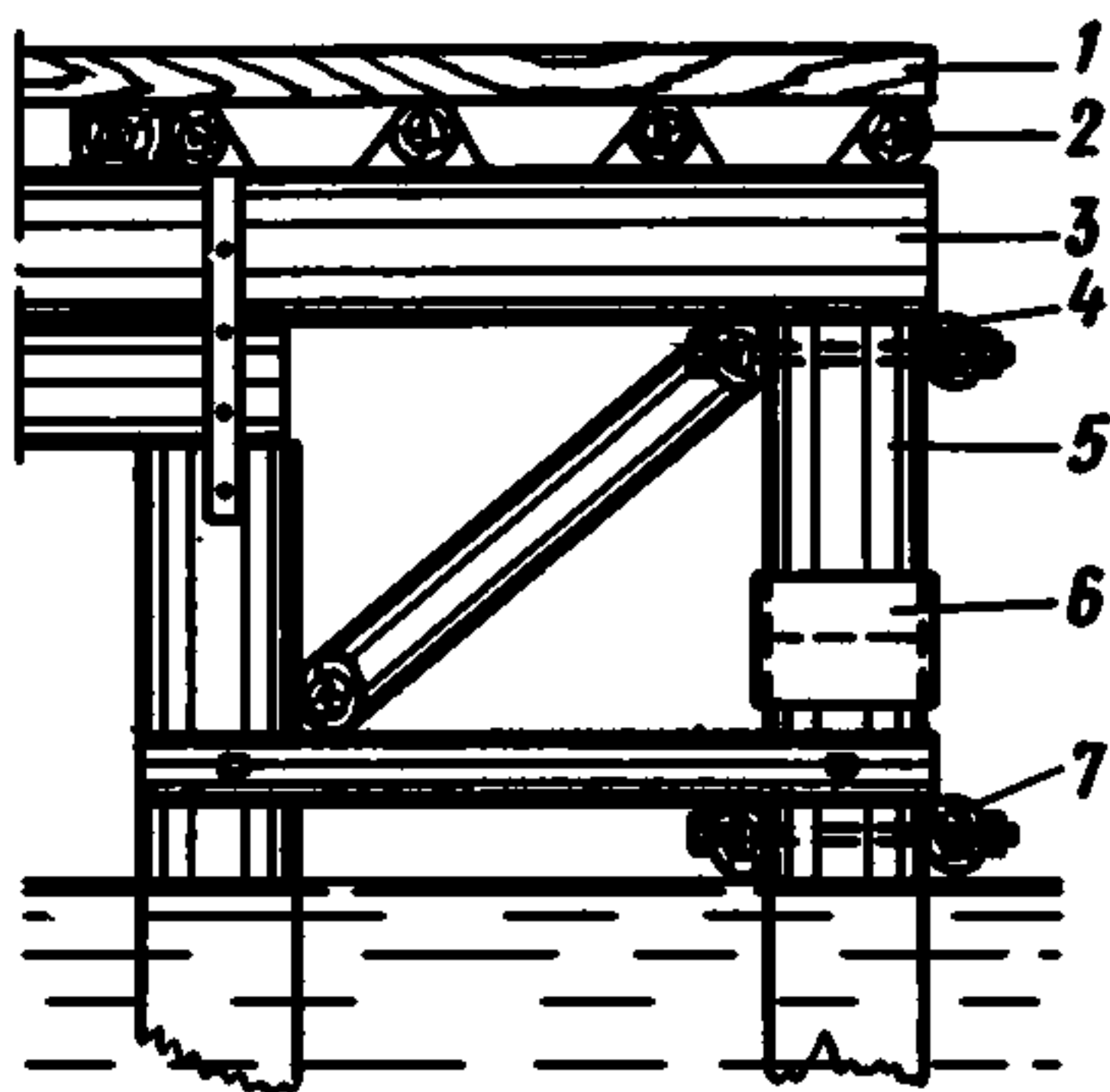
Рис 15. Схема поперечного настила 1 — настил, 2 — прогоны; 3 — насадки; 4 — верхние схватки, 5 — наросток; 6 — металлический стакан; 7 — нижние схватки
