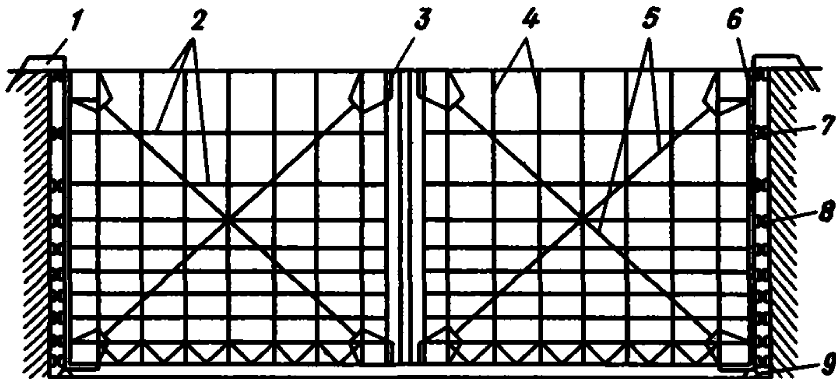
Рис 1 Схема двухстворчатых ворот шлюза
