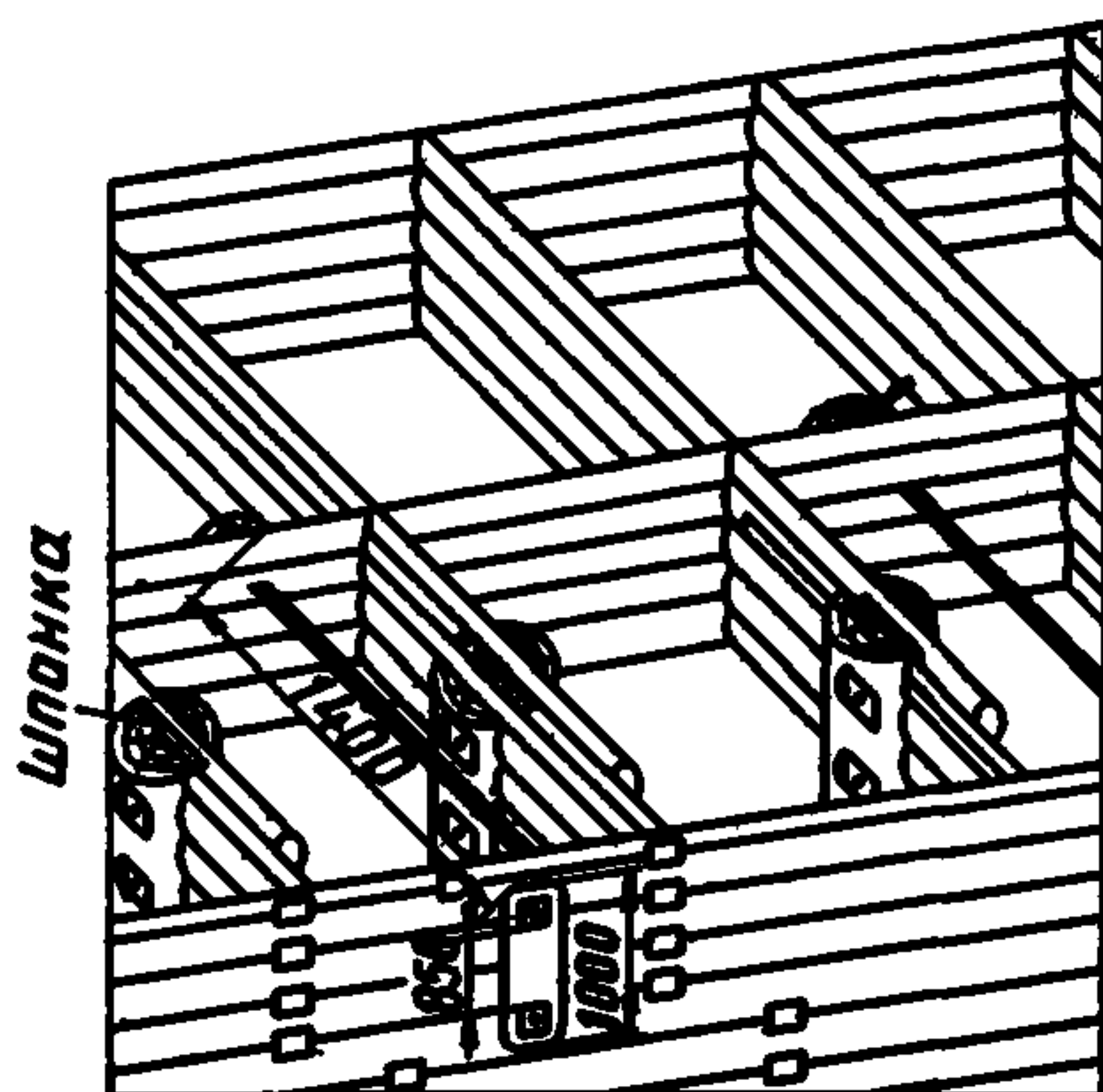
Рис. 19. Второй способ нарубki лицевых стен камеры шлюза
