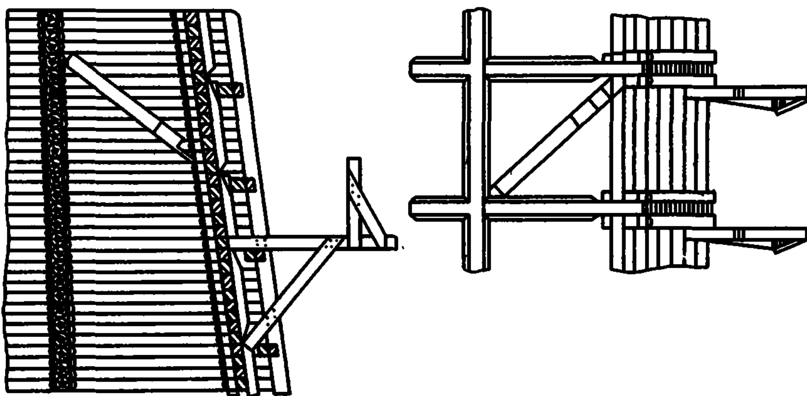
Рис. 29. Схема установки кронштейнов
