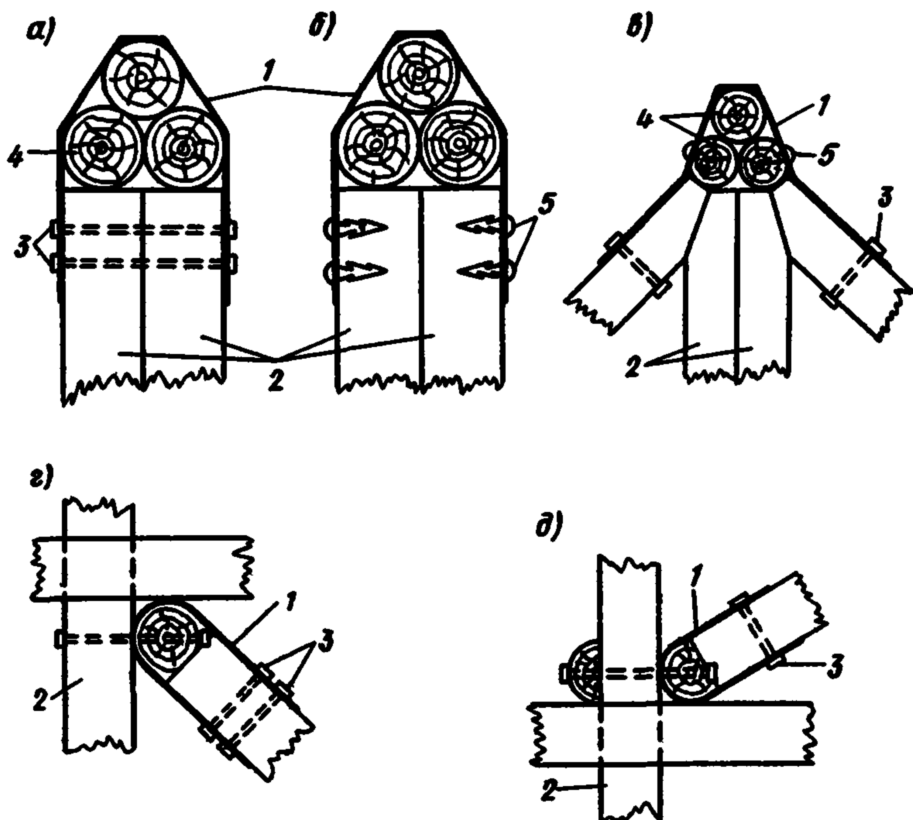
Рис. 26. Крепление хомута
