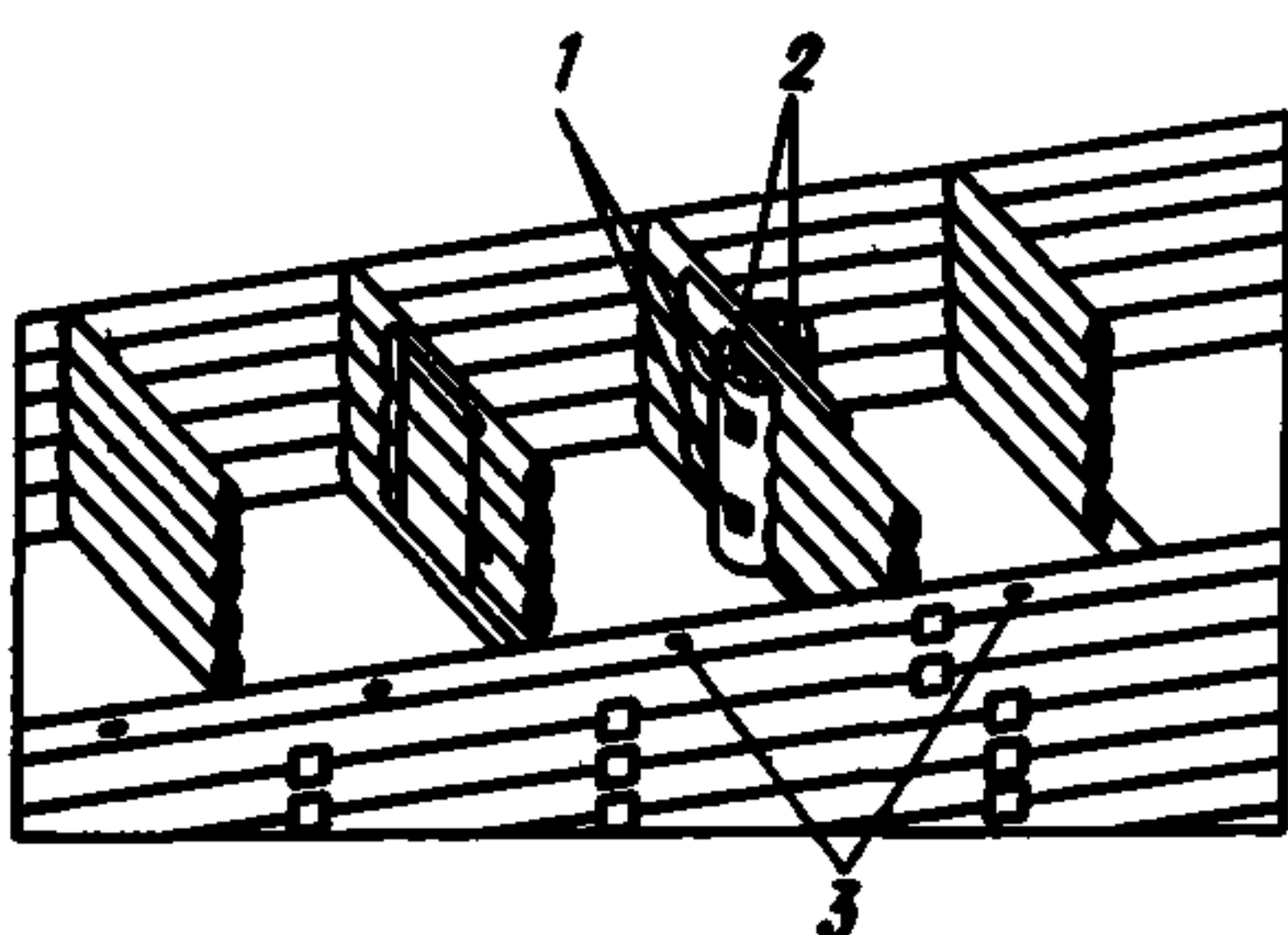
Рис. 18. Первый способ нарубki лицевых стен камеры шлюза
