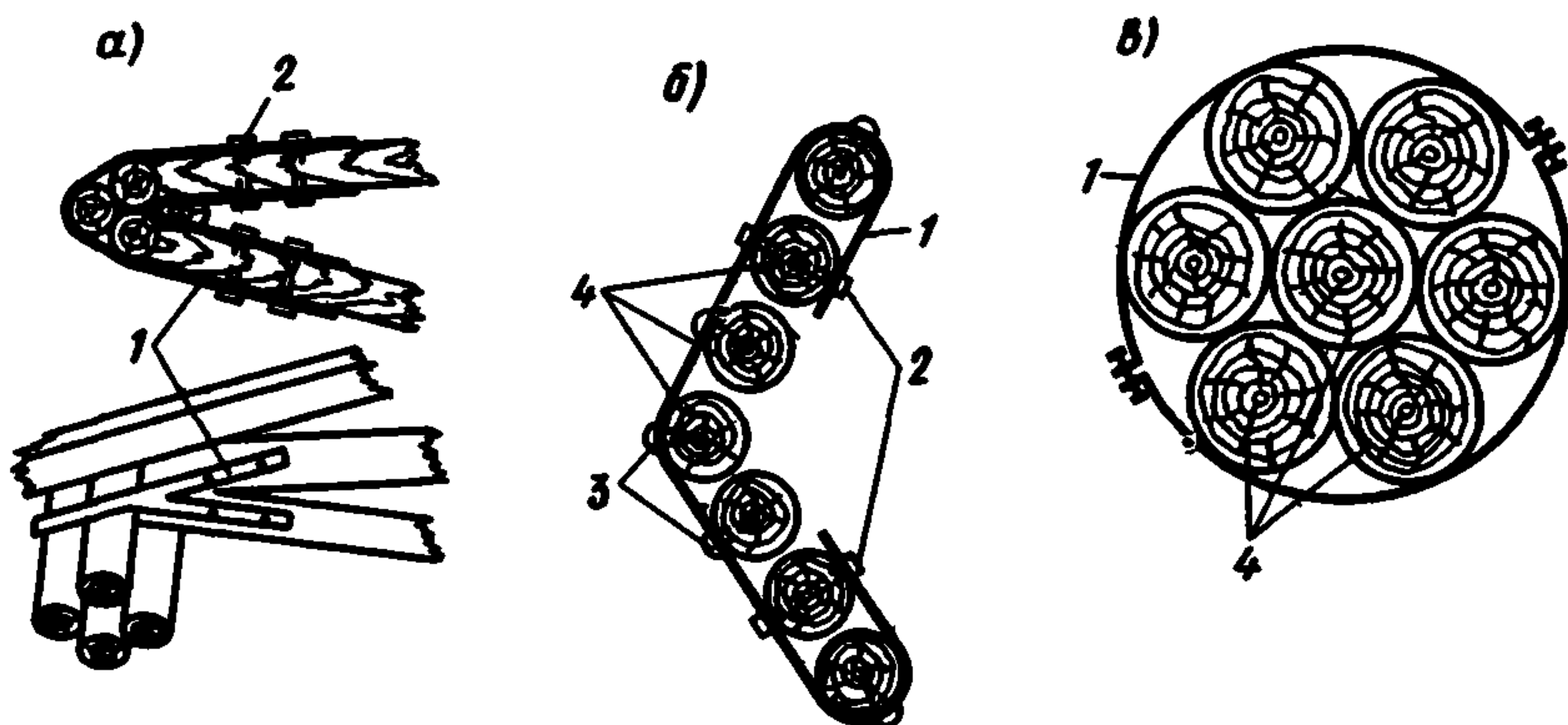
Рис. 25. Установка хомута а — на восьми болтах; б — на двух болтах и пяти штырях; в — разъемного на двух стяжных болтах 1 — хомуты; 2 — болты; 3 — штыри; 4 — сваи
