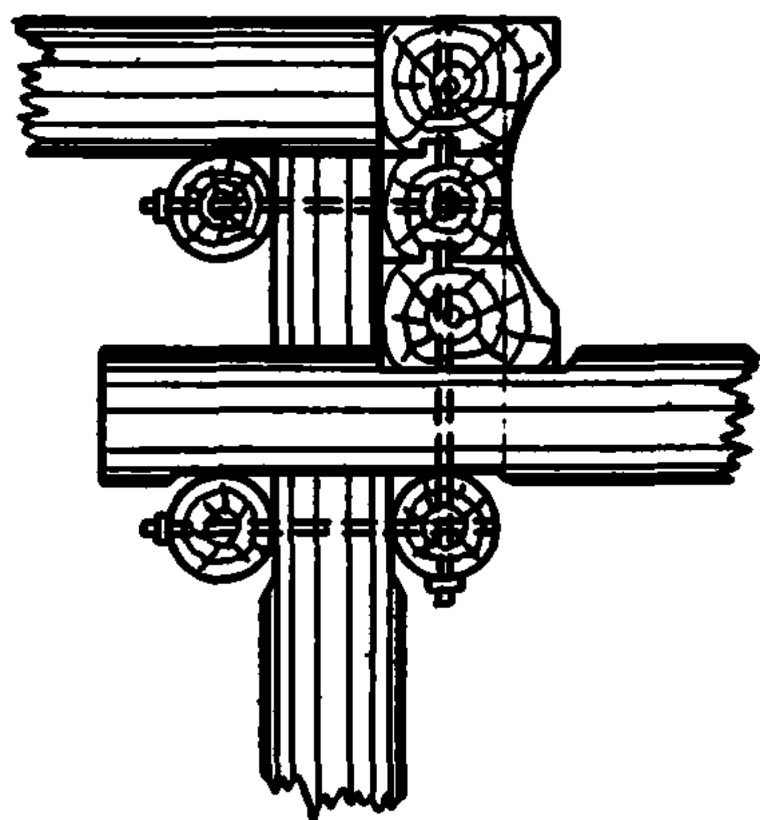
Рис. 14. Схема крепления веревального столба
