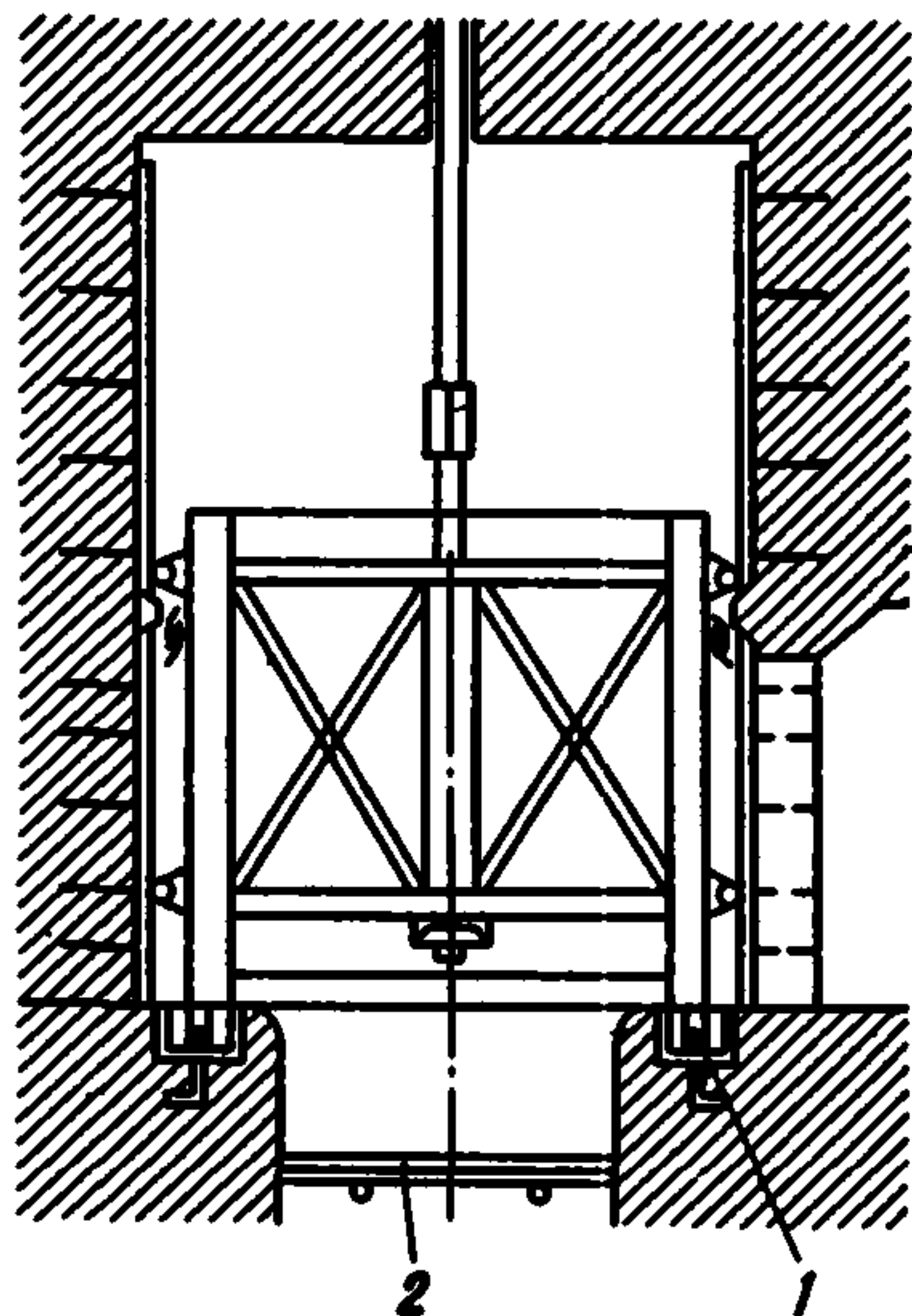
Рис. 8. Схема цилиндрического затвора
