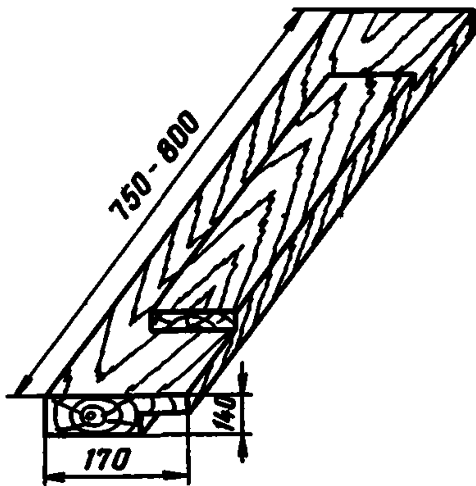
Рис. 12. Шпоночный вкладыш
