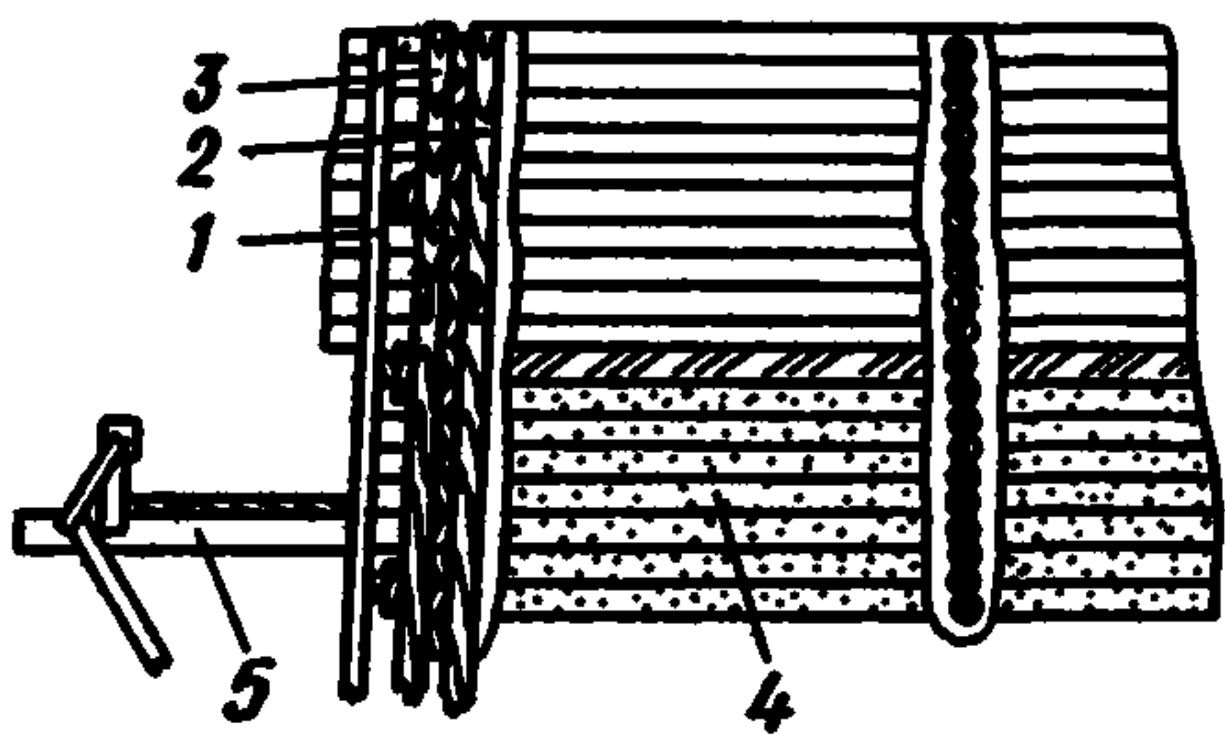
Рис. 20. Схема верхней части ряжевых стен шлюза 1 — отбойная стойка, 2 — внутренний сжим, 3 — наружный сжим, 4 — засыпка; 5 — леса на кронштейнах
