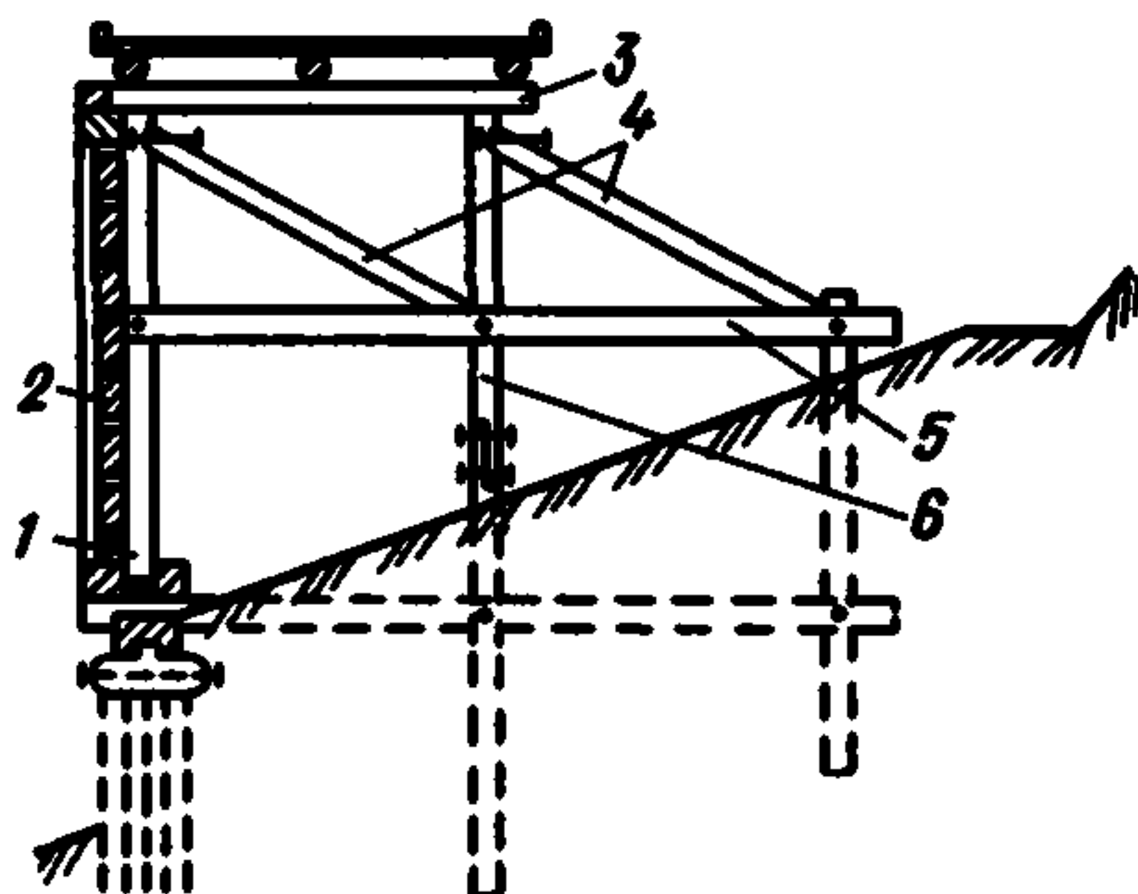
Рис. 27. Поперечный разрез эстакады
