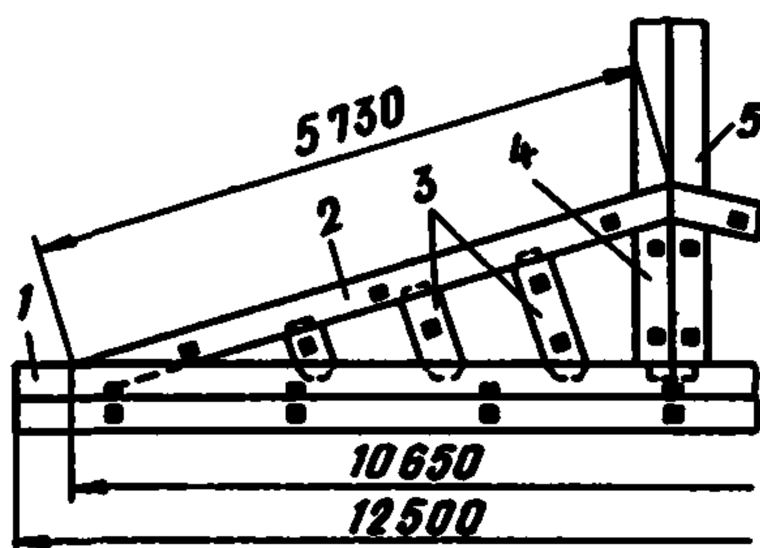
Рис 16. План королевской колоды
