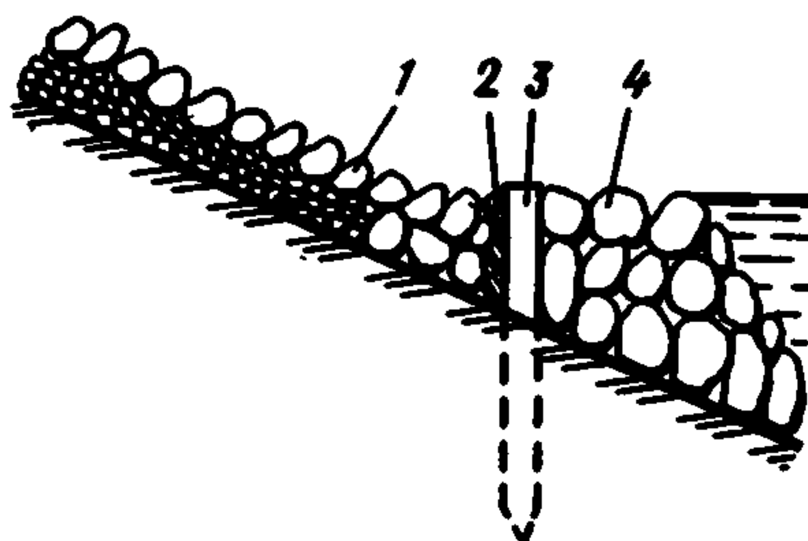
Рис. 13 Поперечный разрез забирки
