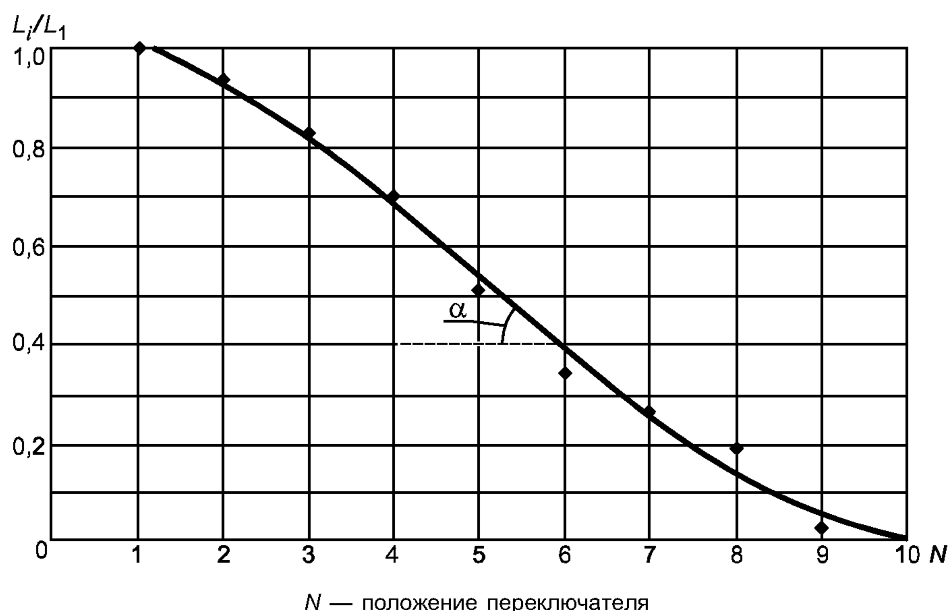
Рисунок 4 — Изменение яркости излучения экранов от регулировки
