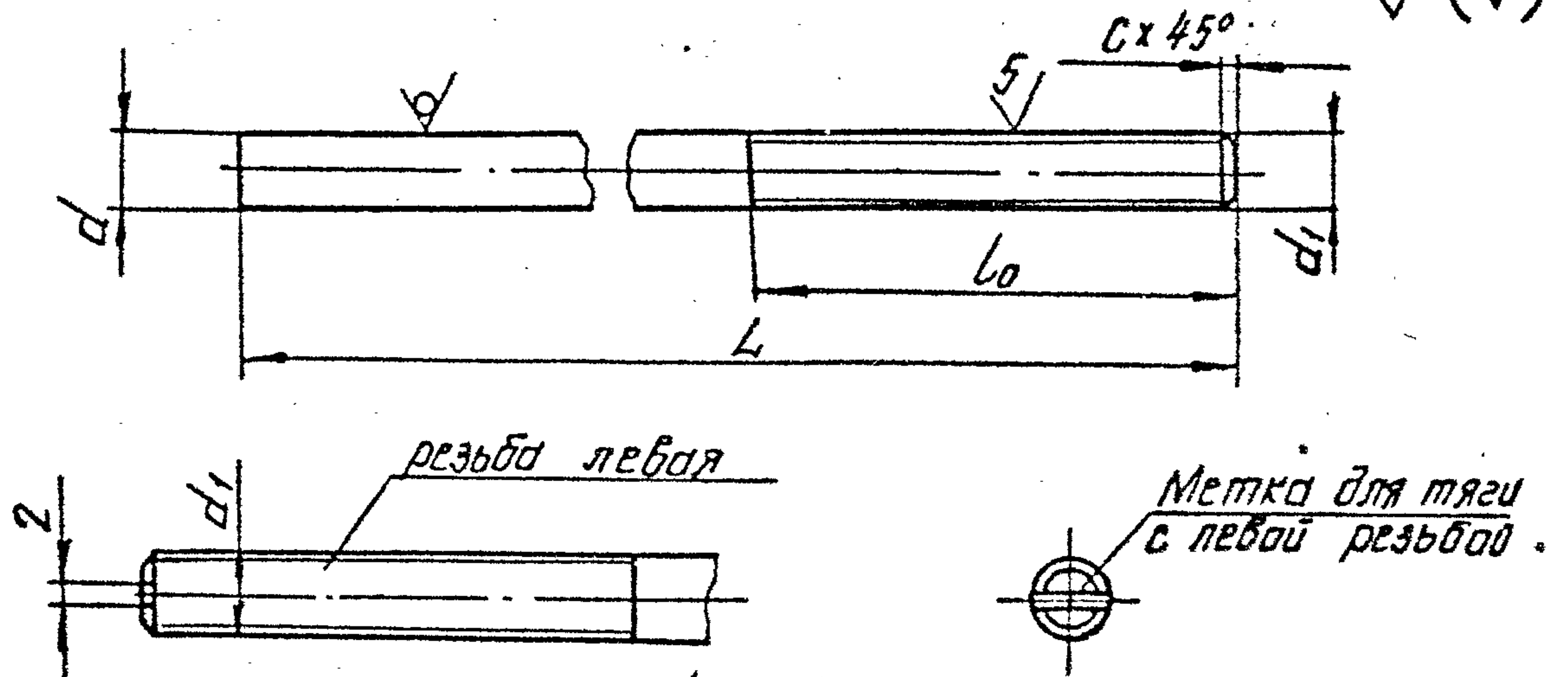
Черт. 6 С правой резьбой Размеры в мм
